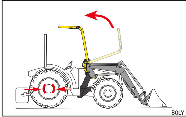
Ábr. 55 OPG felhajtása
