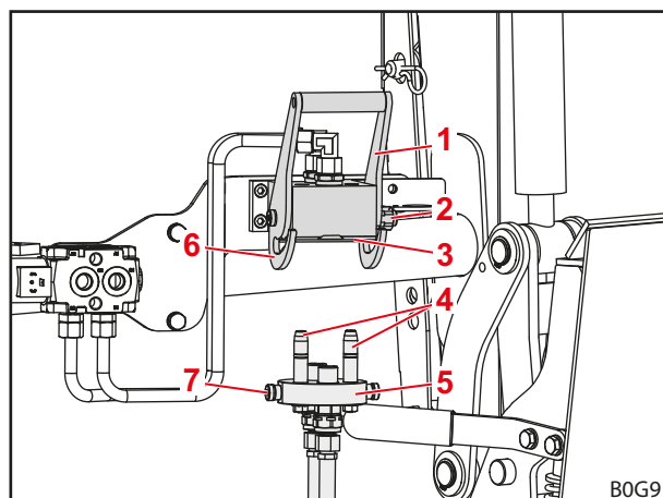
Ábr. 72 Lekapcsolt munkaeszköz-rögzítés
