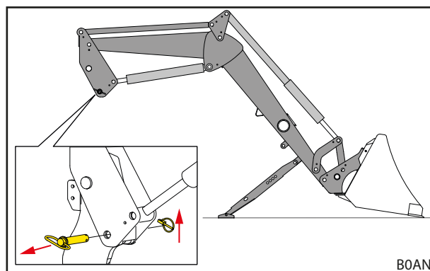
Ábr. 52 Homlokrakodó rögzítő-mechanizmusának kinyitása
