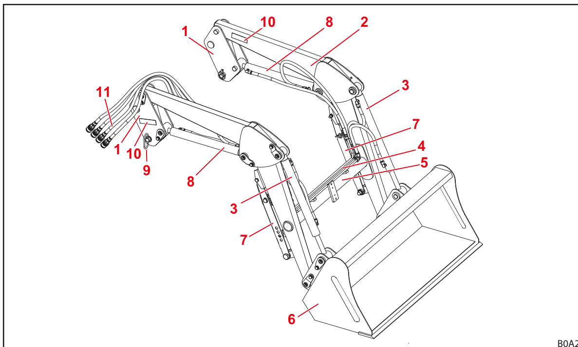
Ábr. 9 L homlokrakodó (példálózó ábra)
