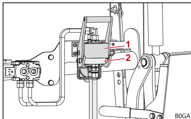
Ábr. 73 Felkapcsolt munkaeszköz-rögzítés
