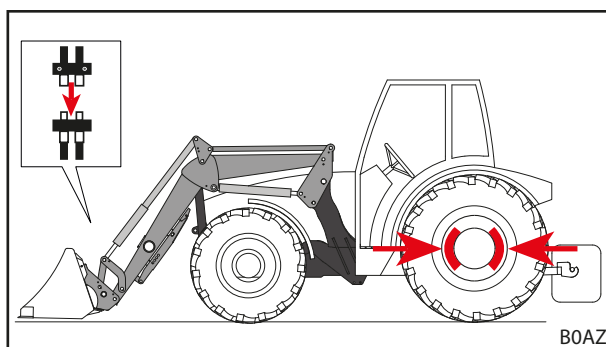
Ábr. 98 Hidraulikakör csatlakoztatása
