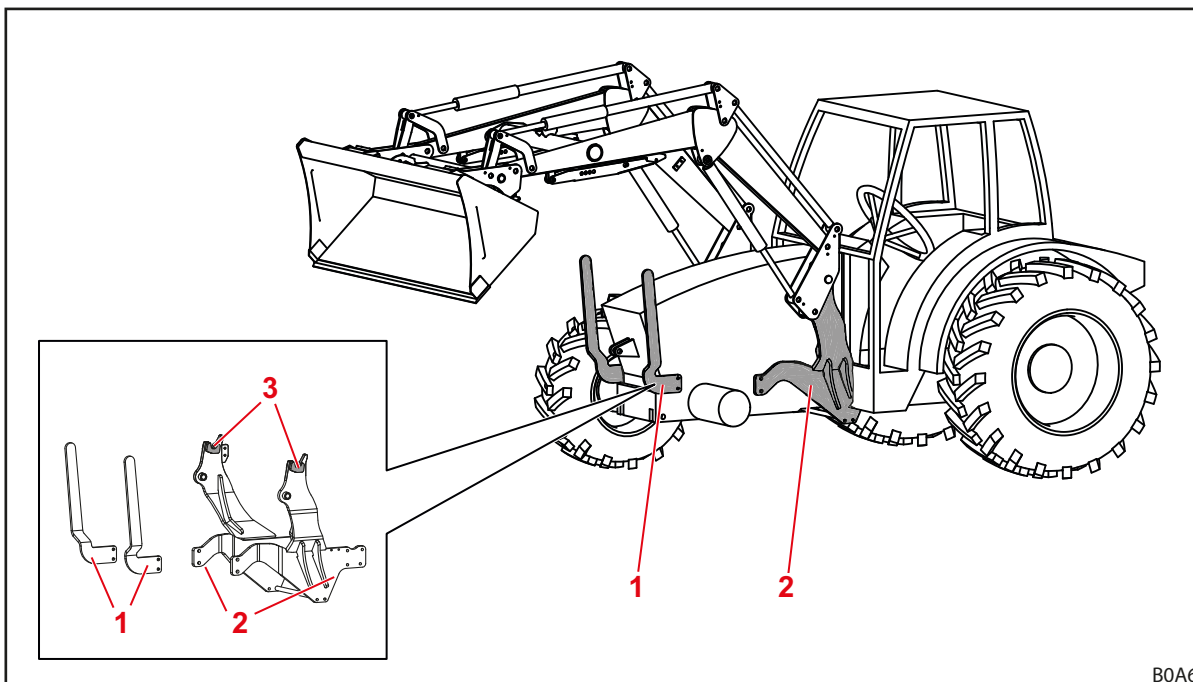
Ábr. 15 Traktor felszerelő készlete
