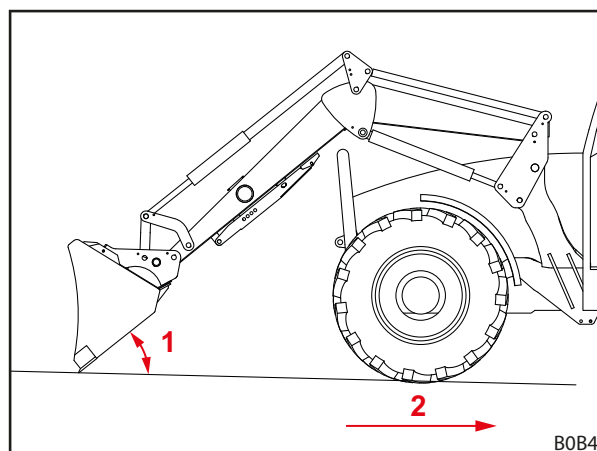
Ábr. 107 Talajegyengetés hátrafelé
