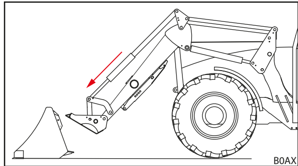
Ábr. 85 Gémszerkezet pozicionálása
