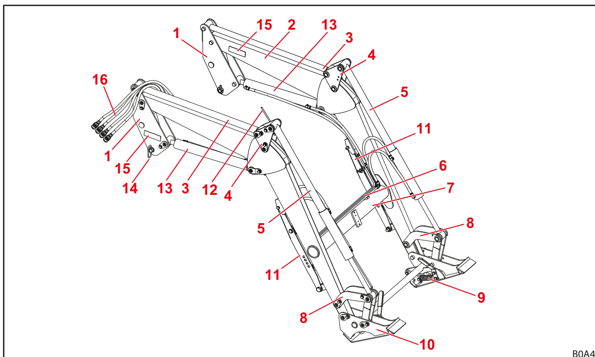
Ábr. 11 Homlokrakodó P (példálózó ábra)
