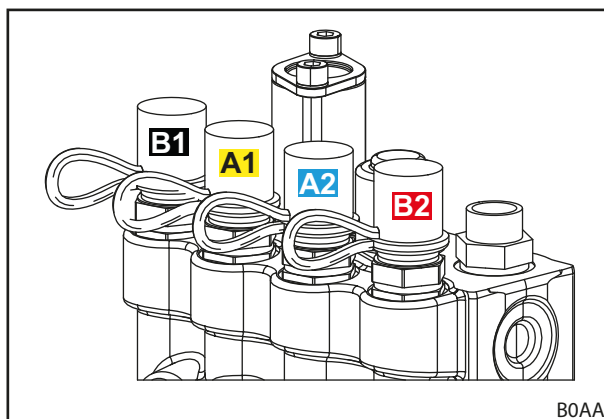
Ábr. 20 Dugós csatlakozók csatlakozója, közvetlenül a hidraulikaszelepen
