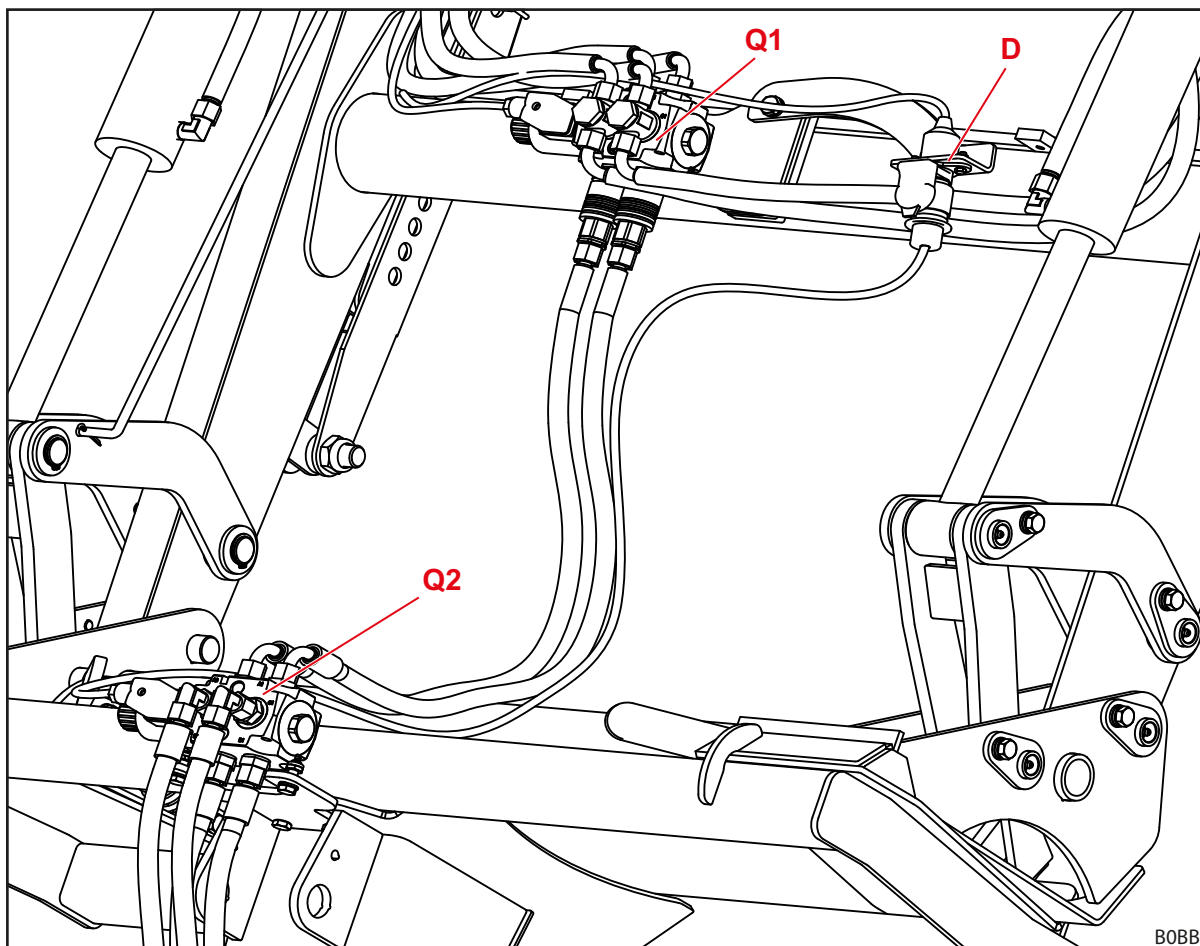
Ábr. 124 Hidraulikus szelepek elrendezése a kiegészítő funkciókhoz
