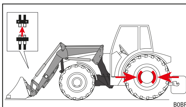
Ábr. 100 Hidraulikavezetékek kioldása
