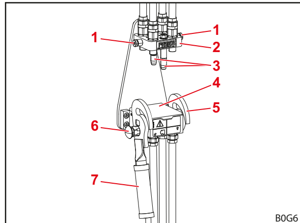
Ábr. 70 Lekapcsolt Hydro-Fix
