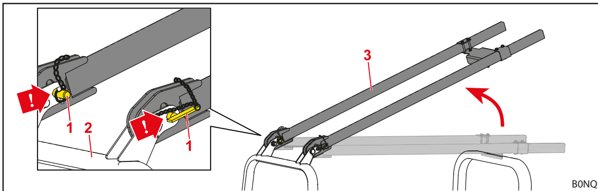
Ábr. 40 Felhajtott és az alsó lyukakban biztosított kereszttartók
