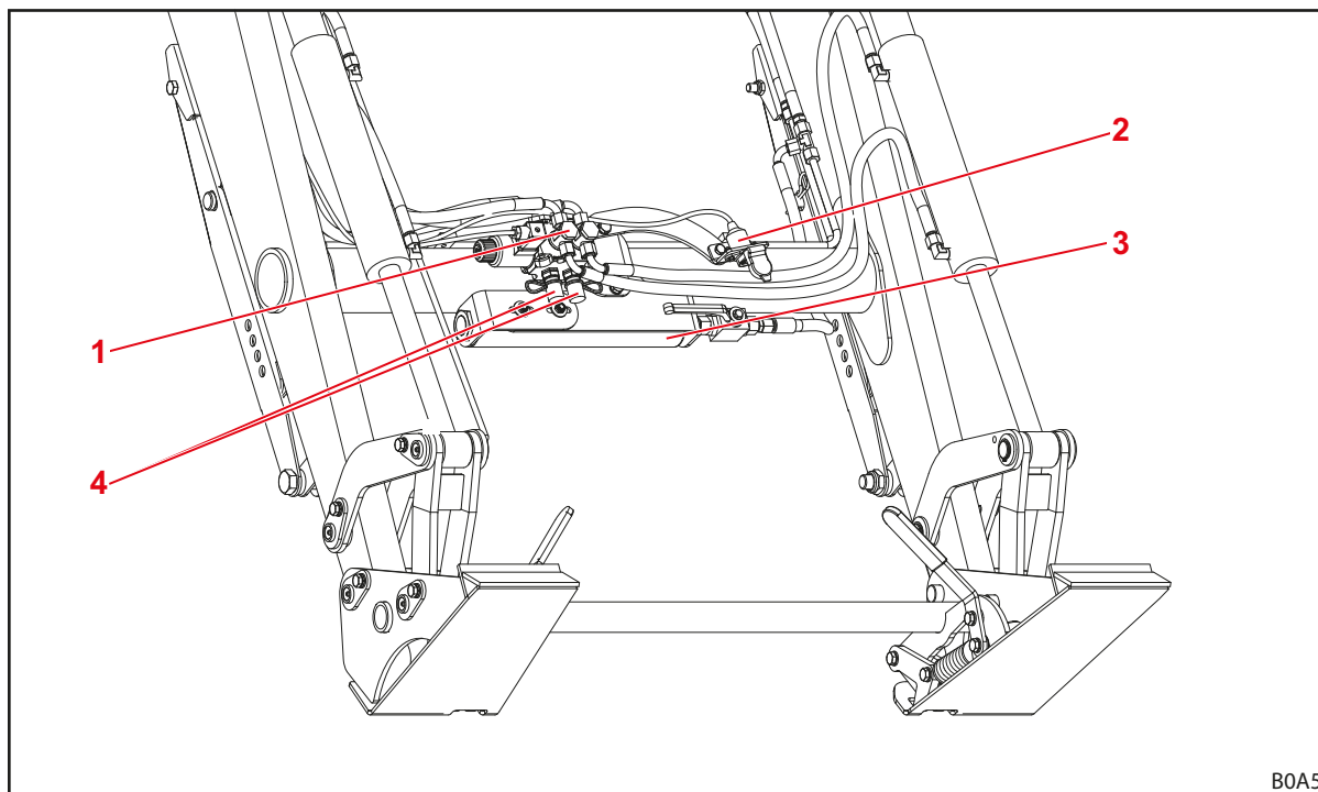
Ábr. 14 Az L, H és P homlokrakodók kiegészítő felszerelése (példálózó ábra)
