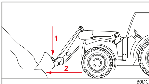
Ábr. 109 Homlokrakodó lesüllyesztése és egyenes bejárás a rakodni kívánt anyagba
