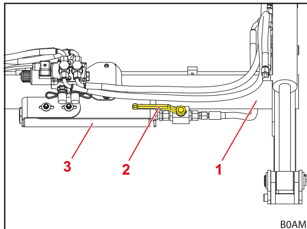
Ábr. 47 Mechanikus működtetésű Comfort-Drive (Comfort-Drive be karállás)
