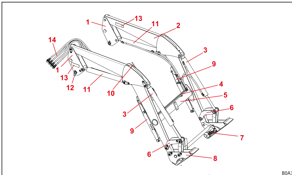
Ábr. 10 H homlokrakodó (példálózó ábra)
