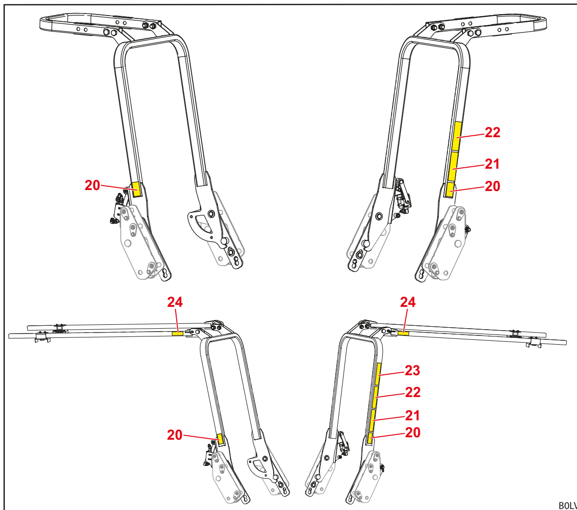
Ábr. 6 OPG hátul elhelyezett 2 cölöpös borulás elleni védelemmel ellátott traktorokhoz (példálózó ábra)
