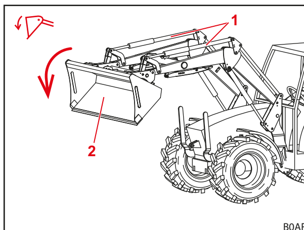
Ábr. 31 Kibillentés funkció
