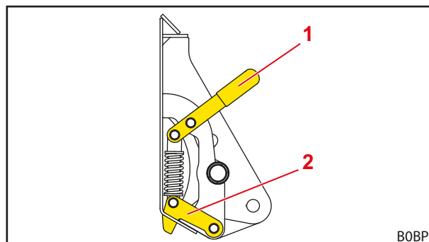
Ábr. 75 Skid-Steer mechanikus munkaeszköz-reteszélése (félig nyitott állapot)
