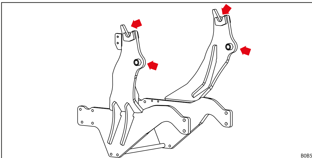
Ábr. 113 Homlokrakodó-tartók kenési pontjai
