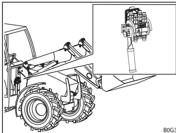
Ábr. 21 Hydro-Fix: elhelyezkedés a homlokrakodón
