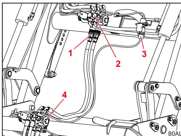
Ábr. 46 További 4. hidraulikakör
