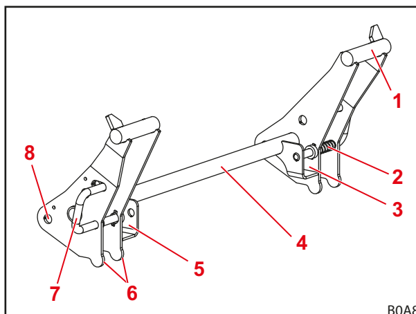
Ábr. 17 Euro-csatlakozókeret
