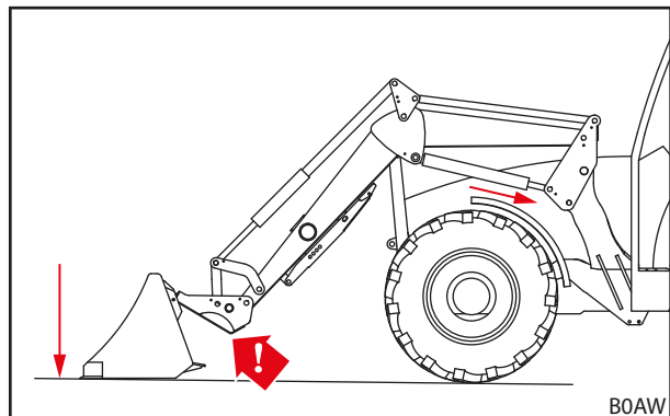
Ábr. 79 Nyomja a munkaeszkőzt a talajra
