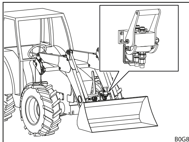
Ábr. 23 Munkaeszköz-rögzítés: elhelyezkedés a homlokrakodón
