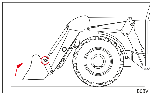
Ábr. 96 A munkaeszköz fenti összekapcsolása a hidraulikus munkahengerekkel
