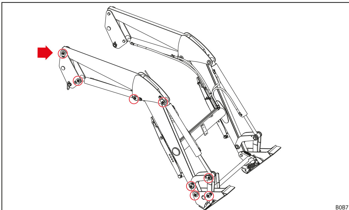
Ábr. 115 H kenési pontjai
