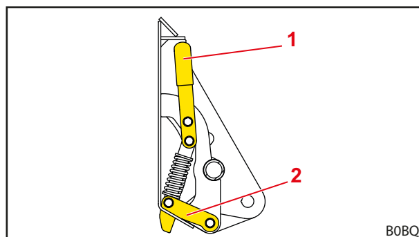
Ábr. 76 Skid-Steer mechanikus munkaeszköz-reteszélése (reteszelt állapot)
