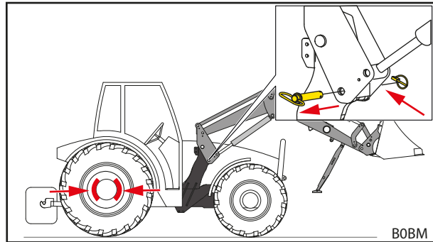
Ábr. 118 Húzza be a kéziféket, és oldja ki a homlokrakodó-reteszelést.
