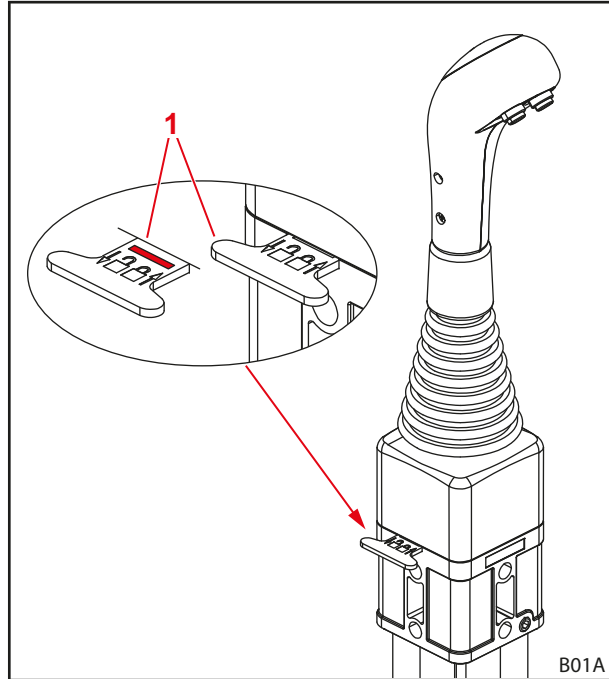
Ábr. 61 A vezérlőkar reteszelése
