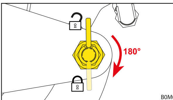
Ábr. 37 A rögzítőreteszt állítsa beretteszelt helyzetbe.
