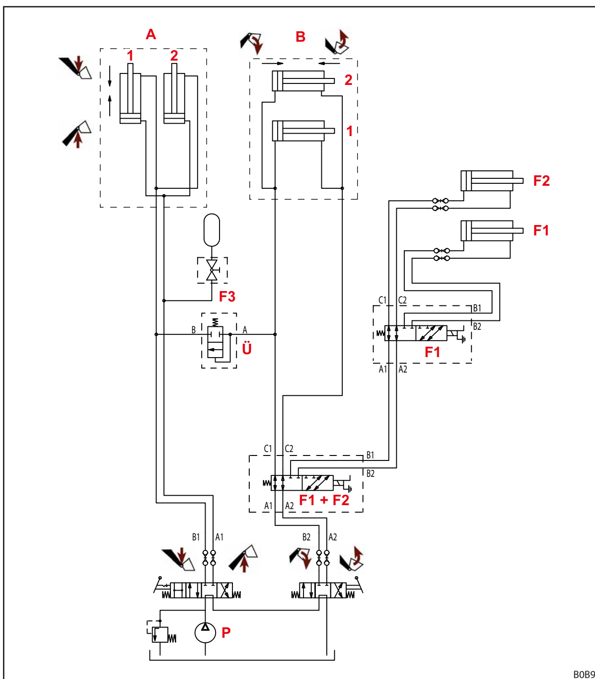
Ábr. 122 Hidraulikaterv FC
