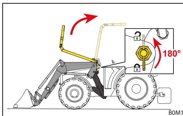
Ábr. 38 OPG felhajtása
