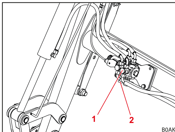
Ábr. 45 További 3. hidraulikakör
