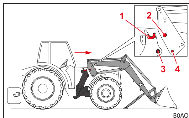
Ábr. 53 Vezesse be a traktort a gémszerkezetre.
