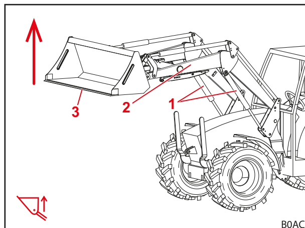
Ábr. 28 Emelés funkció
