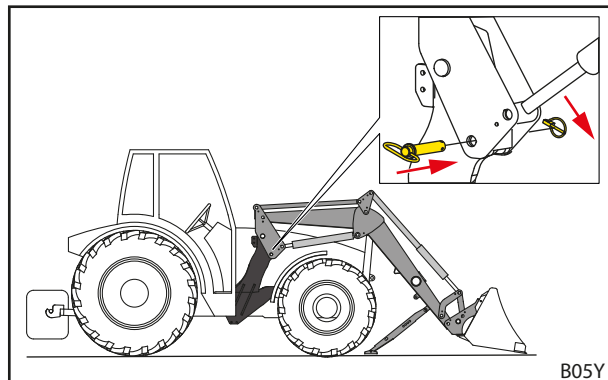
Ábr. 56 Dugja be a reteszelő csapszeget, és biztosítsa a rugós csatlakozóval
