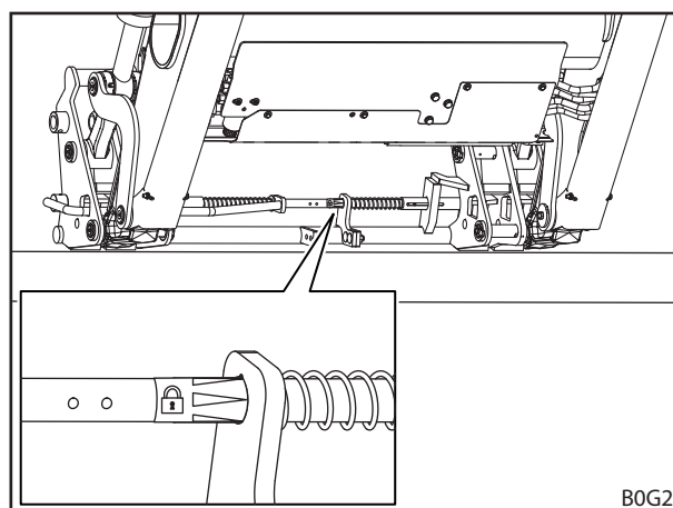
Obr. 84 Kontrola zamykacího mechanismu nářadí podle nálepky (kombinovaný výměnný rám Euro-FR)
