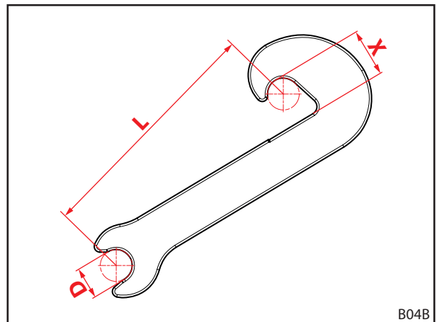
Obr. 118 Míra opotřebení závěsného háku
