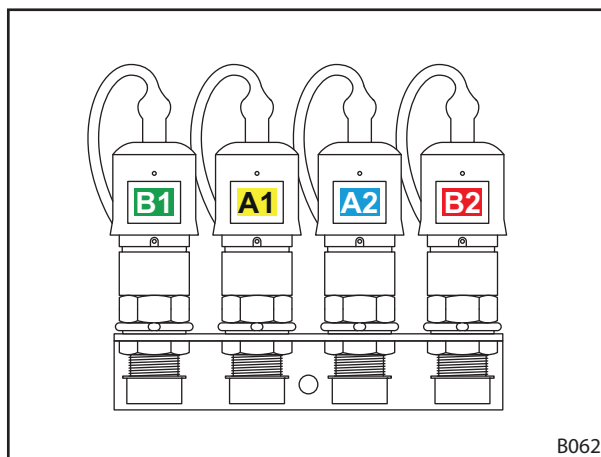
Obr. 23 Připojené rychlospojky
