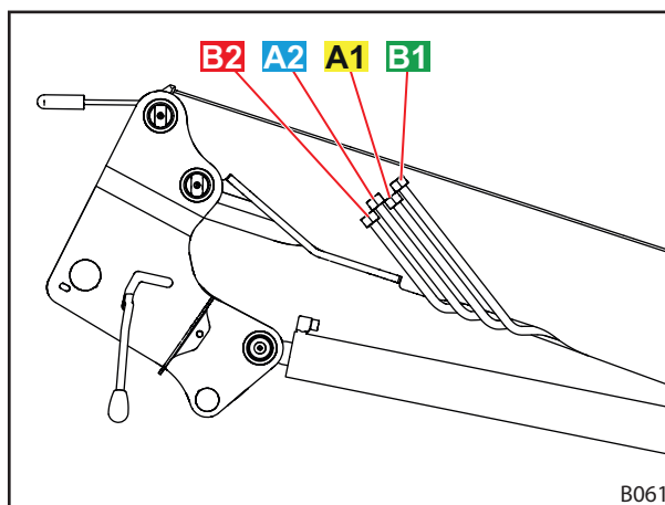
Obr. 22 Hydraulická vedení
