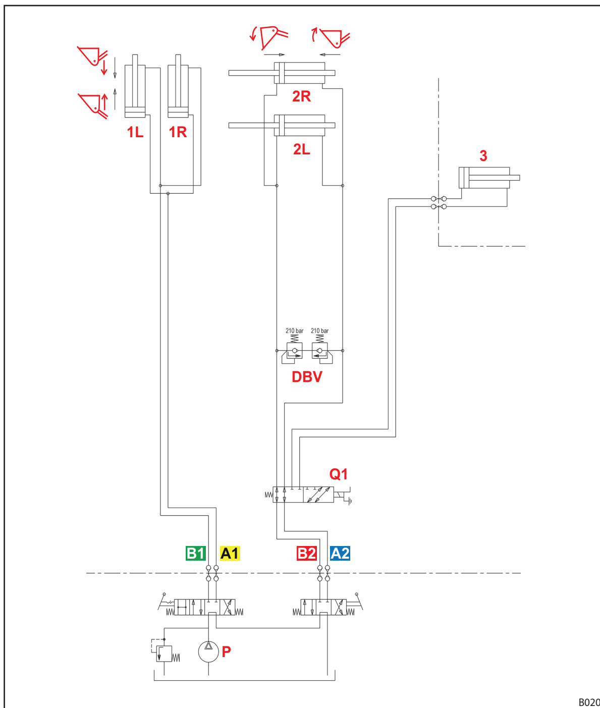
Obr. 127 Hydraulické schéma P
