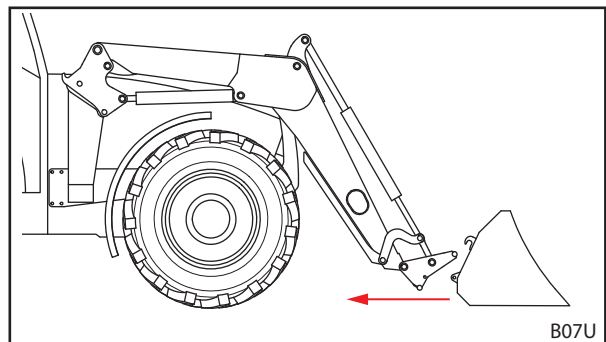
Obr. 108 Odjetí
