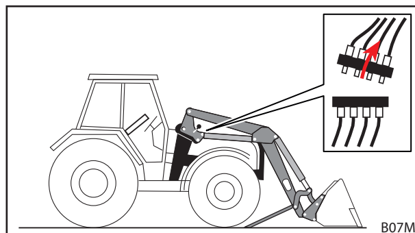
Obr. 124 Odpojení hydrauliky
