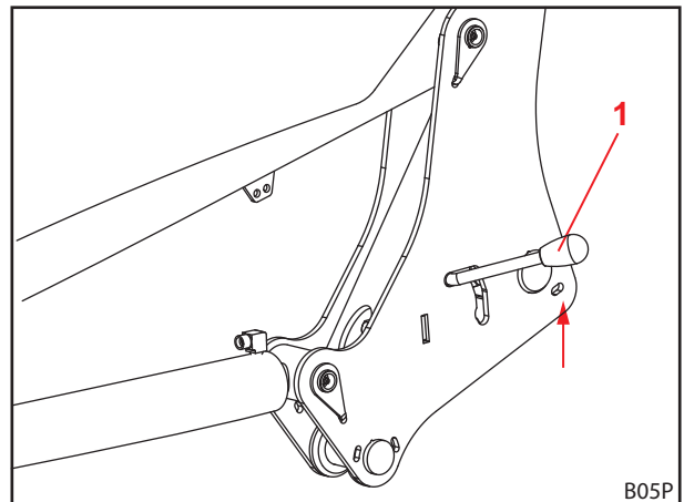
Obr. 119 Kontrola uzamykacího mechanismu čelního nakladače
