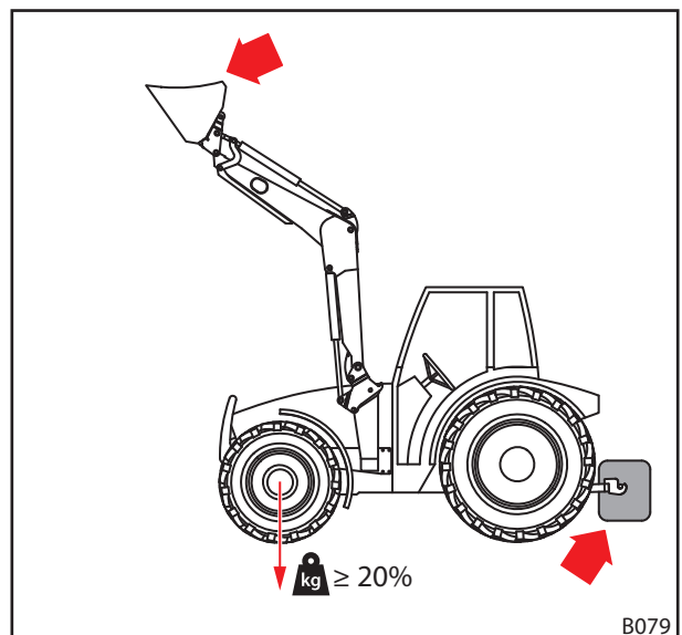
Obr. 51 Zatížení při jízdě po silnici
