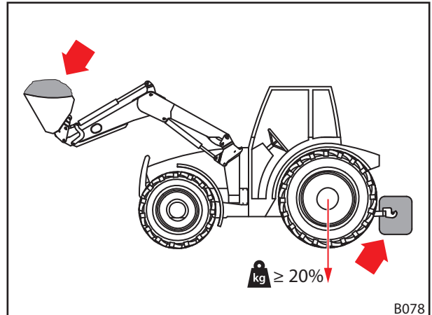
Obr. 50 Zatížení při pracích s čelním nakladačem
