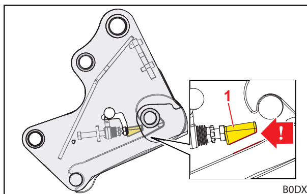
Obr. 59 Správná montážní poloha vklíněnce
