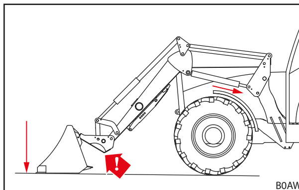
Obr. 82 Zatlačení nářadím na zem
