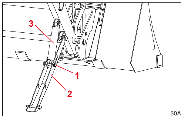
Obr. 68 Odstavná podpěra vyklopená
