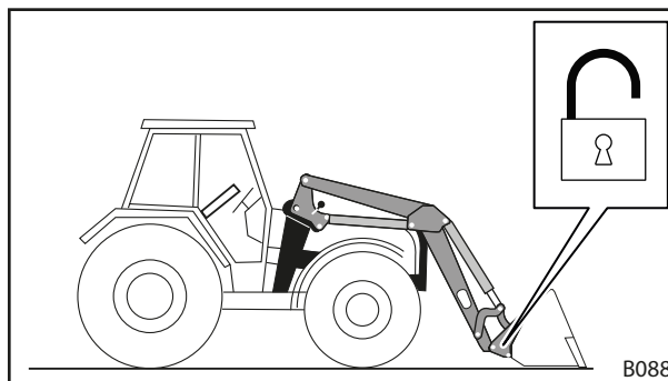
Obr. 89 Otevření zamykacího mechanismu nářadí
