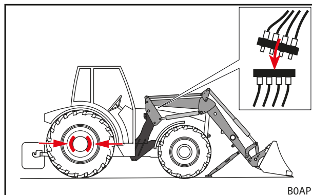
Obr. 54 Vypnutí traktoru a připojení hydraulických vedení
