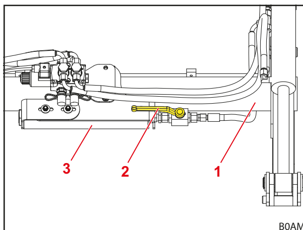
Obr. 47 Mechanicky ovládaný Comfort-Drive (poloha páky Comfort-Drive otevřeno)
