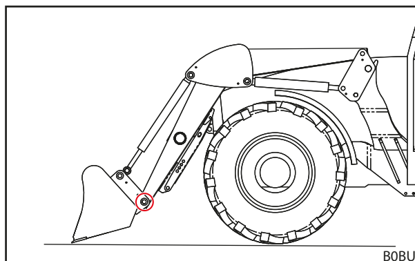
Obr. 95 Připojení nářadí v dolních otvorech na čepy
