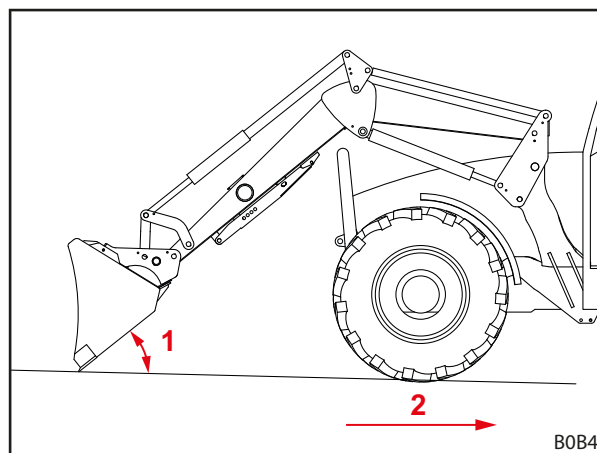
Obr. 107 Zarovnávaní při jízdě vzad
