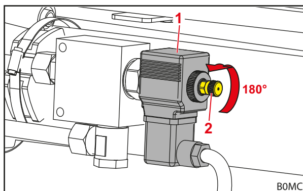
Obr. 35 Otevření ventilu
