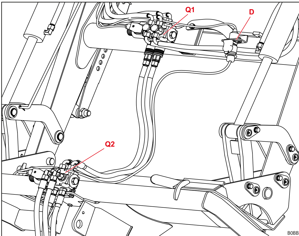
Obr. 124 Přiřazení hydraulických ventilů pro doplňkové funkce
