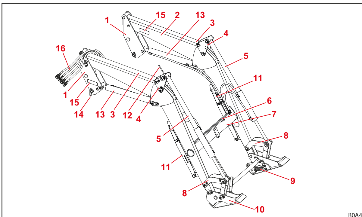
Obr. 11 Čelní nakladač P (ilustrační obrázek)
