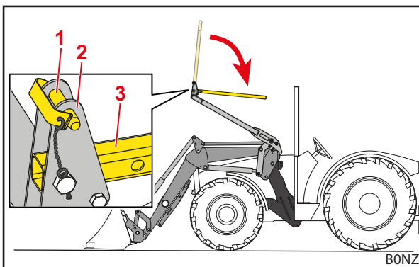
Obr. 43 Dolů sklopená horní konzola
