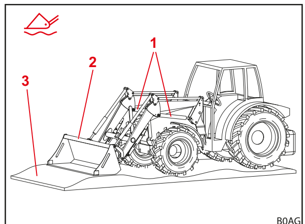
Obr. 32 Čelní nakladač v plovoucí poloze
