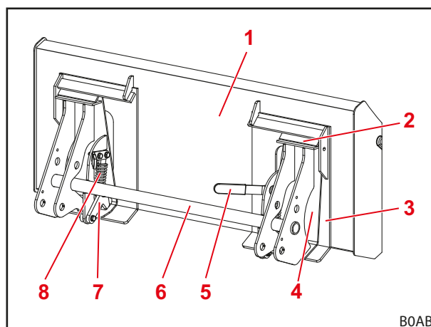
Obr. 25 Otevřený zamykací mechanismus
