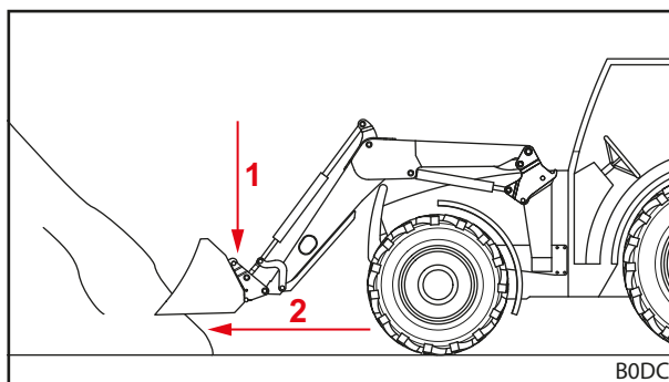
Obr. 109 Čelní nakladač spuštěný dolů a najetí rovně do nakládaného materiálu
