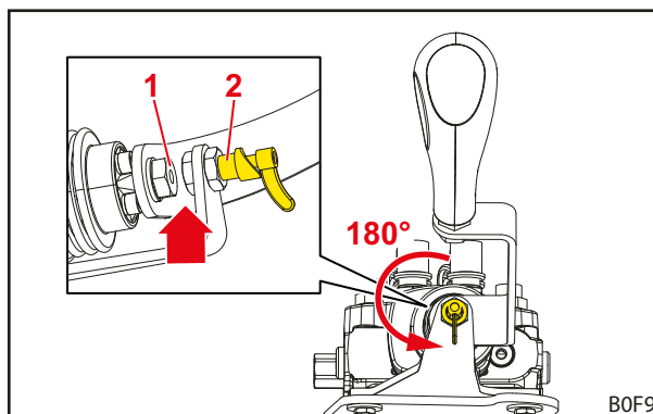
Obr. 65 Odjištěná ovládací páka
