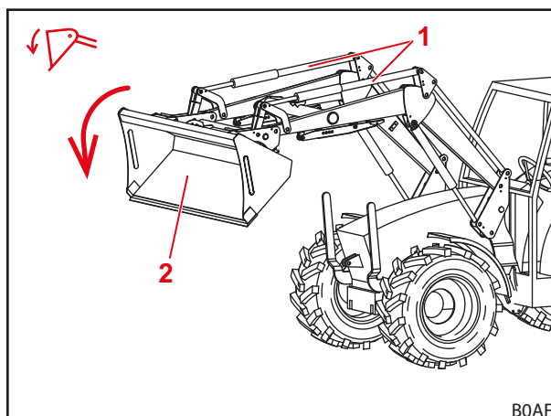
Obr. 31 Funkce vyklápění
