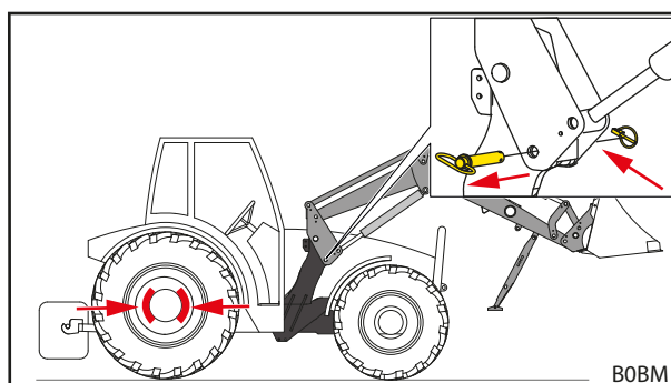
Obr. 118 Zatažení parkovací brzdy a uvolnění zamykacího mechanismu čelního nakladače
