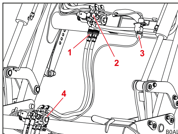
Obr. 46 Přídavný 4. řídicí okruh
