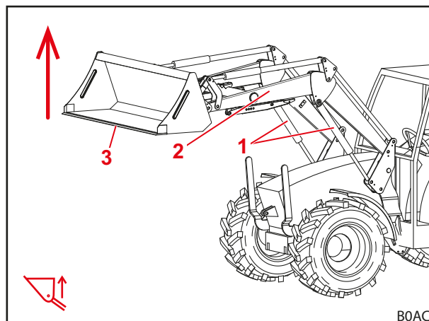
Obr. 28 Funkce zvedání
