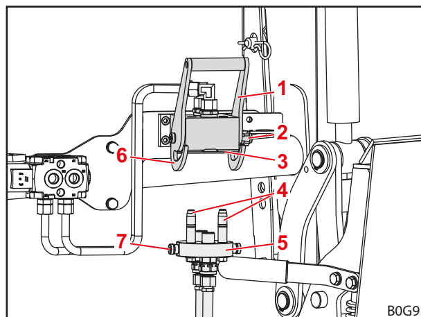
Obr. 72 Odpojená spojka nástroj-Fix
