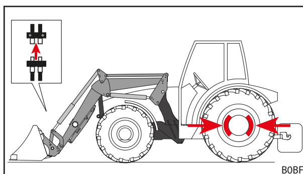
Obr. 100 Uvolnění hydraulických vedení
