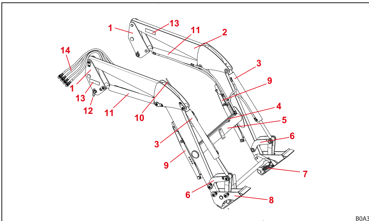
Obr. 10 Čelní nakladač H (ilustrační obrázek)
