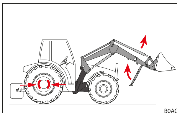
Obr. 57 Složení odstavných podpěr
