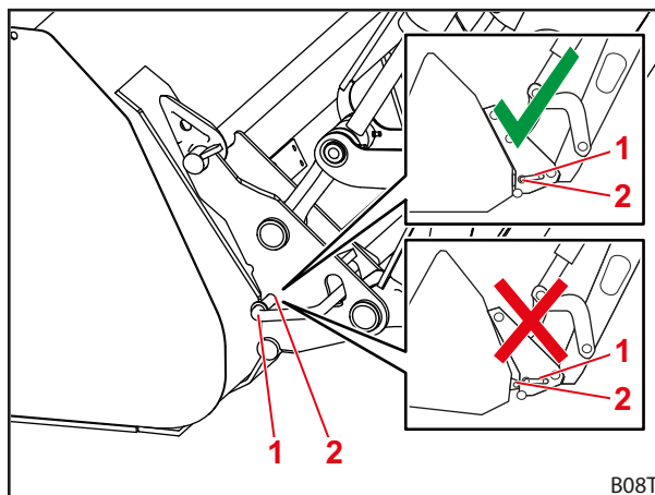
Obr. 81 Kontrola polohy uzamykacích čepů
