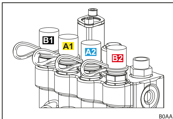
Obr. 20 Zástrčky rychlospojek přímo na hydraulickém ventilu
