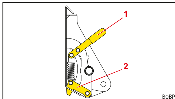
Obr. 75 Mechanický zamykací mechanismus nářadí Skid-Steer (napůl zavřený stav)
