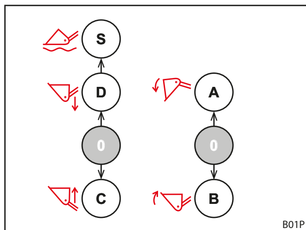
Obr. 59 Obsazení při 2 ovládacích pákách
