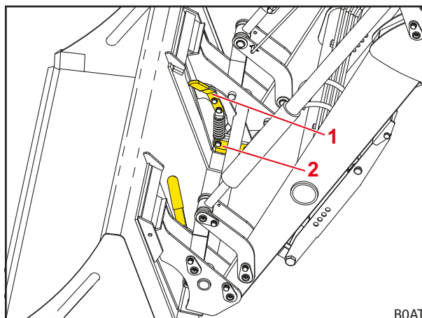
Obr. 77 Mechanický zamykací mechanismus nářadí Skid-Steer (zamknutý stav s nářadím)
