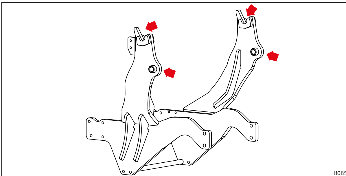
Obr. 113 Mazací místa úchytů čelního nakladače
