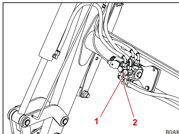
Obr. 45 Přídavný 3. řídicí okruh
