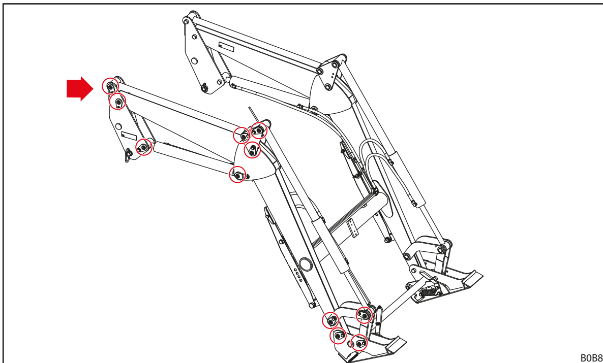
Obr. 116 Mazací místa P
