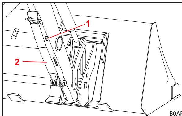
Obr. 67 Odstavná podpěra složená
