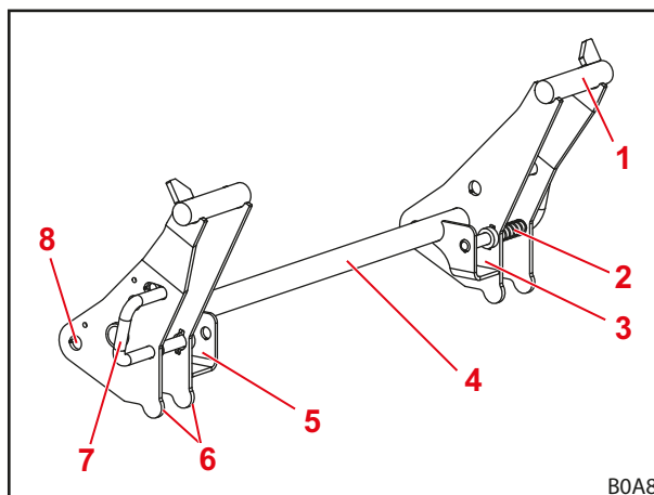
Obr. 27 Výměnný rám Euro
