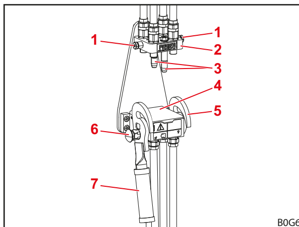
Obr. 70 Odpojená spojka Hydro-Fix
