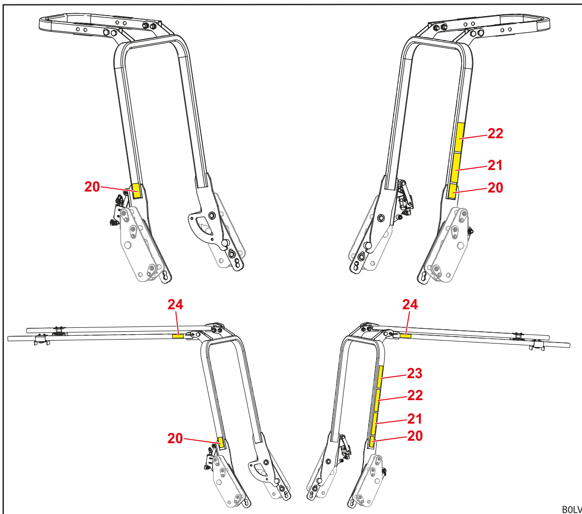
Obr. 6 OPG pro traktory s dvousloupkovou ochrannou konstrukcí při převrácení namontovanou vzadu (ilustrační obrázek)
