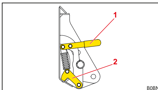
Obr. 74 Mechanický zamykací mechanismus nářadí Skid-Steer (otevřený stav)
