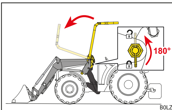
Obr. 36 Sklopení OPG dolů
