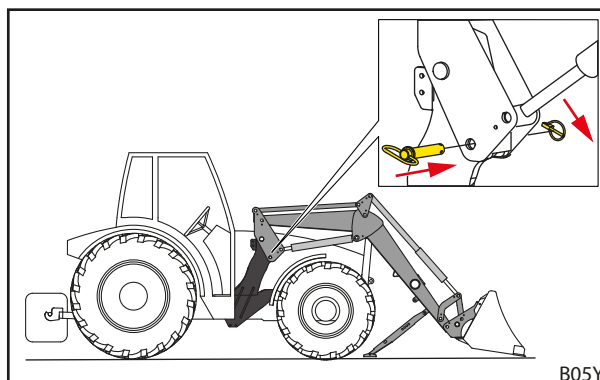
Obr. 56 Zasuňte oba zamykací čepy a zajistěte je sklopnou závlačkou
