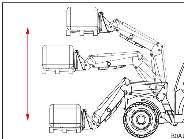
Obr. 34 Paralelní vedení
