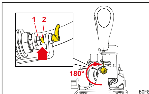
Obr. 64 Uzamknutá ovládací páka
