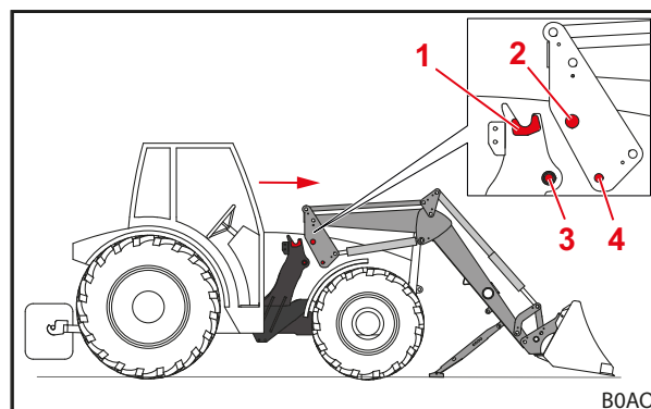
Obr. 53 Zajetí traktorem do výložníku
