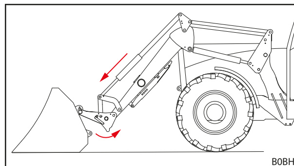
Obr. 101 Vyháknutí výměnného rámu
