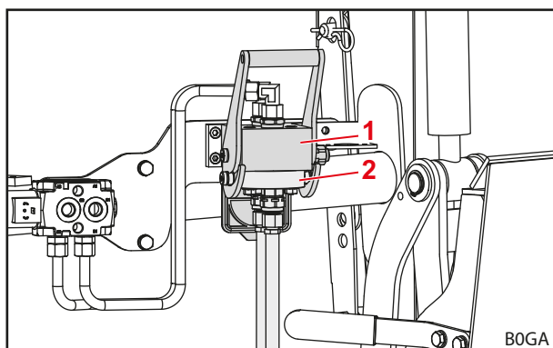
Obr. 73 Připojená spojka nástroj-Fix
