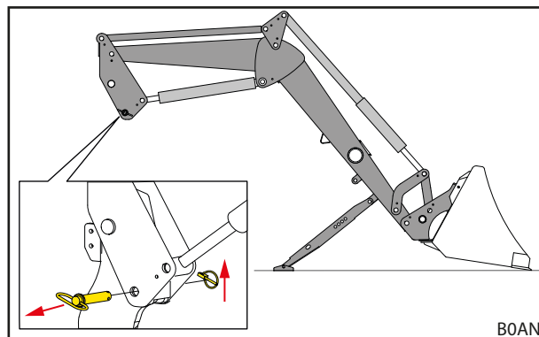
Obr. 52 Otevření uzamykacího mechanismu čelního nakladače
