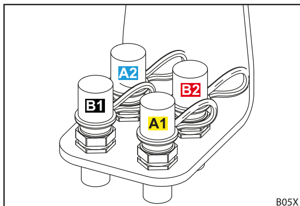
Obr. 19 Zástrčky rychlospojek na připojovaném dílu
