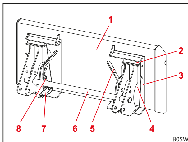
Obr. 26 Uzavřený zamykací mechanismus
