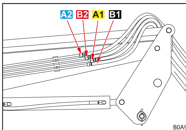
Obr. 18 Hydraulická vedení
