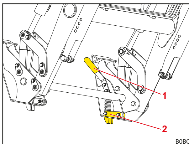
Obr. 78 Mechanický zamykací mechanismus nářadí Skid-Steer (zamknutý stav bez nářadí)
