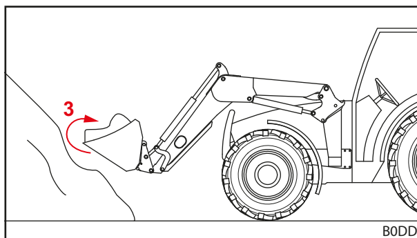
Fig. 110 Volcar el implemento hacia atrás y recoger la carga
