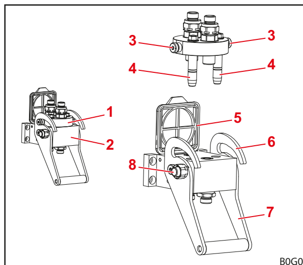
Fig. 24 Estructura del implemento-Fix
