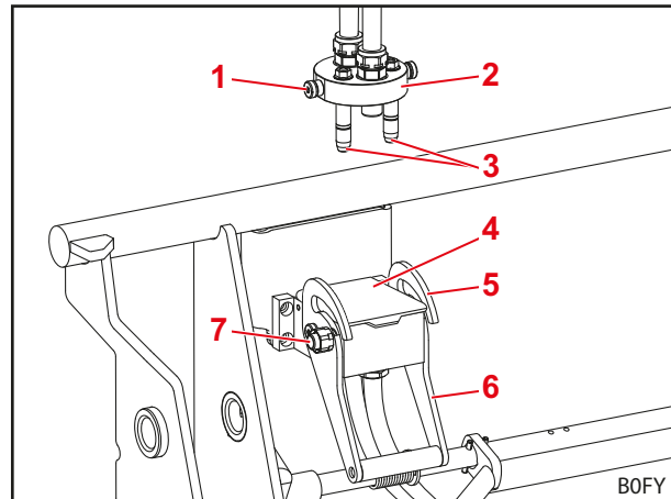
Fig. 78 Implemento-Fix desacoplado
