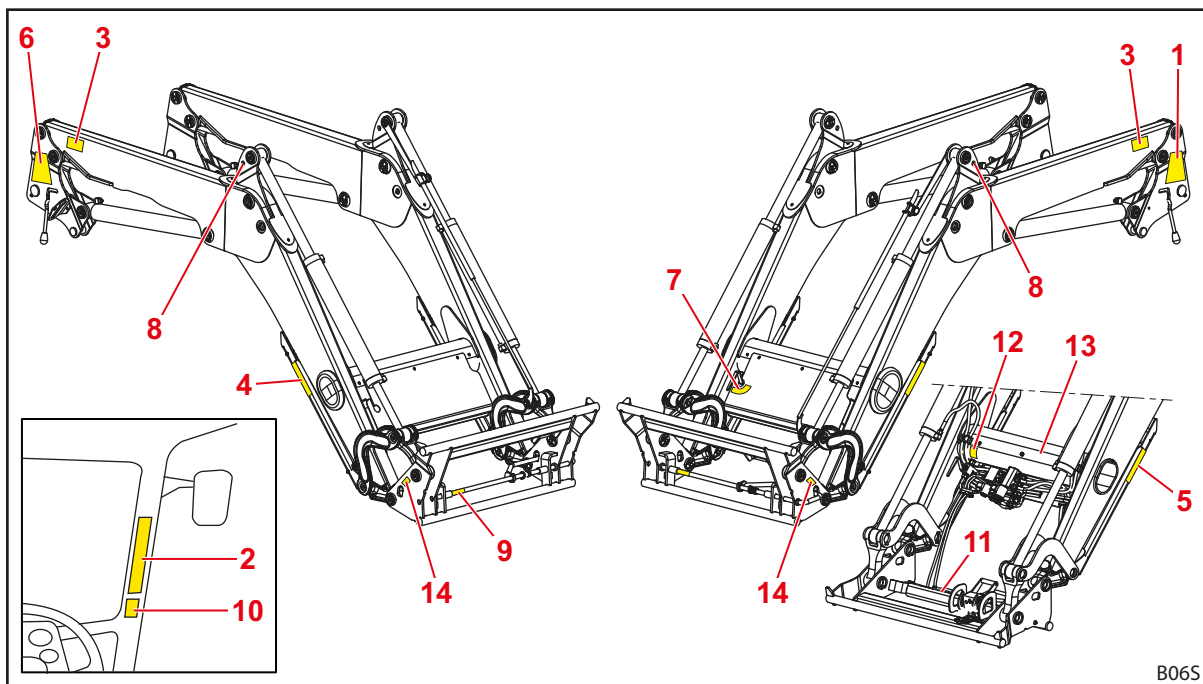
Fig. 4 Cargador frontal FZ (figura de ejemplo)
