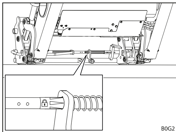
Fig. 82 Comprobar el bloqueo de implemento por medio de la etiqueta (cuadro de cambio combinado Euro-FR)
