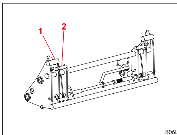
Fig. 13 Cuadro de cambio combinado Euro-Alö3
