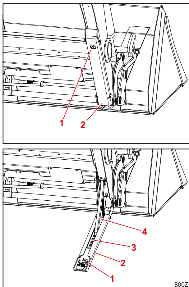
Fig. 74 Pie soporte
