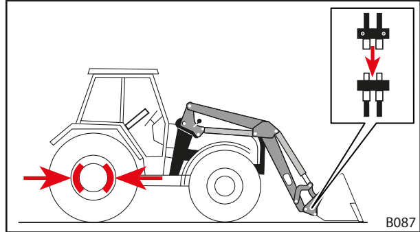
Fig. 97 Unir los conductos hidráulicos del implemento con acoplamientos del cargador frontal
