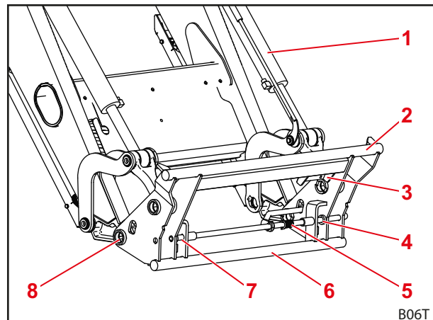
Fig. 10 Cuadro de cambio europeo
