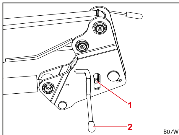
Fig. 118 Comprobar el bloqueo del cargador frontal
