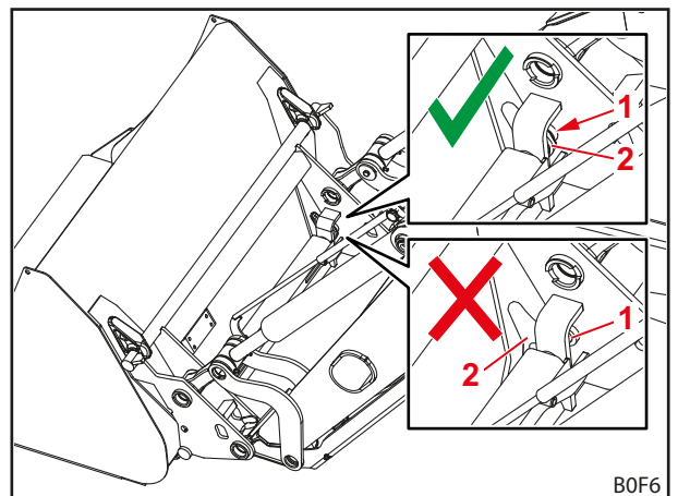
Fig. 90 Comprobar la posición de los pernos de bloqueo
