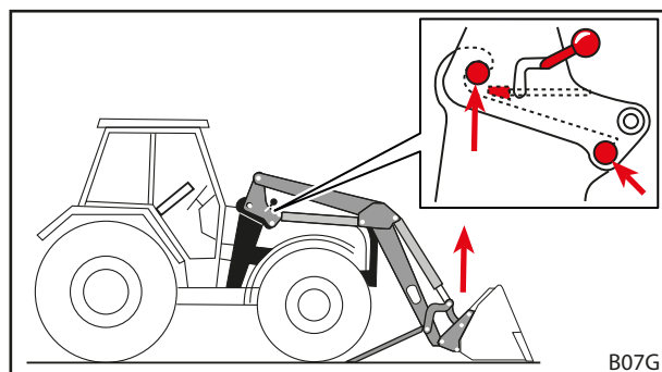
Fig. 50 Utilizar la función Elevar hasta que los bulones tengan contacto con el gancho de retenida
