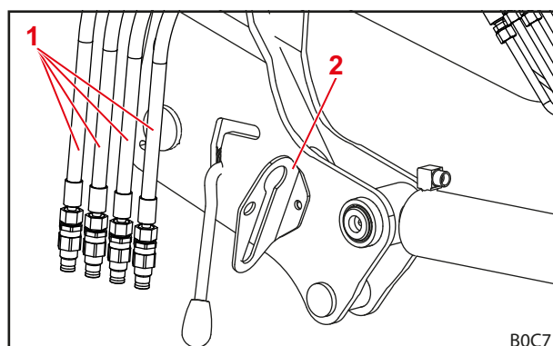
Fig. 126 Enganchar las conducciones hidráulicas a soportes de acoplamiento (representación con acoples de enchufe)
