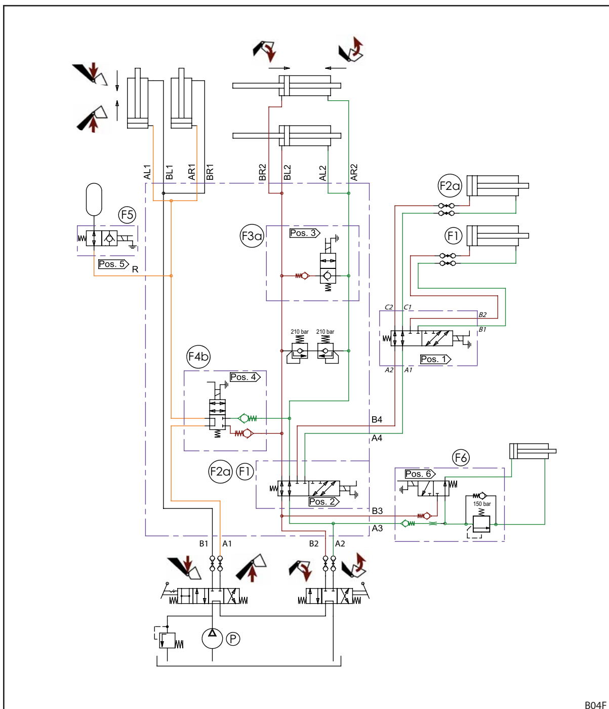
Fig. 129 Esquema hidráulico FZ y FZ-L (en caso de equipamiento con 3.er y 4.º circuito de control)
