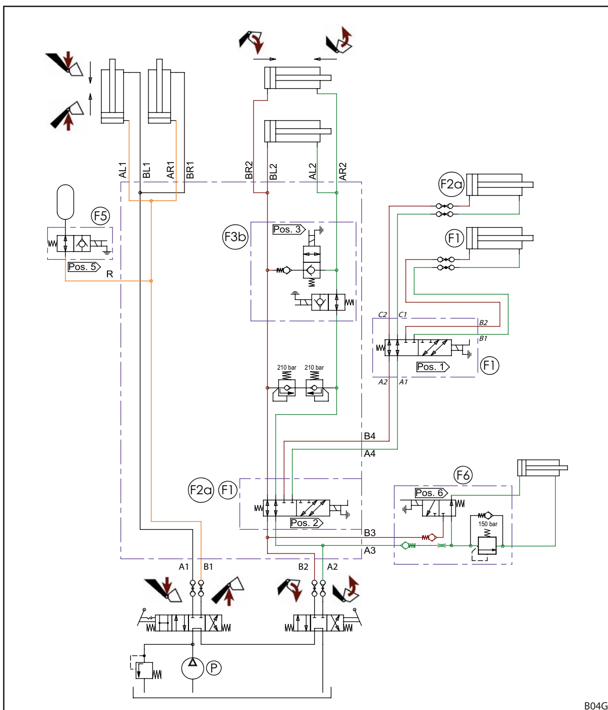
Fig. 127 Esquema hidráulico FS y marcha rápida FS (en caso de equipamiento con 3. a y 4. a función)
