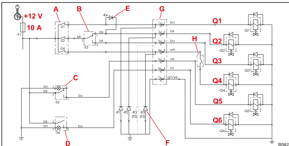
Fig. 131 Esquema eléctrico (en caso de equipamiento con 3.ª y 4.ª función)
