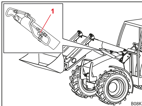
Fig. 42 Válvula de control de descenso
