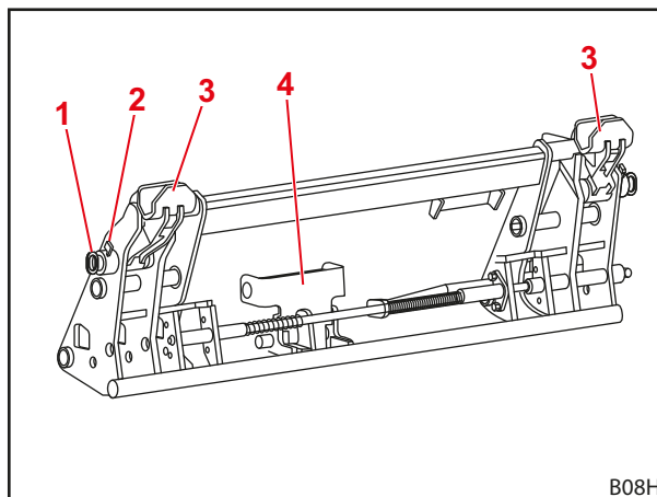
Fig. 14 Cuadro de cambio combinado Euro-FR
