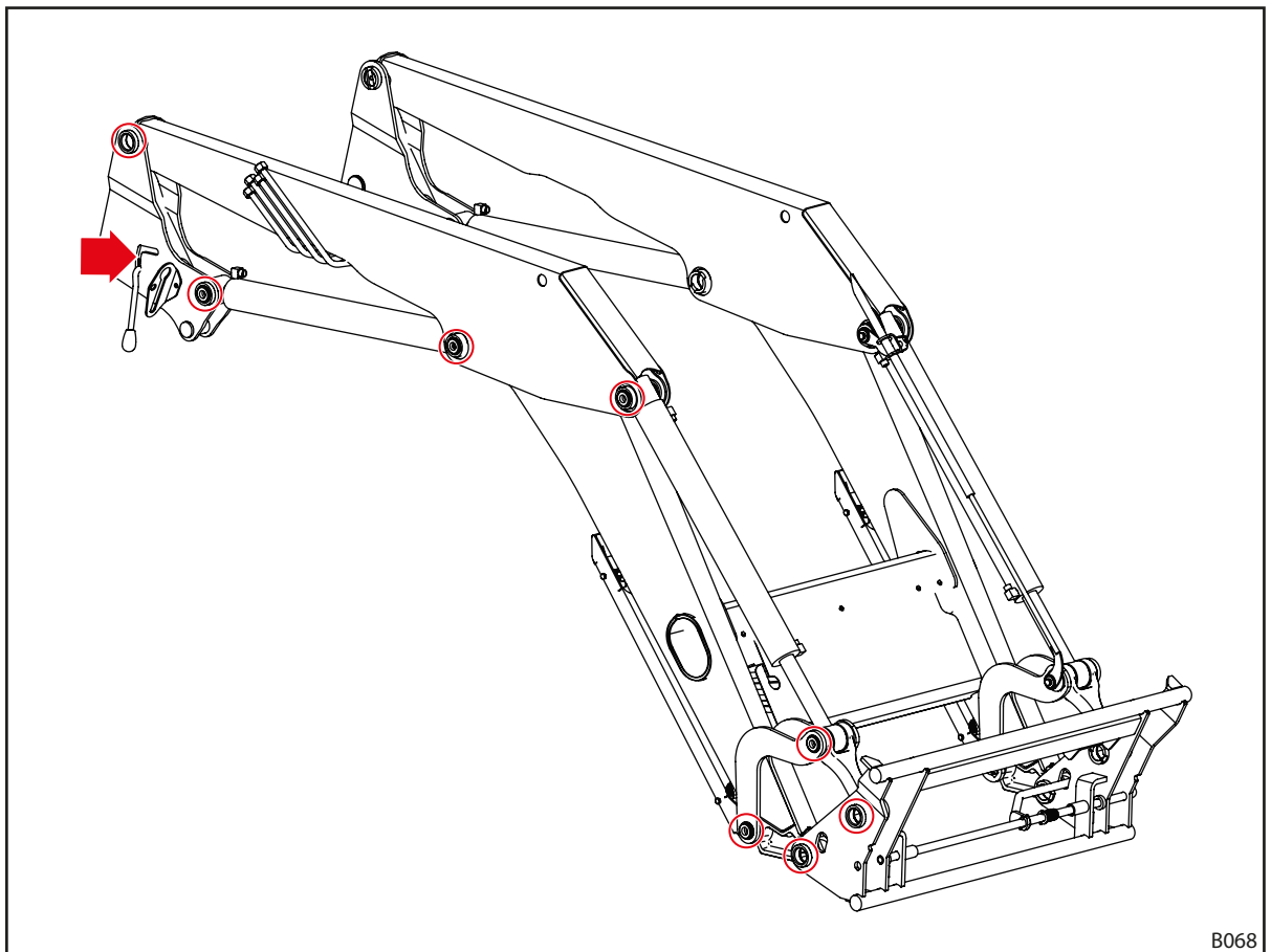
Fig. 114 Puntos de engrase FS
