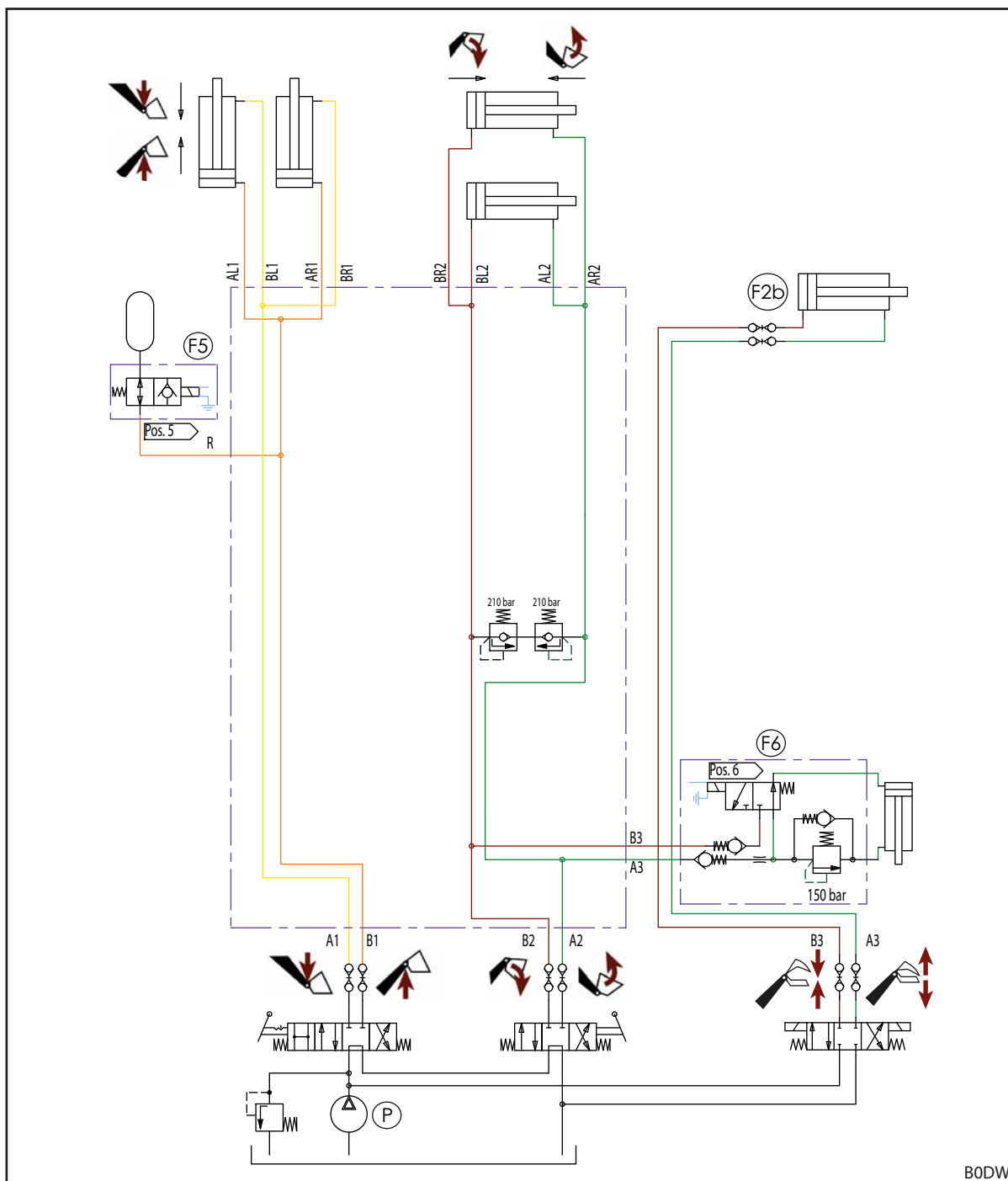
Fig. 128 Esquema hidráulico FS (en caso de equipamiento con REAL 3 )
