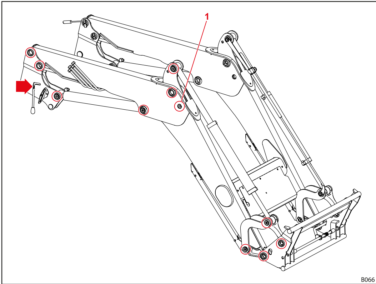
Fig. 115 Puntos de engrase FZ
