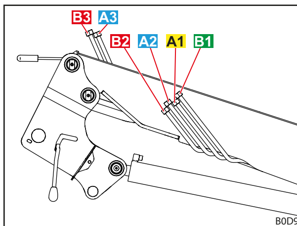
Fig. 18 Conductos hidráulicos (opción REAL 3 )
