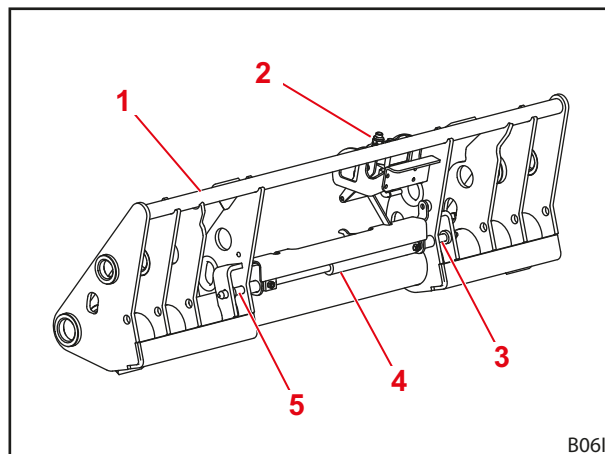
Fig. 16 Cuadro de cambio Euro (FZ 100) reforzado
