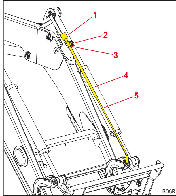
Fig. 36 Sensor Return-To-Level en el indicador visual
