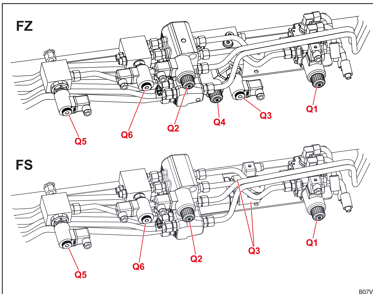
Fig. 133 Disposición de las válvulas hidráulicas para funciones adicionales
