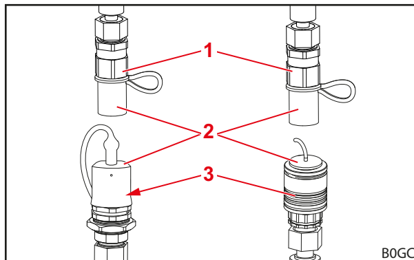
Fig. 75 Acoplamientos por enchufe (figuras de ejemplo)
