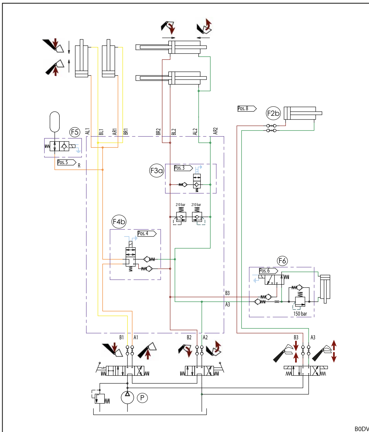
Fig. 130 Esquema hidráulico FZ y FZ-L (en caso de equipamiento con REAL 3 )
