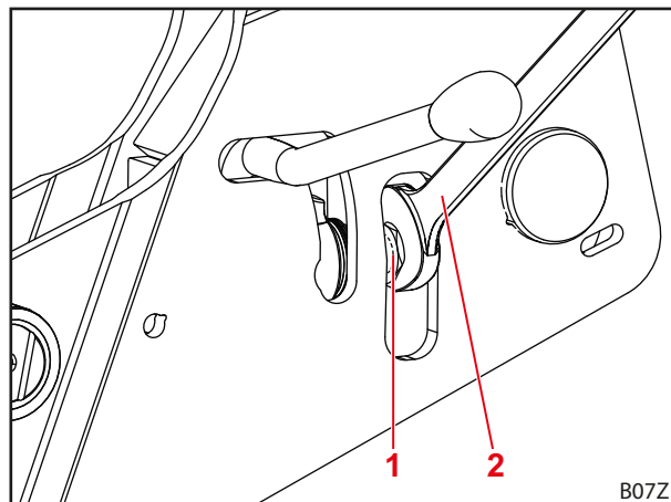
Fig. 58 Colocar el implemento
