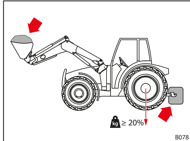
Fig. 44 Carga al trabajar con el cargador frontal
