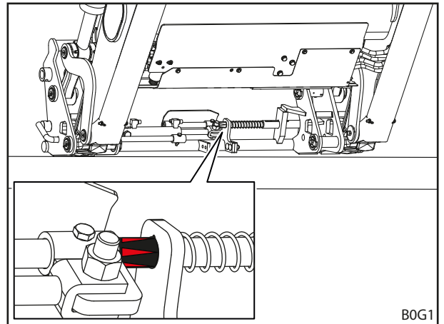
Fig. 88 Comprobar el bloqueo de implemento por medio de la etiqueta
