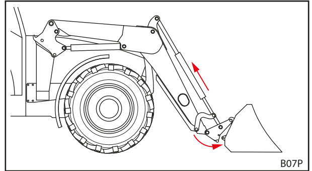
Fig. 103 Enganche
