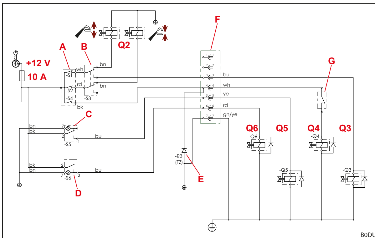
Fig. 132 Esquema eléctrico (en caso de equipamiento con REAL 3 )
