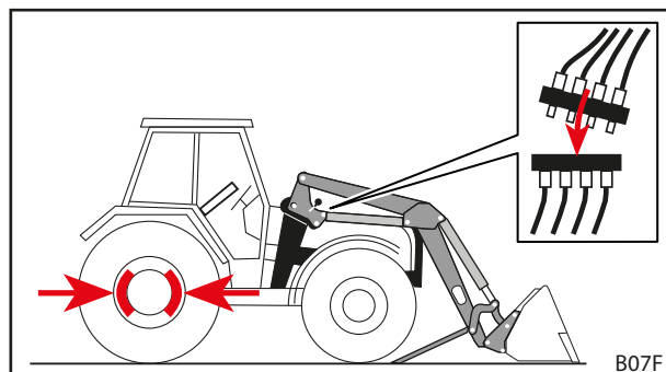
Fig. 49 Desconectar el tractor y conectar los conductos hidráulicos
