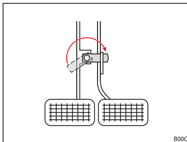
Fig. 43 Conectar los pedales de freno
