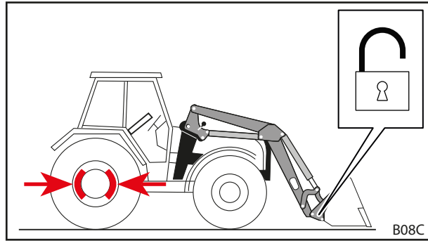
Fig. 104 Abrir bloqueo de implemento
