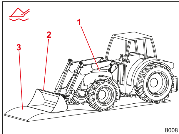
Fig. 31 Cargador frontal en posición flotante
