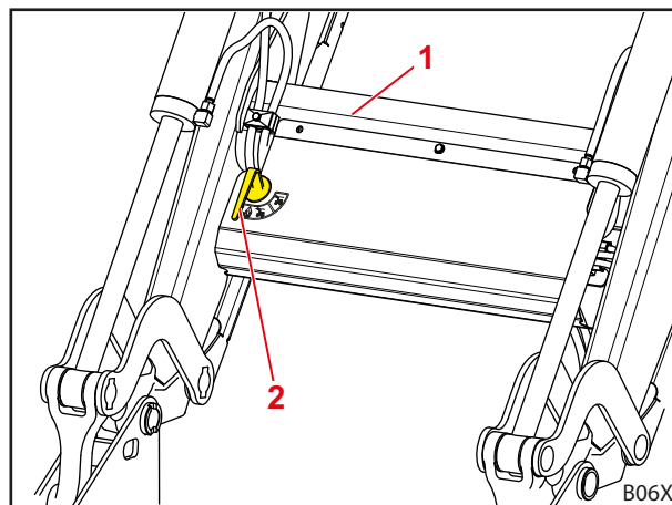
Fig. 40 Comfort-Drive con accionamiento manual
