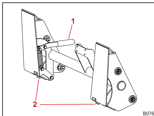
Fig. 15 Cuadro de cambio Skid-Steer
