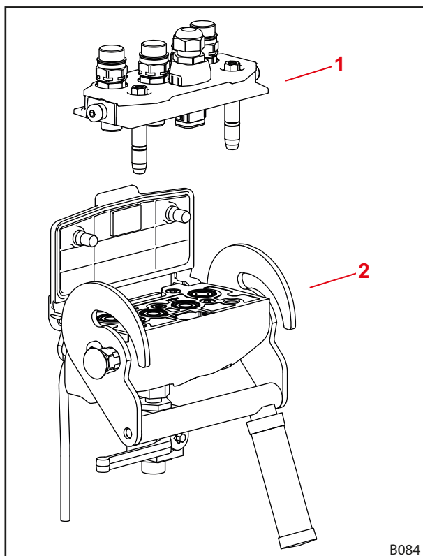
Obr. 20 Konštrukcia Hydro-Fix
