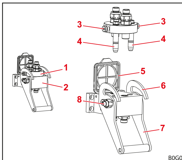
Obr. 22 Konštrukcia Implement-Fix
