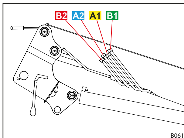
Obr. 15 Hydraulické vedenia
