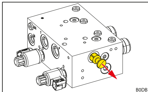
Obr. 76 Vytiahnutie ventilu na odľahčenie od tlaku na ventile REAL 3
