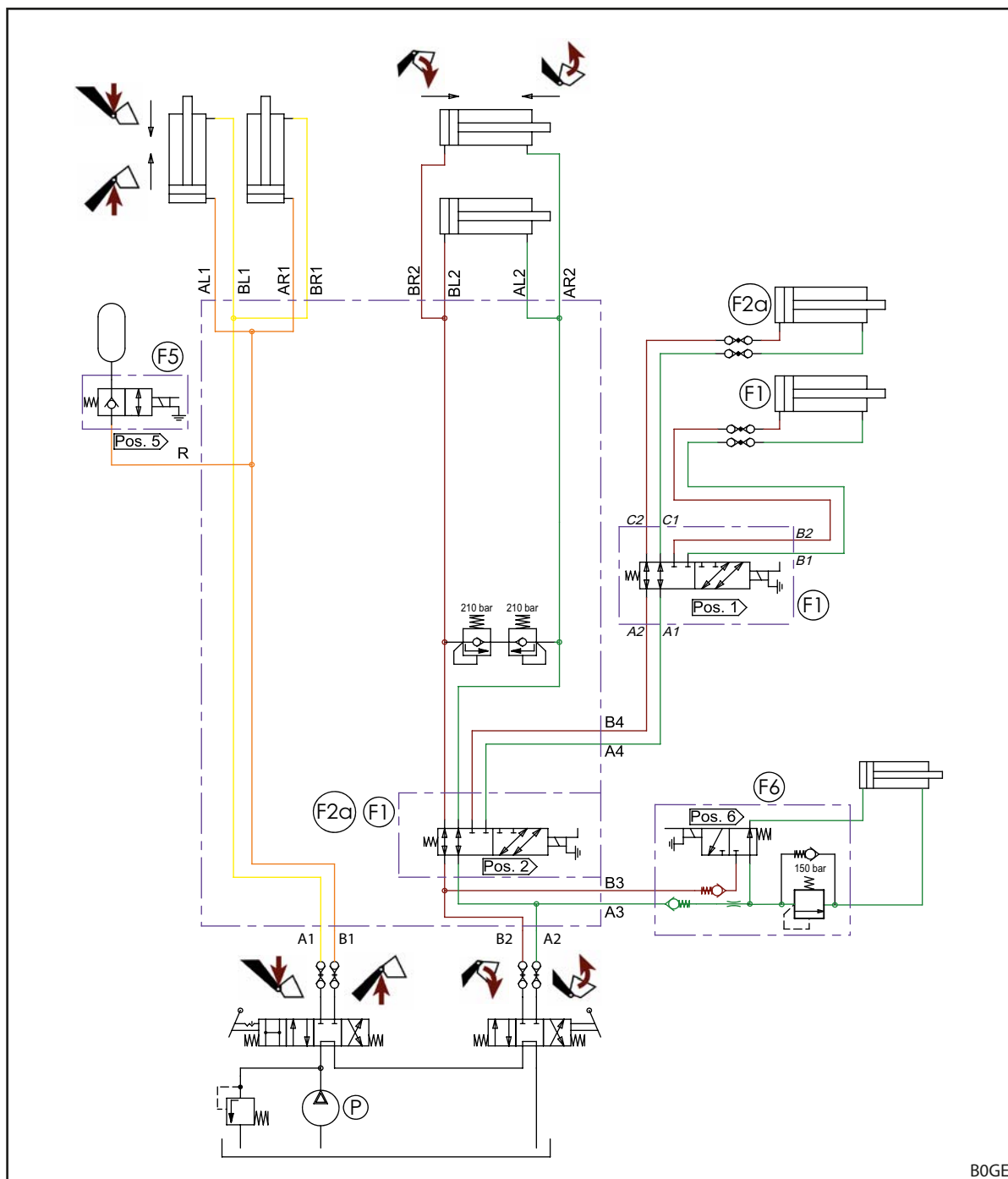
Obr. 131 Hydraulická schéma FS (pri výbave s 3. a 4. riadiacim okruhom)
