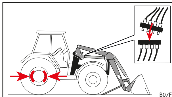
Obr. 52 Vypnutie traktora a pripojenie hydraulických vedení
