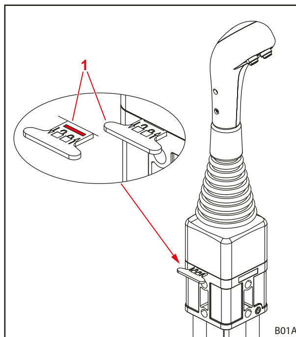
Obr. 68 Zaistenie ovládacej páky
