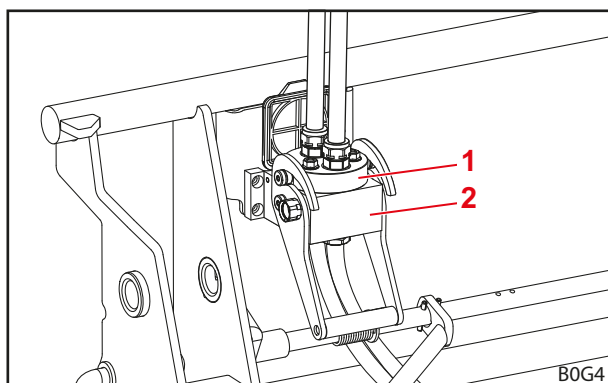
Obr. 83 Pripojené Implement-Fix
