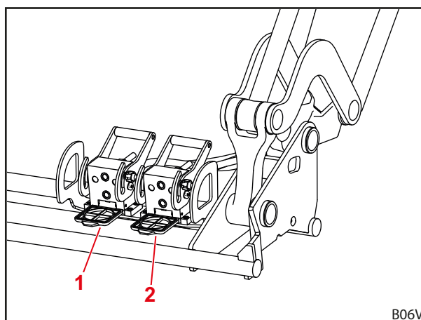
Obr. 36 Dodatočný 4. riadiaci okruh
