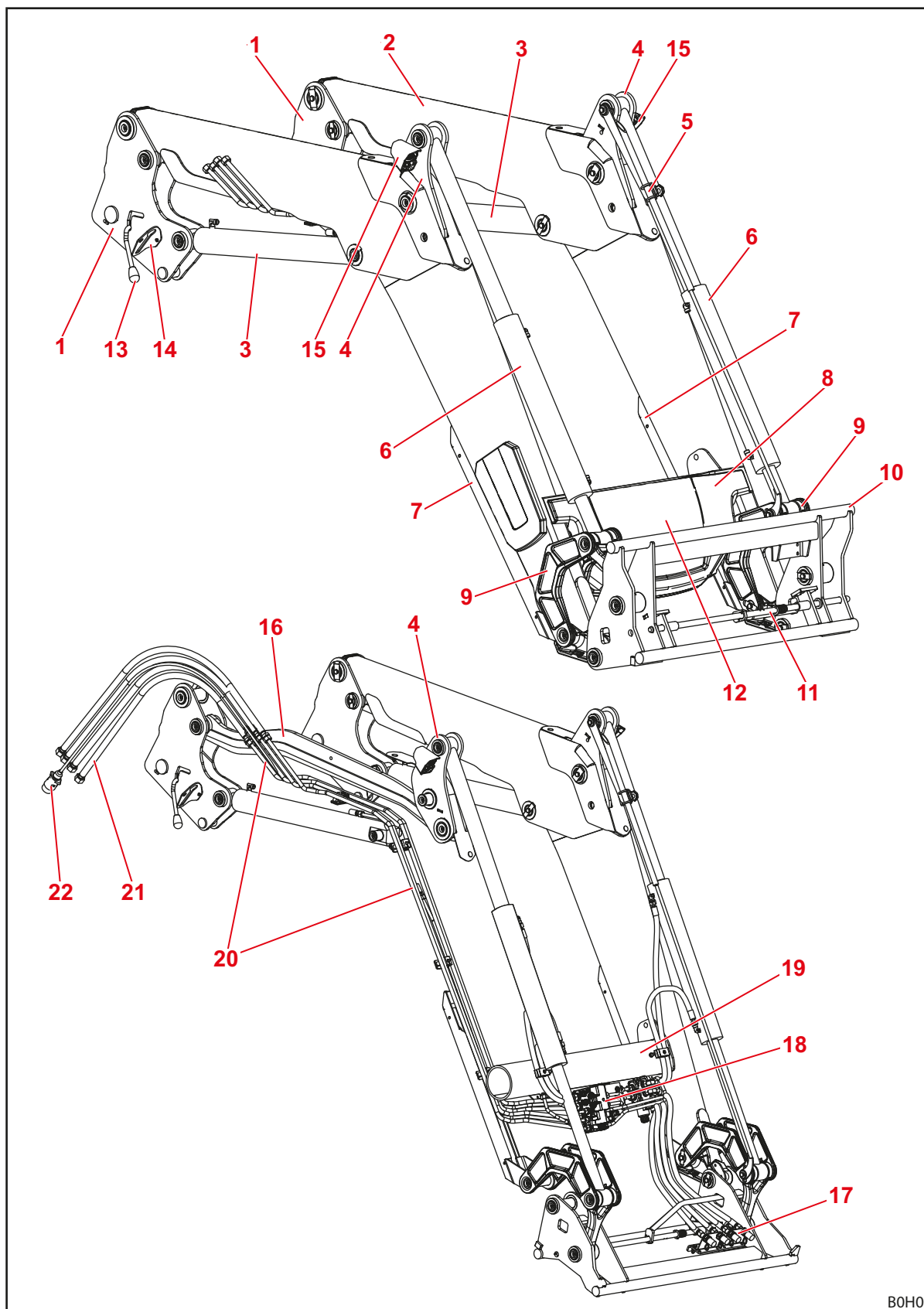
Obr. 8 Čelný nakladač FZ
