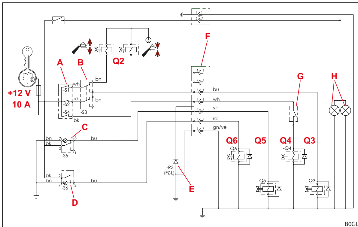
Obr. 138 Elektrická schéma zapojenia (pri výbave s REAL 3 )
