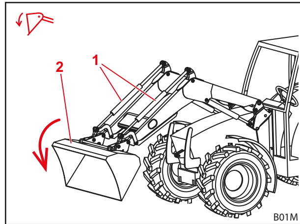
Obr. 28 Funkcia vysypávania
