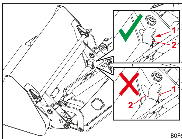
Obr. 93 Kontrola pozície istiaceho čapu
