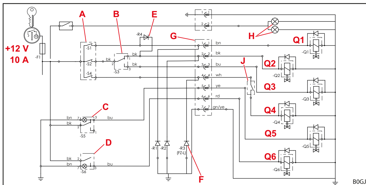
Obr. 137 Elektrická schéma zapojenia (pri výbave s 3. a 4. riadiacim okruhom)
