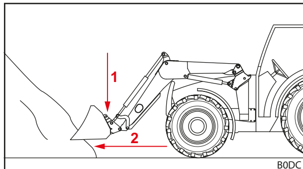
Obr. 113 Spustíte čelný nakladač a vojdete s ním rovno do nakladaného materiálu
