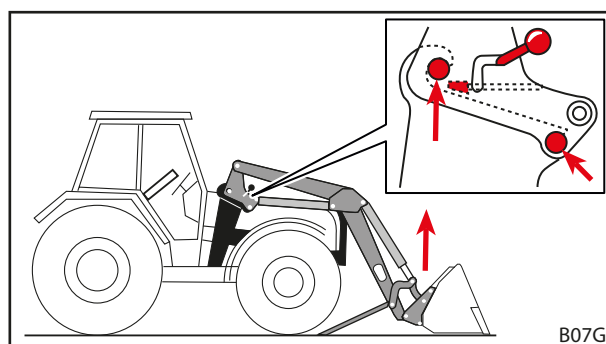
Obr. 53 Funkciu Zdvíhanie používajte dovtedy, kým nebudú čapy čelného nakladača dosadať v zachytávacích hákoch.
