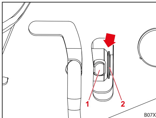
Obr. 123 Kontrola medzery
