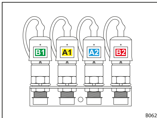
Obr. 17 Zásuvné spojky spojené
