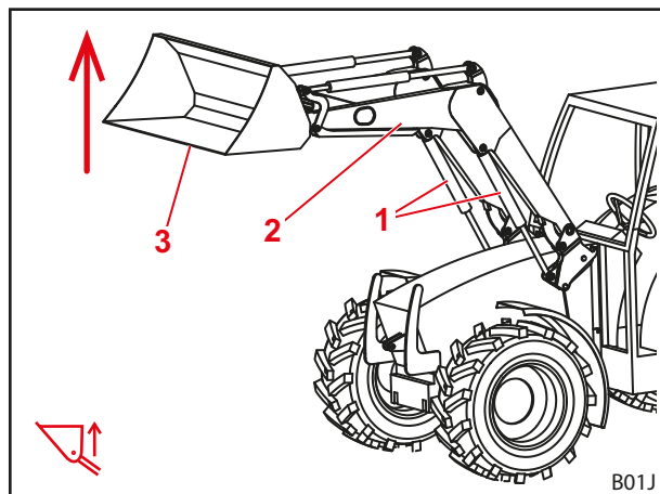
Obr. 25 Funkcia zdvíhania
