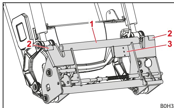
Obr. 11 Kombinovaný výmenný rám Euro-SMS
