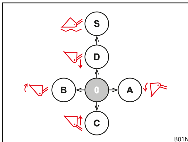
Obr. 65 Obsadenie pri jednej ovládacej páke
