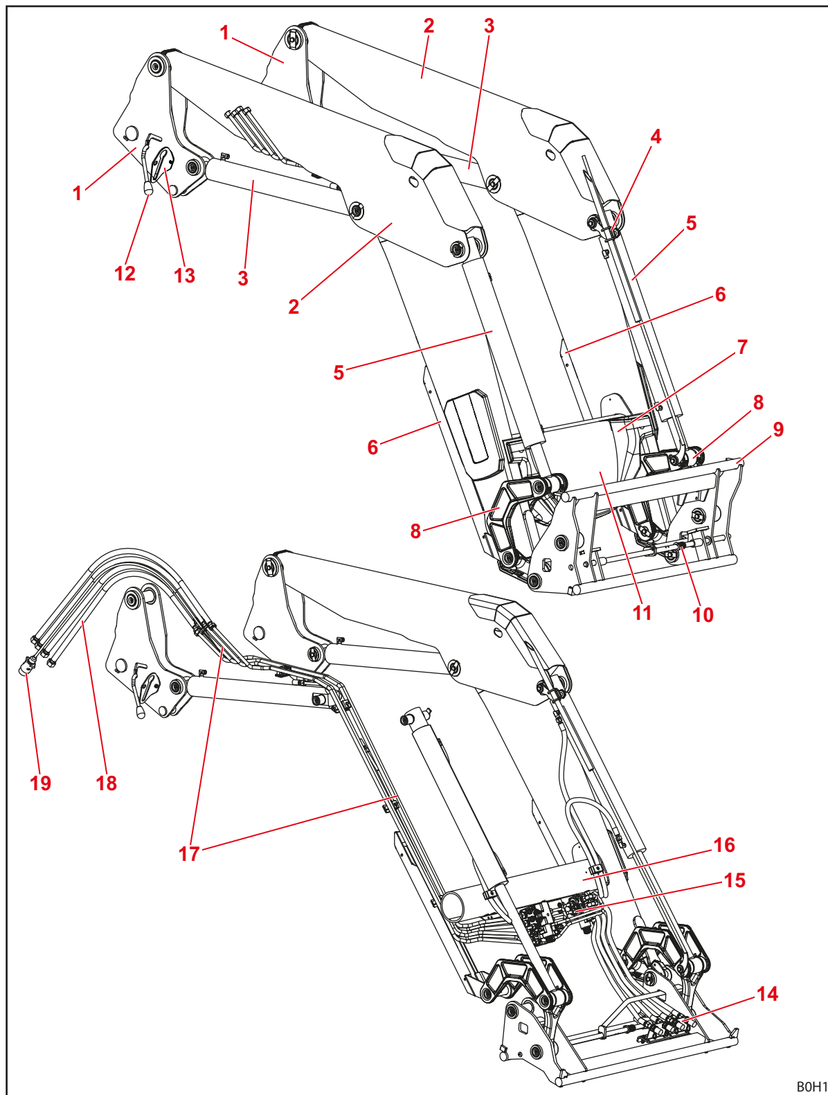
Obr. 7 Čelný nakladač FS
