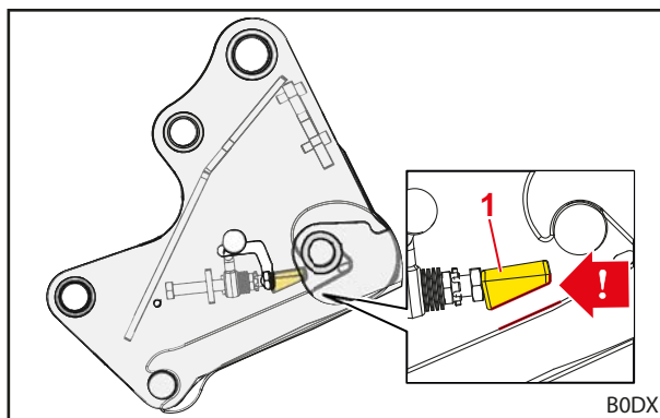
Obr. 55 Správna montážna pozícia upínacieho klinu
