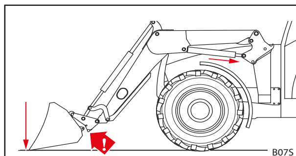
Obr. 87 Zatláčenie nástroja na zem
