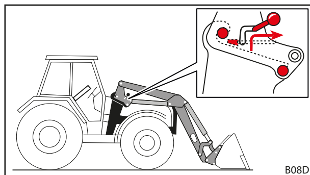
Obr. 126 Uvoľnenie zaistenia čelného nakladača
