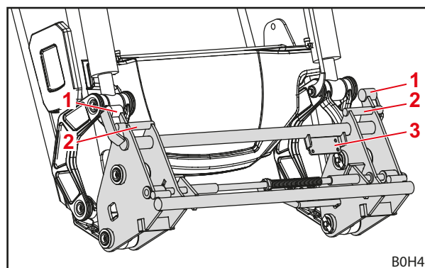
Obr. 12 Kombinovaný výmenný rám Euro-Alö3
