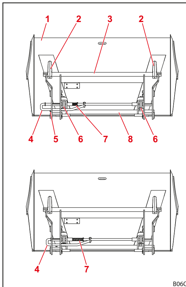
Obr. 23 Otvorené (hore) a zatvorené (dole) zaistenie
