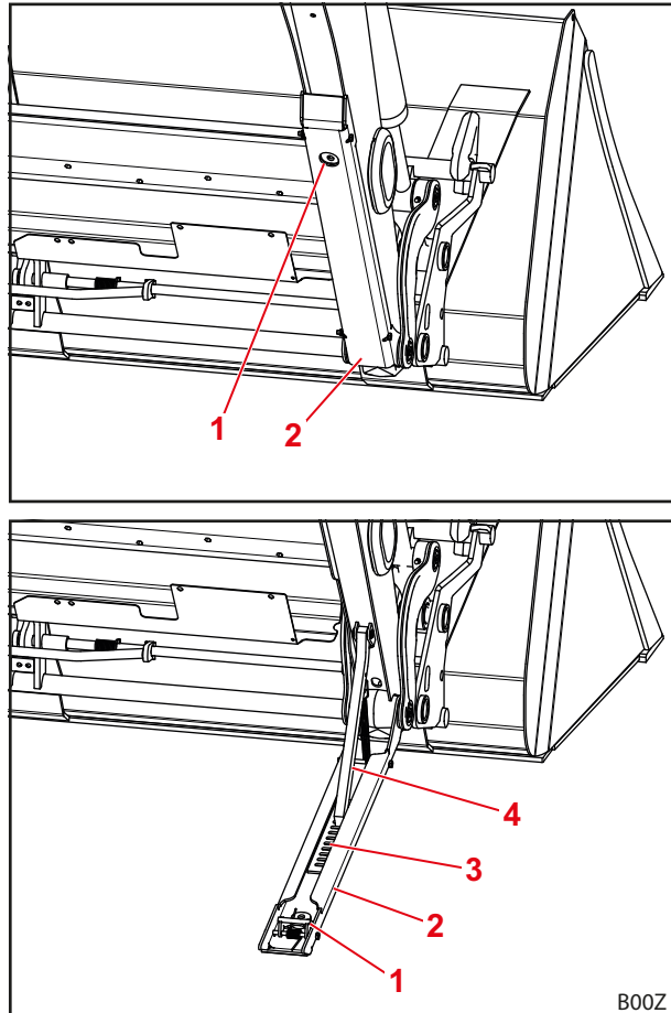
Obr. 78 Odstavovacia podpera
