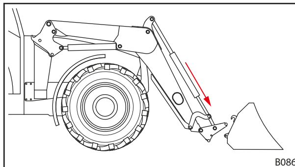
Obr. 96 Polohovanie otočného ramena
