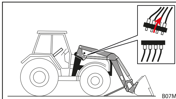
Obr. 128 Odpojenie hydrauliky
