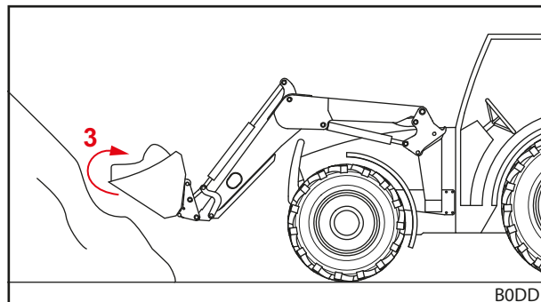
Obr. 114 Sklopenie nástroja dozadu a naloženie nakladaného tovaru
