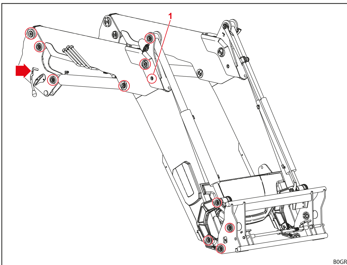
Obr. 119 Miesta mazania FZ
