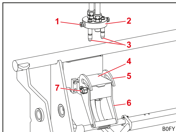
Obr. 82 Odpojené Implement-Fix
