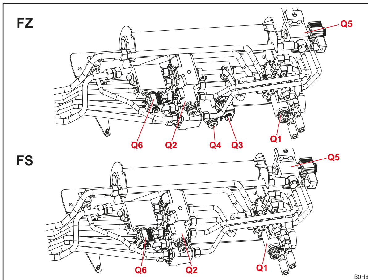
Obr. 139 Usporiadanie hydraulických ventilov pre prídavné funkcie
