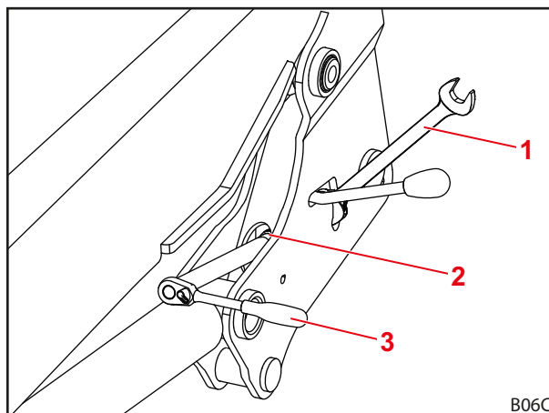
Obr. 57 Založenie nástroja
