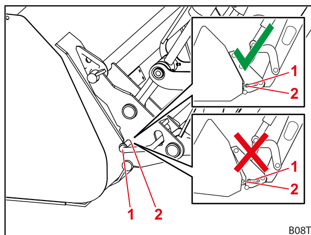
Obr. 86 Kontrola pozície istiaceho čapu
