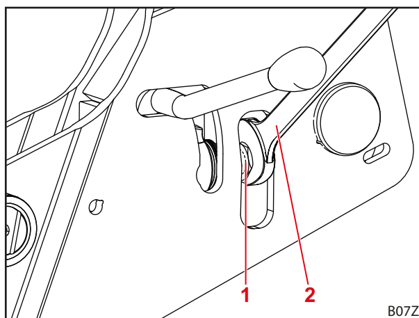
Obr. 64 Utiahnutie poistnej matice
