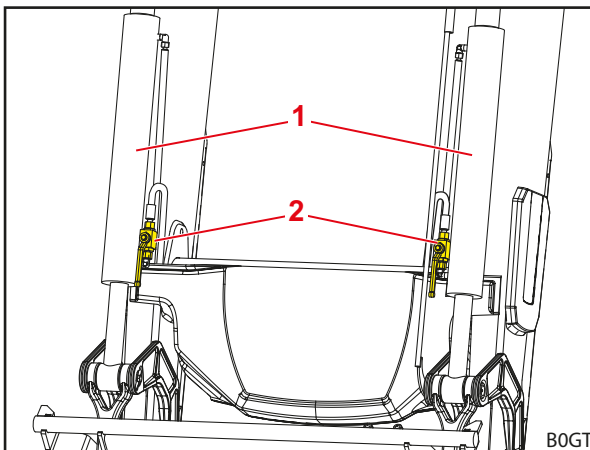
Obr. 42 Uzatváracie kohúty na valcoch nástroja
