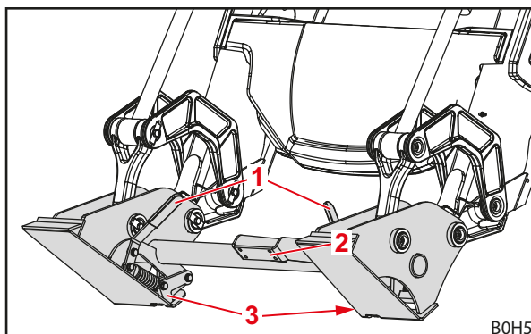
Obr. 13 Výmenný rám Skid-Steer
