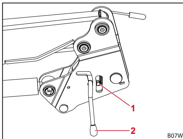
Obr. 122 Kontrola zaistenia čelného nakladača
