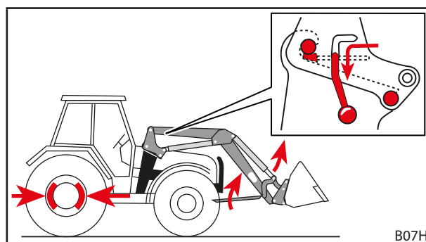
Obr. 54 Sklápanie odstavovacích podpier a zatvorenie zaistení čelného nakladača
