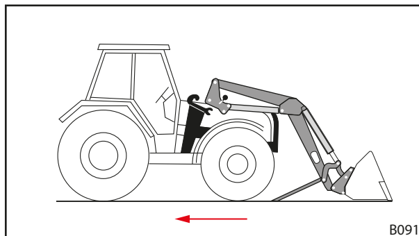
Obr. 129 Presunutie traktora dozadu
