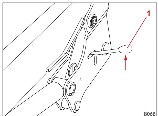
Obr. 121 Kontrola zaistenia čelného nakladača
