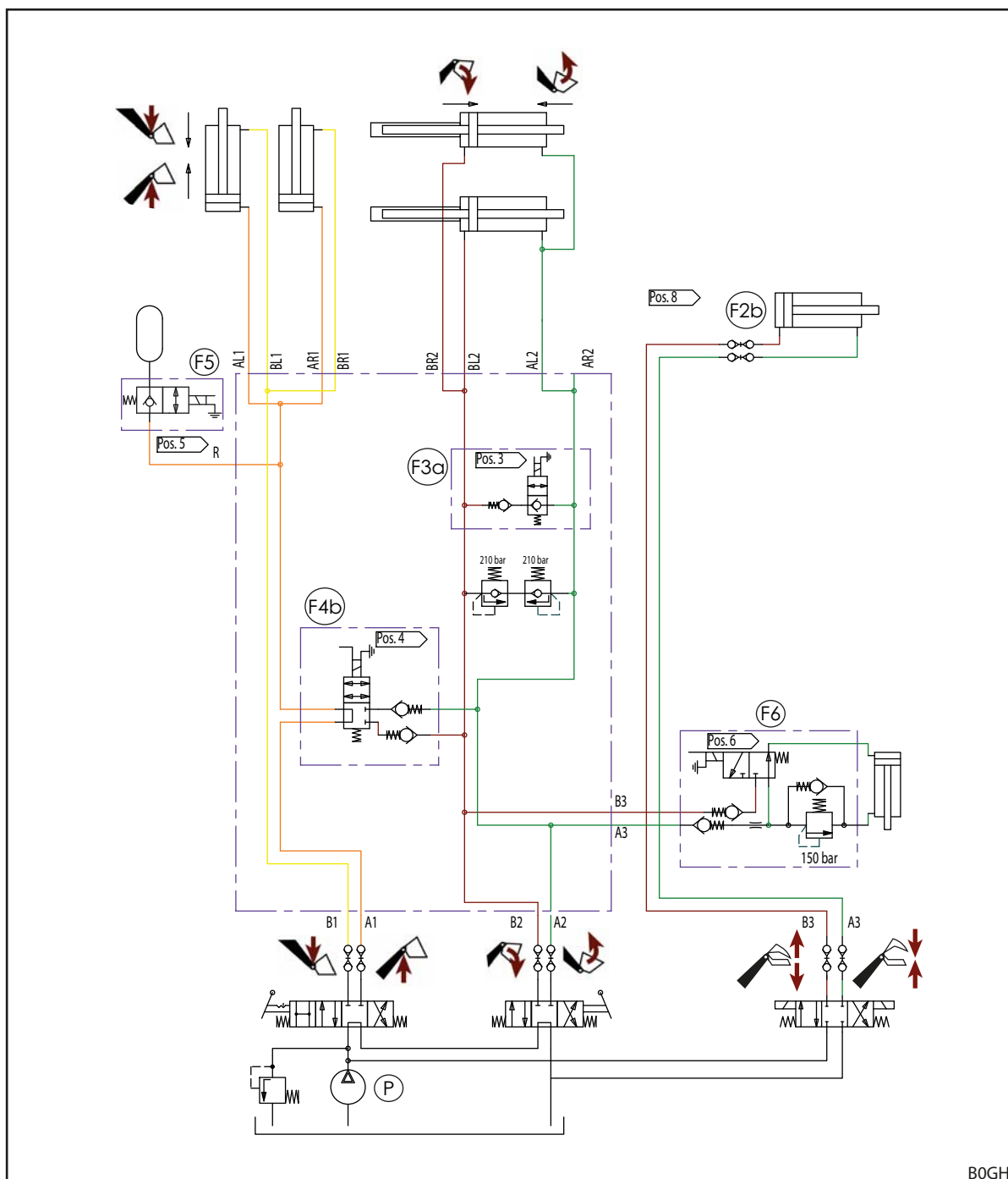
Obr. 134 Hydraulická schéma FZ a FZ-L (pri výbave s REAL 3 )
