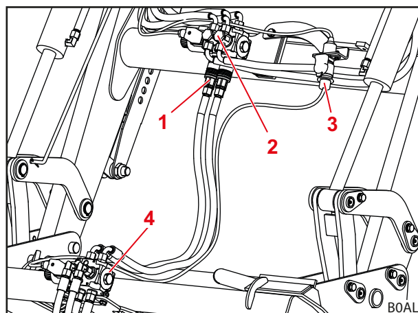
Obr. 46 Dodatočný 4. riadiaci okruh
