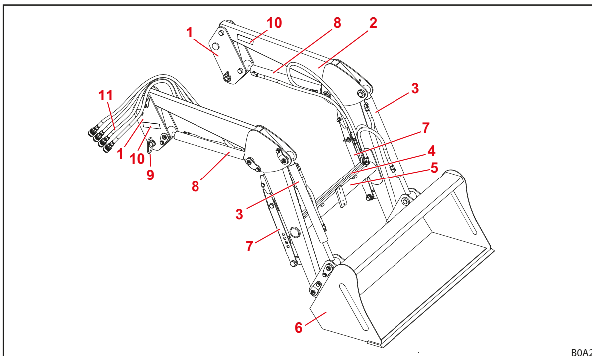
Obr. 9 Čelný nakladač L (príkladný obrázok)
