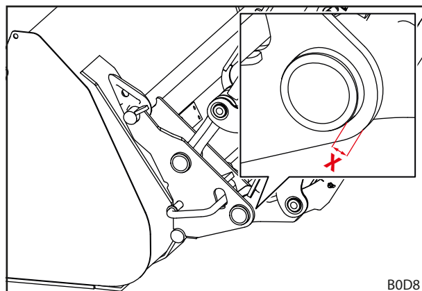
Obr. 117 Rozmer opotrebenia výmenného rámu
