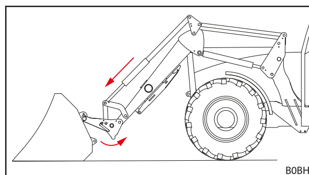
Obr. 101 Vyháknutie výmenného rámu
