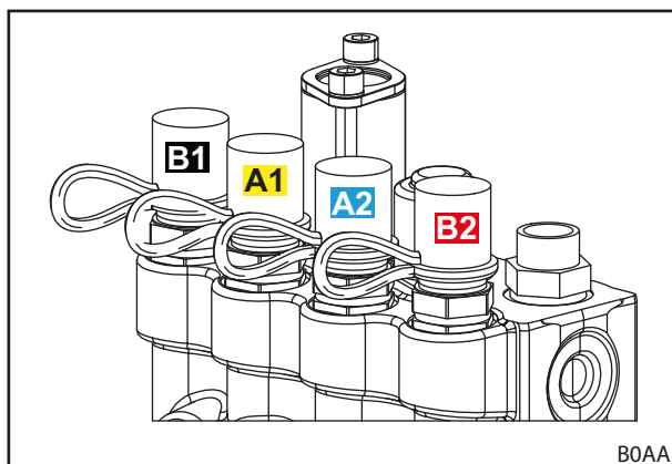
Obr. 20 Zástrčky zásuvných spojok priamo na hydraulickom ventile
