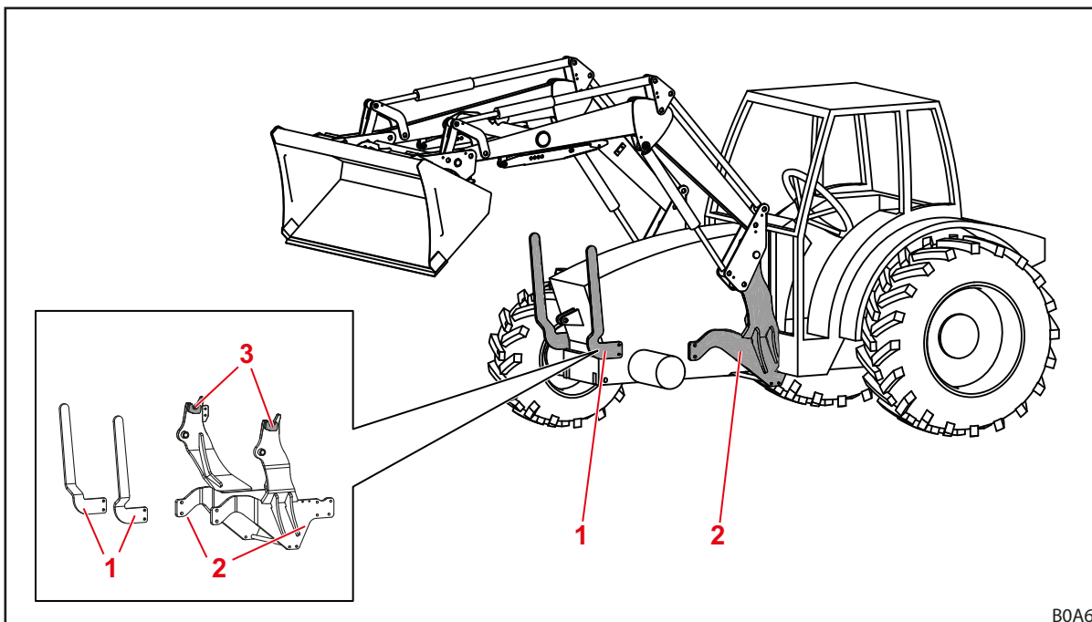
Obr. 15 Sada pre montáž pre traktor
