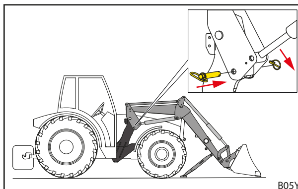
Obr. 56 Zastrčte zaistovacie čapy a zaistite ich sklopnými závlačkami
