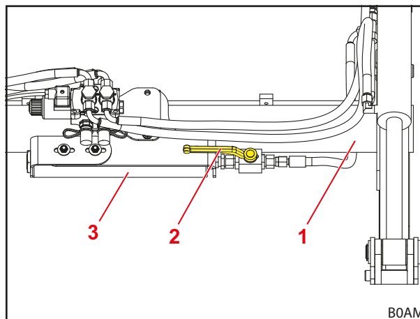
Obr. 47 Mechanicky ovládaný pohon Comfort Drive (poloha páky Comfort-Drive zap)
