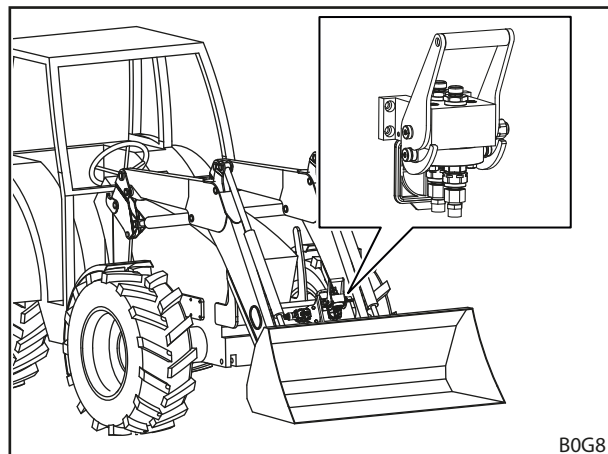
Obr. 23 Implement-Fix: pozícia na čelnom nakladači
