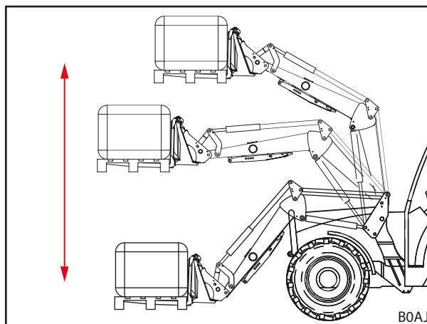
Obr. 34 Paralelné vedenie
