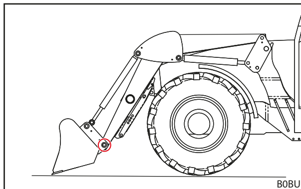
Obr. 105 Vyťahovanie dolných čapov
