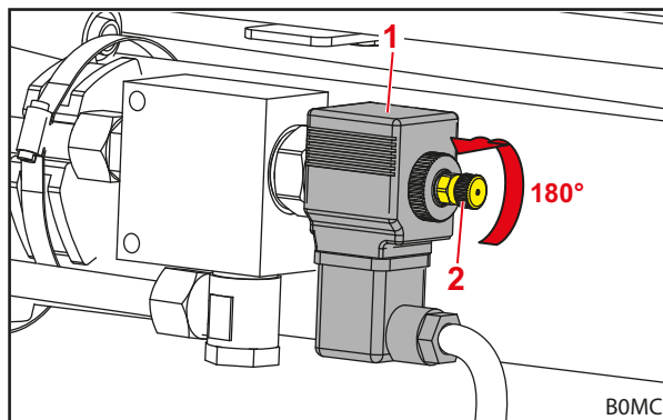
Obr. 35 Otvorenie ventilu
