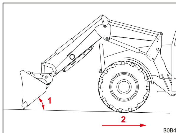
Obr. 107 Vyrovnávanie pôdy pri cúvaní
