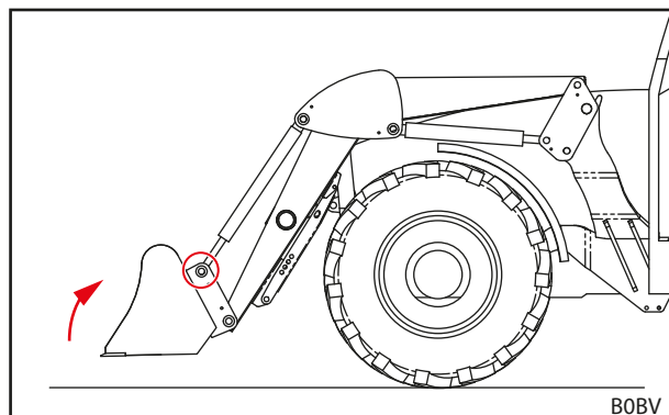
Obr. 96 Spojenie nástroja hore s hydraulickými valcami
