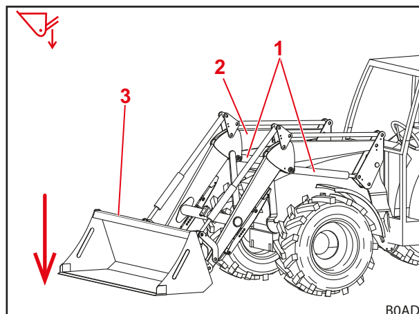
Obr. 29 Funkcia spúšťania
