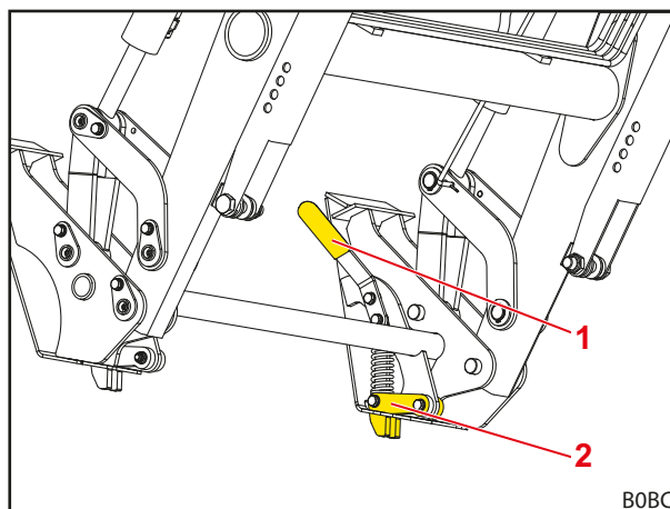
Obr. 78 Mechanické zaistenie nástroja Skid-Steer (zaistený stav bez nástroja)
