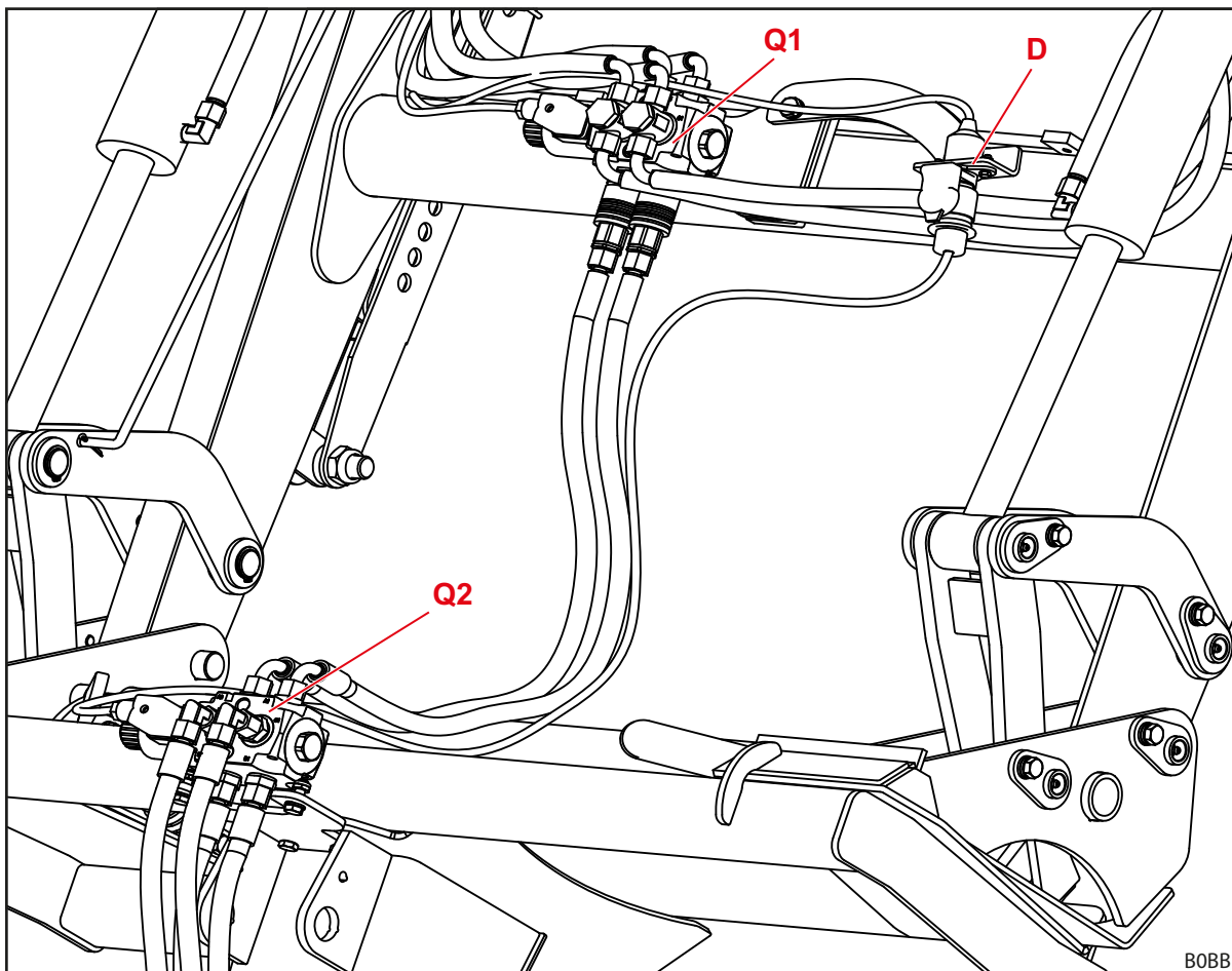
Obr. 124 Usporiadanie hydraulických ventilov pre prídavné funkcie
