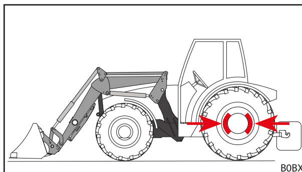
Obr. 99 Polohovanie nástroja na odloženie a zatiahnutie parkovacej brzdy
