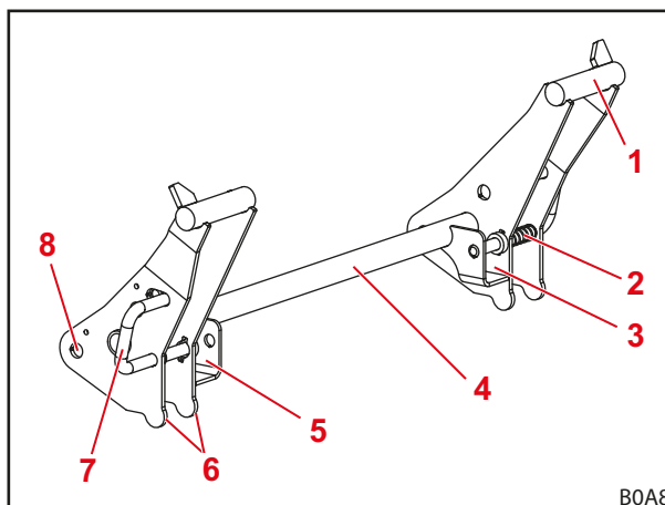
Obr. 17 Výmenný rám Euro
