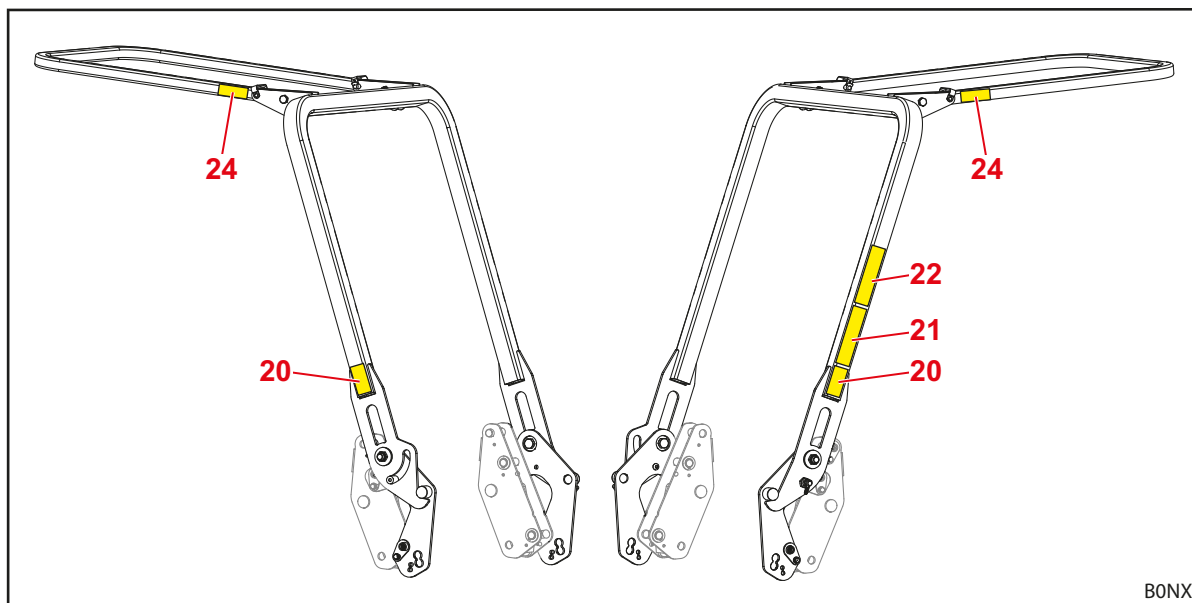
Obr. 7 Ochrana OPG pre traktory s vpredu umiestneným zariadením ochrany pred prevrátením s 2 stípmi (príkladný obrázok)
