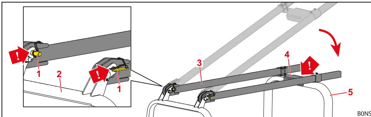
Obr. 42 Sklopené a v horných otvoroch zaistené traverzy
