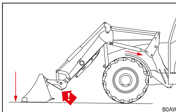
Obr. 82 Zatlačenie nástroja na zem
