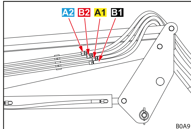
Obr. 18 Hydraulické vedenia
