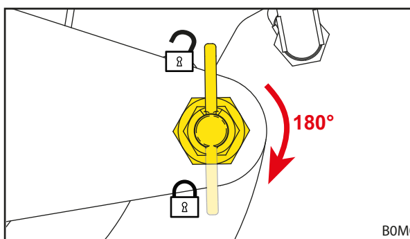
Obr. 37 Prestavenie zaisťovacej poistky do zablokovanej pozície
