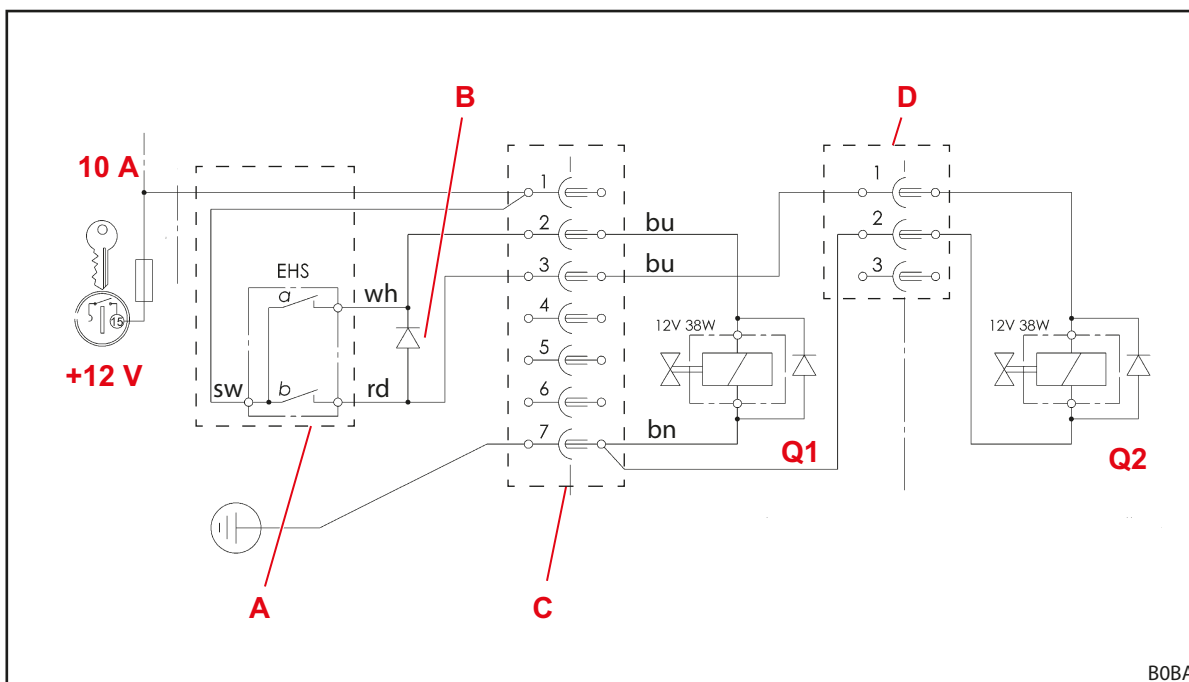
Obr. 123 Elektrická schéma zapojenia
