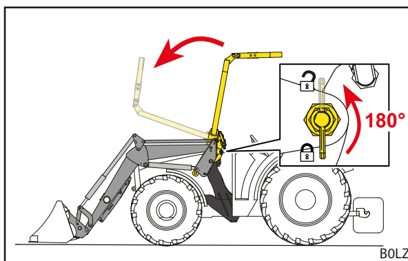
Obr. 36 Sklopenie ochrany OPG nadol
