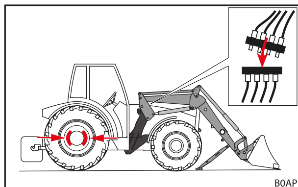
Obr. 54 Vypnutie traktora a pripojenie hydraulických vedení
