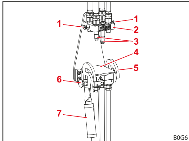
Obr. 70 Odpojené zaistenie Hydro-Fix
