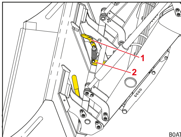
Obr. 77 Mechanické zaistenie nástroja Skid-Steer (zaistený stav s nástrojom)
