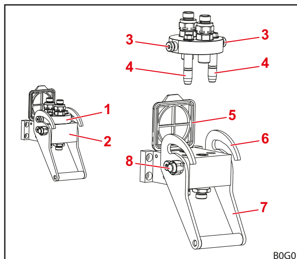
Obr. 24 Konštrukcia Implement-Fix
