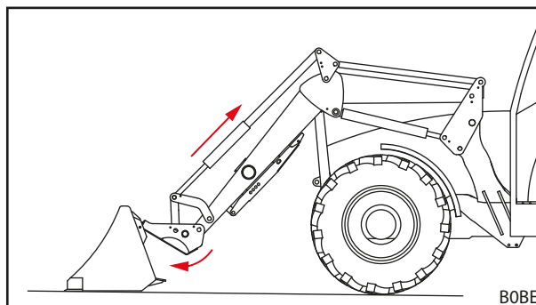
Obr. 86 Zaháknutie
