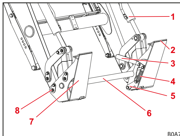
Obr. 16 Výmenný rám Skid-Steer
