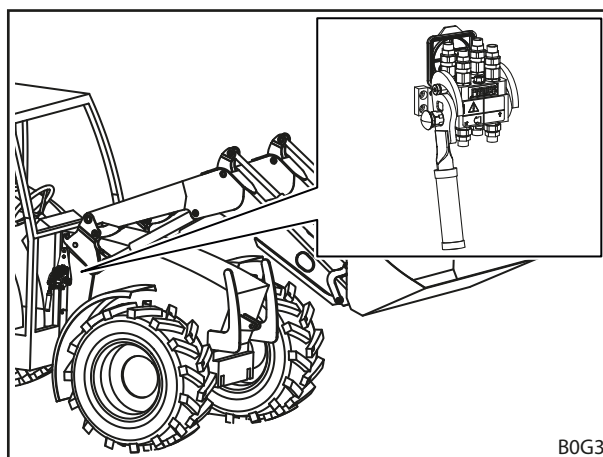
Fig. 21 Hydro-Fix: Poziția la încărcătorul frontal
