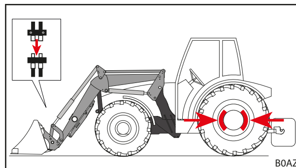
Fig. 88 Cuplarea circuitului de comandă
