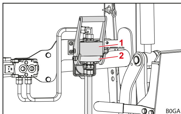
Fig. 73 Dispozitiv unealtă-fix cuplat
