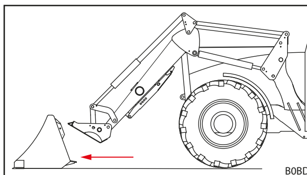
Fig. 84 Deplasare spre
