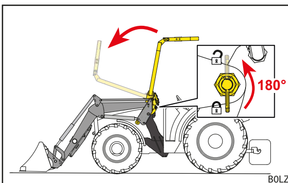
Fig. 36 Rabatare OPG în jos
