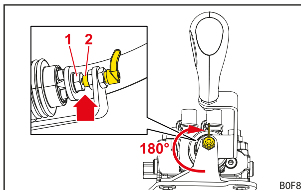
Fig. 64 Maneta de comandă blocată
