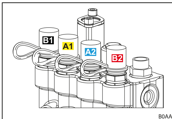
Fig. 20 Conectoarele cuplajelor tip fișă direct la supapa hidraulică
