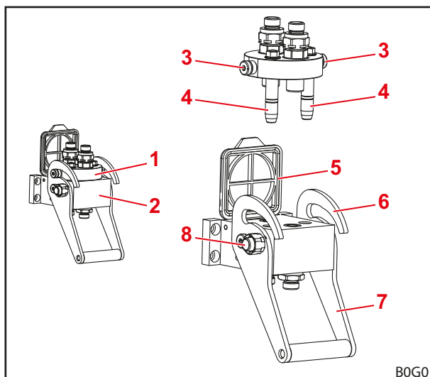
Fig. 24 Structură unealtă-Fix
