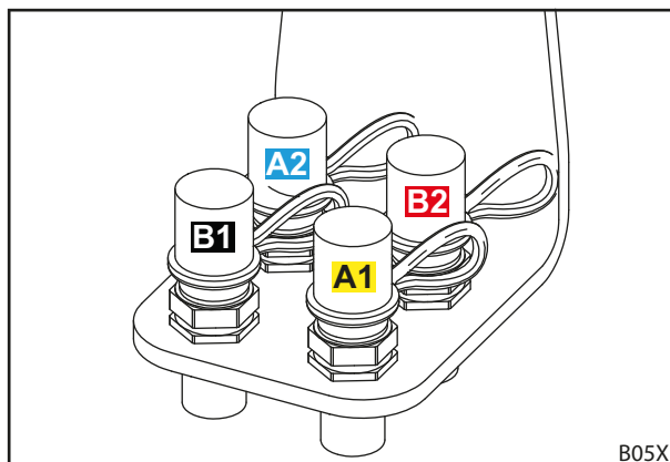
Fig. 19 Conectoarele cuplajelor tip fișă la piesa atașată
