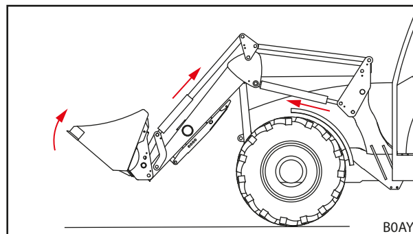
Fig. 87 Desfacerea dispozitivului de blocare a unelei
