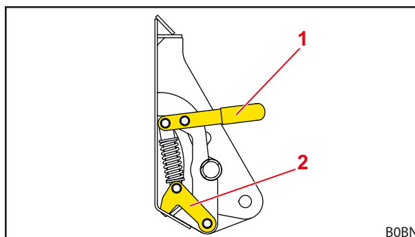
Fig. 74 Dispozitiv mecanic de blocare a uneltei Skid-Steer (starea deschisă)
