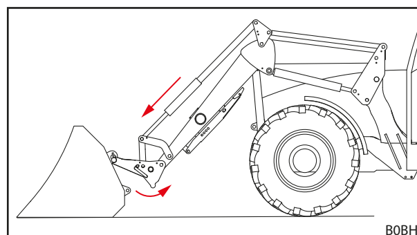
Fig. 101 Scoaterea din cârlig a cadrului de înlocuire
