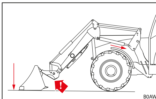
Fig. 82 Apăsați unealta pe sol
