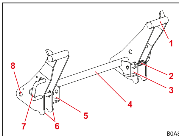
Fig. 27 Cadru de înlocuire Euro
