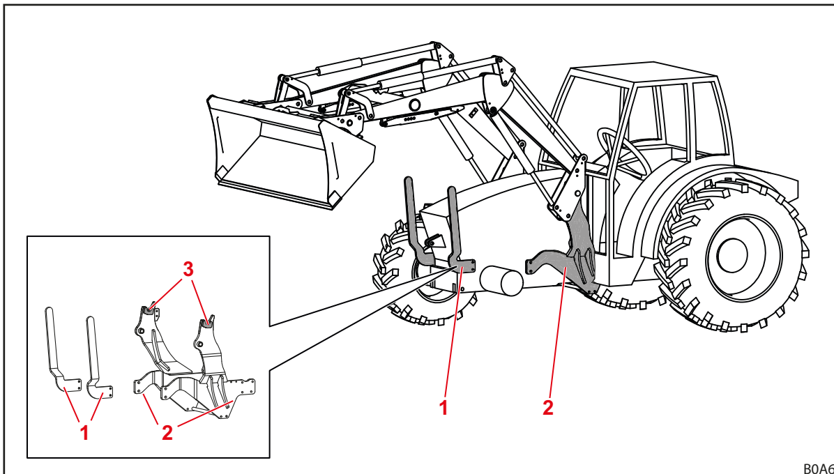
Fig. 15 Set de atașare pentru tractor
