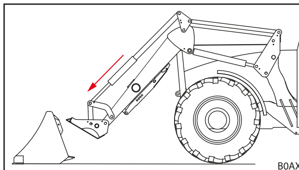
Fig. 85 Poziționarea brațului oscilant
