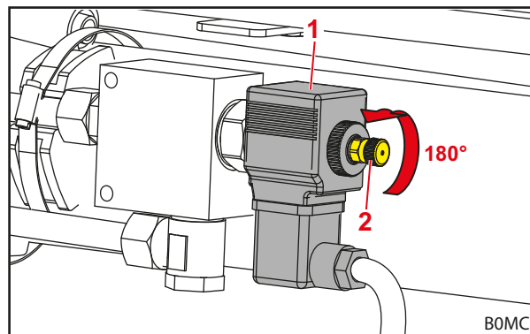
Fig. 35 Deschidere supapă
