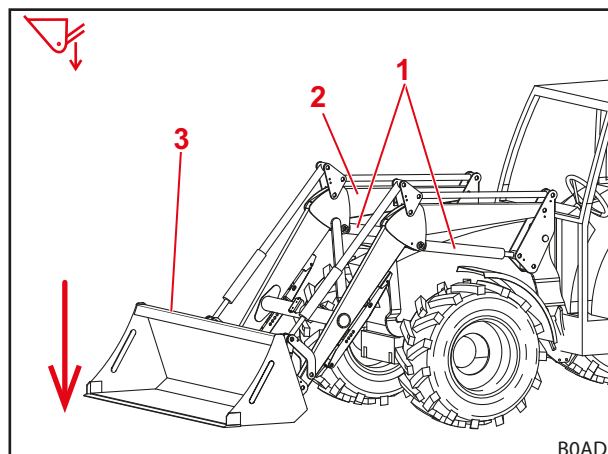
Fig. 29 Funcția Coborâre
