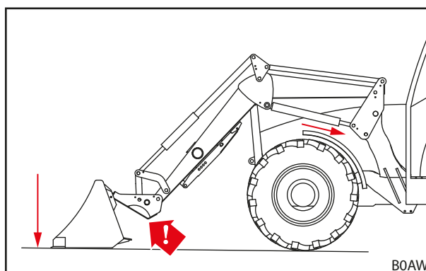
Fig. 79 Apăsați unealta pe sol
