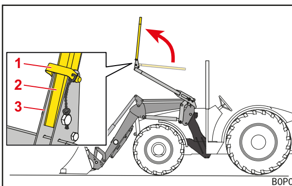
Fig. 44 Etrier superior rabatat în sus
