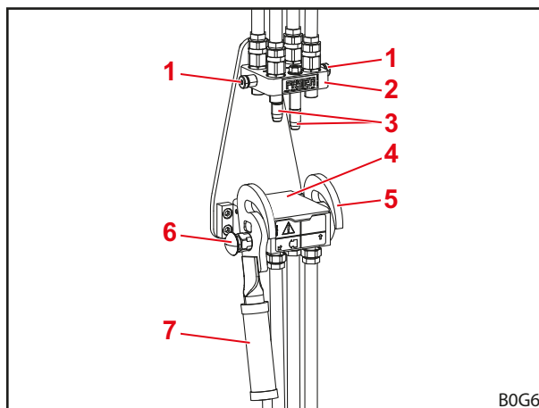
Fig. 70 Dispozitiv Hydro-fix decuplat
