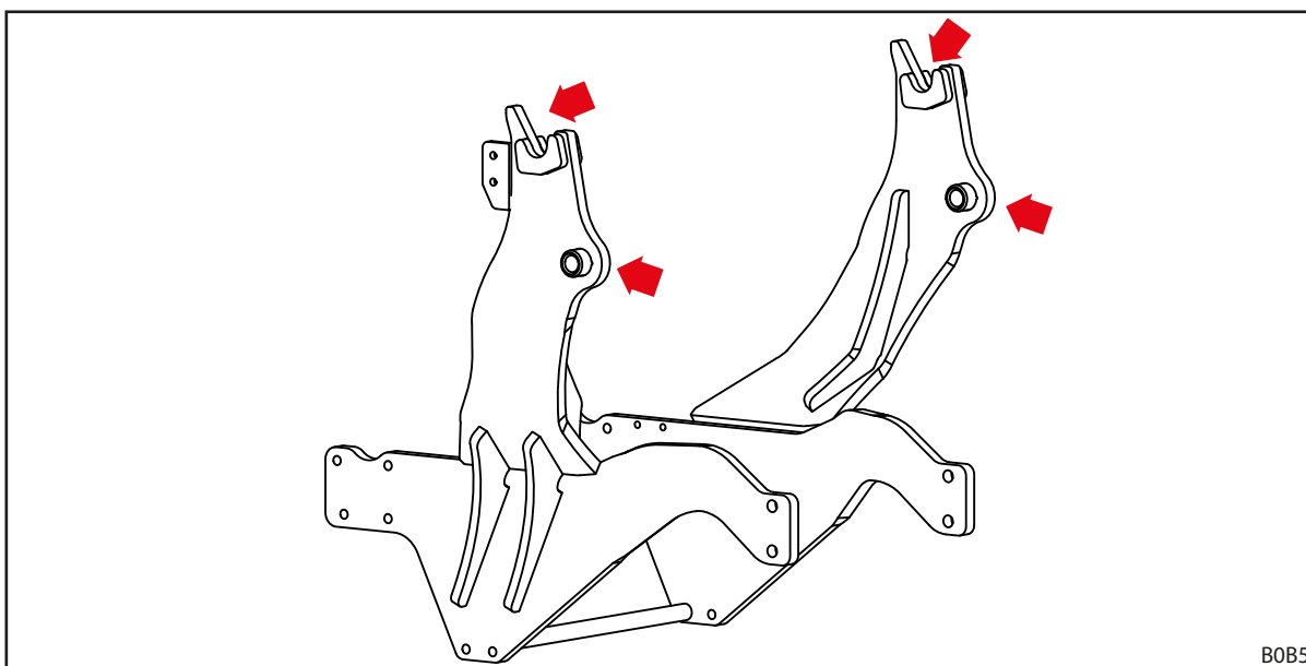
Fig. 113 Puncte de lubrifiere elemente de preluare încărcător frontal
