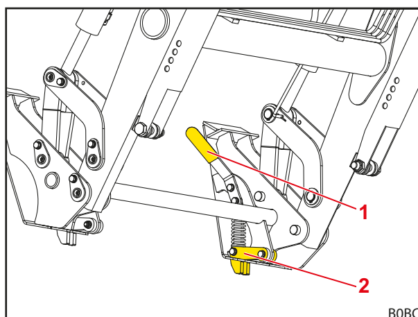
Fig. 78 Dispozitiv mecanic de blocare a uneltei Skid-Steer (starea blocată fără unealtă)
