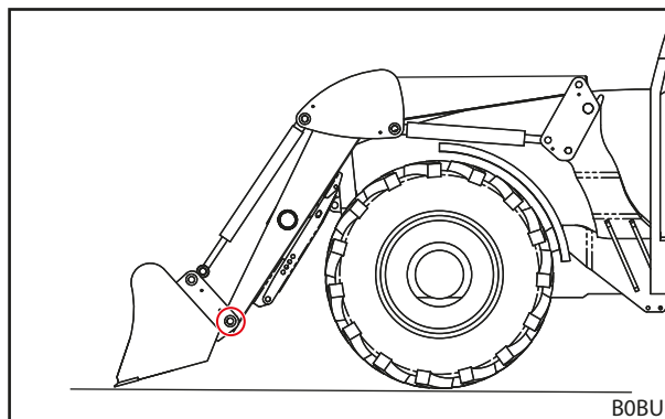
Fig. 95 Conectați unealta în orificiile inferioare de bolt
