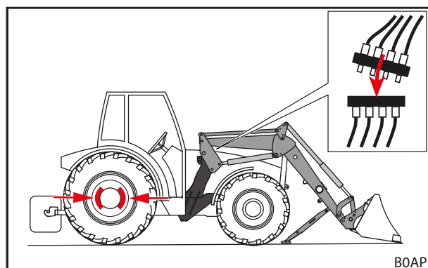
Fig. 54 Deconectarea tractorului și racordarea conductelor hidraulice
