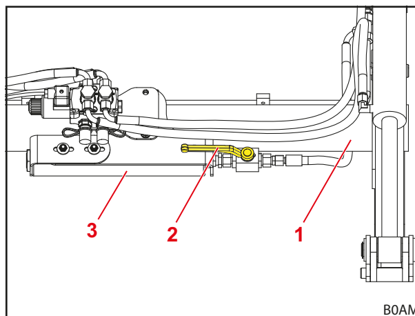
Fig. 47 Comfort Drive acționat mecanic (poziție manetă Comfort-Drive activată)
