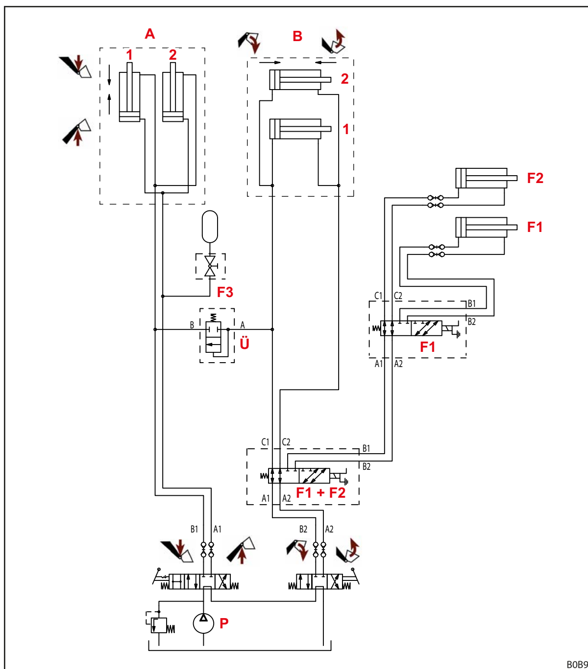
Fig. 122 Schema hidraulică FC
