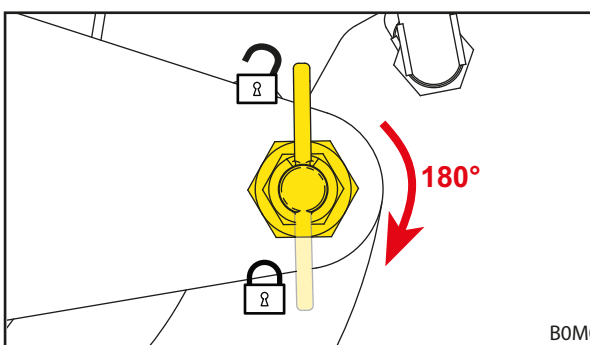
Fig. 37 Aducerea zăvorului de înclichetare în poziția blocat
