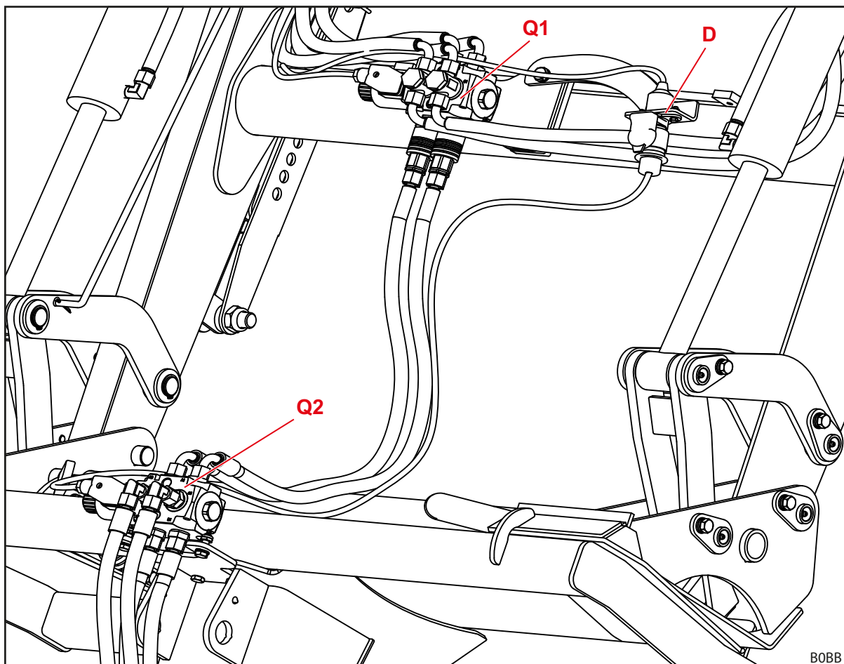
Fig. 124 Dispunerea supapelor hidraulice pentru funcțiile suplimentare
