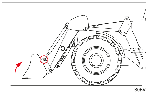
Fig. 96 Conectarea unelei sus cu cilindrul hidraulic
