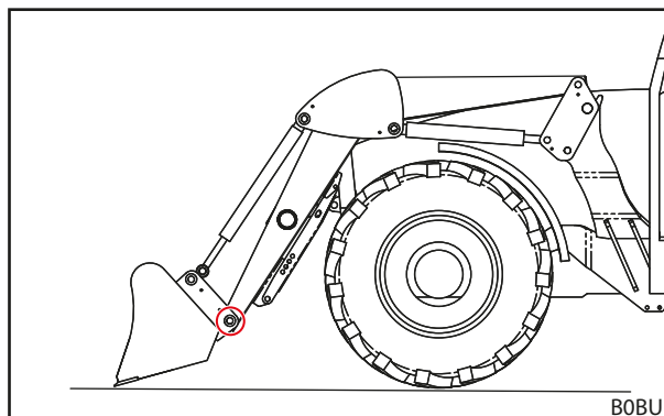
Fig. 105 Scoaterea prin tragere în afară a bolțurilor de jos
