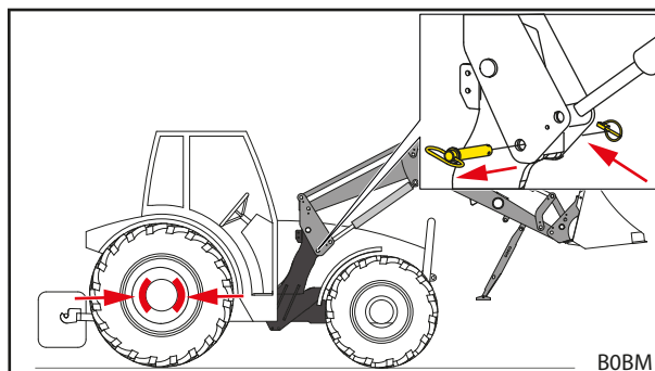
Fig. 118 Trageți frâna de parcare și desfaceți dispozitivul de blocare al încărcătorului frontal
