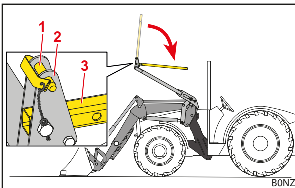
Fig. 43 Etrier superior rabatat în jos
