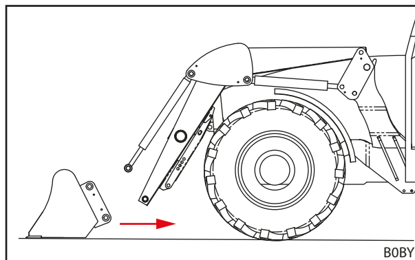
Fig. 106 Deplasare de îndepărtare
