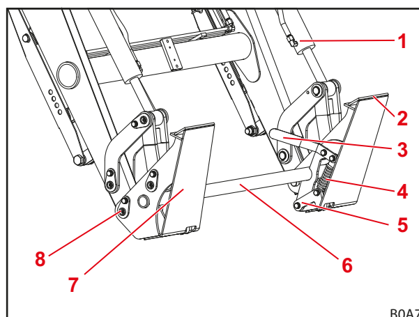
Fig. 16 Cadru de înlocuire Skid-Steer
