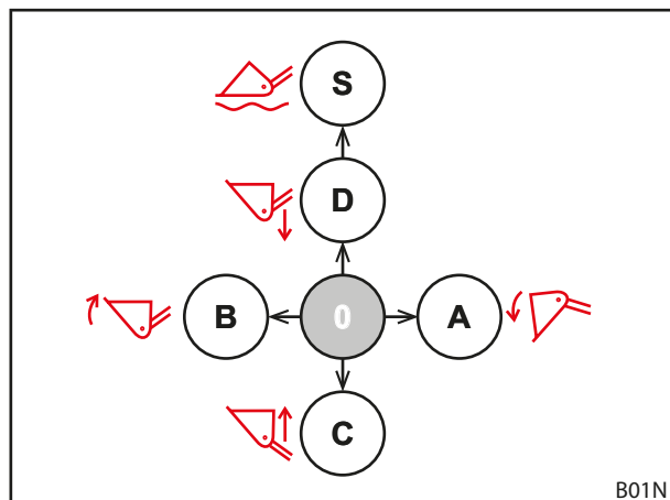
Fig. 58 Alocare la o manetă de comandă
