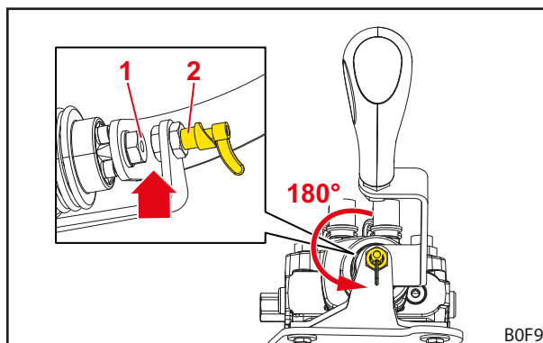
Fig. 65 Maneta de comandă deblocată
