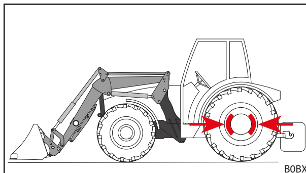
Fig. 99 Poziționați unealta pentru depunere și trageți frâna de imobilizare
