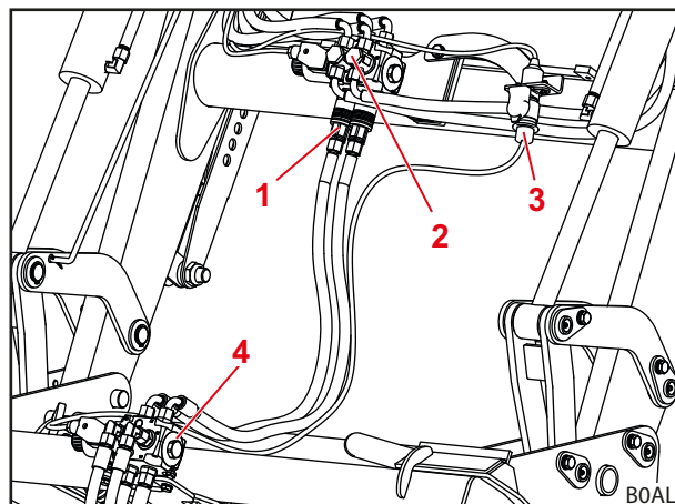
Fig. 46 Al 4-lea circuit de comandă suplimentar
