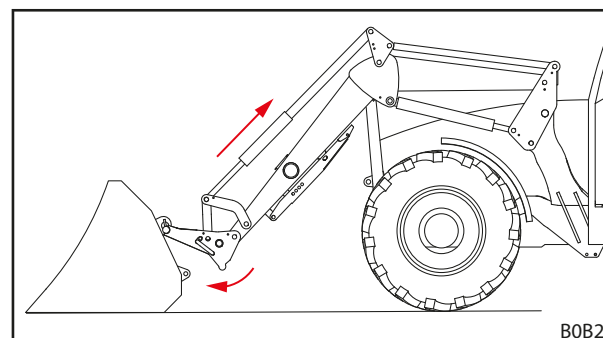
Fig. 91 Introducerea în cârlig
