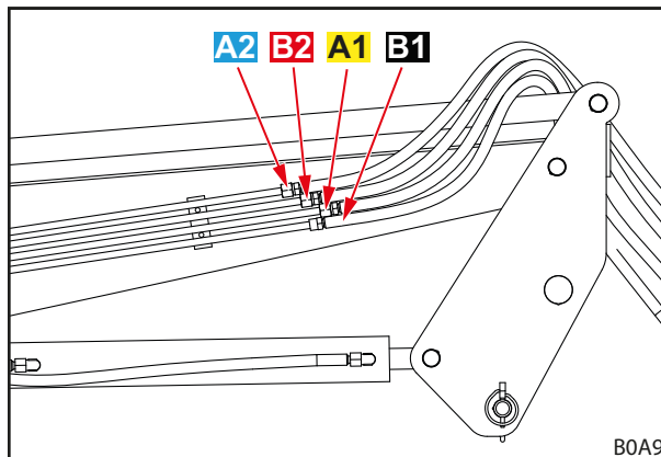
Fig. 18 Conductele hidraulice
