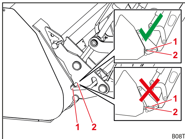
Fig. 81 Verificarea poziției bolțurilor de blocare
