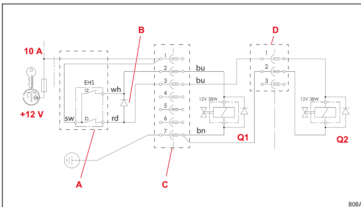
Fig. 123 Schema circuitelor electrice
