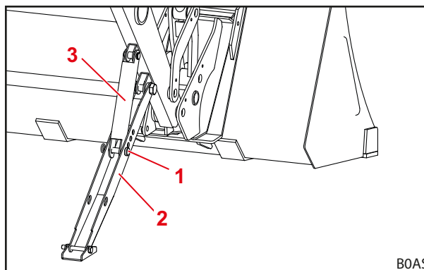
Fig. 68 Picioarele de sprijin rabatate deschis
