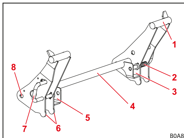
Fig. 80 Dispozitivul de blocare a uneltei la cadrul de înlocuire Euro
