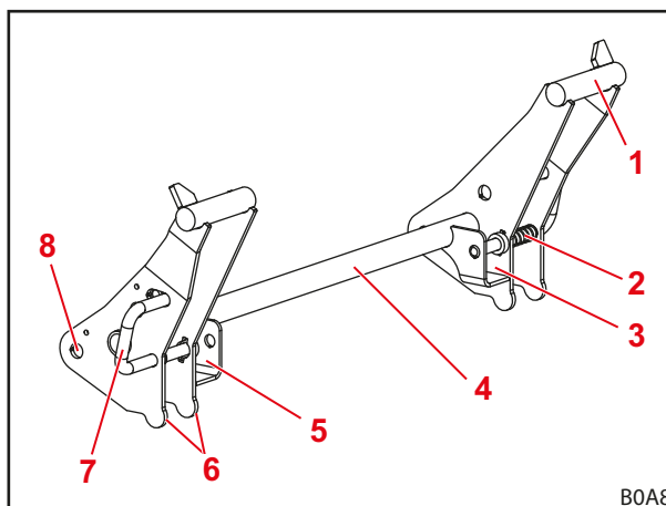
Fig. 17 Cadru de înlocuire Euro
