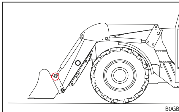
Fig. 104 Scoaterea prin tragere în afară a bolțurilor de sus
