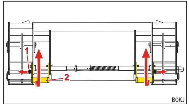
Pav. 91 Prispaudiklių pasukimas į viršų
