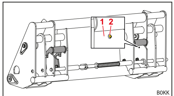
Pav. 92 Pasukti į viršų prispaudikliai (vaizdas iš galo)
