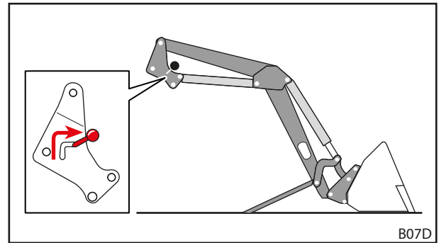
Pav. 53 Priekinio krautuvo fiksatoriaus atidarymas
