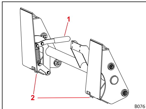
Pav. 87 Padargo fiksatorius ant keičiamojo rėmo „Skid-Steer“
