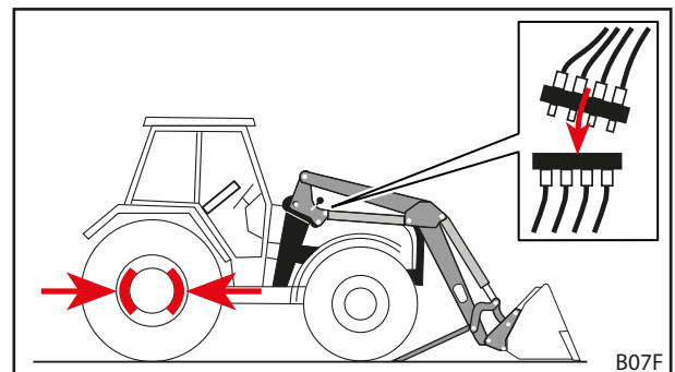
Pav. 55 Traktoriaus išjungimas ir hidraulinių linijų prijungimas
