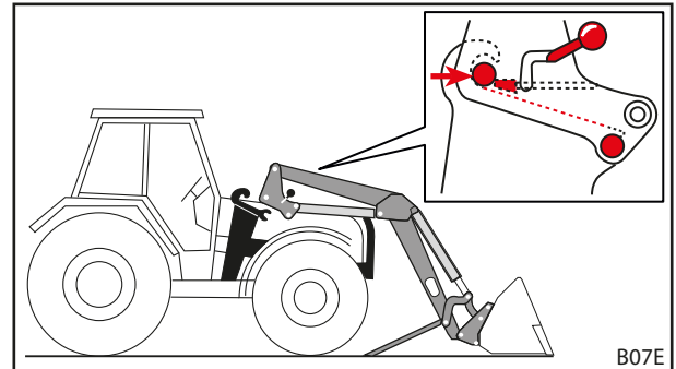
Pav. 54 Traktoriaus įvažiavimas į strėlę
