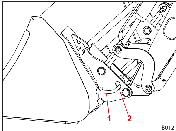
Pav. 82 Mechaninis padargo fiksatorius
