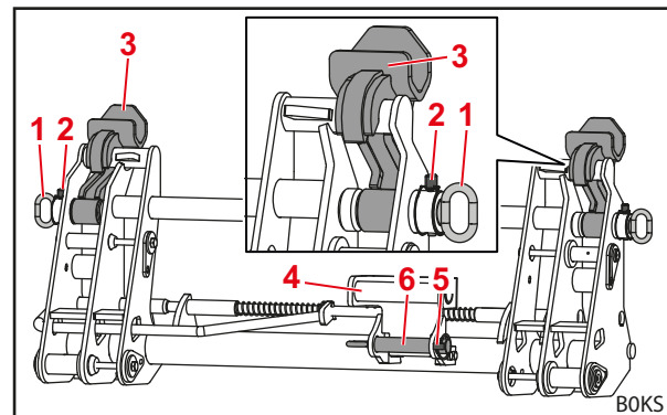
Pav. 94 Adapteris darbo padėtyje (keičiamasis rėmas paruoštas FR padargui)
