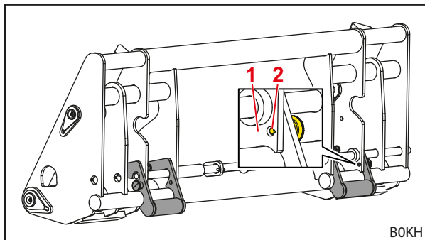
Pav. 90 Pasukti į apačią prispaudikliai
