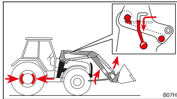
Pav. 58 Statymo atramų užlenkimas ir priekinio krautuvo fiksatoriaus uždarymas
