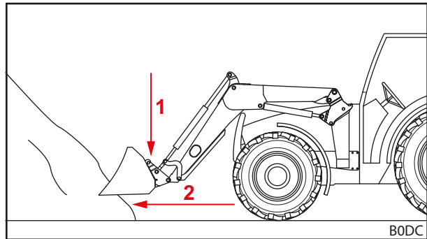
Pav. 111 Priekinio krautuvo nuleidimas ir įvažiavimas tiesiai į krovinį
