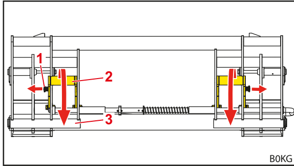
Pav. 89 Prispaudiklių pasukimas į apačią
