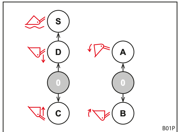
Pav. 65 Paskirstymas, kai yra dvi valdymo svirtys
