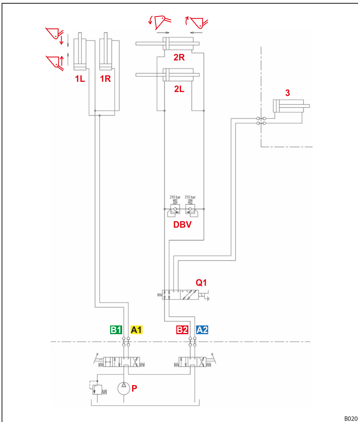
Pav. 127 P hidraulinės sistemos schema
