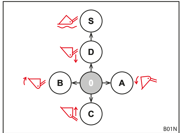
Pav. 64 Paskirstymas, kai yra viena valdymo svirtis
