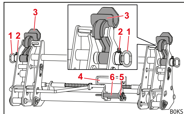
Mynd 94 Millistykki í vinnslustöðu (skiptigrind undirbúin fyrir FR-verkfæri)
