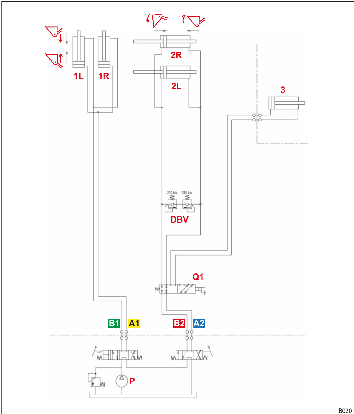
Mynd 127 Yfirlitsmynd af vökvakerfi P
