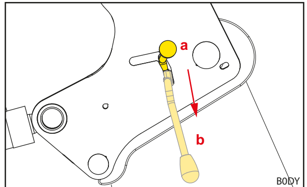
Mynd 62 Læsiarmurinn spennur
