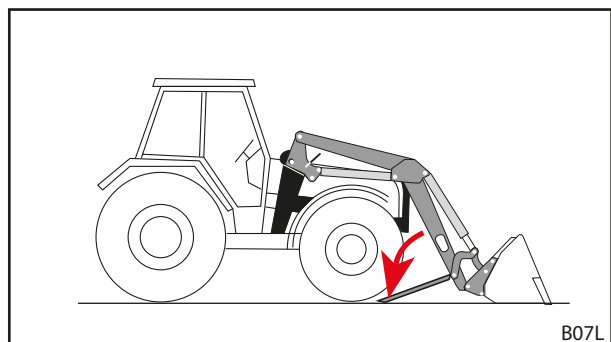
Mynd 123 Stoðfætur settir niður
