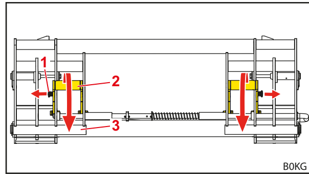
Mynd 89 Stoðirnar færðar niður
