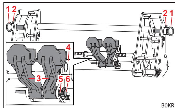
Fig. 93 Adapter op parkeerpositie (wisselframe voorbereid voor Euro-werktuig)
