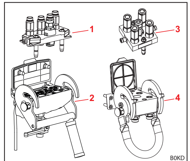
Fig. 25 Opbouw Hydro-Fix en multikoppeling
