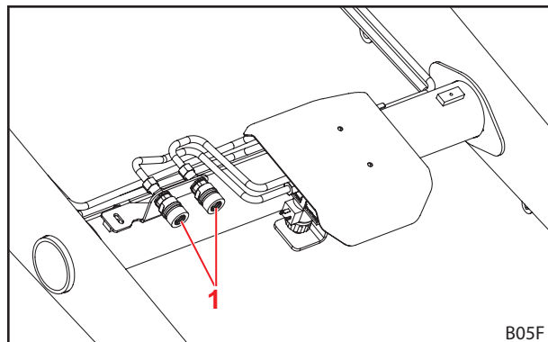
Fig. 45 Bijkomende 3e stuurkring
