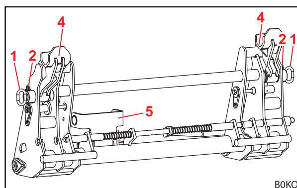
Fig. 21 Kombi-wisselframe Euro-FR (voorbereid voor FR-werktuig)
