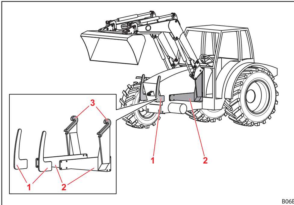
Fig. 14 Montageset voor tractor
