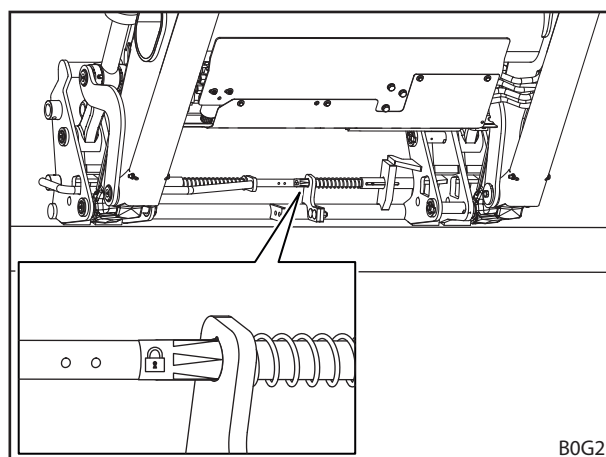
Fig. 84 Werktuigvergrendeling controleren aan de hand van de sticker (combiwisselframe Euro-FR)
