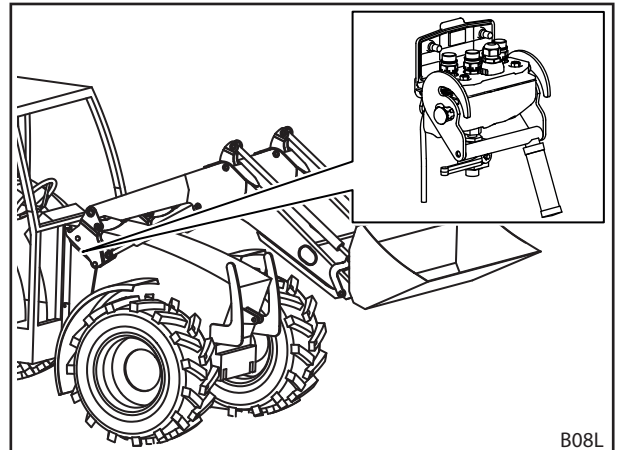
Fig. 24 Hydro-Fix: positie aan de frontlader
