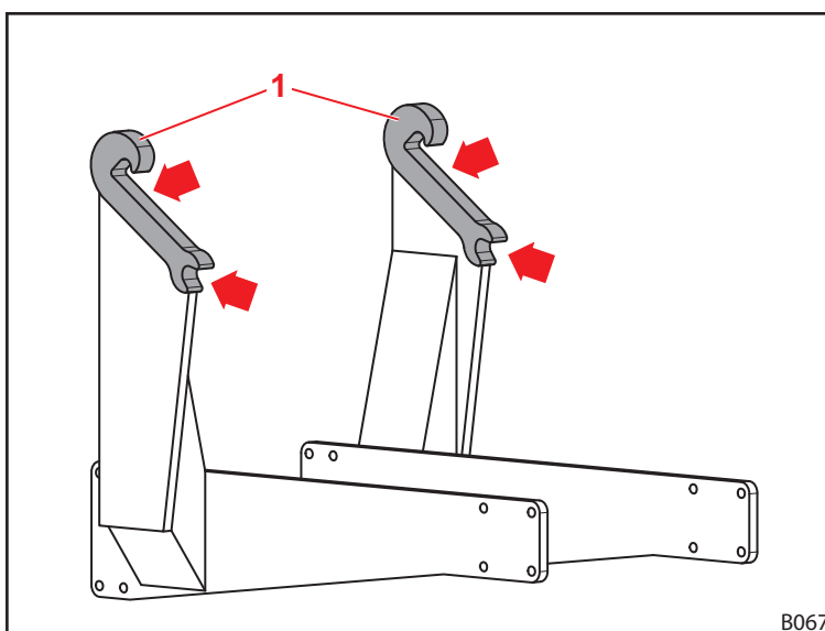
Fig. 115 Smeerpunten frontlader-opneempunten
