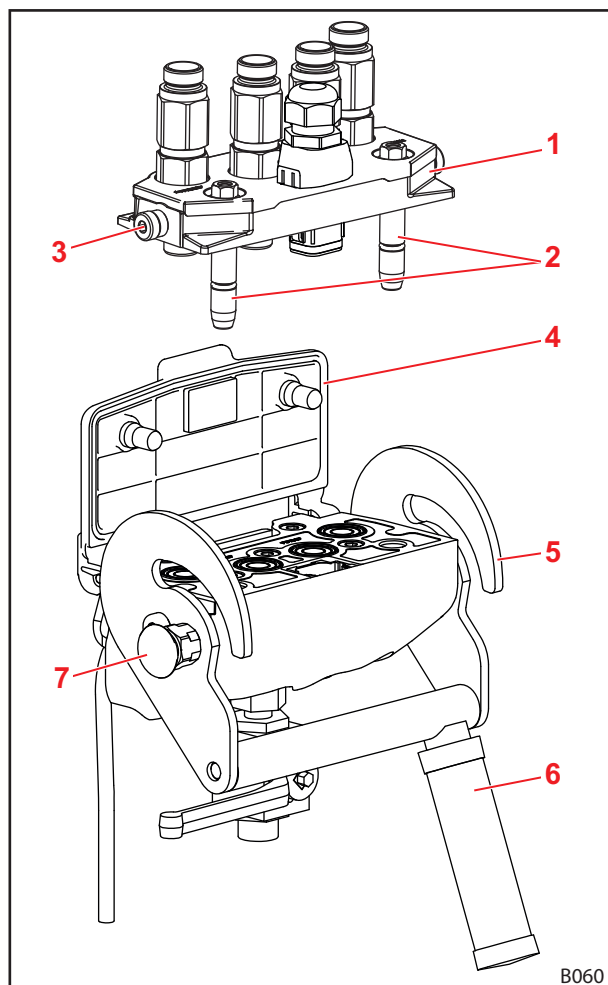
Fig. 81 Hydro-Fix (voorbeeld: Hydro-Fix 4-voudig)
