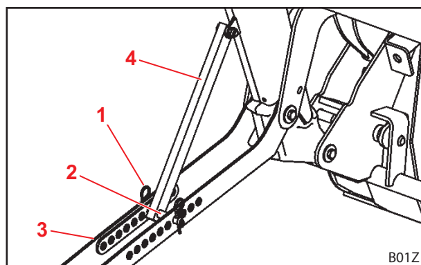
Fig. 78 Parkeersteun
