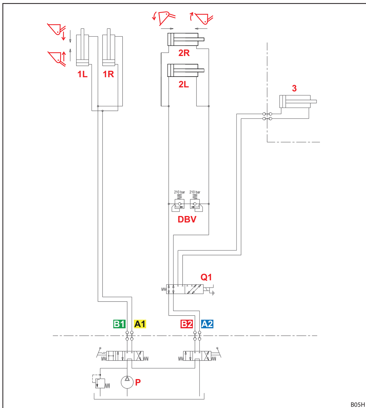
Fig. 126 Hydraulisch schema H
