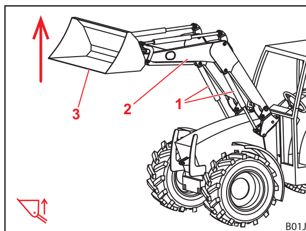
Fig. 28 Optillen-functie
