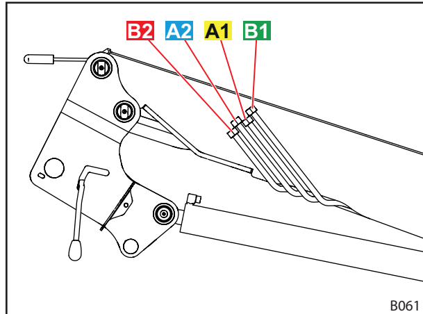
Fig. 22 Hydraulische leidingen
