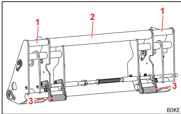
Fig. 17 Combi-wisselframe Euro-SMS (voorbereid voor Euro-werktuig)
