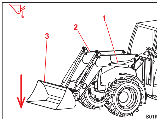
Fig. 29 Neerlaten-functie
