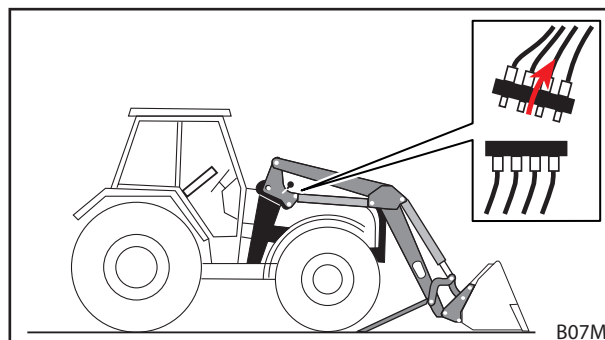
Fig. 124 Hydraulica afkoppelen
