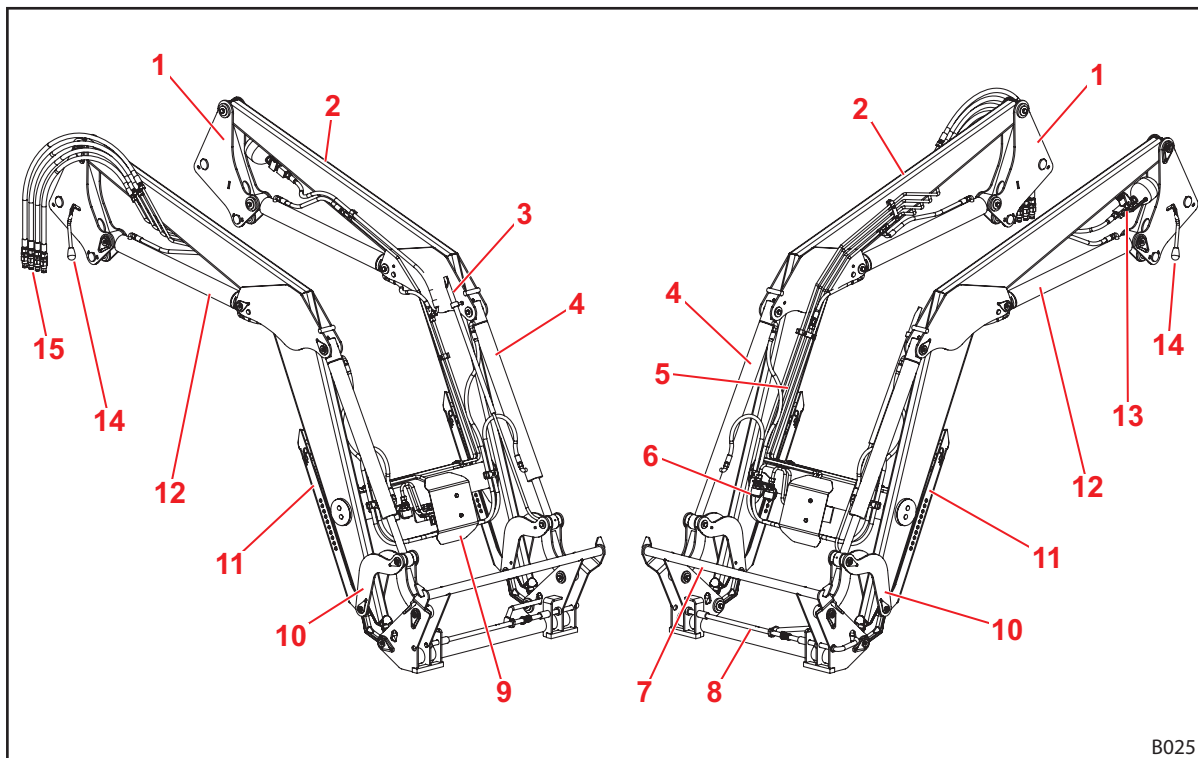
Fig. 10 Frontlader H (zonder mechanische parallelgeleiding)
