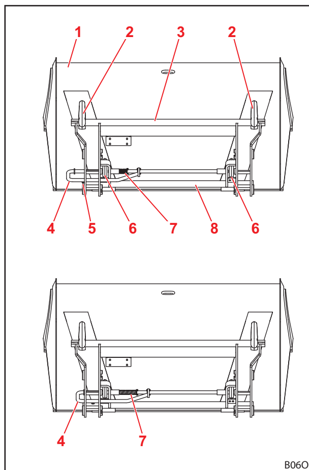
Fig. 26 Geopende (boven) en gesloten (onder) vergrendeling
