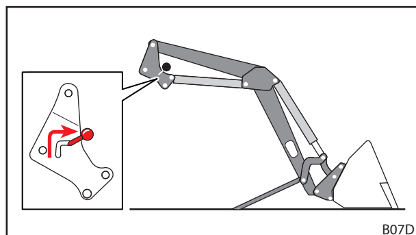
Fig. 53 Frontlader-vergrendeling openen
