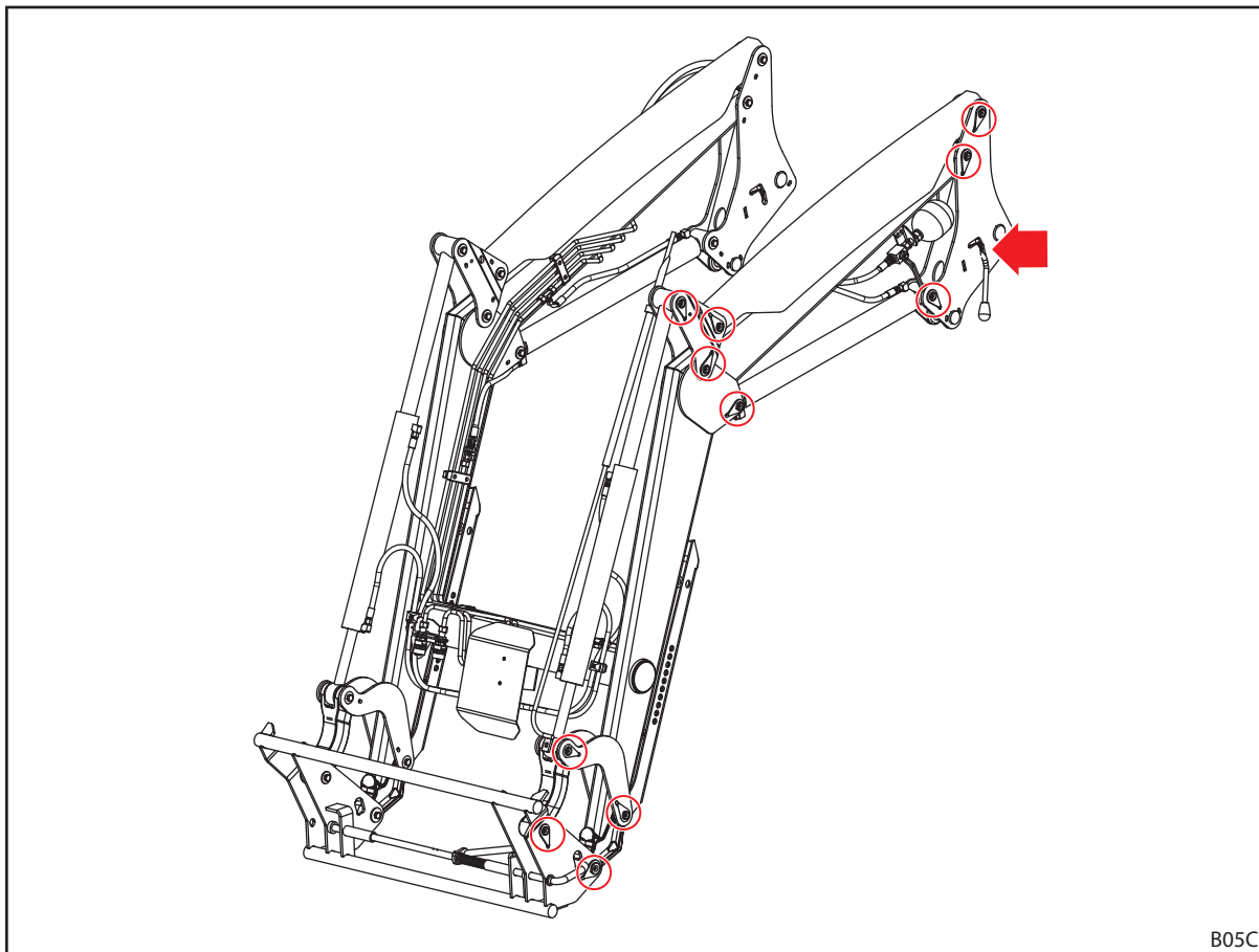
Fig. 117 Smeerpunten P
