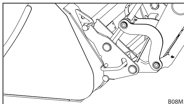
Fig. 95 Werktuigvergrendeling openen
