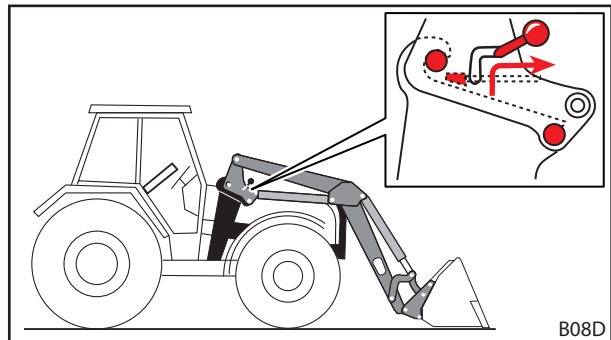
Fig. 122 Frontlader-vergrendeling losmaken
