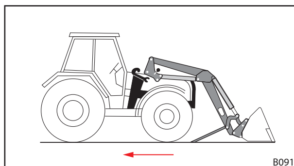
Fig. 125 Tractor achteruit verwijderen
