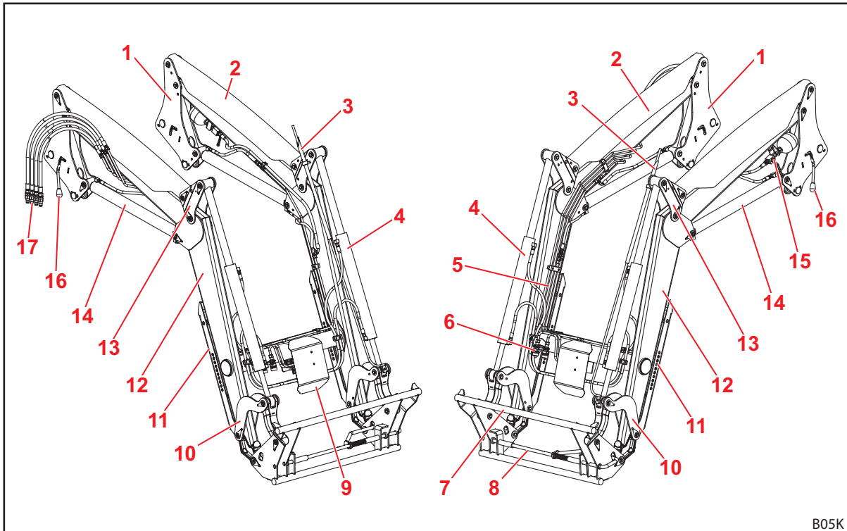
Fig. 11 Frontlader P (met mechanische parallelgeleiding)
