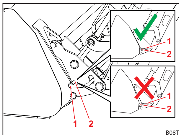
Fig. 85 Positie van de vergrendelingspennen controleren
