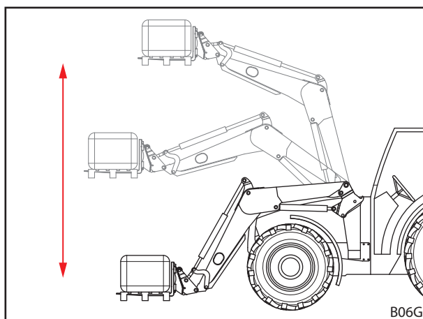
Fig. 34 Mechanische parallelgeleiding
