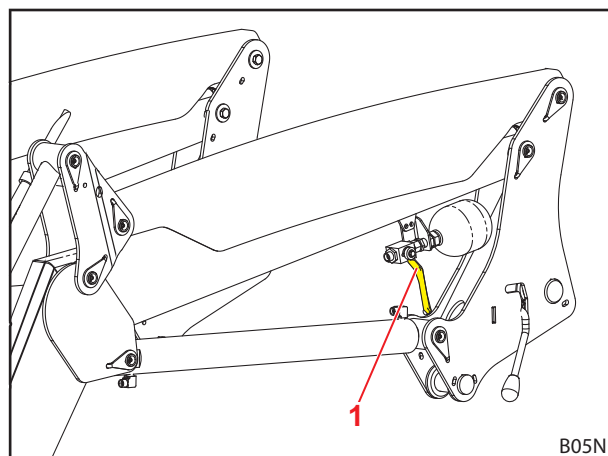
Fig. 47 Mechanisch bediende Comfort-Drive
