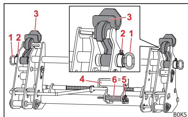
Fig. 94 Adapter op werkpositie (wisselframe voorbereid voor FR-werktuig)
