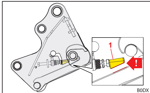
Fig. 59 Correcte inbouwpositie van de klamp
