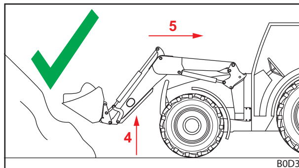
Fig. 114 Achteruit rijden onder last – juist
