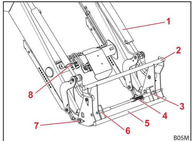
Fig. 15 Euro-wisselframe
