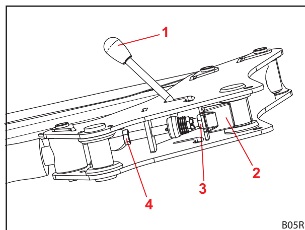
Fig. 63 Onderaanzicht van de frontlader-vergrendeling
