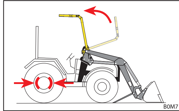
Fig. 56 OPG omhoog klappen
