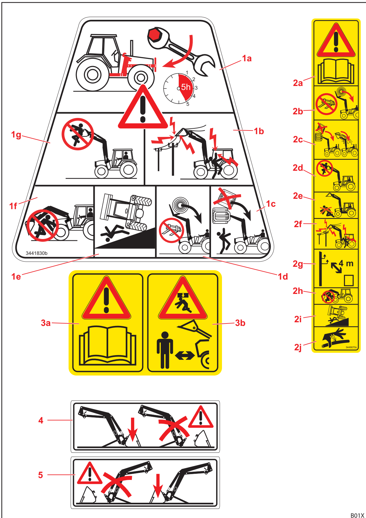
Fig. 5 Veiligheidsstickers positie 1-5
