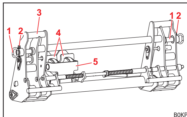
Fig. 20 Kombi-wisselframe Euro-FR (voorbereid voor Euro-werktuig)
