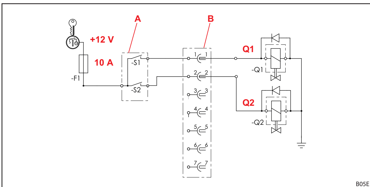
Fig. 128 Elektrisch schakelschema
