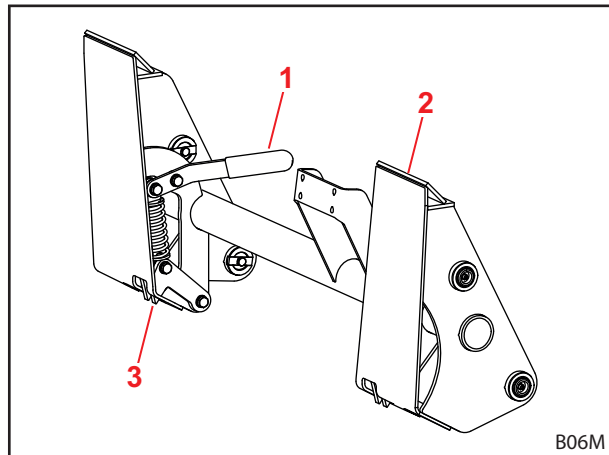
Fig. 27 Mechanische werktuigvergrendeling aan het Skid-Steer-wisselframe
