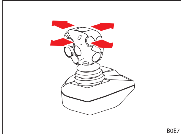
Fig. 75 Joystick naar alle eindposities bewegen
