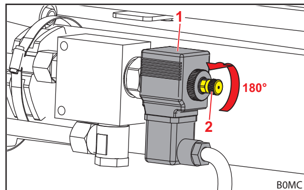
Fig. 35 Ventiel openen
