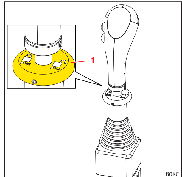
Fig. 68 Vergrendeling van de bedieningshendel (verticale vergrendeling)
