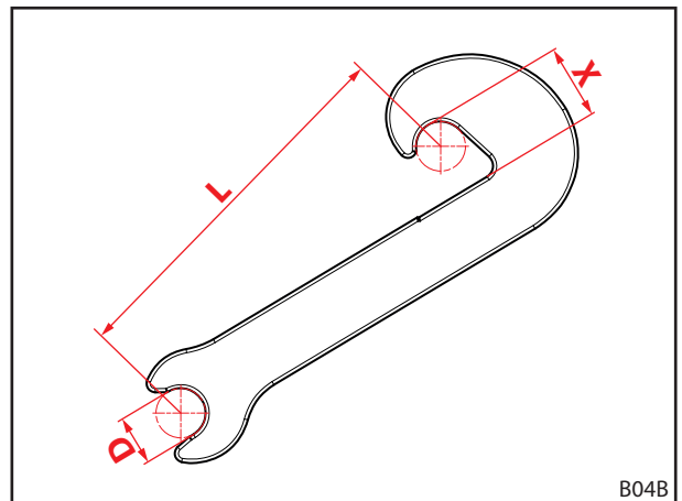
Fig. 118 Slijtagematen van de vanghaak
