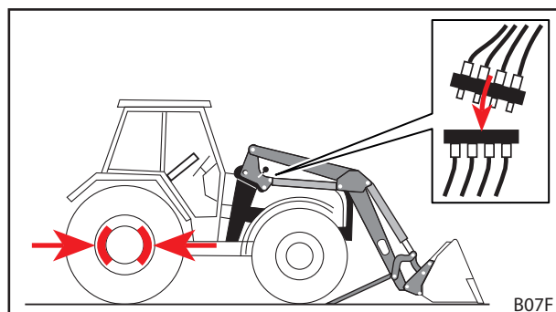
Fig. 55 Tractor uitschakelen en hydraulische leidingen aansluiten
