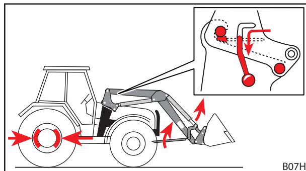
Fig. 58 Parkeersteunen inklappen en frontlader-vergrendeling sluiten
