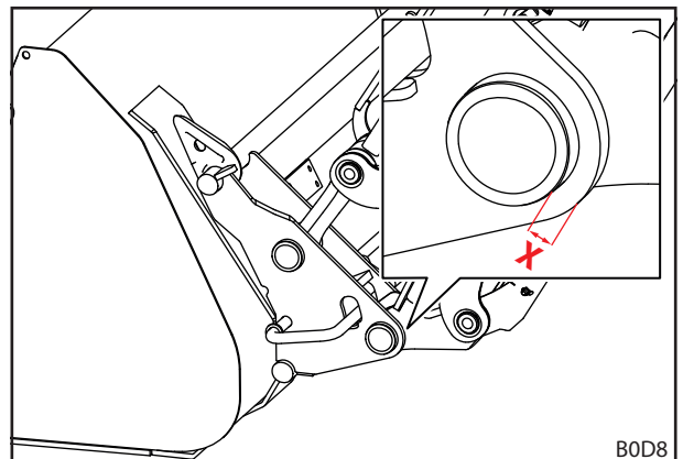
Fig. 120 Slijtagemaat van het wisselframe
