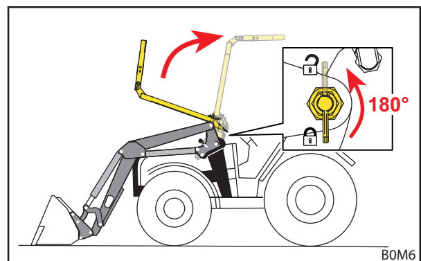
Fig. 38 OPG omhoog klappen
