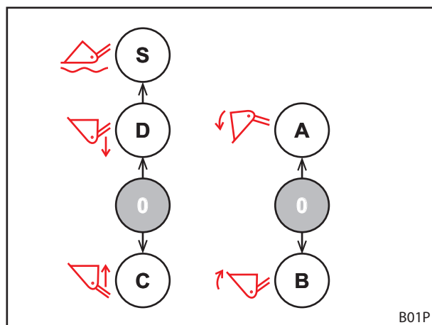
Fig. 65 Configuratie bij twee bedieningshendels
