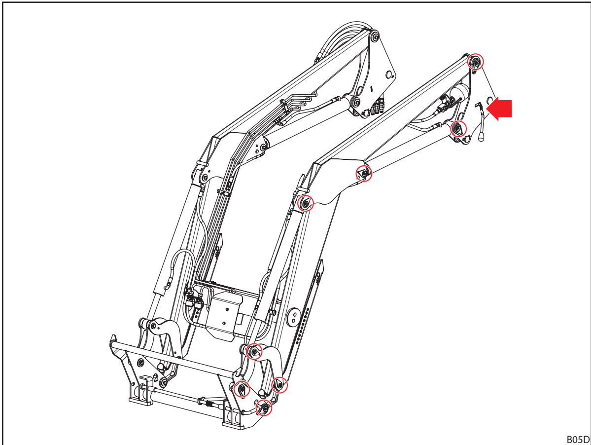
Fig. 116 Smeerpunten H
