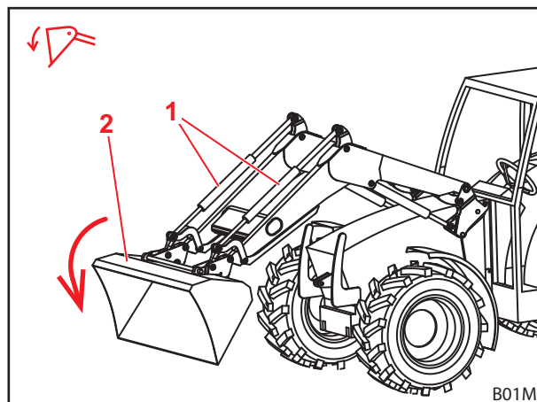
Fig. 31 Storten-functie
