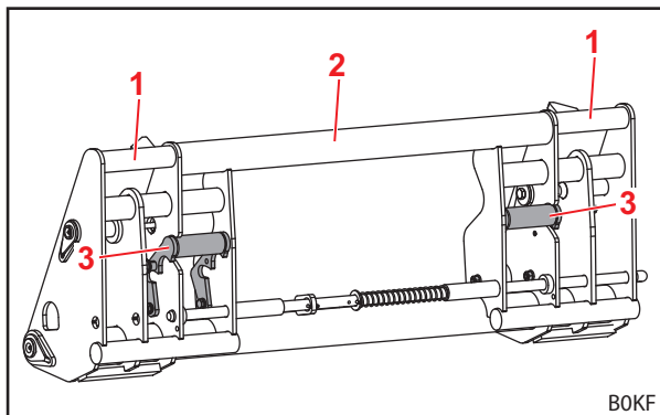
Fig. 18 Combi-wisselframe Euro-SMS (voorbereid voor SMS-werktuig)
