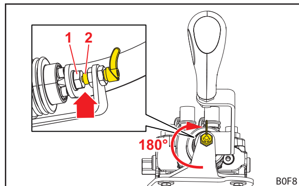
Fig. 71 Vergrendelde bedieningshendel
