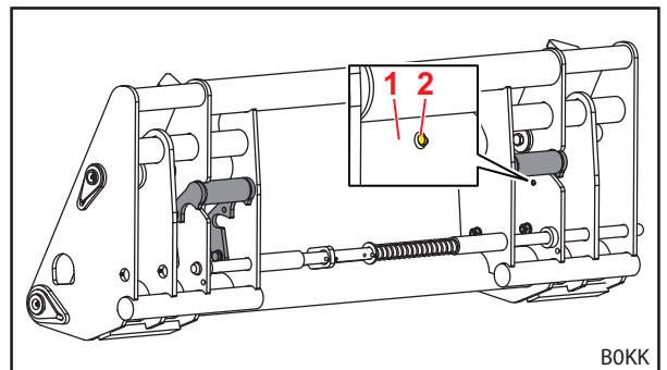
Fig. 92 Omhoog geklapte installaties (achteraanzicht)
