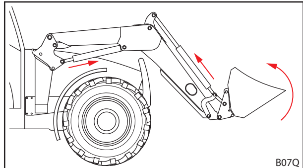
Fig. 99 Werktuigvergrendeling activeren
