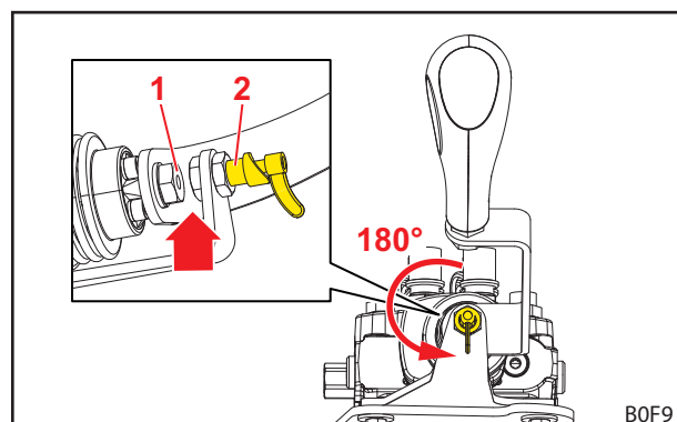
Fig. 72 Ontgrendelde bedieningshendel
