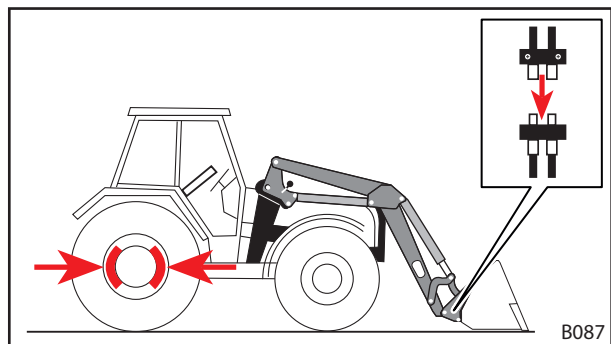
Fig. 100 Hydraulische leidingen van het werktuig verbinden met frontladerkoppelingen
