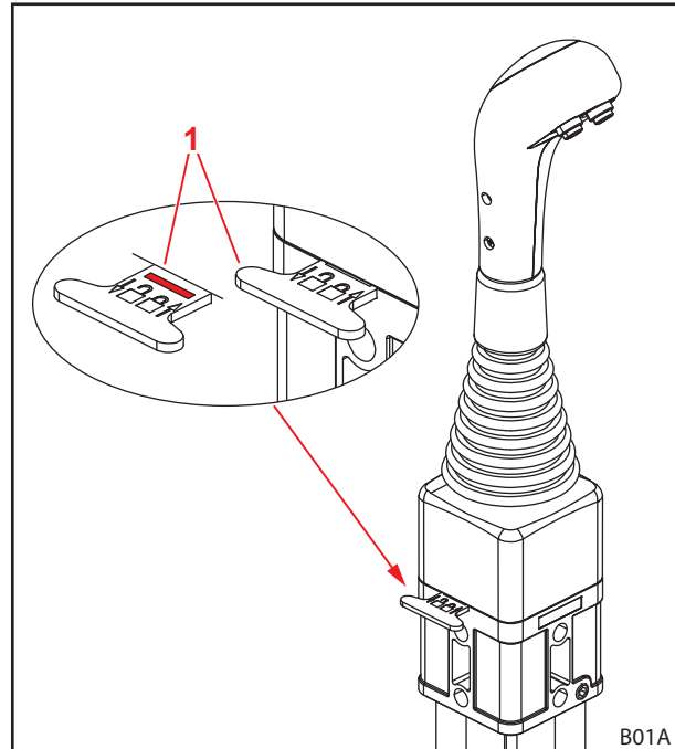
Fig. 67 Vergrendeling van de bedieningshendel (horizontale vergrendeling)
