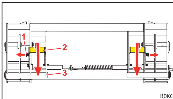
Fig. 89 Installaties neerklappen
