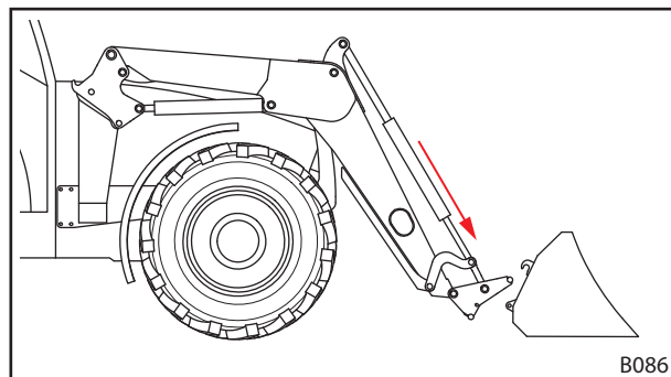
Fig. 96 Arm positioneren
