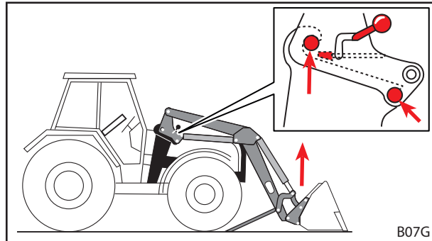
Fig. 57 Optillen-functie gebruiken tot de frontladerpennen in de vanghaken liggen
