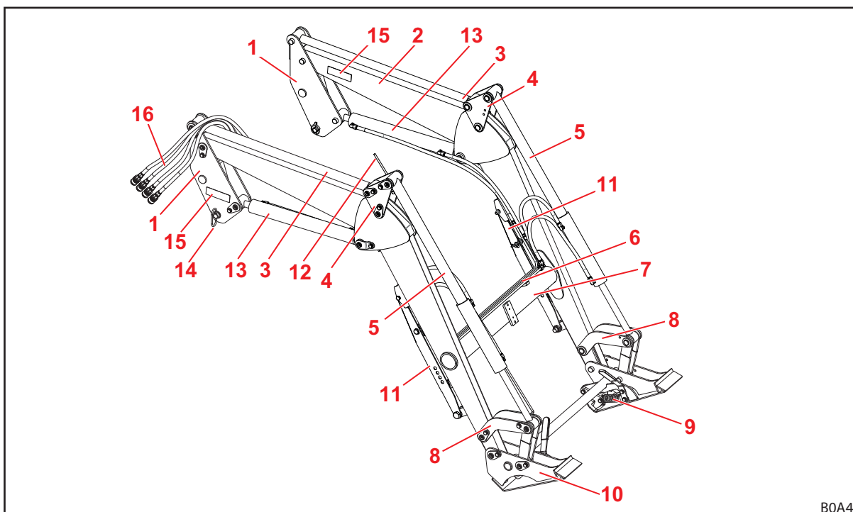
Fig. 11 Frontlader P (voorbeeld)
