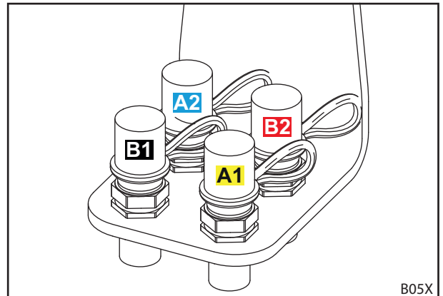
Fig. 19 Stekkers van de steekkoppelingen op het aanbouwdeel
