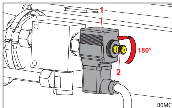
Fig. 35 Ventiel openen
