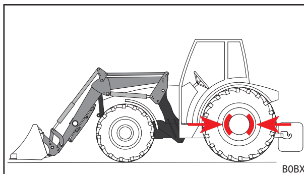
Fig. 103 Werktuig positioneren voor het neerleggen en parkeerrem aantrekken
