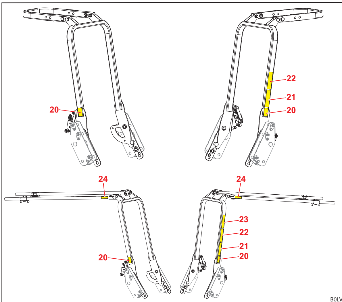
Fig. 6 OPG voor tractoren met achter gemonteerde Kantelbeveiliging met 2 poten (afbeelding als voorbeeld)
