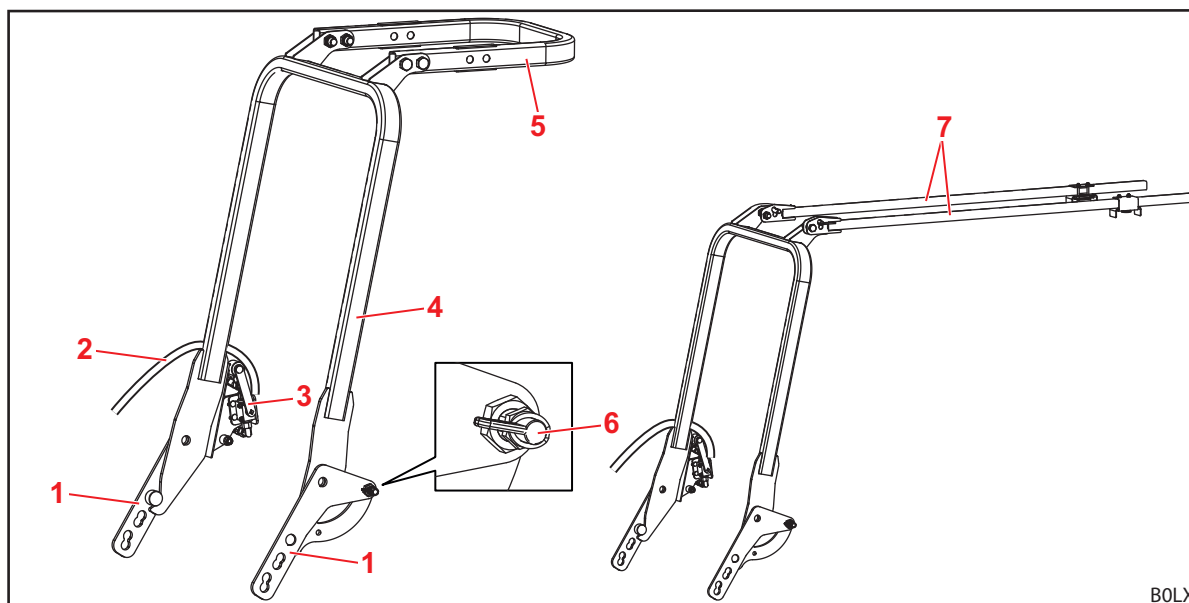
Fig. 12 Operator Protective Guard, OPG, voor tractoren met achteraan gemonteerde kantelbeveiliging met 2 poten (afbeelding als voorbeeld)
