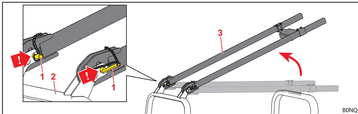
Fig. 40 Omhoog geklapte en in onderste boringen geborgde traversen
