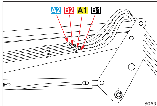
Fig. 18 Hydraulische leidingen
