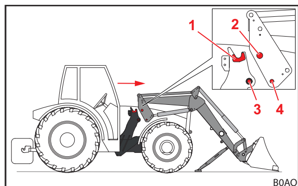
Fig. 53 Tractor in de arm rijden
