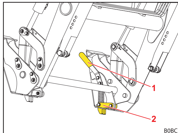
Fig. 78 Mechanische werktuigvergrendeling Skid-Steer (vergrendelde toestand zonder werktuig)
