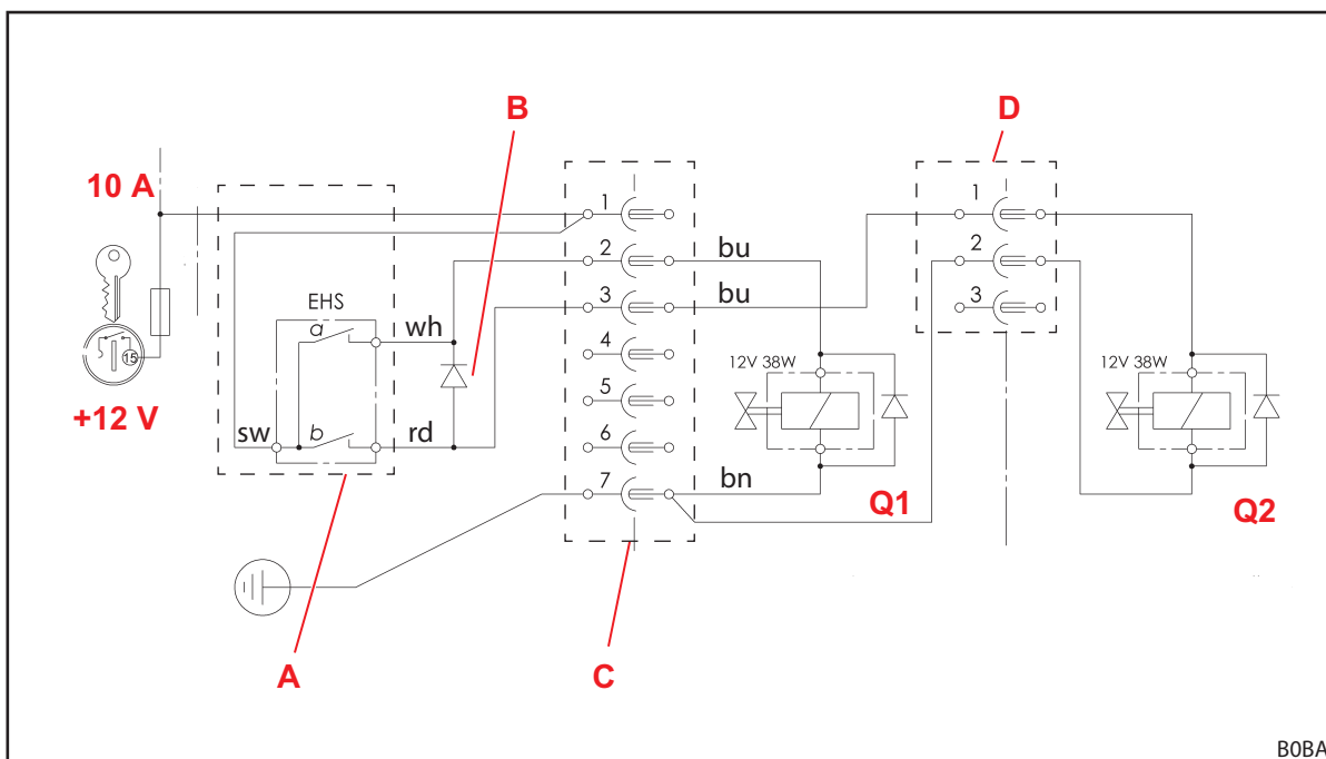
Fig. 123 Elektrisch schakelschema
