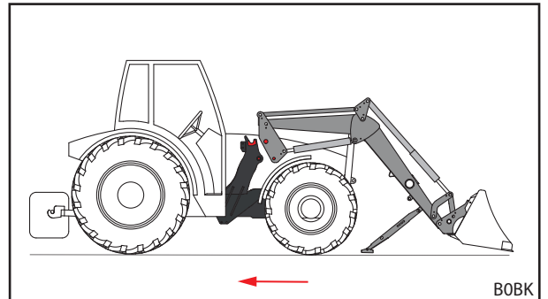
Fig. 121 Tractor achteruit verwijderen
