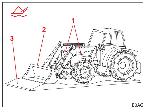
Fig. 32 Frontlader op zweefstand
