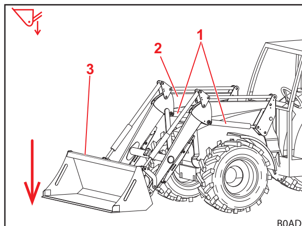
Fig. 29 Neerlaten-functie
