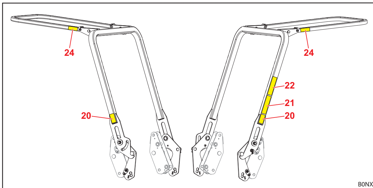
Fig. 7 OPG voor tractoren met vooraan gemonteerde kantelbeveiliging met 2 poten (afbeelding als voorbeeld)
