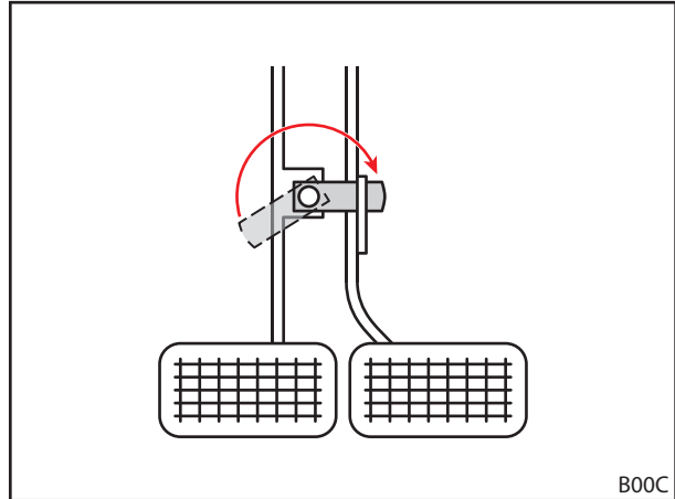
Fig. 48 Rempedalen verbinden
