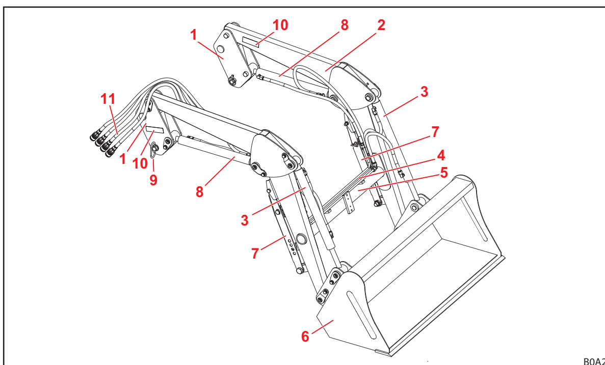
Fig. 9 Frontlader L (voorbeeld)
