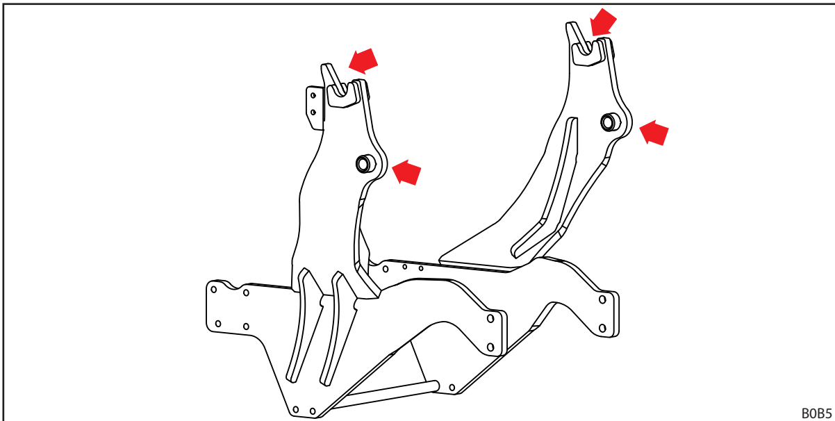
Fig. 113 Smeerpunten frontlader-opneempunten
