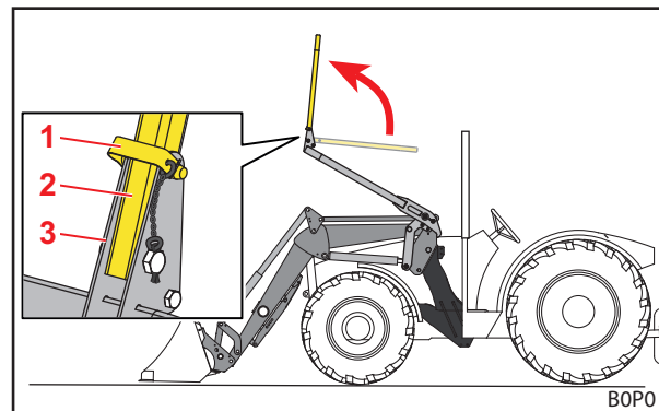
Fig. 44 Omhoog geklapte bovenste beugel
