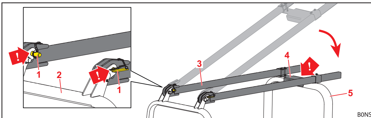
Fig. 42 Omlaag geklapte en in de bovenste boringen geborgde traversen
