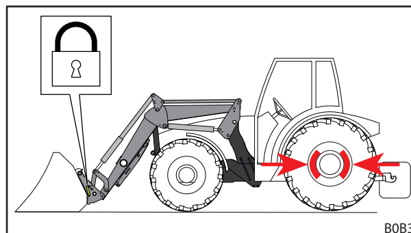
Fig. 92 Werktuigvergrendeling sluiten
