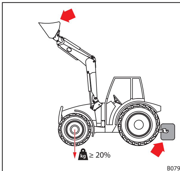
Fig. 50 Belasting bij rijden op de weg
