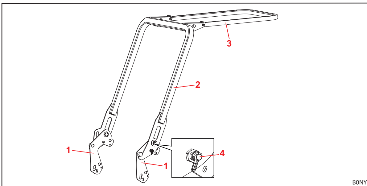
Fig. 13 Operator Protective Guard, OPG, voor tractoren met vooraan gemonteerde kantelbeveiliging met 2 poten (afbeelding als voorbeeld)
