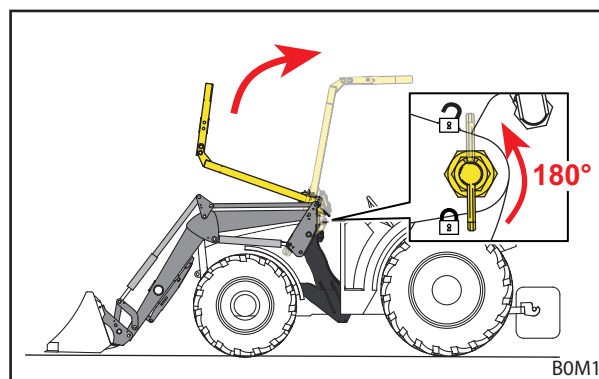
Fig. 38 OPG omhoog klappen
