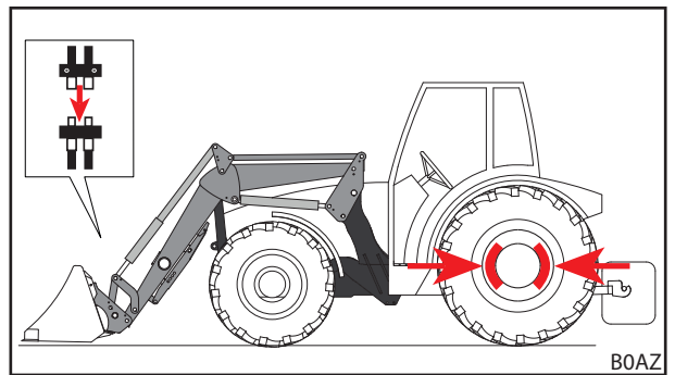
Fig. 98 Stuurkring aankoppelen
