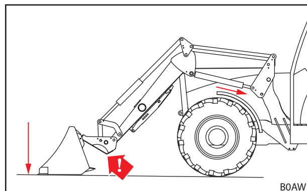
Fig. 79 Werktuig op de bodem drukken
