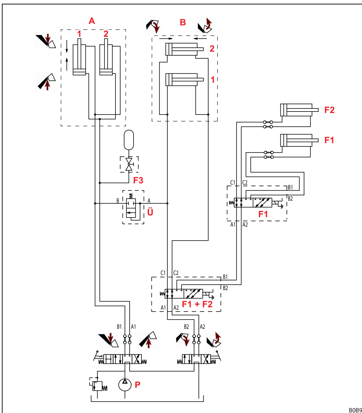
Fig. 122 Hydraulisch schema FC
