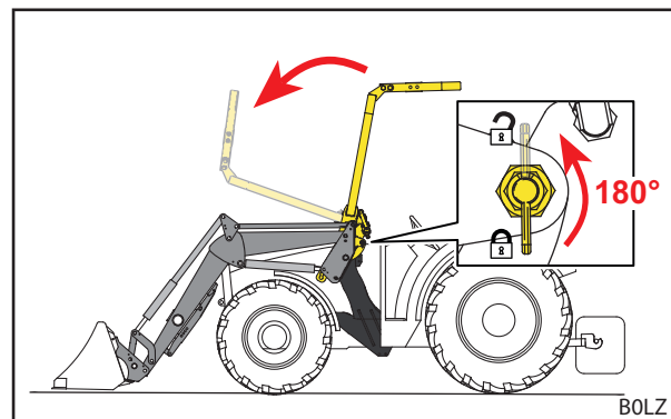
Fig. 36 OPG omlaag klappen
