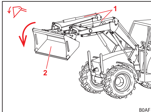
Fig. 31 Storten-functie
