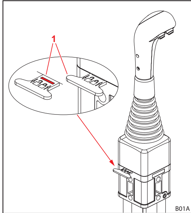
Fig. 61 Vergrendeling van de bedieningshendel
