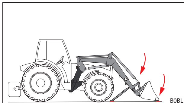
Fig. 119 Frontlader neerlaten en werktuig storten
