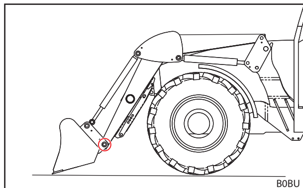
Fig. 95 Werktuig in de onderste pengaten verbinden
