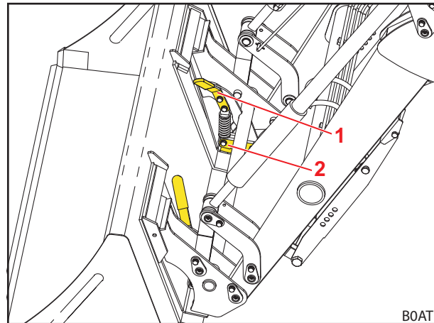
Fig. 77 Mechanische werktuigvergrendeling Skid-Steer (vergrendelde toestand met werktuig)
