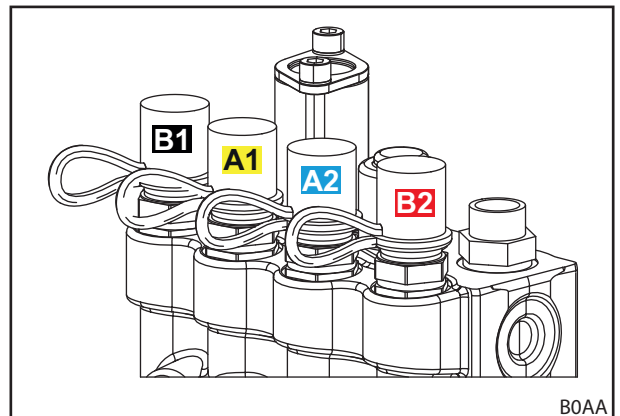
Fig. 20 Stekkers van de steekkoppelingen direct op de hydraulische klep
