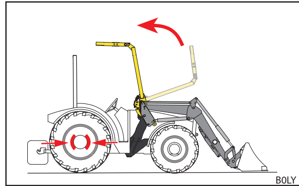
Fig. 55 OPG omhoog klappen
