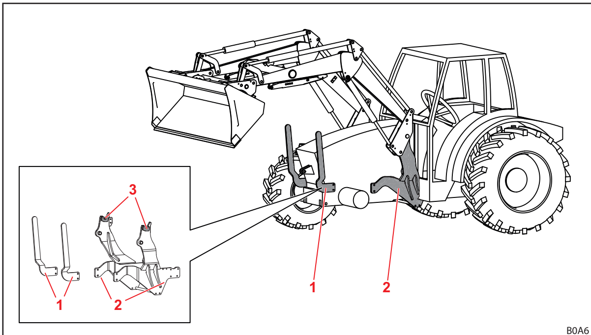
Fig. 15 Montageset voor tractor
