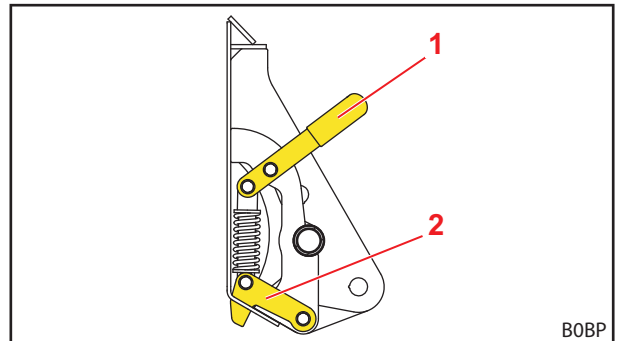
Fig. 75 Mechanische werktuigvergrendeling Skid-Steer (half gesloten toestand)
