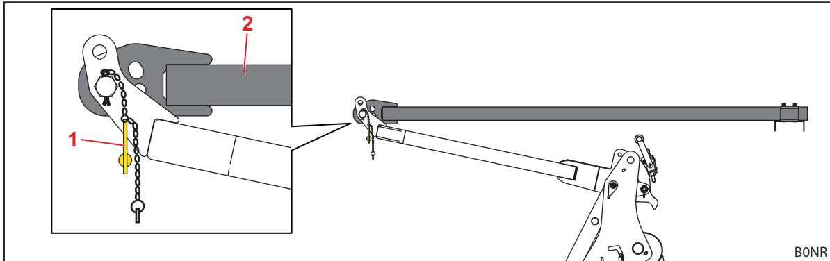
Fig. 41 Volledig omlaag geklapte traversen
