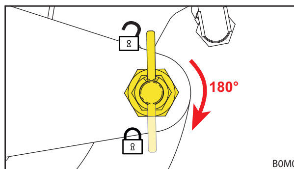
Fig. 39 Vergrendeling in de vergrendelingspositie zetten.
