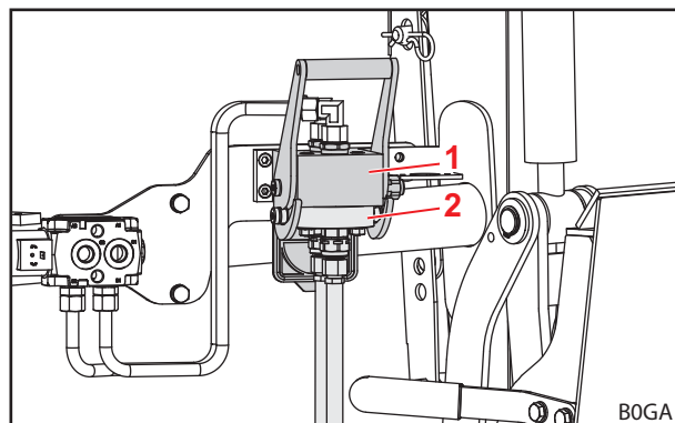
Fig. 73 Aangekoppeld werktuig-fix
