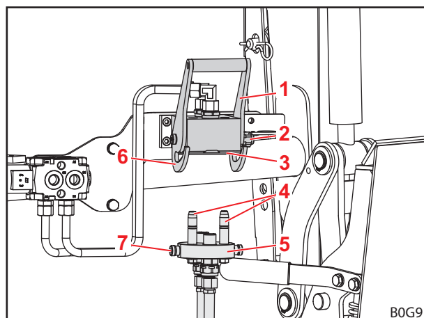
Fig. 72 Afgekoppelde werktuig-fix
