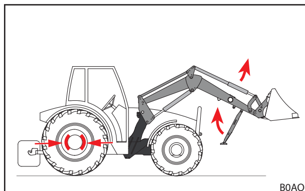
Fig. 57 Parkeersteunen inklappen
