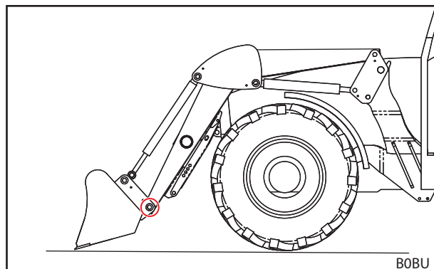
Fig. 105 Onderste pen uittrekken
