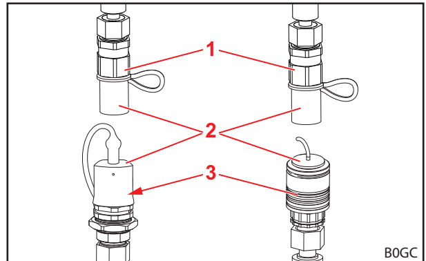
Fig. 69 Steekkoppelingen (voorbeeld)
