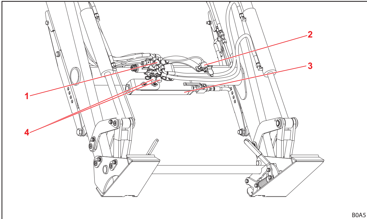
Fig. 14 Extra uitrusting voor frontladers L, H en P (voorbeeld)
