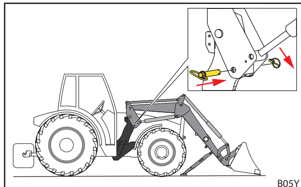
Fig. 56 Vergrendelingspen aanbrengen en met borgpen beveiligen
