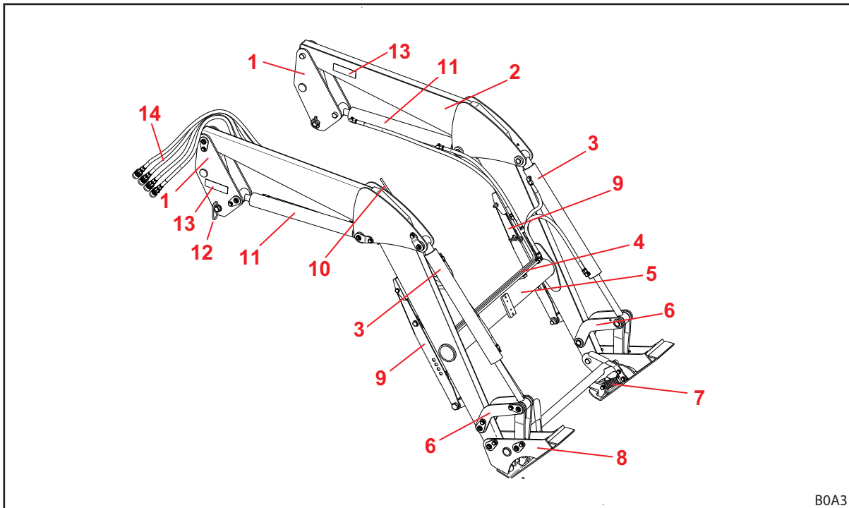
Fig. 10 Frontlader H (voorbeeld)
