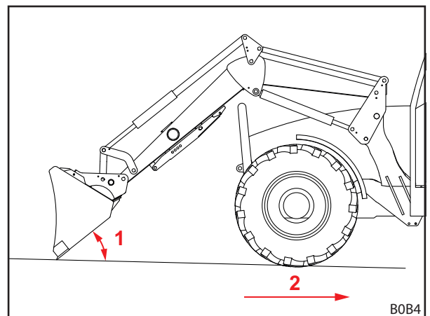
Fig. 107 Achteruit egaliseren
