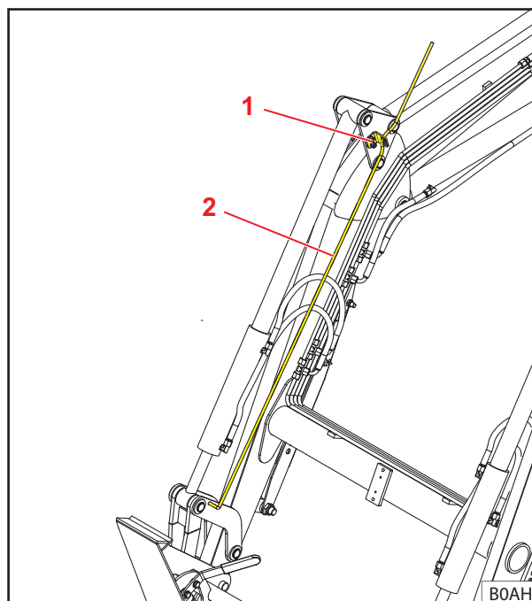
Fig. 33 Indicator voor werktuigpositie
