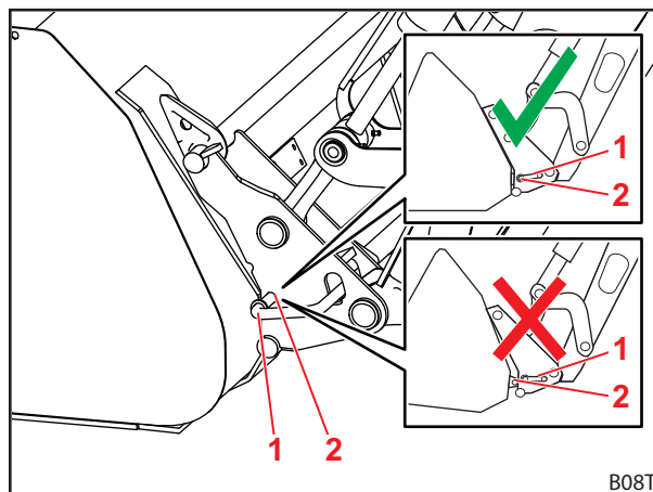
Fig. 81 Positie van de vergrendelingspennen controleren
