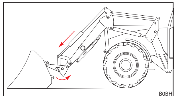
Fig. 101 Wisselframe loshaken
