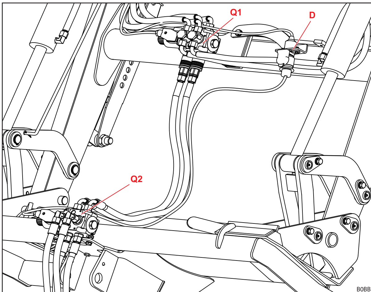
Fig. 124 Indeling van de hydraulische kleppen voor extra functies
