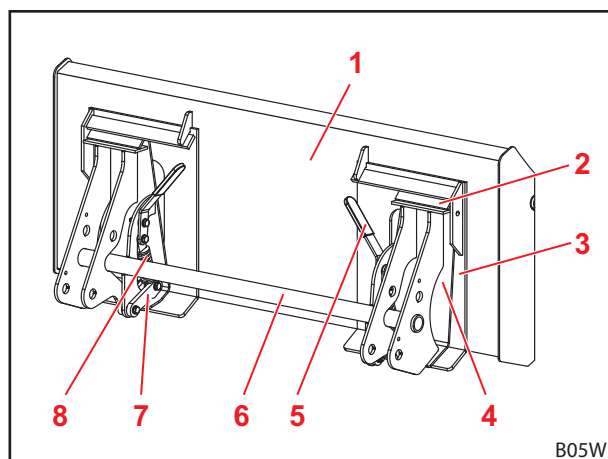
Fig. 26 Gesloten vergrendeling
