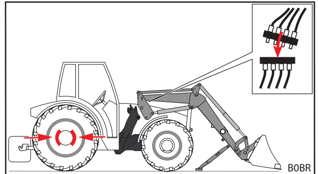
Fig. 120 Hydraulica afkoppelen
