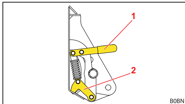
Fig. 74 Mechanische werktuigvergrendeling Skid-Steer (geopende toestand)
