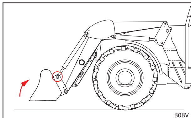
Fig. 96 Werktuig aan de bovenkant verbinden met de hydraulische cilinders
