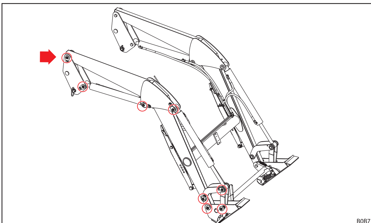
Fig. 115 Smeerpunten H
