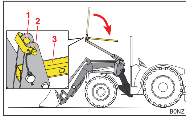
Fig. 43 Omlaag geklapte bovenste beugel
