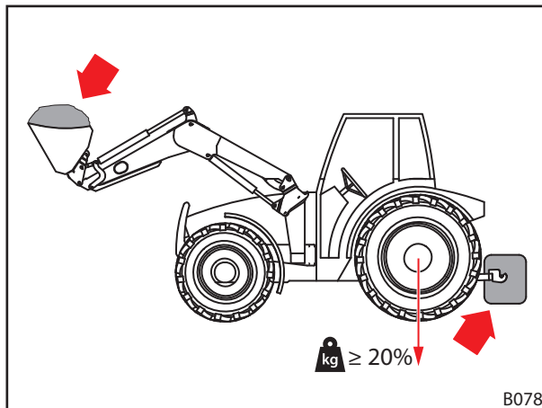
Fig. 49 Belasting bij frontladerwerkzaamheden
