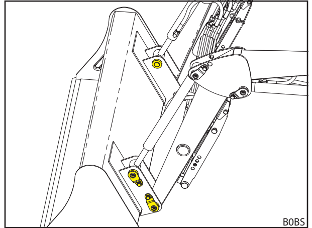
Fig. 97 Aangekoppeld werktuig
