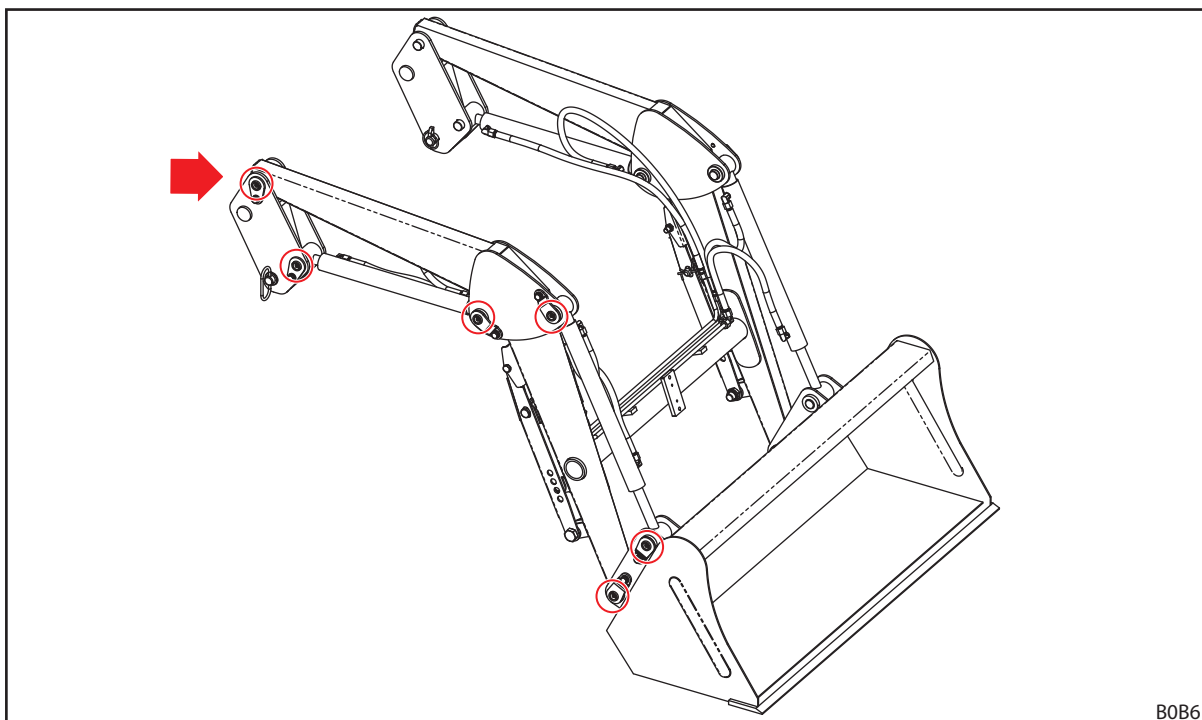
Fig. 114 Smeerpunten L
