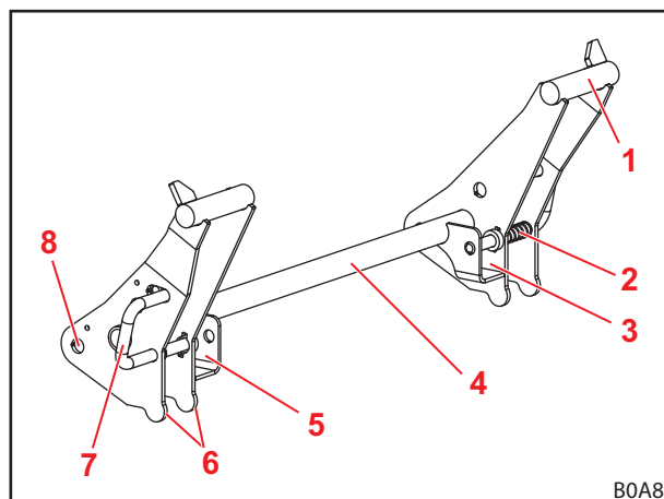
Fig. 80 Werktuigvergrendeling aan het Euro-wisselframe
