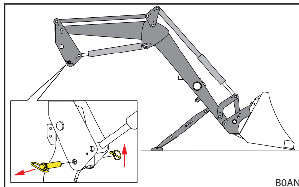
Fig. 52 Frontlader-vergrendeling openen
