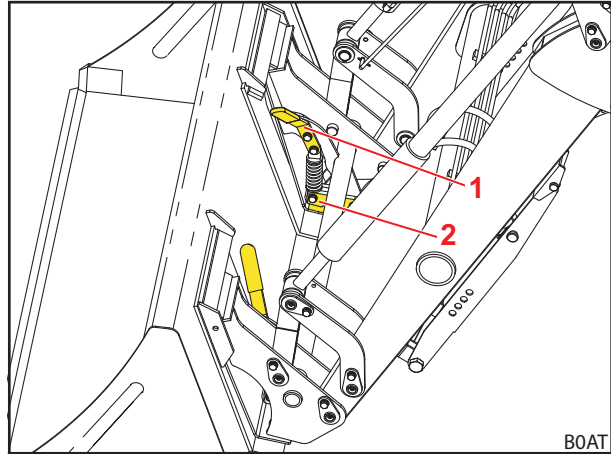
Fig. 83 Werktuigvergrendeling openen
