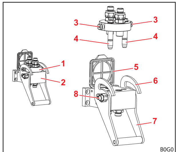
Fig. 24 Opbouw werktuig-Fix
