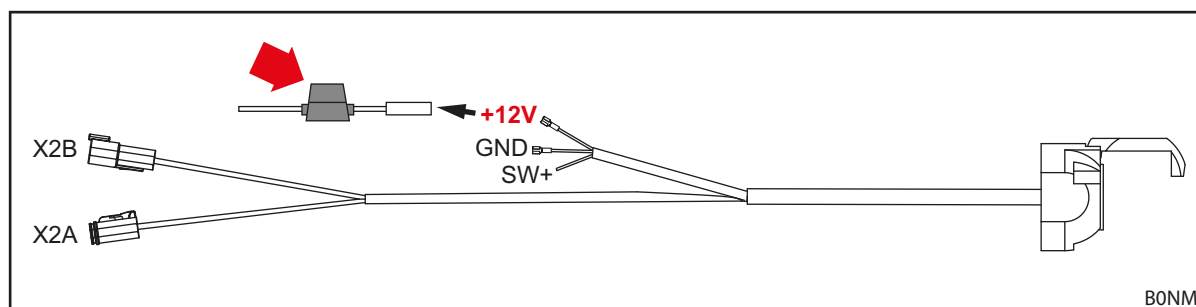
Σχ. 53 Πλεξούδα καλωδίων STOLL-ISOBUS
