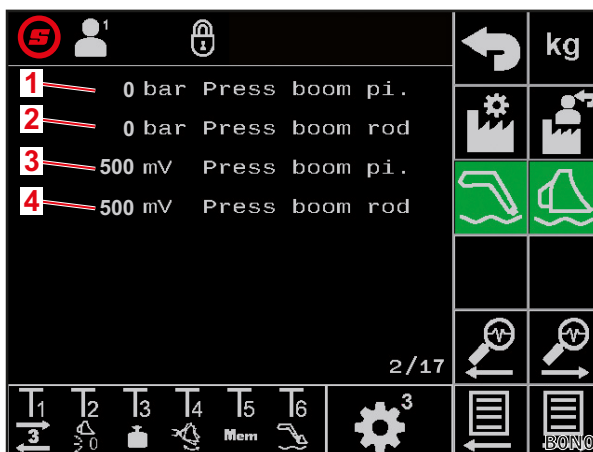
Σχ. 38 Αισθητήρες πίεσης του περιστροφικού βραχίονα
