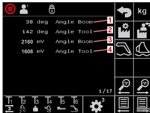
Σχ. 37 Αισθητήρες γωνίας περιστροφικού βραχίονα και εργαλείου
