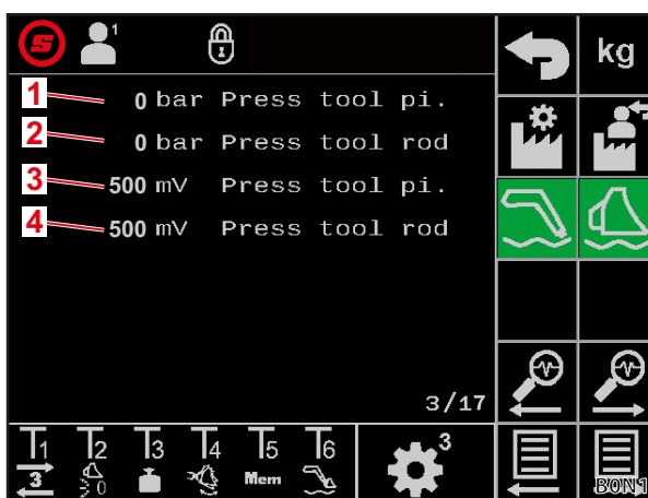
Σχ. 39 Αισθητήρες πίεσης του εργαλείου
