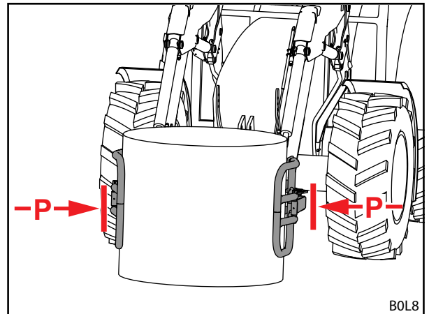
Σχ. 29 Ρύθμιση πίεσης
