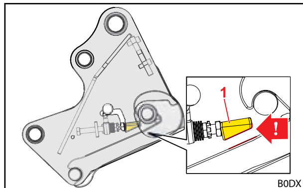
Σχ. 58 Σωστή θέση τοποθέτησης της σφήνας σύσφιξης
