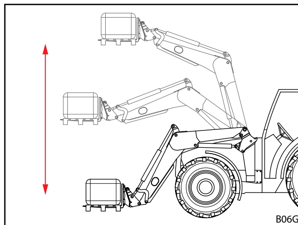
Σχ. 42 Μηχανικός παράλληλος οδηγός
