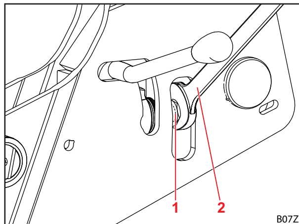
Σχ. 64 Εφαρμογή εργαλείου
