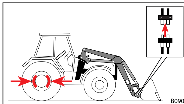
Σχ. 102 Λύσιμο υδραυλικών αγωγών
