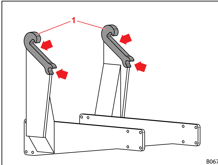
Σχ. 112 Σημεία λίπανσης υποδοχών εμπρόσθιου φορτωτή
