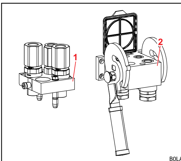
Σχ. 20 Διάταξη Hydro-Fix
