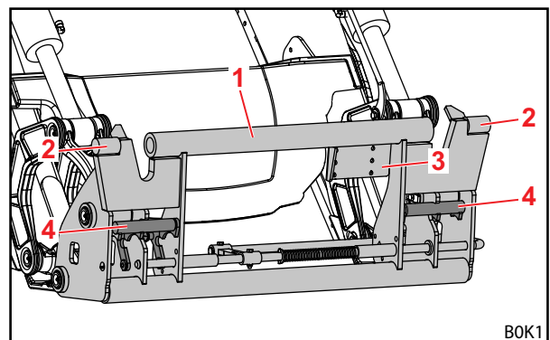
Σχ. 12 Σύνθετο πλαίσιο εναλλαγής Euro-SMS (προετοιμασμένο για εργαλείο SMS)
