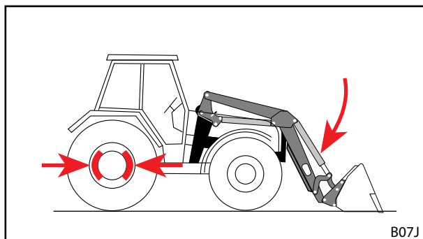
Σχ. 120 Τραβήξτε το χειρόφρενο και κατεβάστε τον εμπρόσθιο φορτωτή
