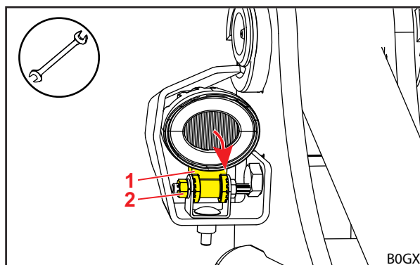
Σχ. 48 Κάθετη ρύθμιση προβολέα
