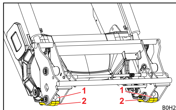
Σχ. 16 Πέδιλα φθοράς
