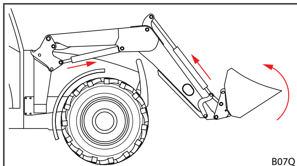
Σχ. 97 Ενεργοποίηση μηχανισμού ασφάλισης εργαλείου
