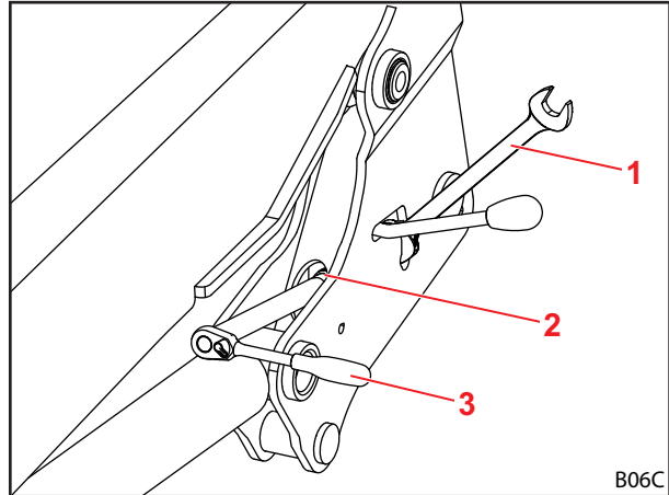
Σχ. 60 Εφαρμογή εργαλείου
