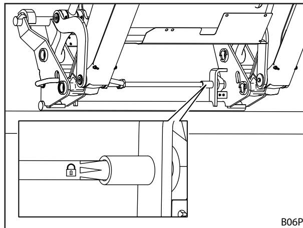
Σχ. 78 Έλεγχος μηχανισμού ασφάλισης εργαλείων με τη βοήθεια του αυτοκόλλητου
