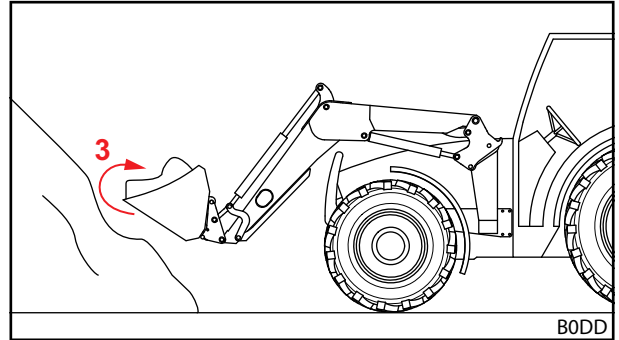
Σχ. 108 Γείρετε προς τα πίσω το εργαλείο και παραλάβετε το φορτίο
