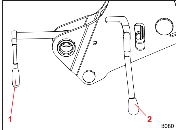
Σχ. 65 Περάστε το σωληνωτό κλειδί προς τη βίδα
