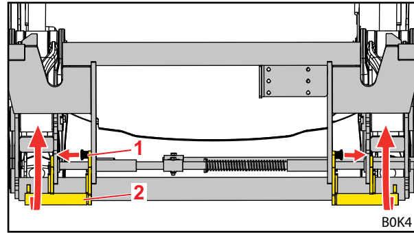
Σχ. 89 Ανέβασμα διατάξεων
