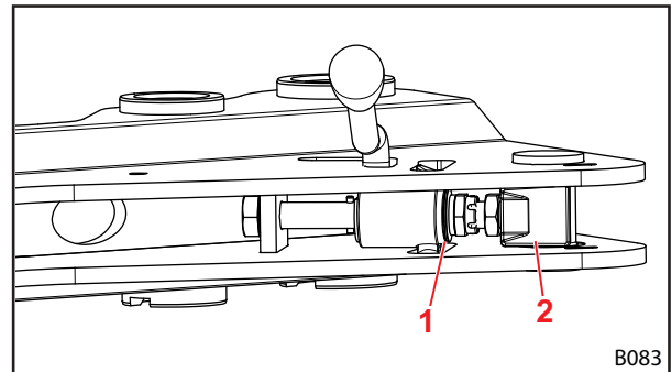
Σχ. 66 Όψη του κλειδώματος του εμπρόσθιου φορτωτή από κάτω
