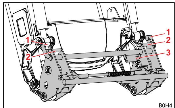
Σχ. 13 Σύνθετο πλαίσιο εναλλαγής Euro-AIö 3
