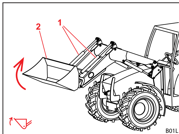
Σχ. 26 Λειτουργία συλλογής
