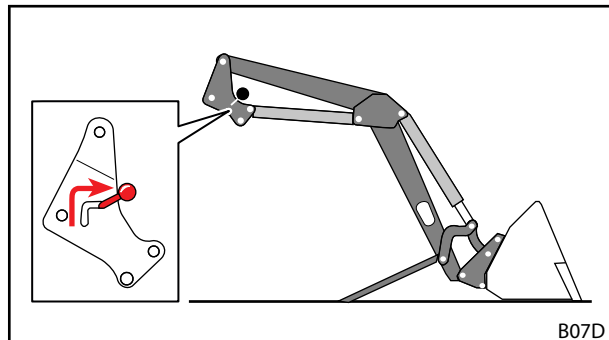
Σχ. 53 Άνοιγμα κλειδώματος εμπρόσθιου φορτωτή
