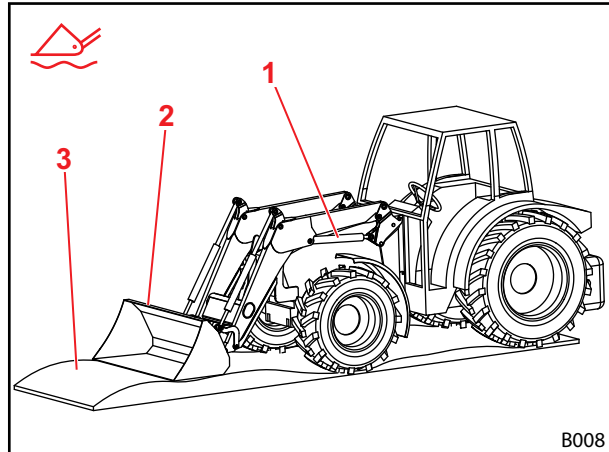
Σχ. 40 Εμπρόσθιος φορτωτής σε θέση πλεύσης
