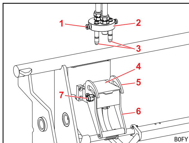
Σχ. 75 Αποσυνδεδεμένη στερέωση εργαλείων
