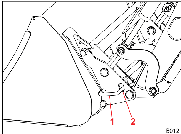
Σχ. 77 Μηχανικός μηχανισμός ασφάλισης εργαλείων
