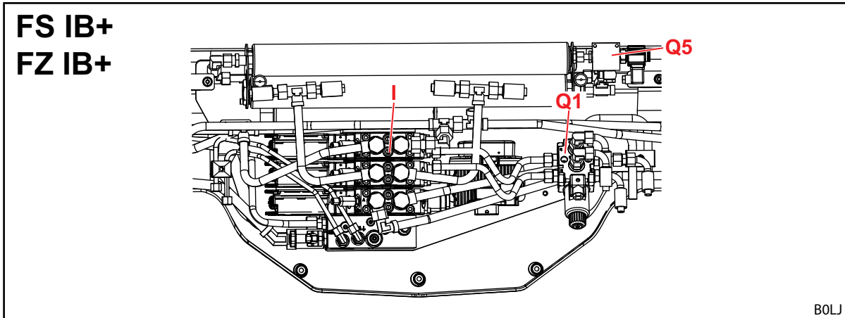
Σχ. 128 Διάταξη υδραυλικών βαλβίδων για πρόσθετες λειτουργίες
