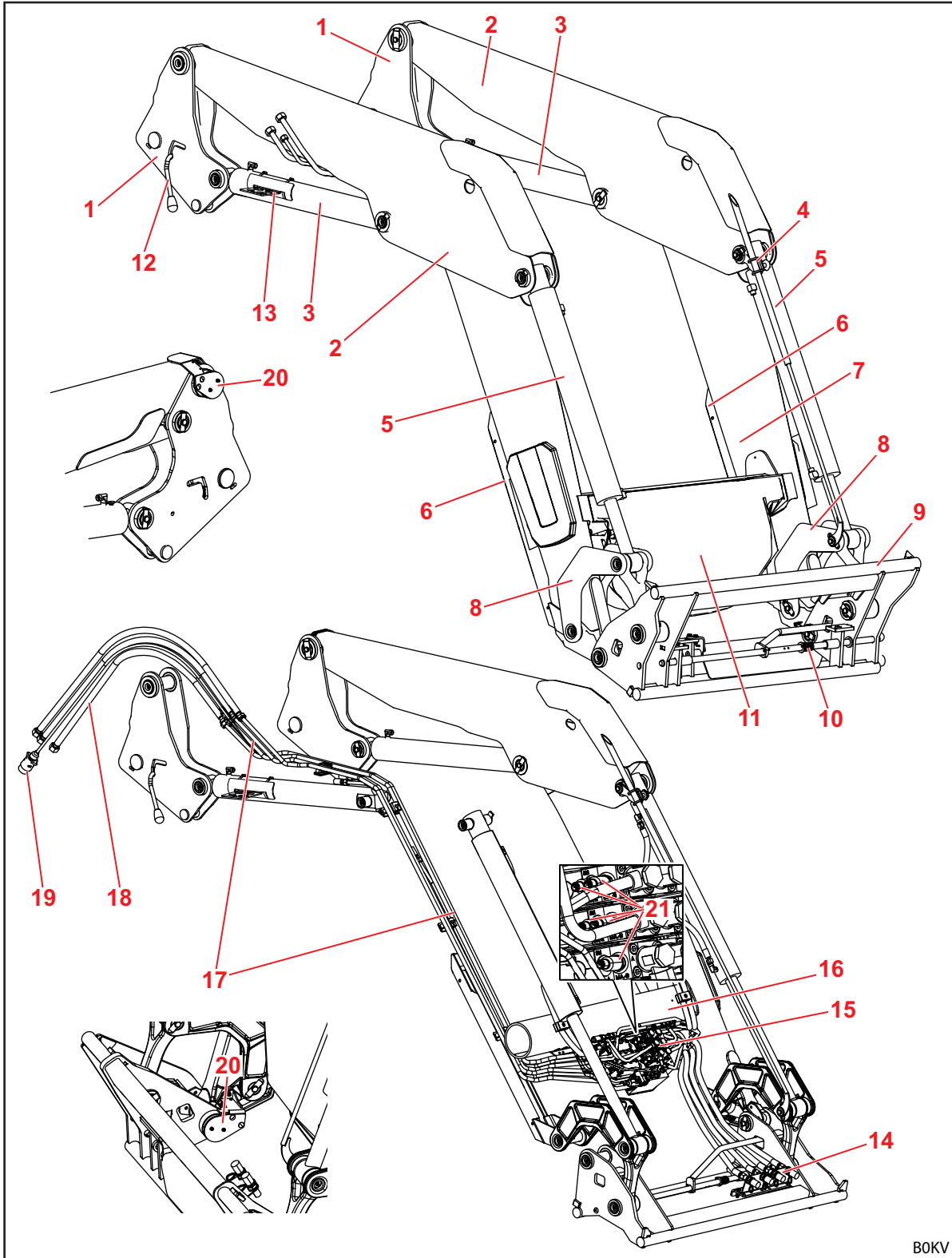
Σχ. 7 Εμπρόσθιος φορτωτής FS IB+
