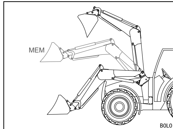
Σχ. 31 Επιστροφή στη θέση
