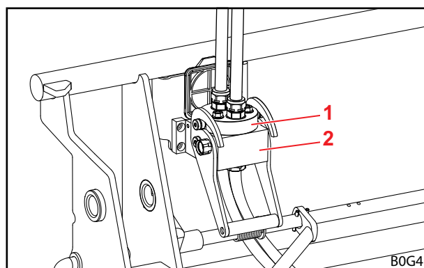
Σχ. 76 Συνδεδεμένη στερέωση εργαλείων
