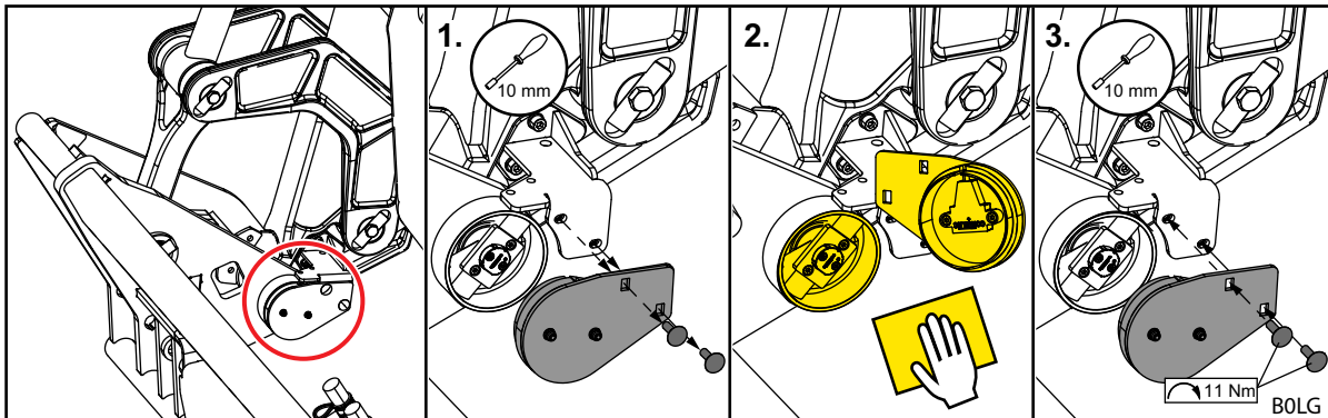
Σχ. 111 Καθαρισμός αισθητήρα γωνίας περιστροφής
