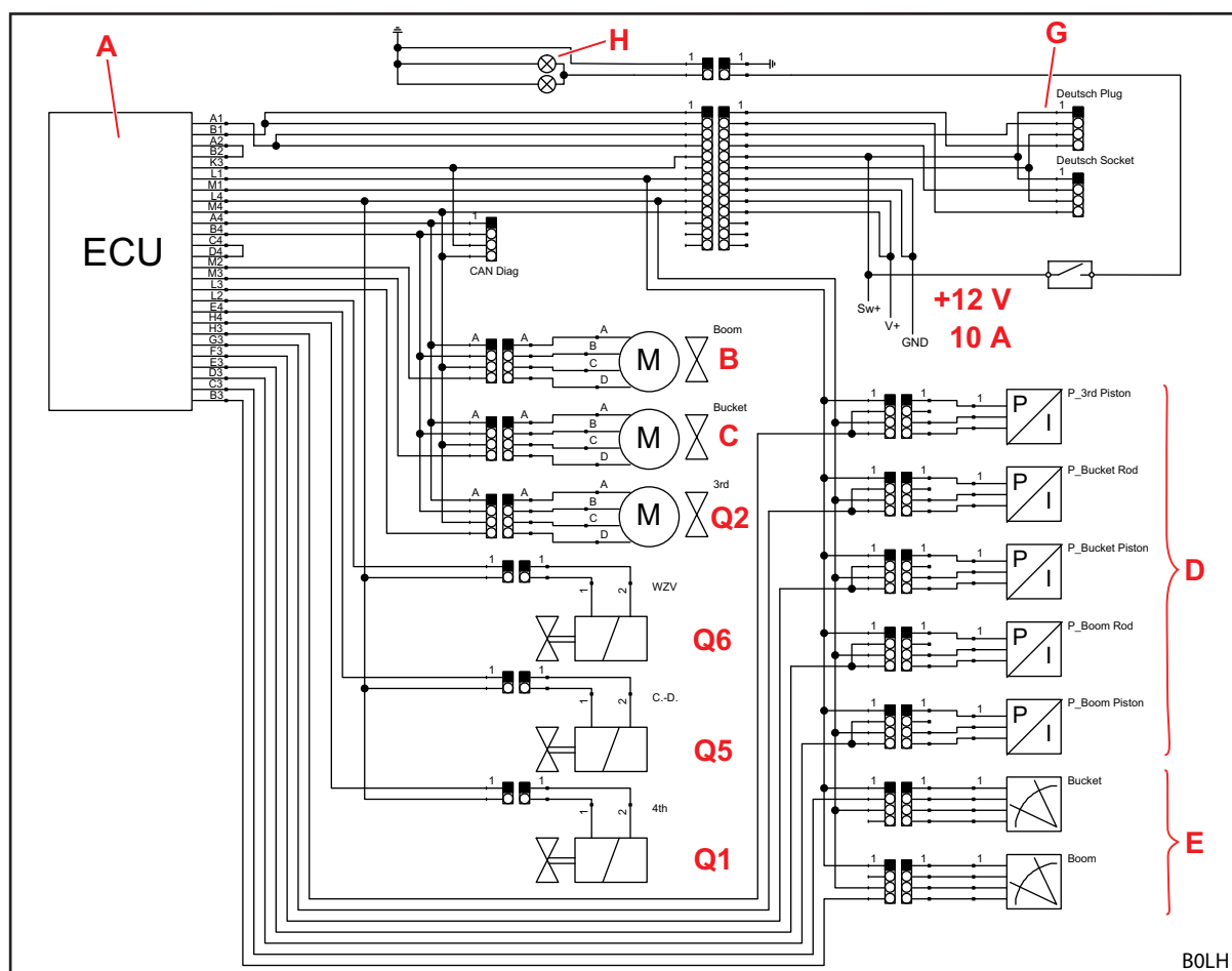
Σχ. 127 Ηλεκτρικό διάγραμμα συνδεσμολογίας
