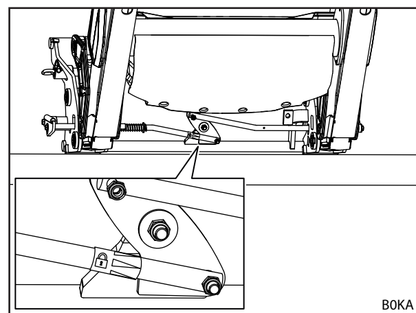
Σχ. 79 Έλεγχος μηχανισμού ασφάλισης εργαλείων με τη βοήθεια του αυτοκόλλητου (σύνθετο πλαίσιο εναλλαγής Euro-MX)
