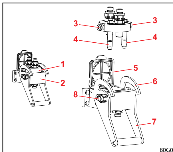
Σχ. 22 Διάταξη στερέωσης εργαλείων
