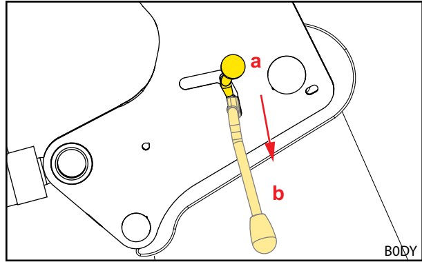
Σχ. 61 Διαδικασία σύσφιξης του μοχλού ασφάλισης
