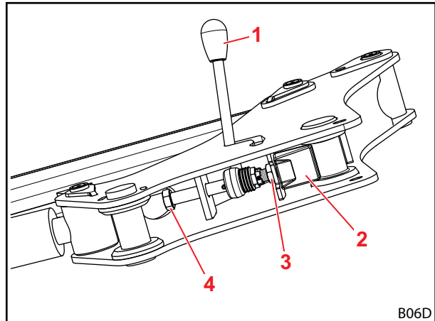
Σχ. 62 Όψη του κλειδώματος του εμπρόσθιου φορτωτή από κάτω
