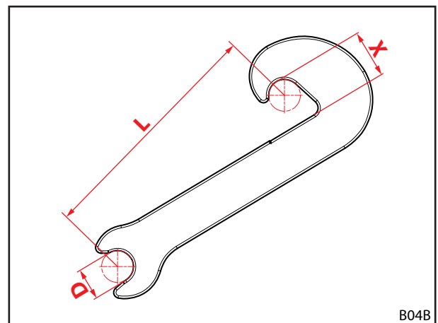
Σχ. 115 Διαστάσεις φθοράς του άγκιστρου
