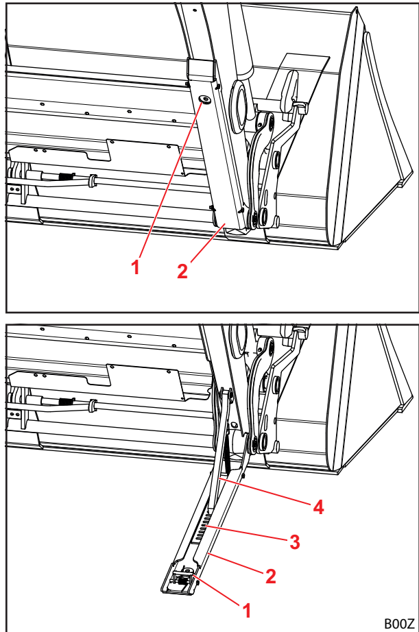
Σχ. 71 Στήριγμα στάθμευσης
