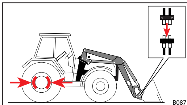
Σχ. 98 Σύνδεση υδραυλικών αγωγών εργαλείου με τους συνδέσμους του εμπρόσθιου φορτωτή
