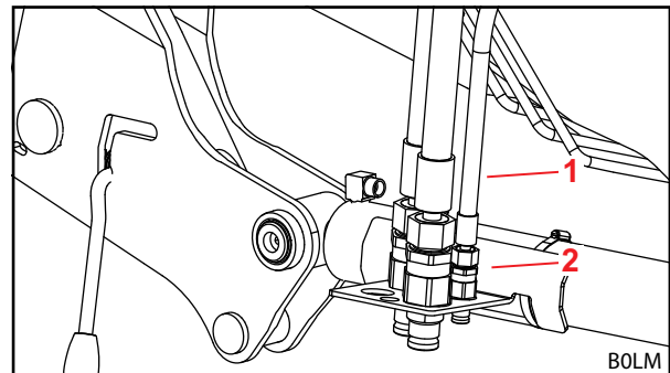
Σχ. 125 Αναρτάτε τους υδραυλικούς αγωγούς στη βάση συνδέσμου (απεικόνιση με κουμπωτούς συνδέσμους)
