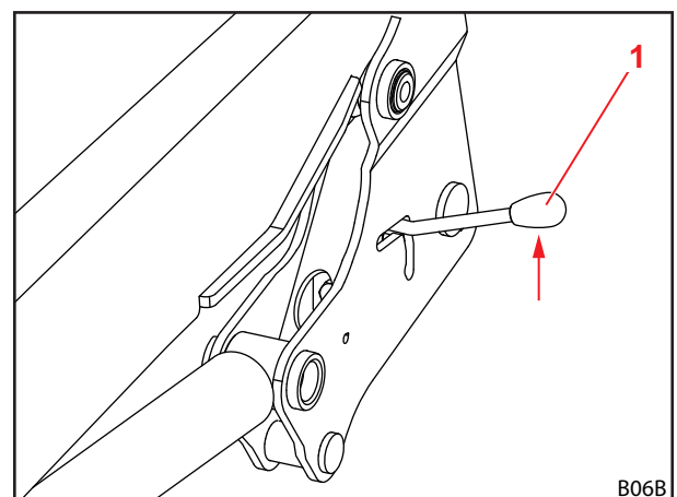
Σχ. 116 Έλεγχος κλειδώματος εμπρόσθιου φορτωτή
