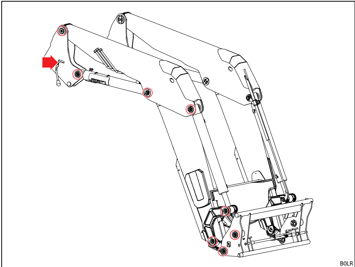
Σχ. 113 Σημεία λίπανσης FS IB+
