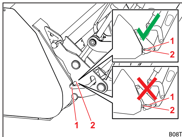
Σχ. 80 Έλεγχος θέσης πείρων ασφάλισης
