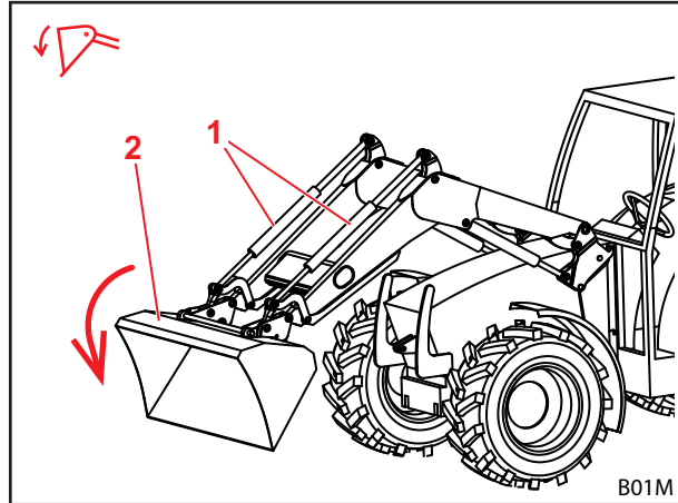
Σχ. 27 Λειτουργία απόθεσης
