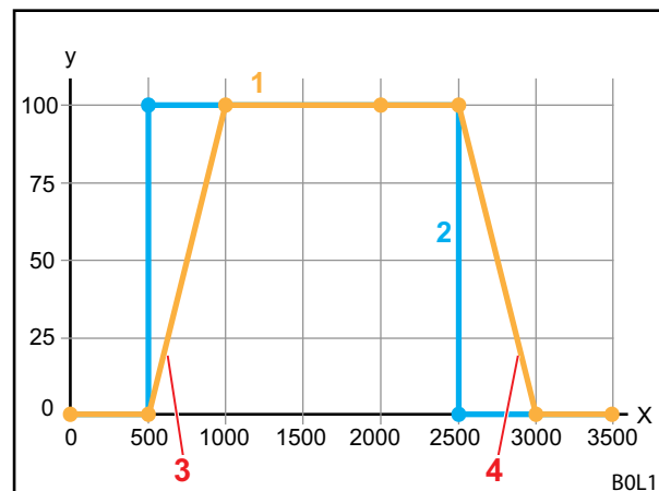
Σχ. 32 Ρυθμιζόμενη συμπεριφορά απόκρισης
