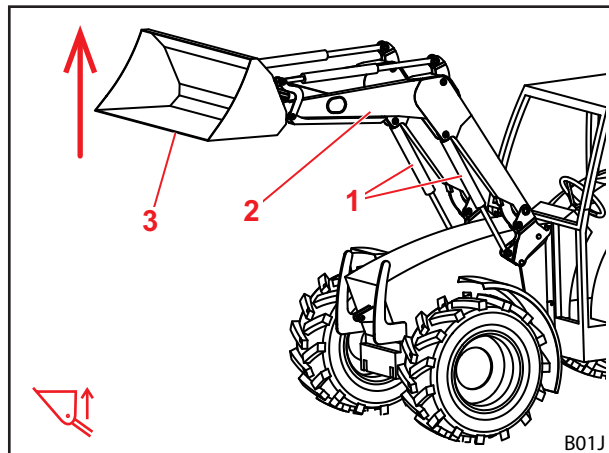
Σχ. 24 Λειτουργία ανύψωσης
