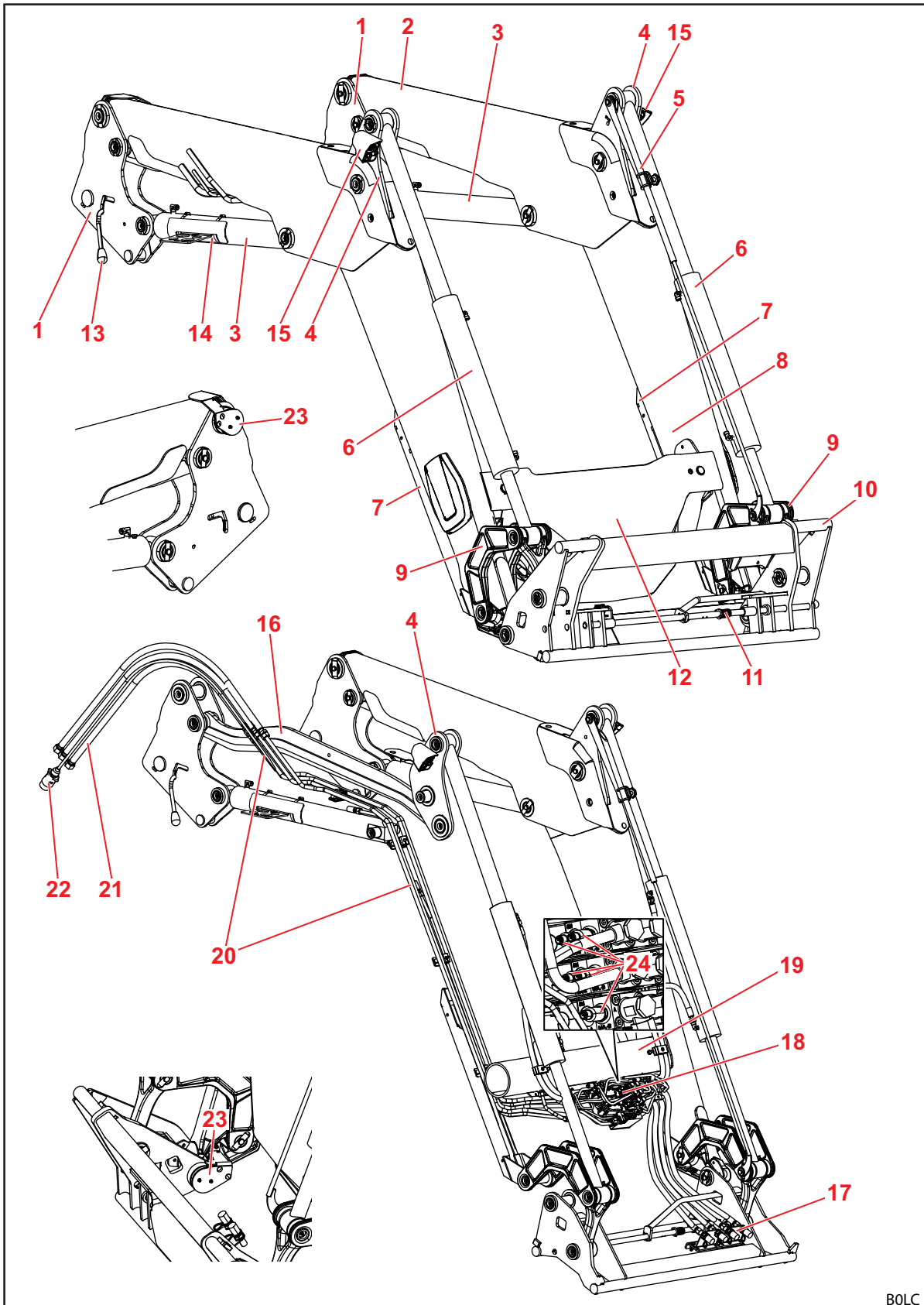
Σχ. 8 Εμπρόσθιος φορτωτής FZ IB+
