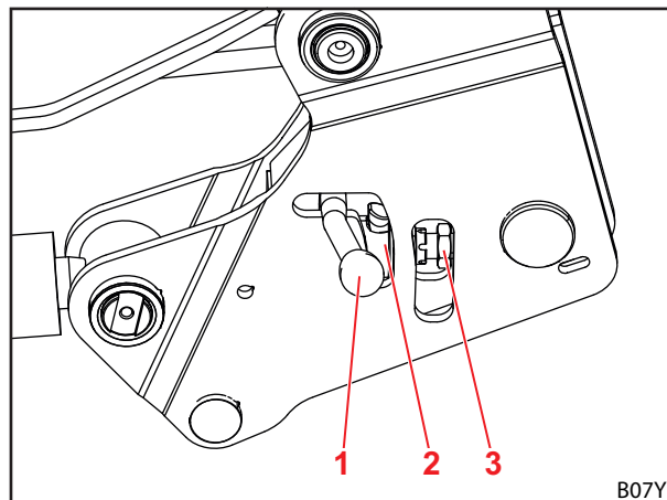
Σχ. 63 Άνοιγμα κλειδώματος εμπρόσθιου φορτωτή
