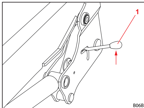
Σχ. 59 Ανοίγμα κλειδώματος εμπρόσθιου φορτωτή
