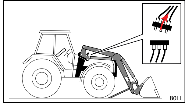
Σχ. 123 Αποσύνδεση υδραυλικού συστήματος
