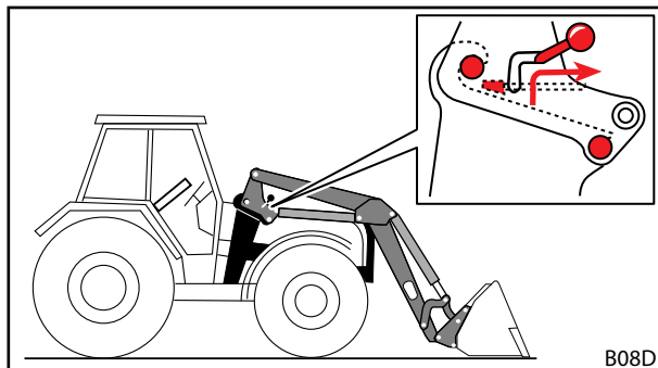
Σχ. 121 Λύσιμο κλειδώματος εμπρόσθιου φορτωτή
