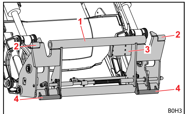
Σχ. 11 Σύνθετο πλαίσιο εναλλαγής Euro-SMS (προετοιμασμένο για εργαλείο Euro)
