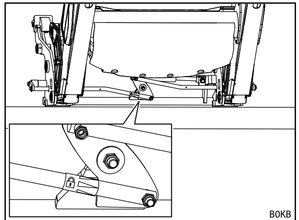
Σχ. 84 Έλεγχος μηχανισμού ασφάλισης εργαλείων με τη βοήθεια του αυτοκόλλητου
