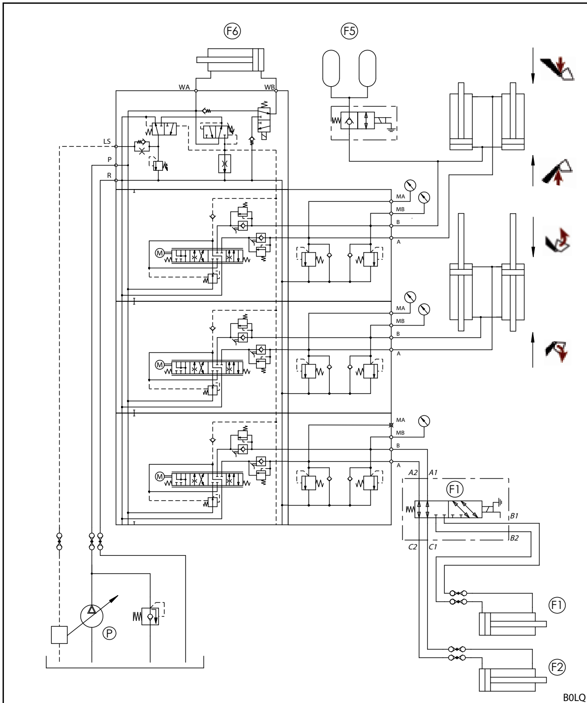
Σχ. 126 Υδραυλικό σχέδιο FS IB+ και FZ IB+
