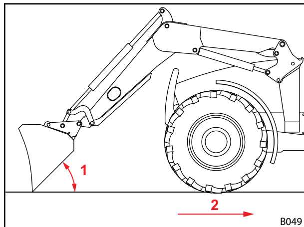
Σχ. 105 Ισοπέδωση με όπισθεν
