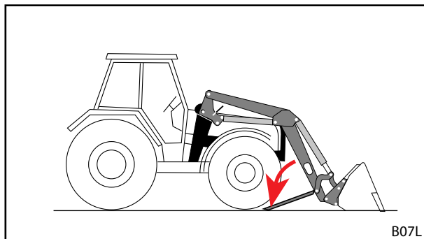
Σχ. 122 Άνοιγμα στηριγμάτων στάθμευσης
