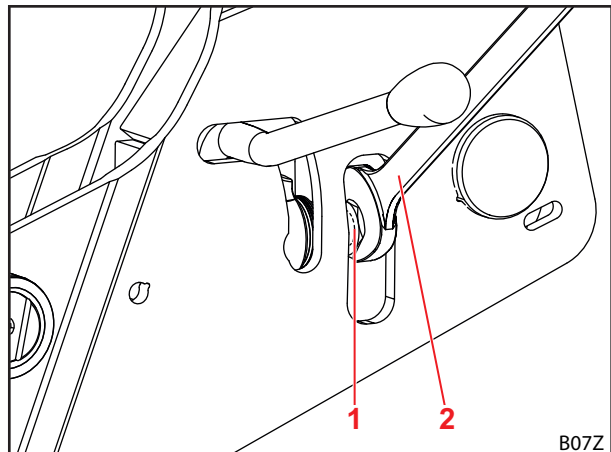
Σχ. 67 Σφίξτε το κόντρα παξιμάδι
