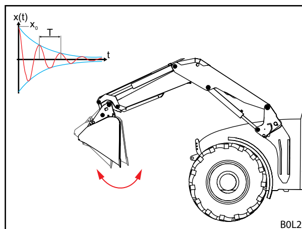
Σχ. 35 Ανακίνηση κουβά
