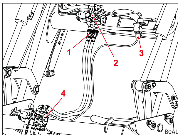
Σχ. 46 Πρόσθετο 4ο κύκλωμα ελέγχου
