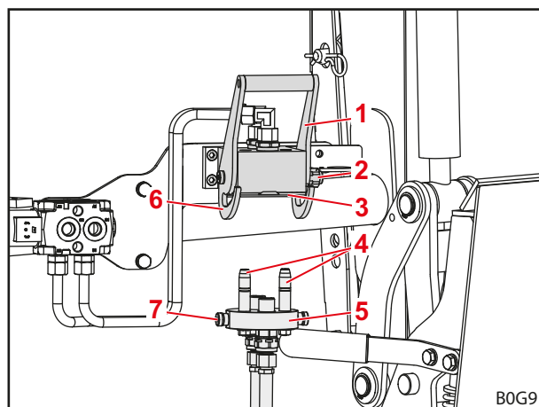
Σχ. 72 Αποσυνδεδεμένη στερέωση εργαλείων
