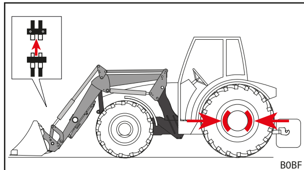
Σχ. 100 Λύσιμο υδραυλικών αγωγών
