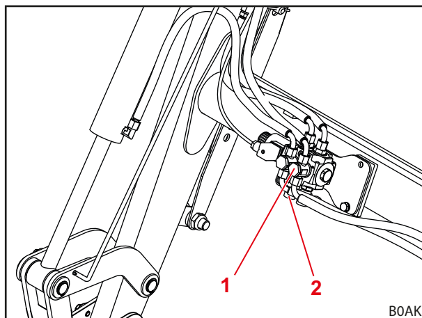
Σχ. 45 Πρόσθετο 3ο κύκλωμα ελέγχου
