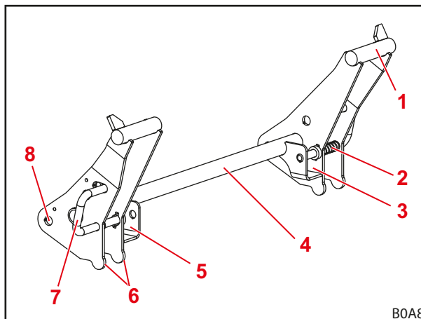
Σχ. 17 Πλαίσιο εναλλαγής Euro
