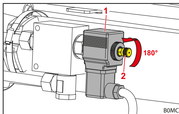
Σχ. 35 Ανοιγμα βαλβίδας
