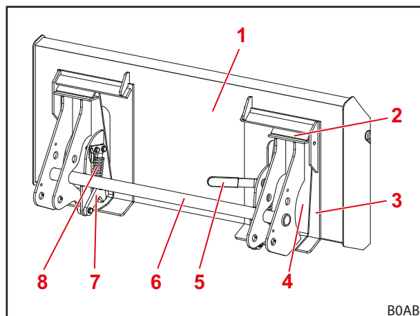
Σχ. 25 Ανοιχτός μηχανισμός ασφάλισης
