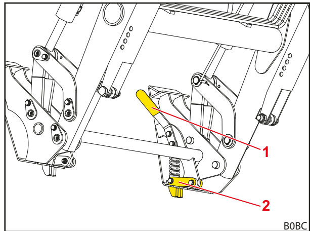
Σχ. 78 Μηχανικός μηχανισμός ασφάλισης εργαλείου Skid-Steer (κλειδωμένη κατάσταση χωρίς εργαλείο)
