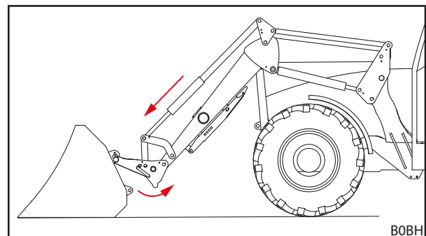
Σχ. 101 Απαγκίστρωση πλαισίου εναλλαγής
