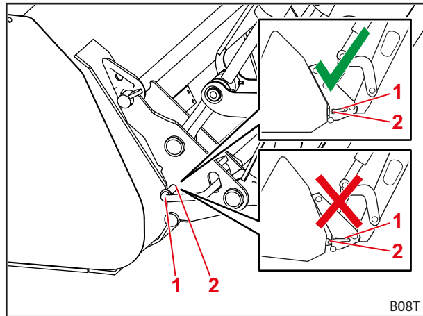
Σχ. 81 Έλεγχος θέσης πείρων ασφάλισης
