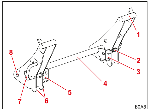
Σχ. 80 Χειρισμός μηχανισμού ασφάλισης εργαλείου στο πλαίσιο εναλλαγής Euro
