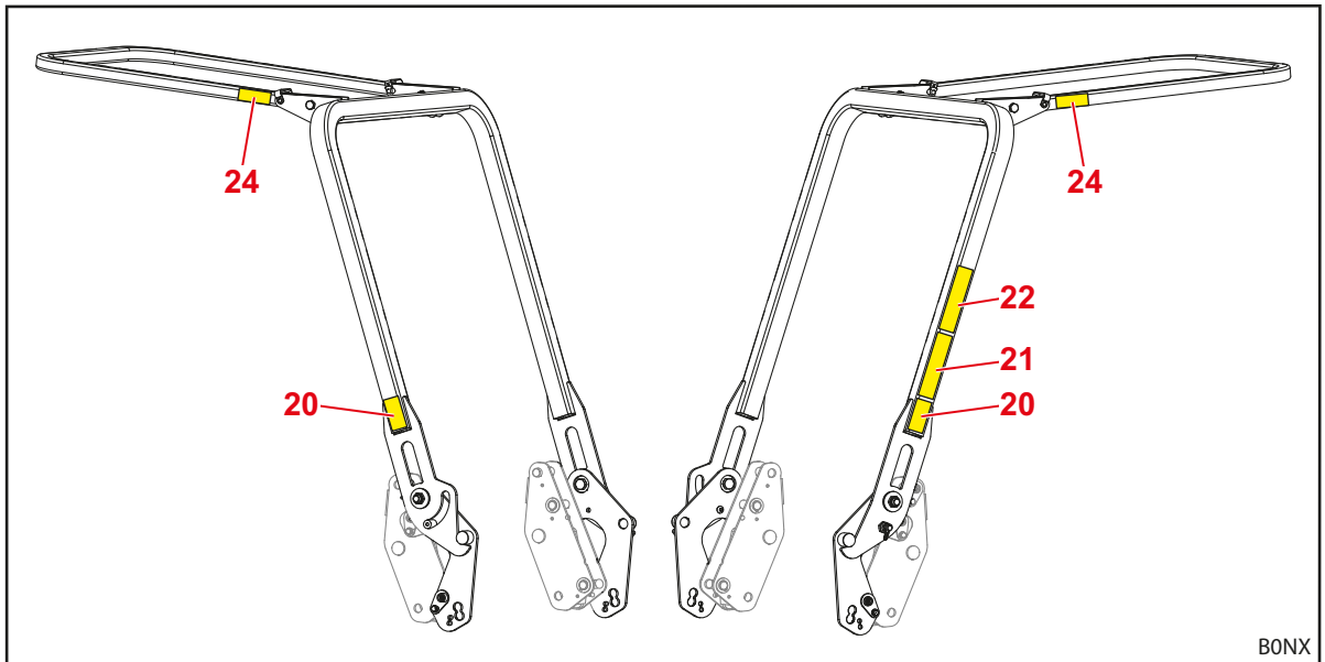
Σχ. 7 OPG για τρακτέρ με μπροστά τοποθετημένη διάταξη προστασίας από ανατροπή 2 κολώνων (ενδεικτική εικόνα)
