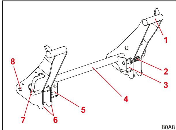
Σχ. 27 Πλαίσιο εναλλαγής Euro
