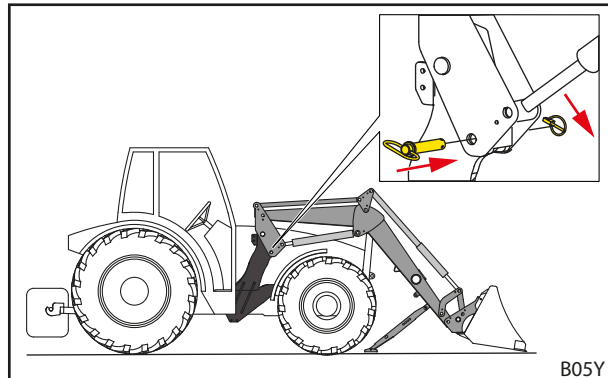
Σχ. 56 Τοποθετήστε τους πείρους κλειδώματος και ασφαλίστε τους με περόνη
