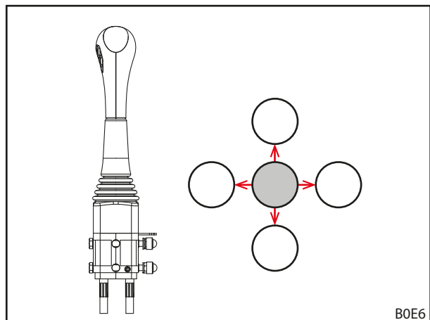
Σχ. 62 Μετακίνηση μοχλού χειρισμού σε όλες τις θέσεις τερματισμού
