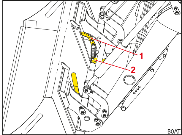
Σχ. 77 Μηχανικός μηχανισμός ασφάλισης εργαλείου Skid-Steer (κλειδωμένη κατάσταση με εργαλείο)
