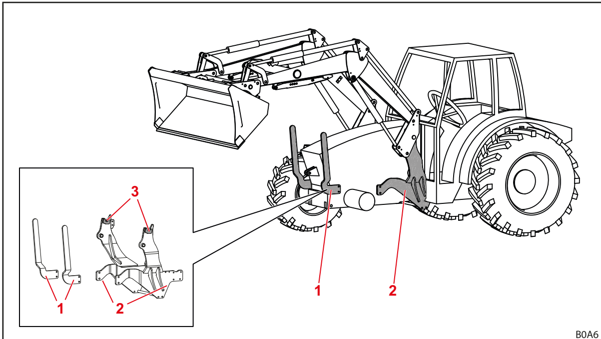
Σχ. 15 Σετ προσάρτησης για τρακτέρ
