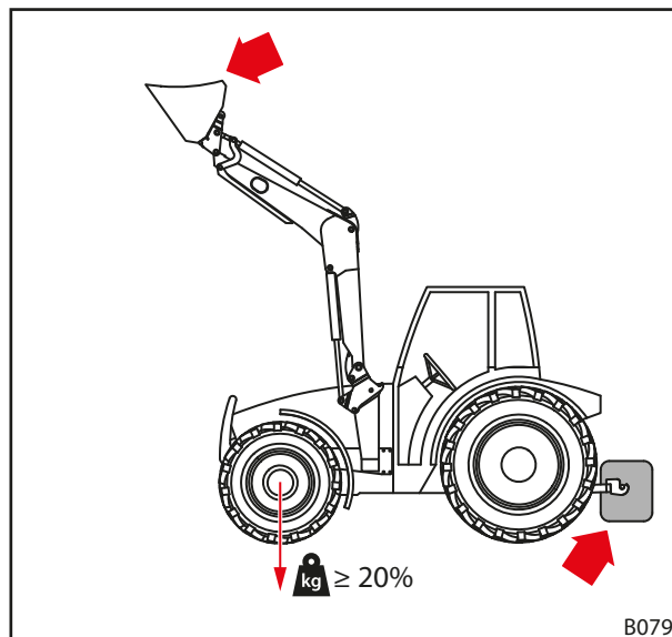
Σχ. 50 Φορτίο σε διαδρομές στον δρόμο
