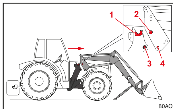
Σχ. 53 Εισαγωγή τρακτέρ στον περιστροφικό βραχίονα
