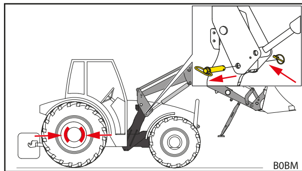
Σχ. 118 Τράβηγμα του χειρόφρενου και λύσιμο της ασφάλισης του εμπρόσθιου φορτωτή
