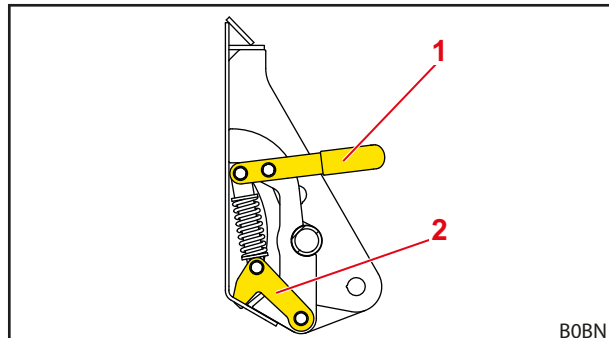
Σχ. 74 Μηχανικός μηχανισμός ασφάλισης εργαλείου Skid-Steer (ανοιχτή κατάσταση)
