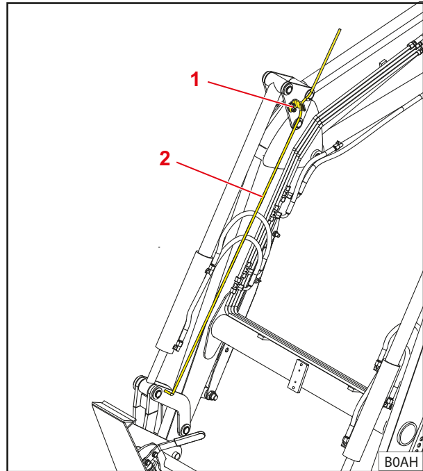
Σχ. 33 Οπτική ένδειξη για τη θέση του εργαλείου
