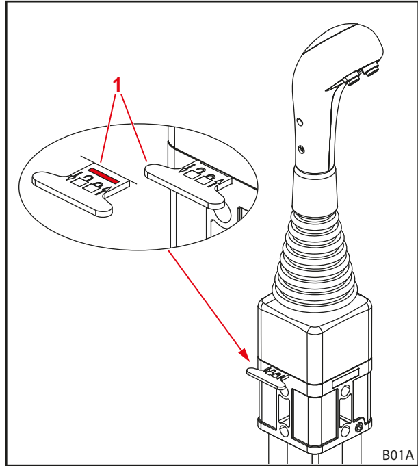
Σχ. 61 Ασφάλιση του μοχλού χειρισμού
