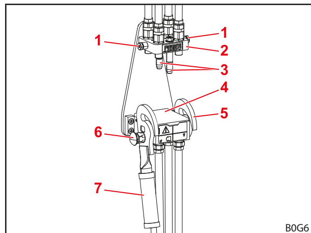
Σχ. 70 Αποσυνδεδεμένο Hydro-Fix
