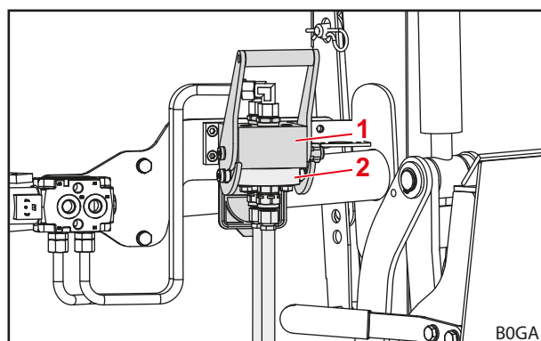
Σχ. 73 Συνδεδεμένη στερέωση εργαλείων
