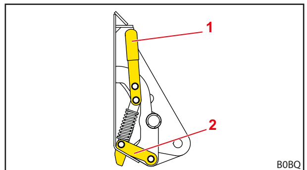
Σχ. 76 Μηχανικός μηχανισμός ασφάλισης εργαλείου Skid-Steer (κλειδωμένη κατάσταση)
