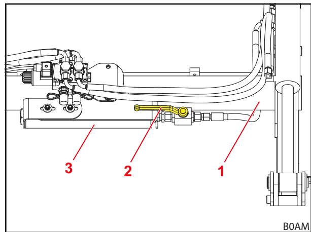
Σχ. 47 Μηχανικά ενεργοποιούμενο Comfort-Drive (θέση μοχλού Comfort-Drive ON)
