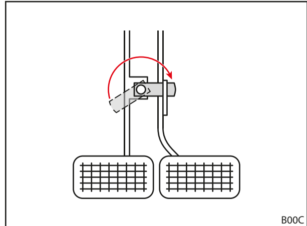
Σχ. 48 Σύνδεση πεντάλ φρένων
