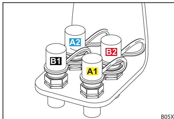
Σχ. 19 Βύσματα των κουμπωτών συνδέσμων στο προσαρτώμενο τμήμα
