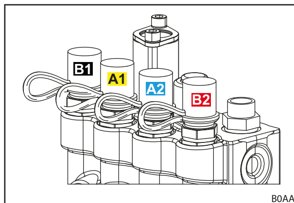
Σχ. 20 Βύσματα των κουμπωτών συνδέσμων απευθείας στην υδραυλική βαλβίδα
