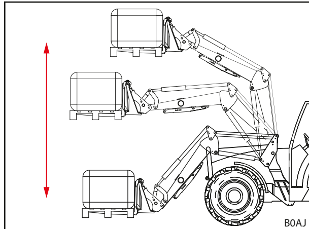
Σχ. 34 Παράλληλος οδηγός
