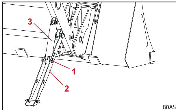
Σχ. 68 Στήριγμα στάθμευσης ανοιχτό
