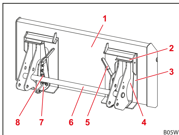
Σχ. 26 Κλειστός μηχανισμός ασφάλισης
