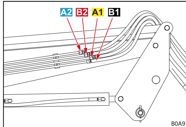
Σχ. 18 Υδραυλικοί σωλήνες
