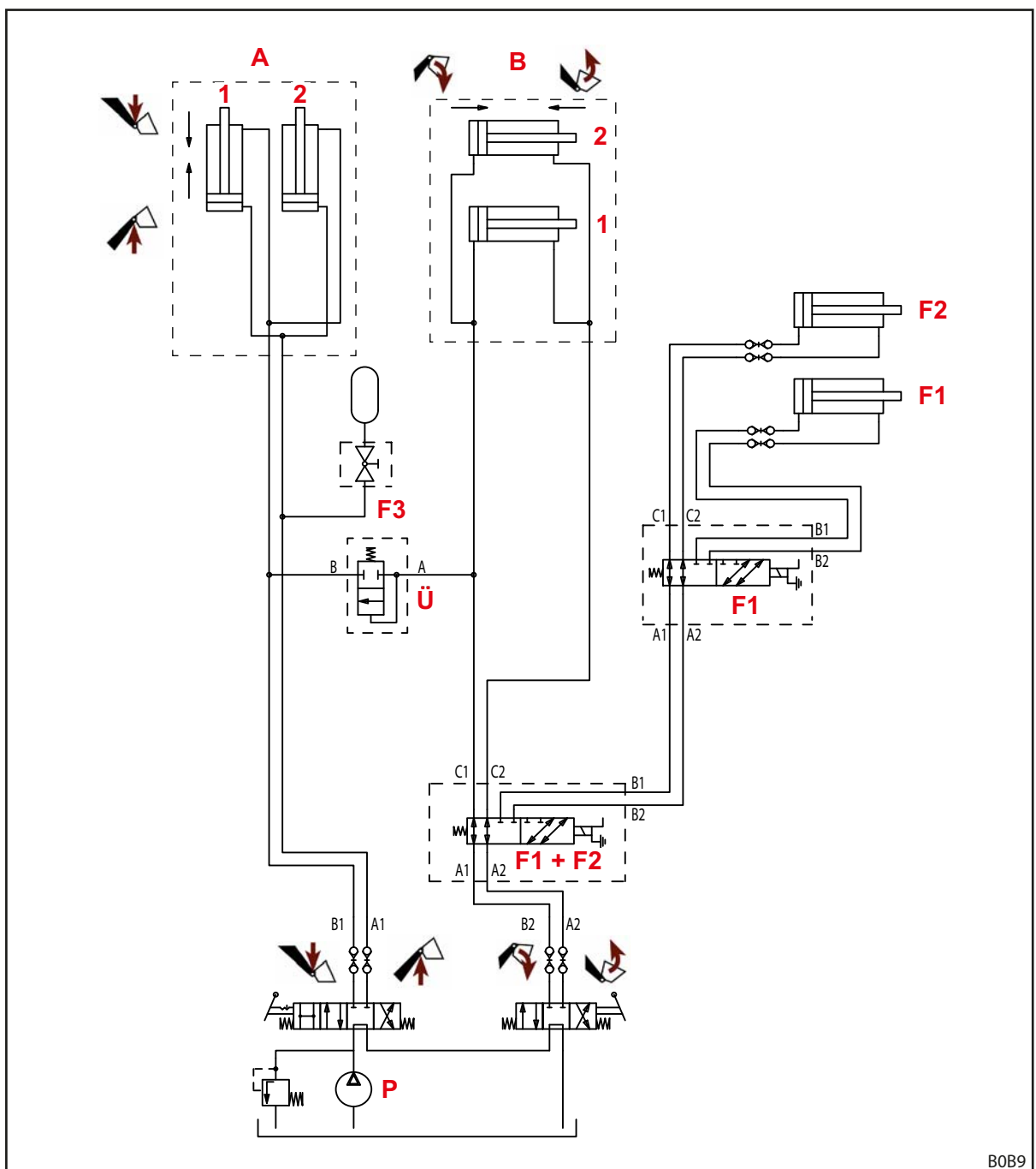
Σχ. 122 Υδραυλικό σχέδιο FC
