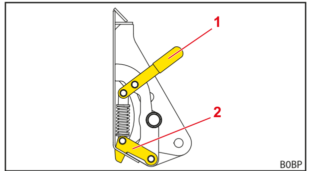
Σχ. 75 Μηχανικός μηχανισμός ασφάλισης εργαλείου Skid-Steer (ημίκλειστη κατάσταση)
