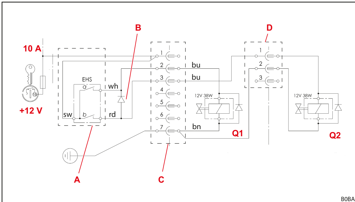
Σχ. 123 Ηλεκτρικό διάγραμμα συνδεσμολογίας
