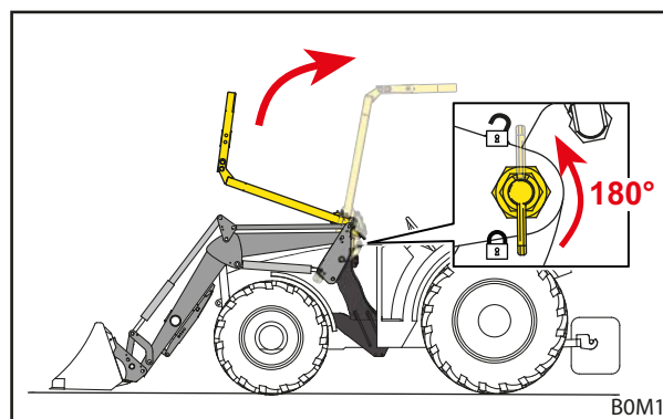
Σχ. 38 Ανέβασμα OPG
