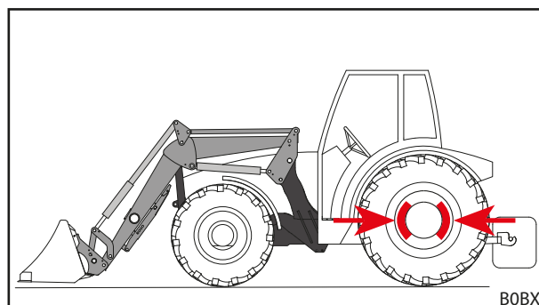
Σχ. 103 Τοποθετήστε το εργαλείο για απόθεση και τραβήξτε το χειρόφρενο
