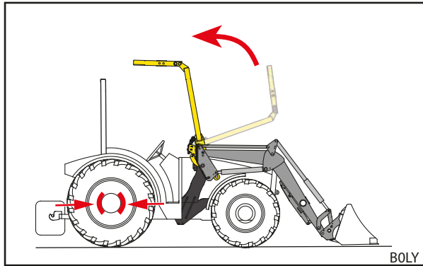
Σχ. 55 Ανέβασμα OPG
