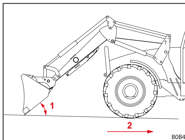
Σχ. 107 Ισοπέδωση με όπισθεν
