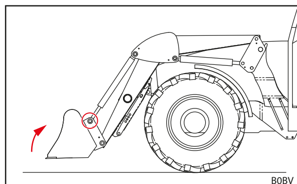
Σχ. 96 Σύνδεση εργαλείου επάνω με τους υδραυλικούς κυλίνδρους
