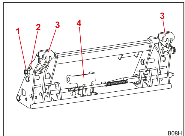
Fig. 14 Cadre porte-outils combiné Euro-FR
