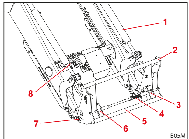
Fig. 10 Cadre porte-outils Euro
