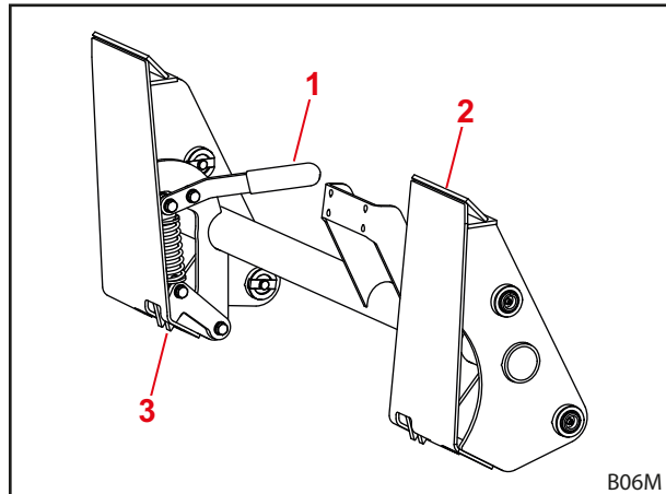
Fig. 20 Verrouillage mécanique de l'outil sur le cadre porte-outils Skid Steer
