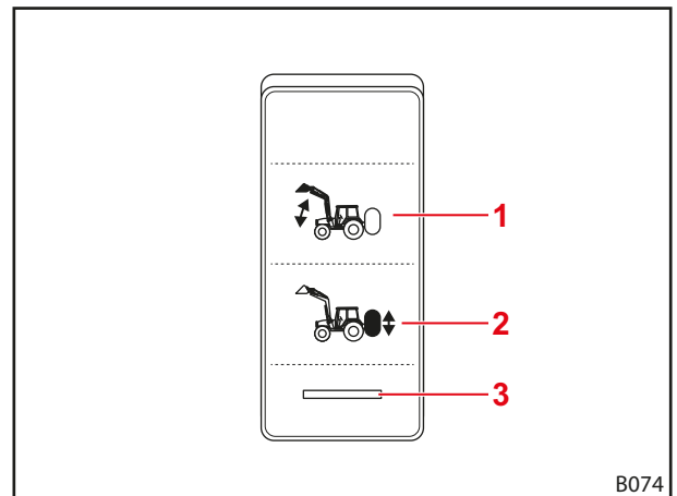
Fig. 54 Commutateur pour l'hydraulique confort
