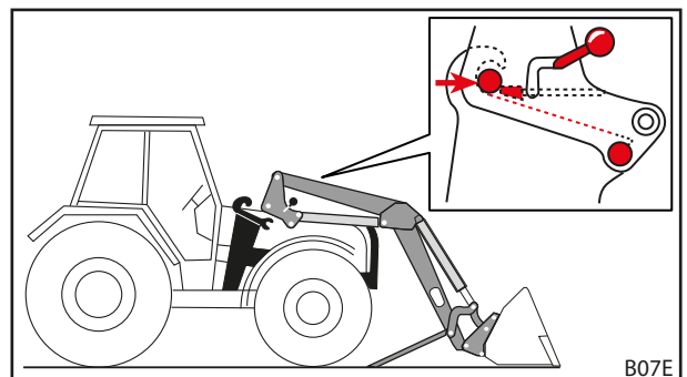
Fig. 37 Avancer le tracteur dans le brancard
