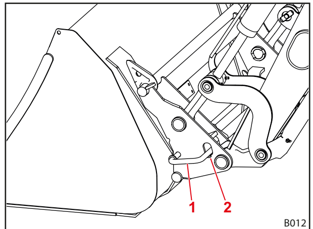
Fig. 59 Verrouillage mécanique de l'outil
