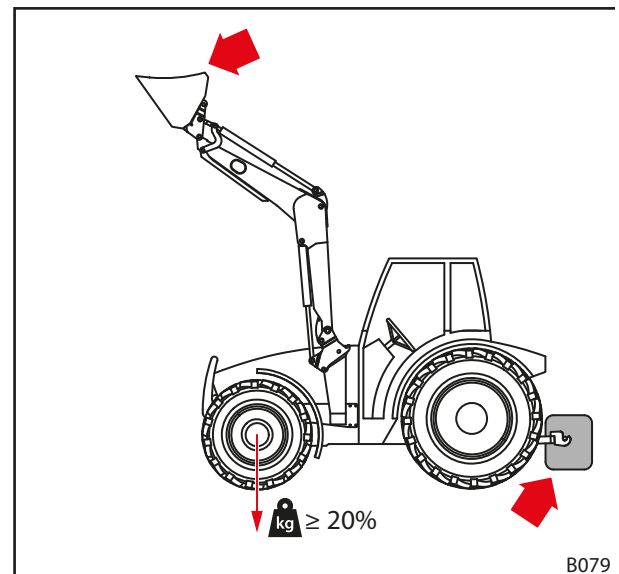
Fig. 34 Charge lors de la conduite sur route
