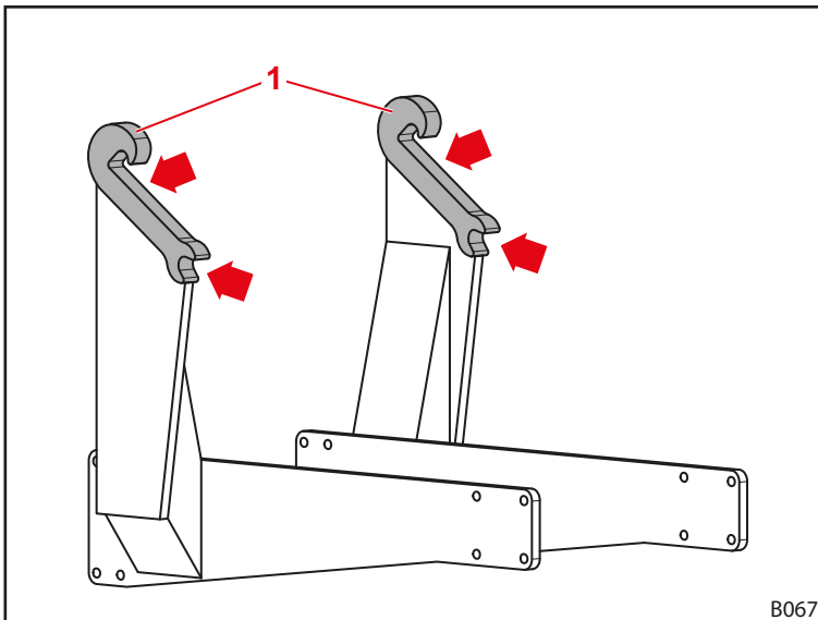
Fig. 86 Points de lubrification des logements du chargeur frontal
