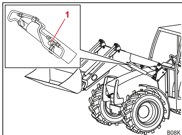
Fig. 31 Clapets limiteurs de descente
