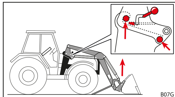
Fig. 39 Utiliser la fonction levage jusqu'à ce que les axes du chargeur frontal se trouvent dans le crochet d'arrêt
