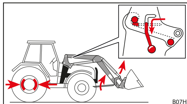
Fig. 40 Replier les béquilles et fermer le verrouillage du chargeur frontal
