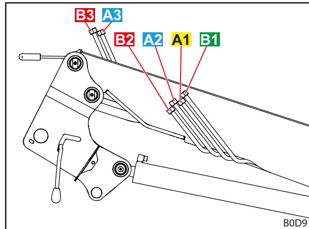
Kuva 18 Hydraulikkalinjat (erikoisvaruste REAL 3 )
