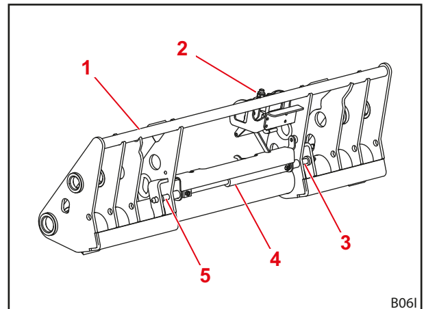
Kuva 16 Vahvistettu Euro-vaihtorunko (FZ 100)
