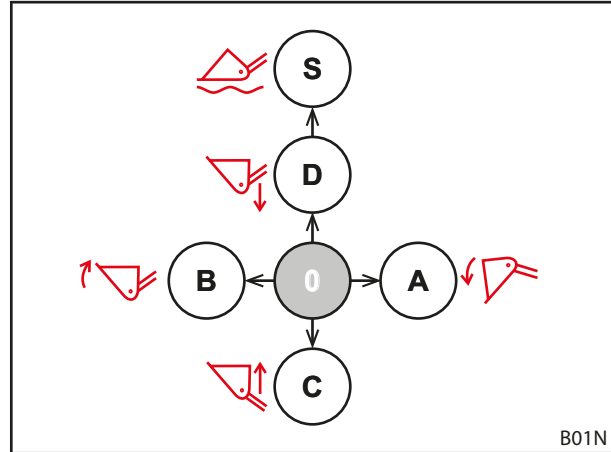
Kuva 62 Varaus, jos varustuksessa on yksi ohjausvipu
