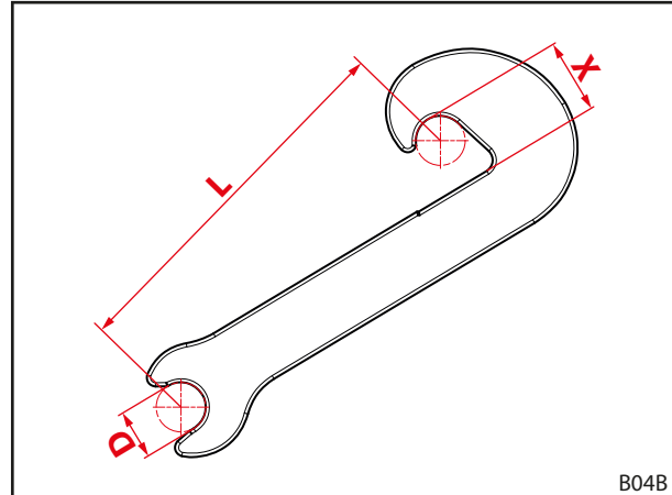
Kuva 116 Jarrutuskoukun kulumismitat
