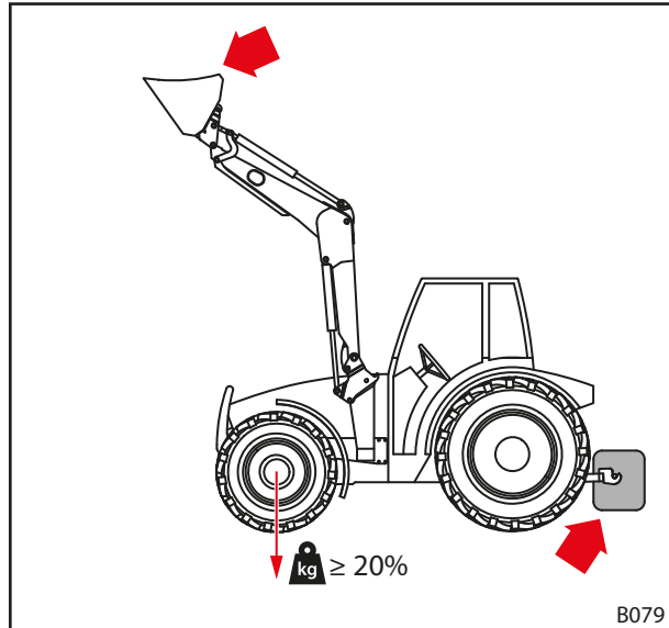
Kuva 45 Kuormitus julkisilla teillä ajettaessa
