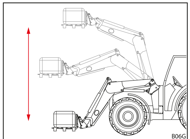
Kuva 33 Suoraviivaisen liikkeen ohjain
