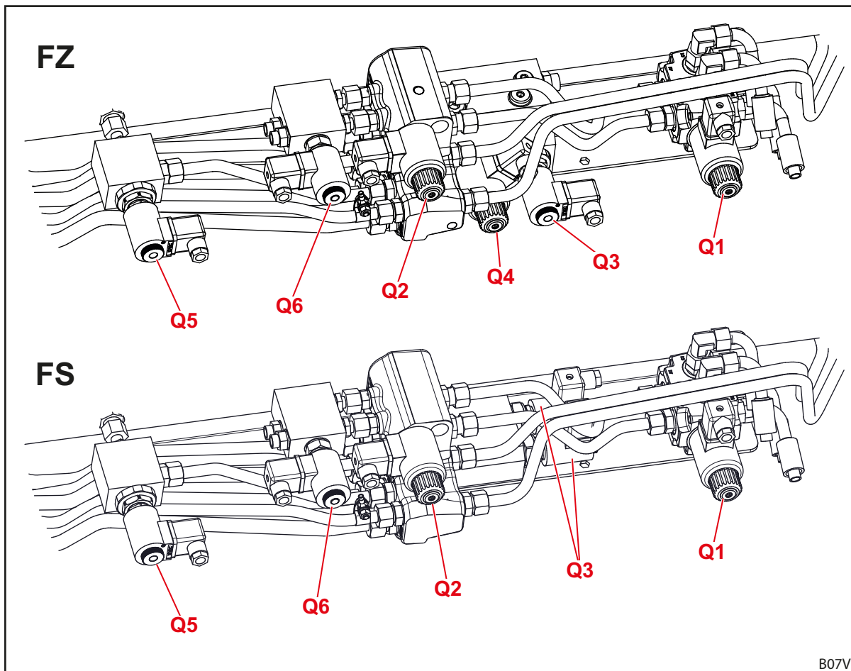
Kuva 133 Lisätoimintojen hydraulikkaventtiilien asettelu
