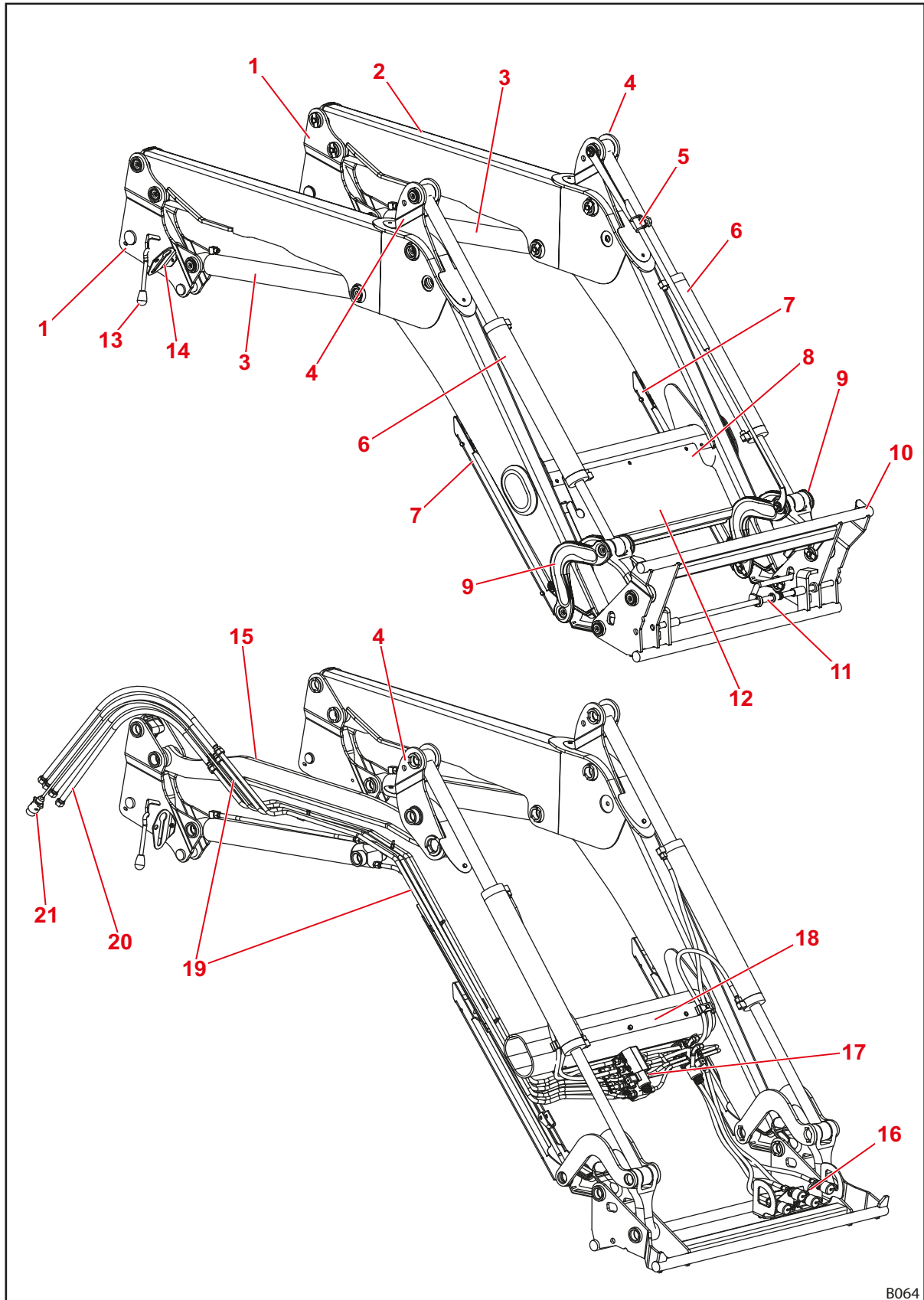
Kuva 8 Etukuormain FZ
