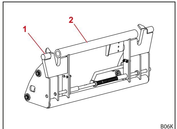
Kuva 12 Yhdistelmävaihtorunko Euro-SMS
