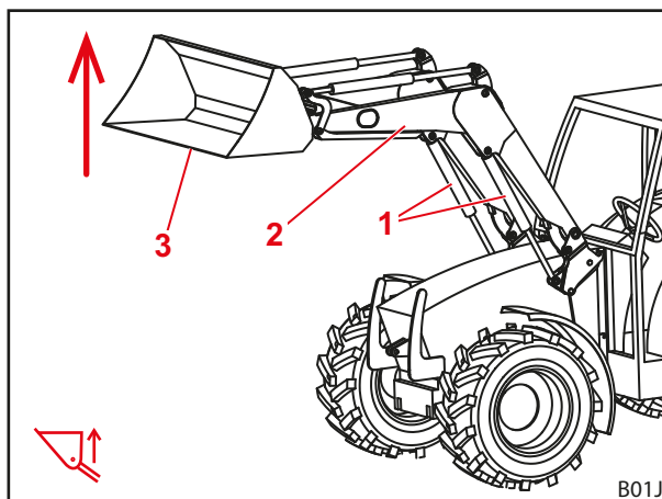
Kuva 27 Nosto-toiminto
