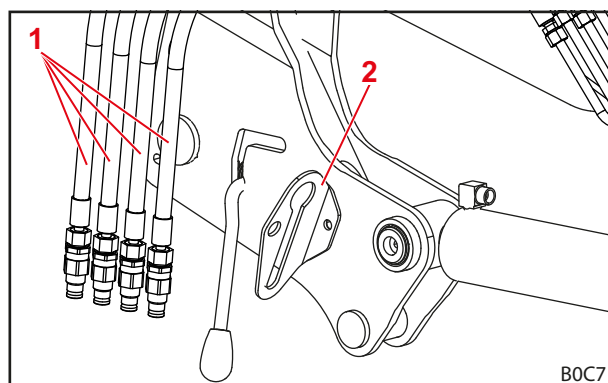
Kuva 126 Hydraulikkalinjojen kiinnittäminen kytkimen varteen (kuvassa pistoliitännöillä varustettuna)
