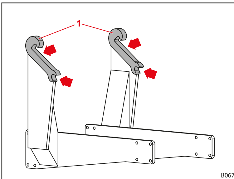
Kuva 113 Etukuormaimen kiinnittimien voitelukohdat
