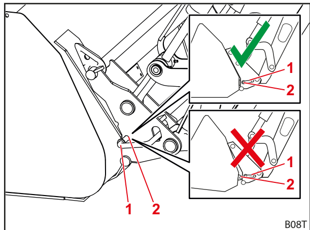
Kuva 83 Lukituspulttien sijainnin tarkastaminen
