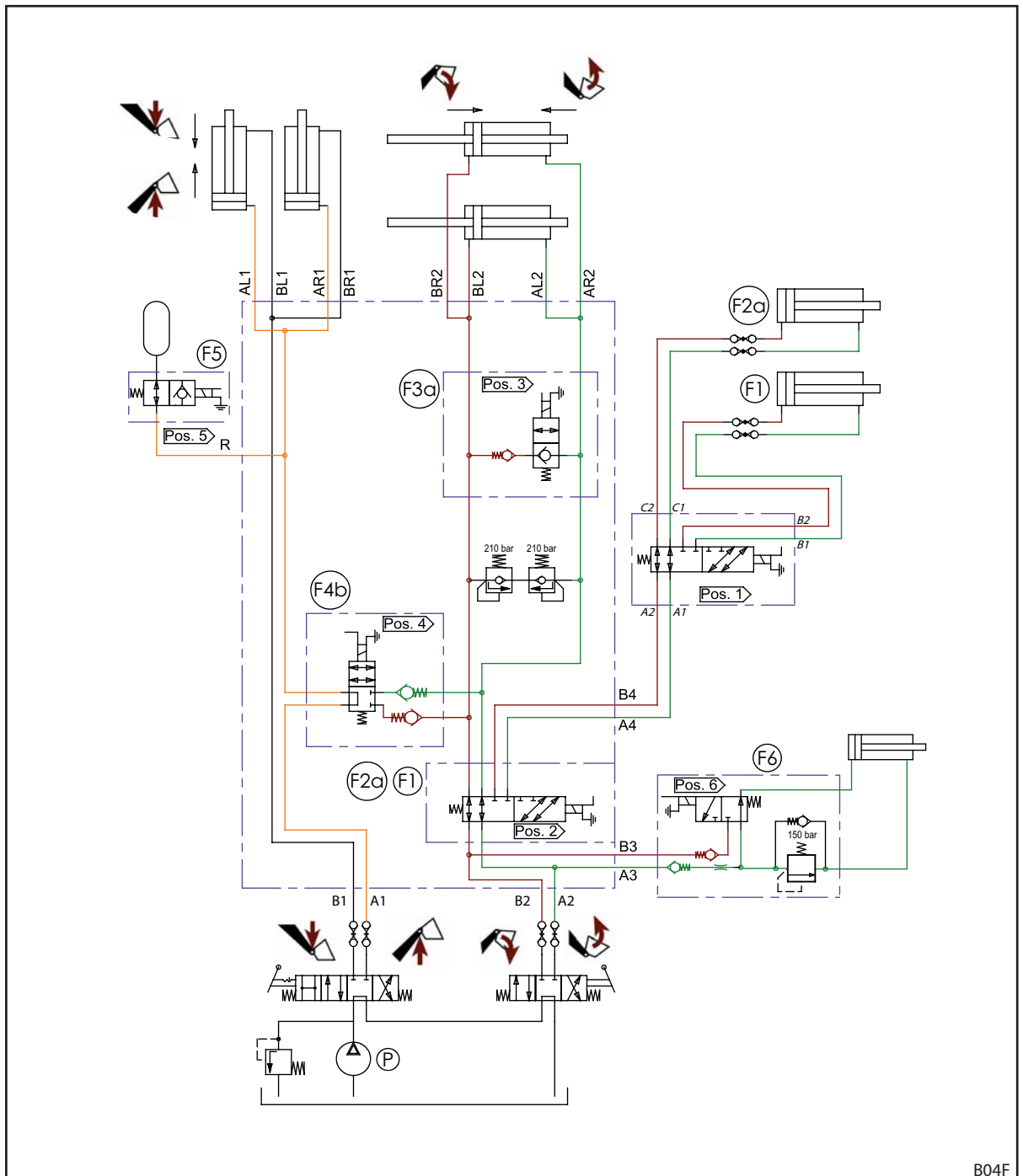
Kuva 129 Hydraulikkapiirustus FZ ja FZ-L (jos varustukseen kuuluu 3. ja 4. ohjauspiiri)
