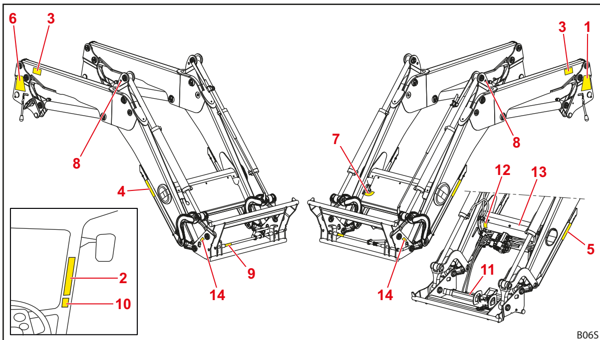
Kuva 4 Etukuormain FZ (kuva esimerkinomainen)
