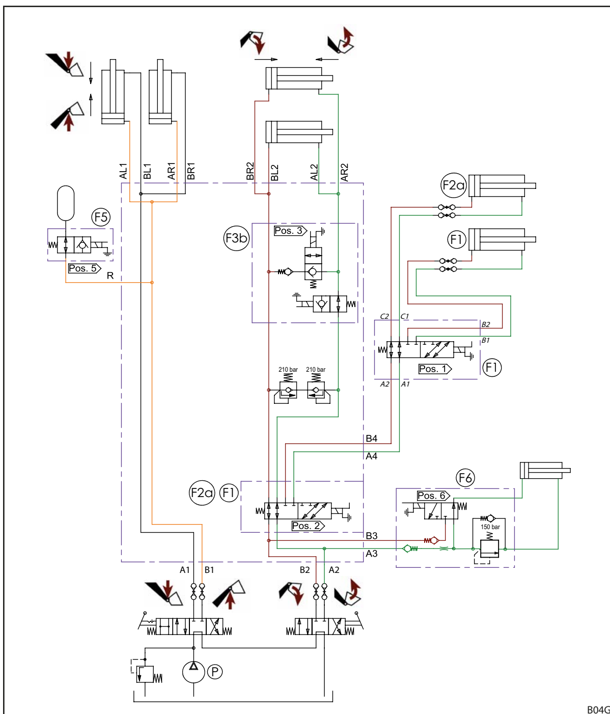
Kuva 127 Hydraulikkapiirustus FS ja FS-pikaliike (jos varustukseen kuuluu 3. ja 4. ohjauspiiri)
