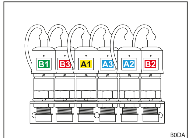
Kuva 20 Pistoliitännät liitettyinä (erikoisvaruste REAL 3 )
