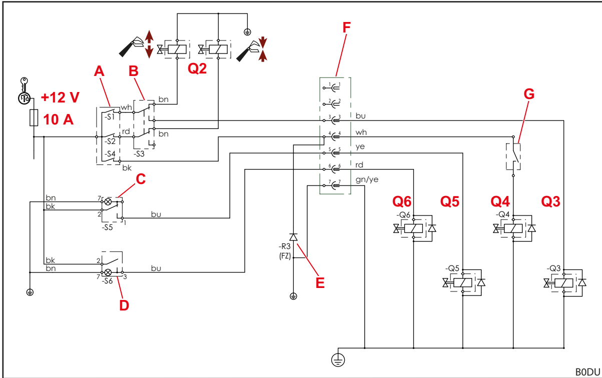
Kuva 132 Sähkökytkentäkaavio (jos varustukseen kuuluu REAL 3 )
