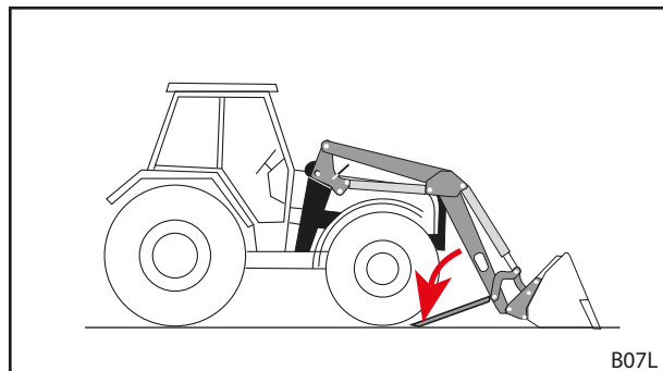
Kuva 123 Tukijalkojen taittaminen auki
