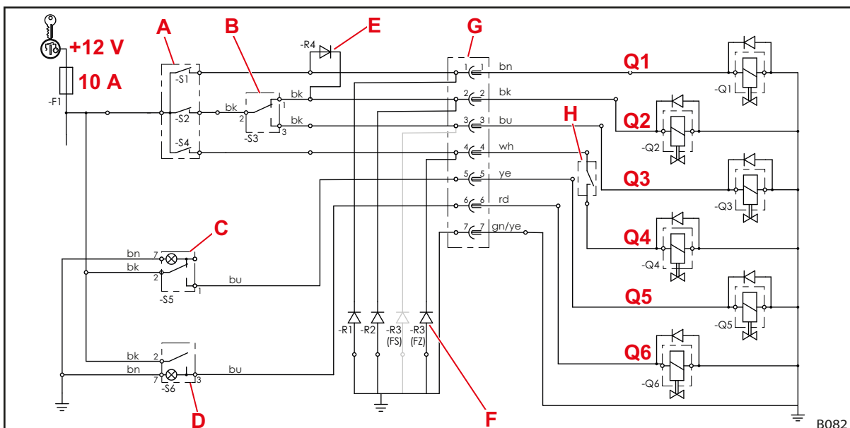
Kuva 131 Sähkökytkentäkaavio (jos varustukseen kuuluu 3. ja 4. ohjauspiiri)
