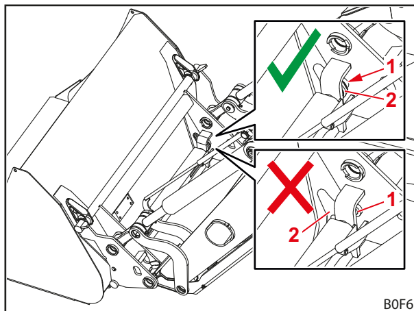
Kuva 90 Lukituspulttien sijainnin tarkastaminen
