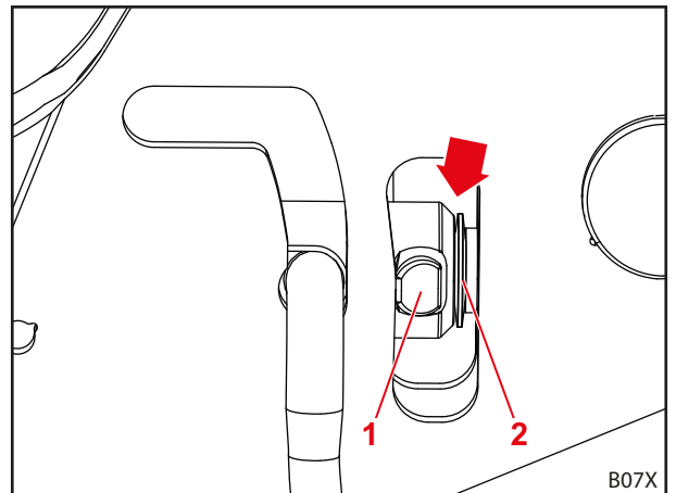
Kuva 119 Raon tarkastaminen
