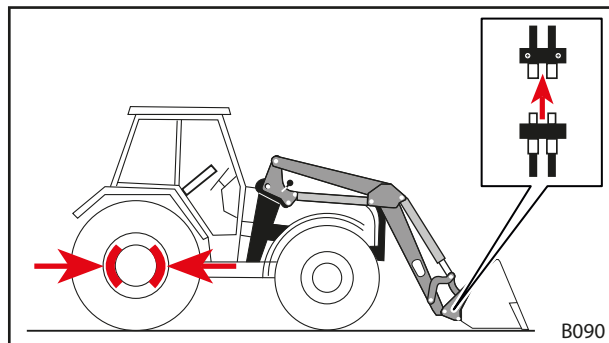
Kuva 105 Hydraulikkalinjojen irrotus
