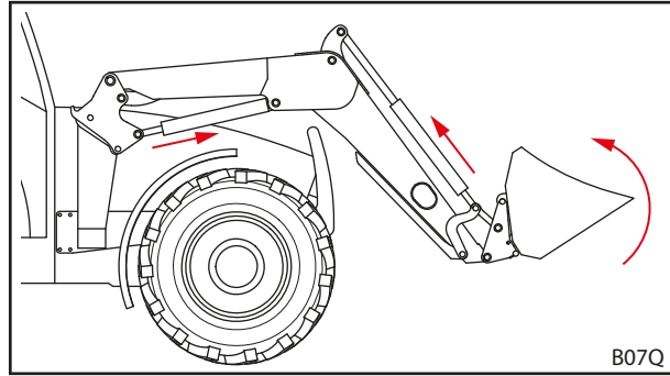
Kuva 96 Työkalun lukituksen laukaiseminen
