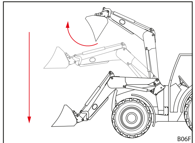
Kuva 35 Return-To-Level-toiminto
