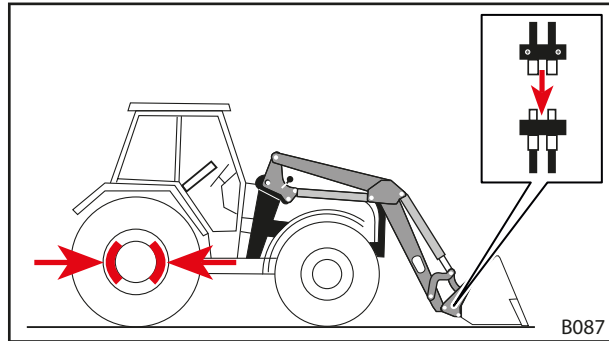
Kuva 97 Työkalun hydraulikkalinjojen liittäminen etukuormaimen liittimiin
