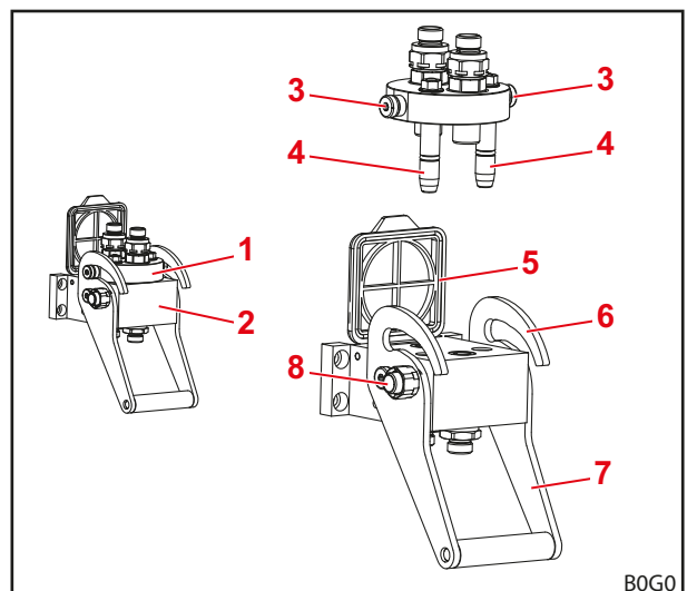
Kuva 24 Työkalu-Fix-liitännän rakenne
