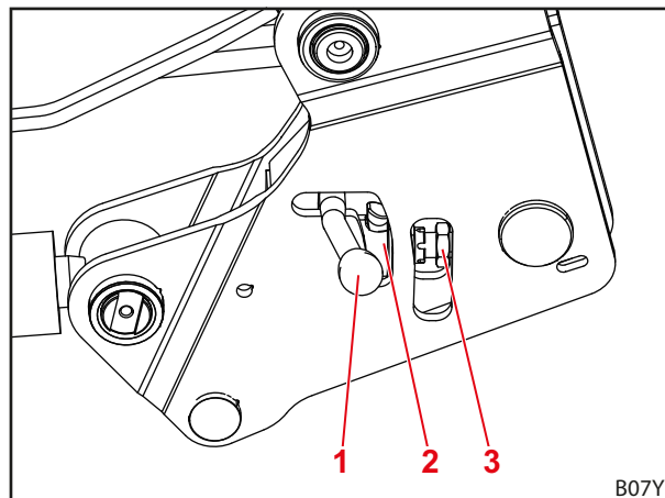
Kuva 57 Etukuormaimen lukituksen avaaminen
