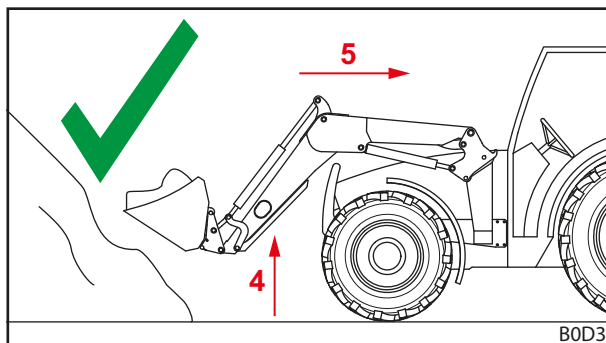
Kuva 112 Taaksepäin ajaminen kuorman kanssa – oikein
