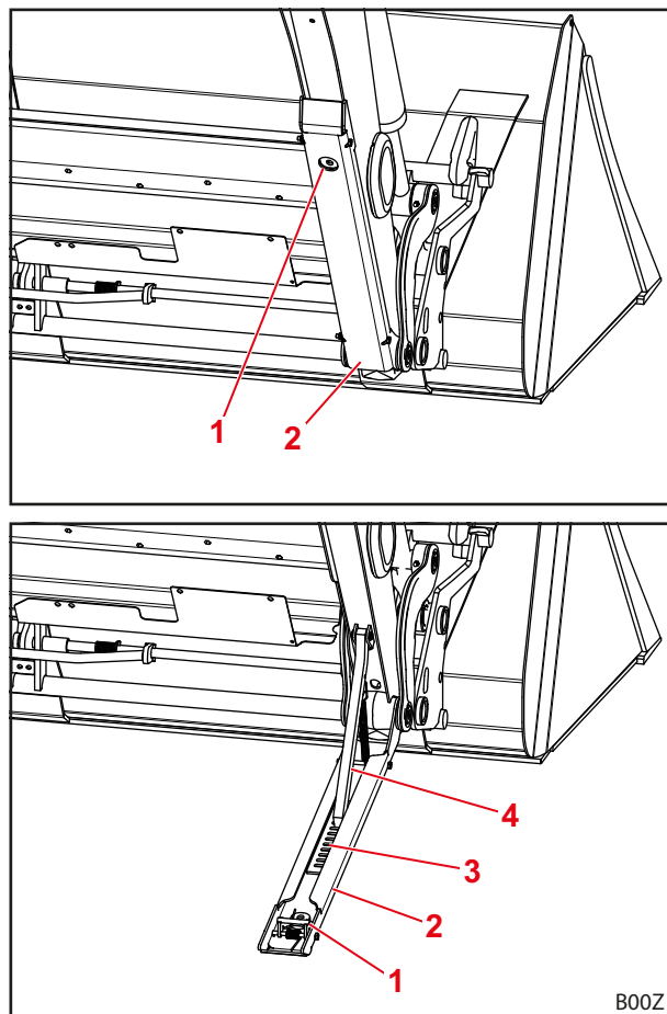
Kuva 74 Tukijalka
