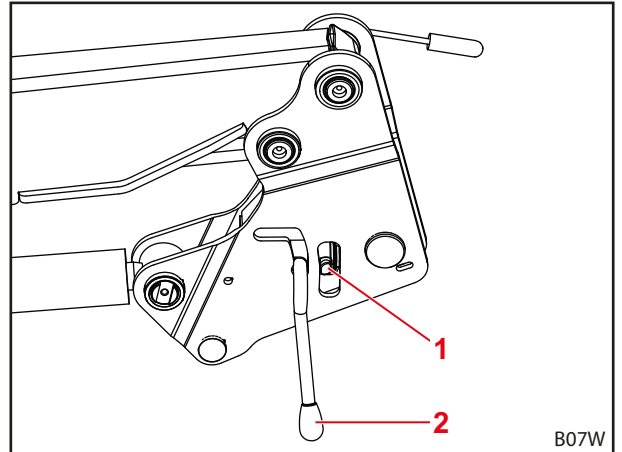
Kuva 118 Etukuormaimen lukituksen tarkastus
