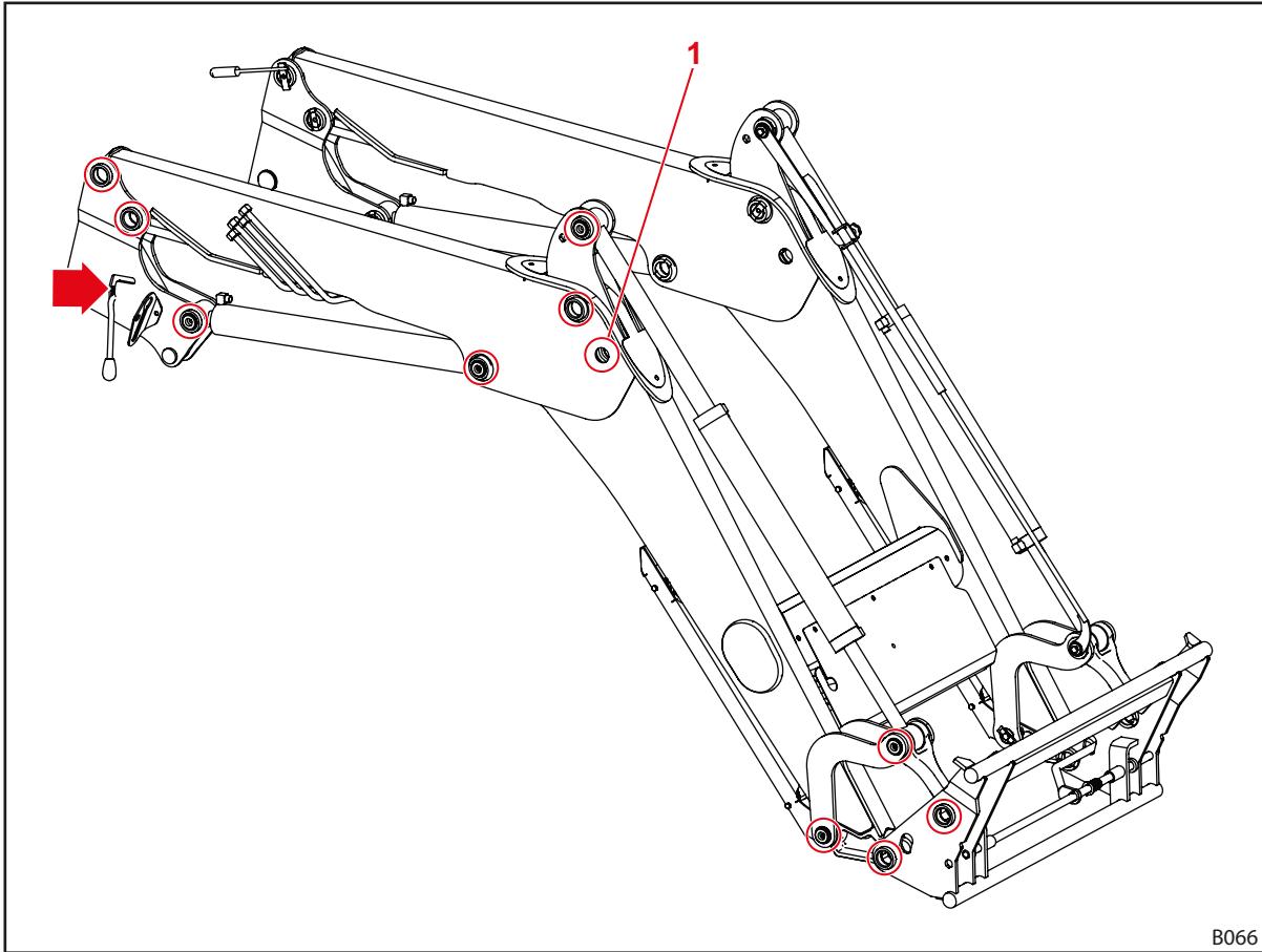
Kuva 115 Voitelukohdat FZ
