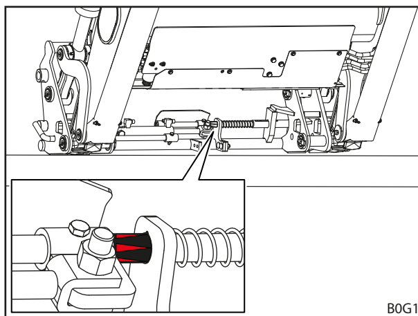
Kuva 88 Tarkasta työkalun lukitus tarran perusteella
