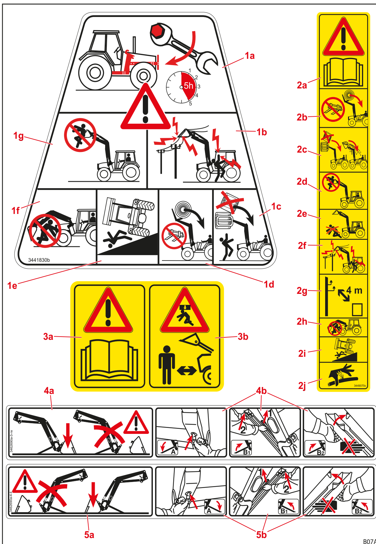
Kuva 5 Varoitustarrat, sijainti 1-5
