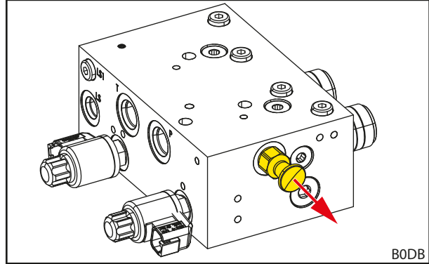
Kuva 72 Vedä REAL 3 -venttiilin paineenalennusventtiili ulos
