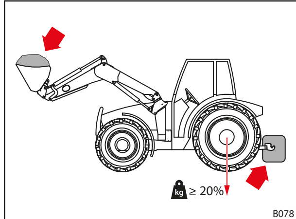
Kuva 44 Kuormitus etukuormaimella työskenneltäessä
