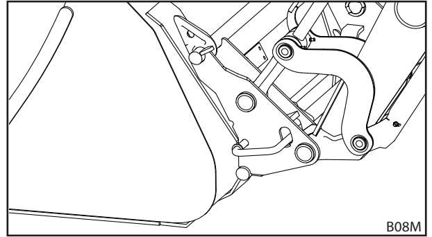
Kuva 92 Työkalun lukituksen avaaminen
