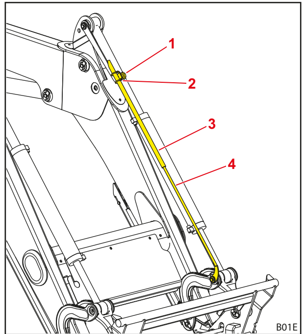
Kuva 32 Työkalun asennon näyttö
