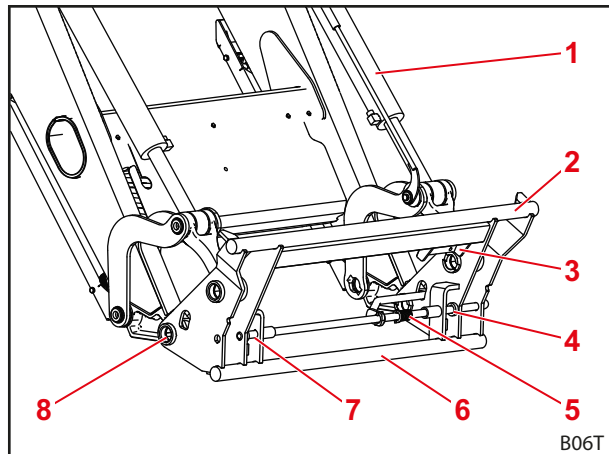
Kuva 10 Euro-vaihtorunko
