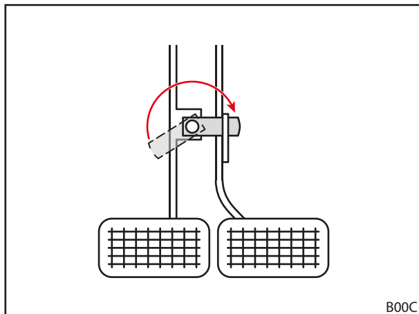
Kuva 43 Jarrupolkimien kytkeminen
