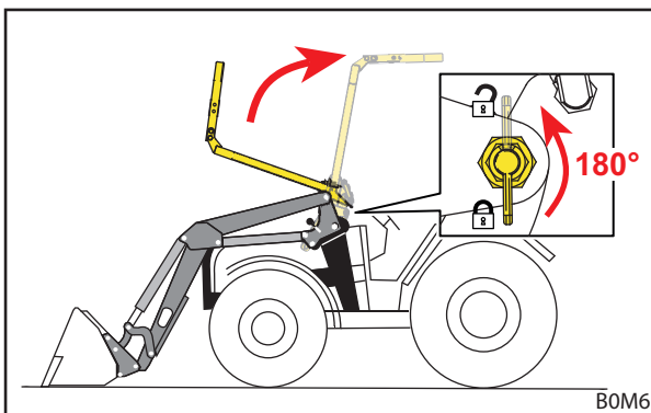
jn 38 OPG ülespööramine
