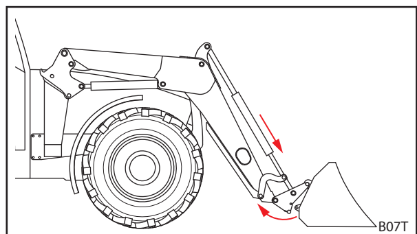
jn 107 Vahetusraami lahtihaakimine
