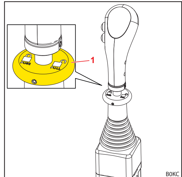
jn 68 Juhthoova lukustamine (vertikaalne lukustus)
