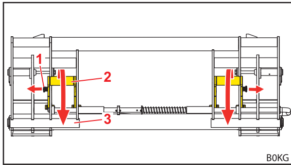
jn 89 Seadmete allapööramine
