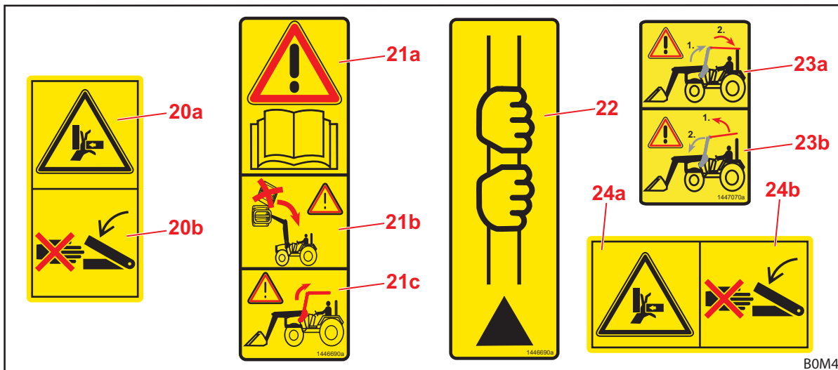
jn 9 Turvakleebised
