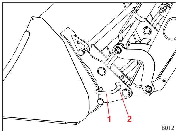
jn 82 Tööseadise mehaaniline lukustus
