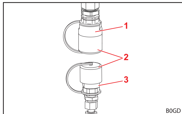
jn 80 Keermesliitmikud (näitlik joonis)
