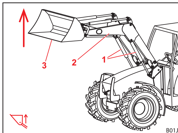
jn 28 Tõstmisfunktsioon
