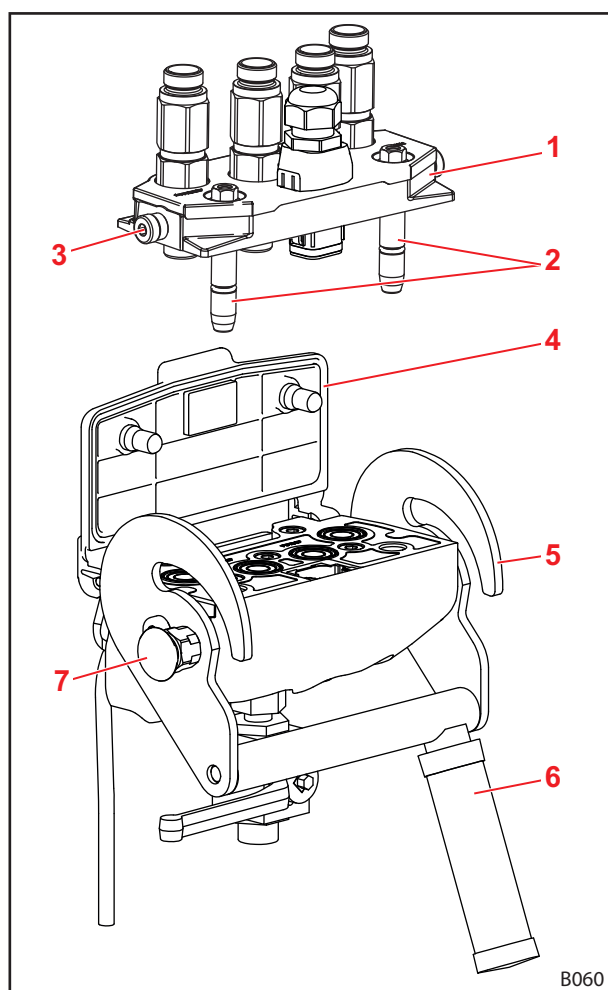
jn 81 Hydro-Fix (näide: Hydro-Fix 4-kordne)
