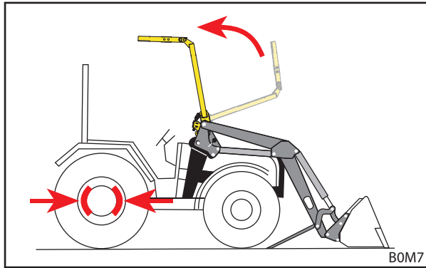
jn 56 OPG ülespööramine
