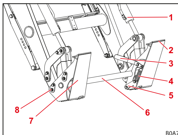
jn 16 Skid-Steer vahetusraam
