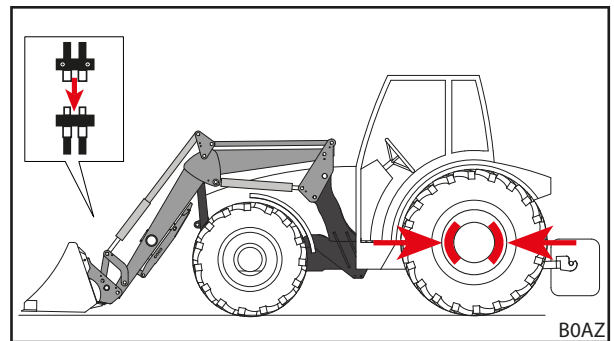
jn 93 Juhtkontuuri külgeühendamine
