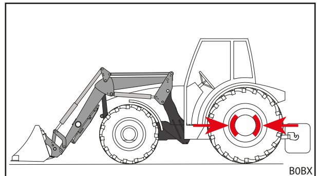
jn 103 Tööseadise positsioneerimine eemaldamiseks ja seisupiduri rakendamine
