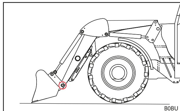
jn 95 Ühendage tööseadis poltide alumiste avade kaudu külge
