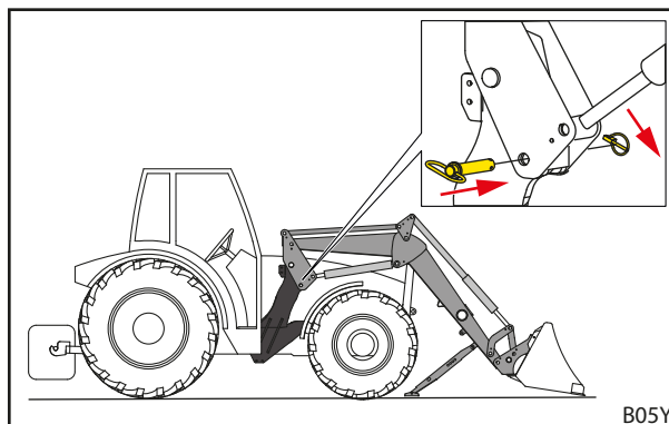
jn 56 Lukustuspoltide sisselükkamine ja rõngassplintidega fikseerimine
