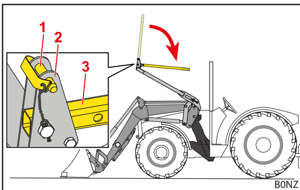
jn 43 Allapööratud ülemine kaar
