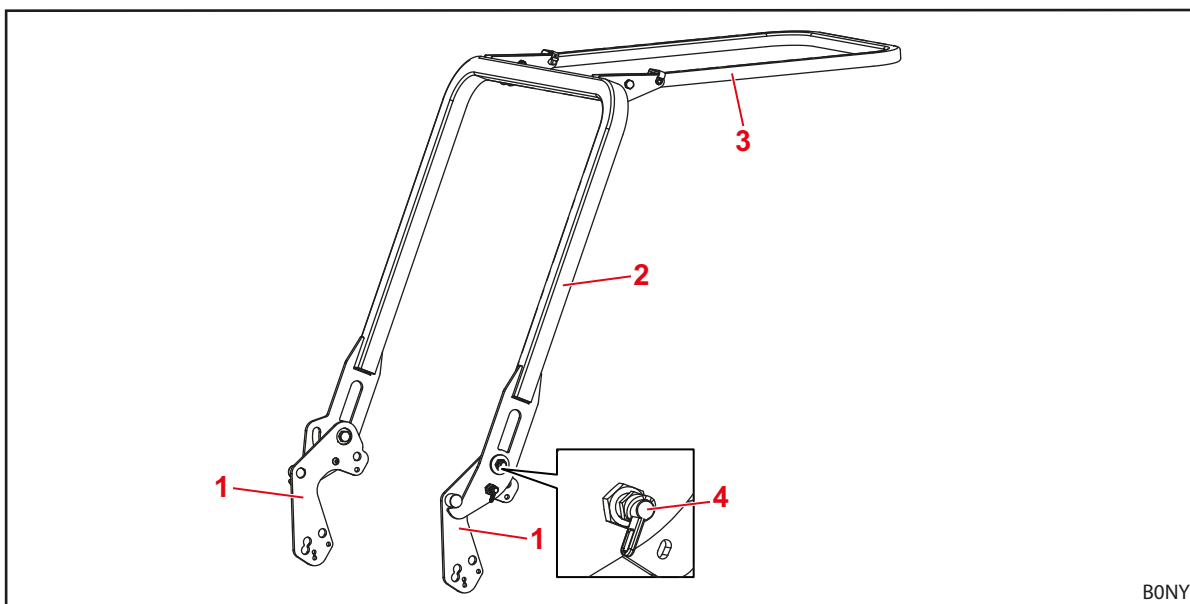
jn 13 Operator Protective Guard, OPG ette paigaldatud 2-postiga ümberminekukaitsetarindiga traktorite jaoks (näitlik kujutis)
