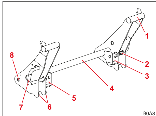
jn 27 Euro-vahetusraam
