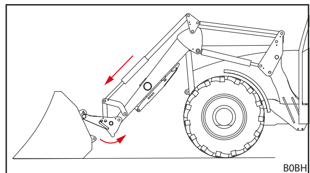
jn 101 Vahetusraami lahtihaakimine
