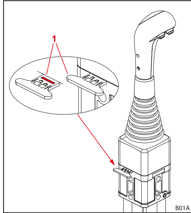
jn 61 Juhthoova lukustus
