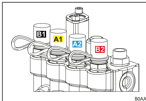
jn 20 Pistikmuhvide pistikud vahetult hüdroventiili küljes
