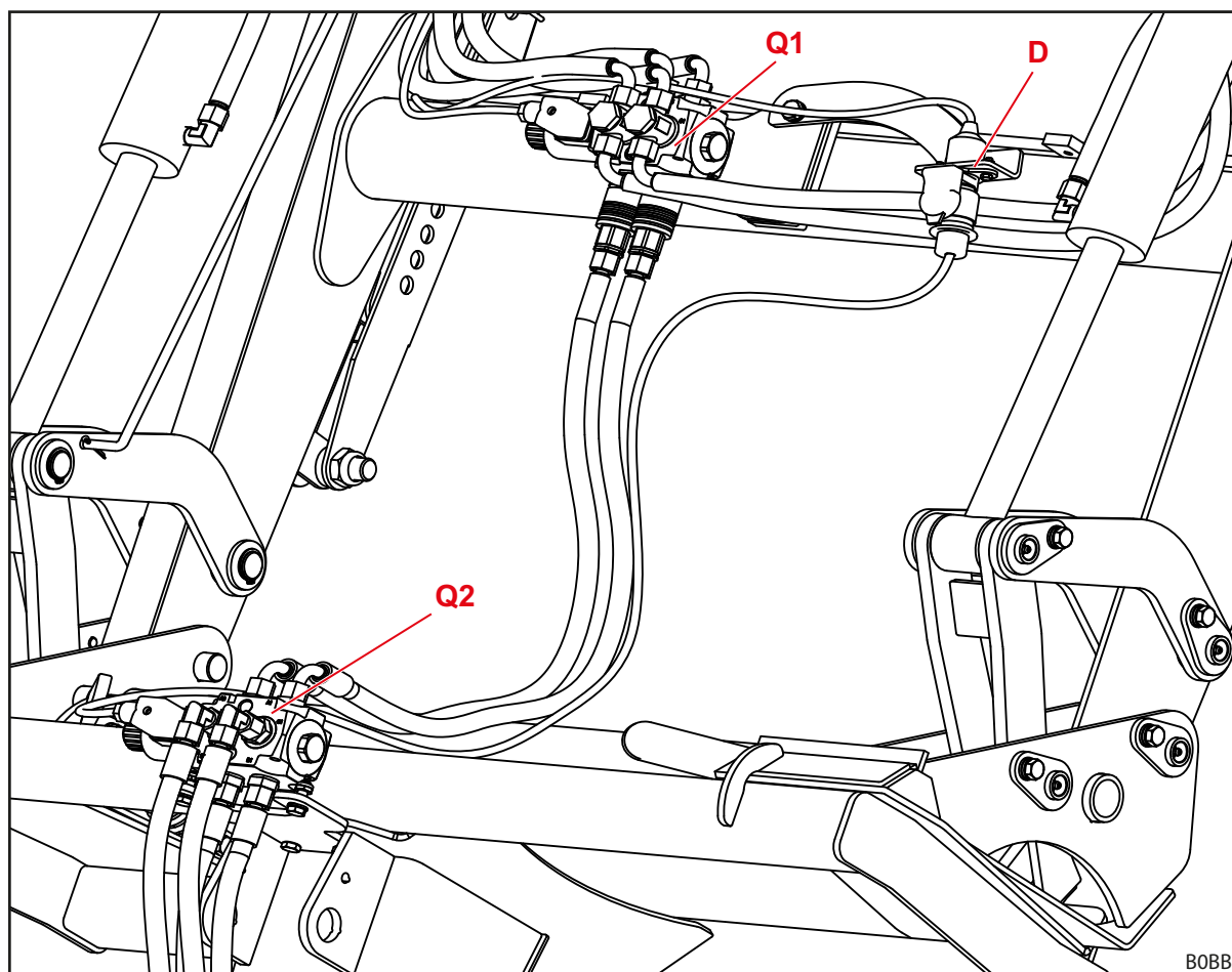
jn 124 Lisafunktsioonide hüdroventiilide paigutus
