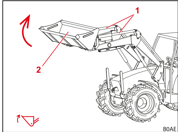
jn 30 Kopa täitmise funktsioon
