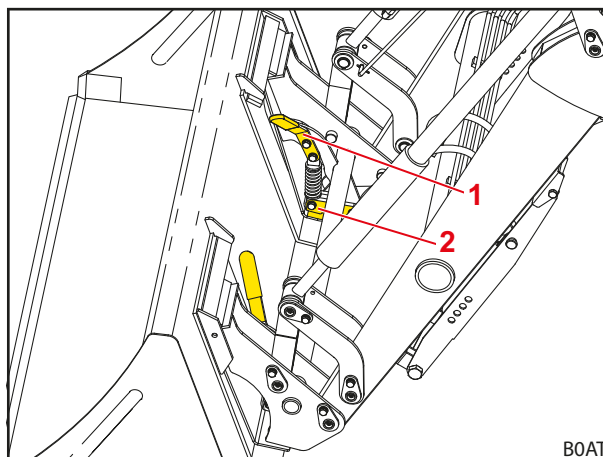
jn 77 Skid-Steeri tööseadise mehaaniline lukustus (lukustatud olek koos tööseadisega)
