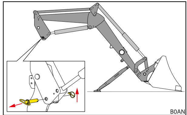
jn 52 Lauplaaduri lukustuse avamine
