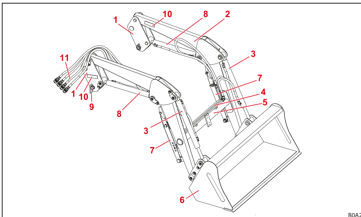
jn 9 Lauplaadur L (näitlik joonis)
