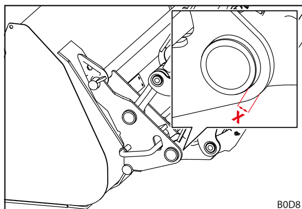
jn 117 Vahetusraami kulumismõõt
