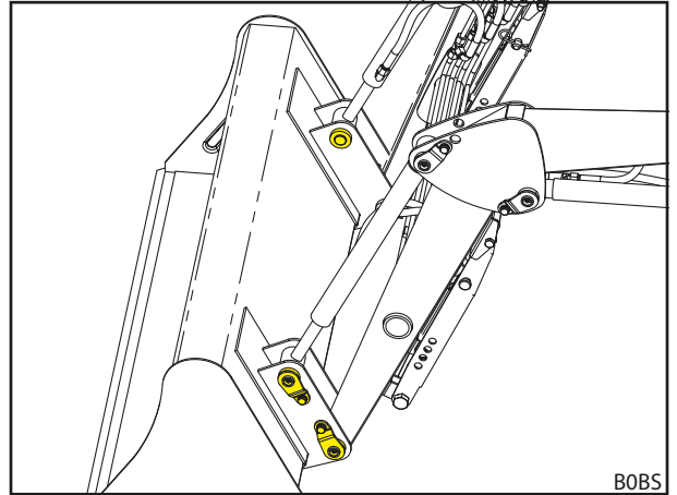
jn 97 Külgeühendatud tööseadis
