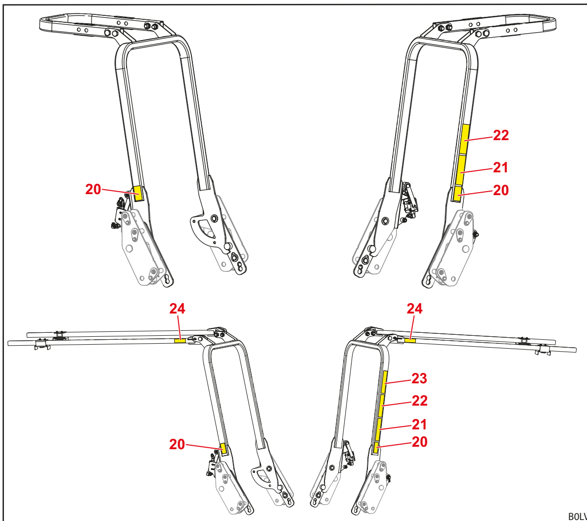
jn 6 OPG taha paigaldatud 2-postiga ümberminekukaitsetarindiga traktorite jaoks (näitlik kujutis)
