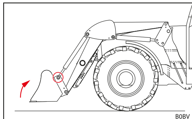
jn 96 Ühendage tööseadis üleval hüdrosilindritega
