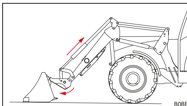
jn 86 Külgehaakimine
