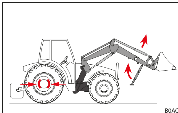
jn 57 Tugiseadiste sissepööramine
