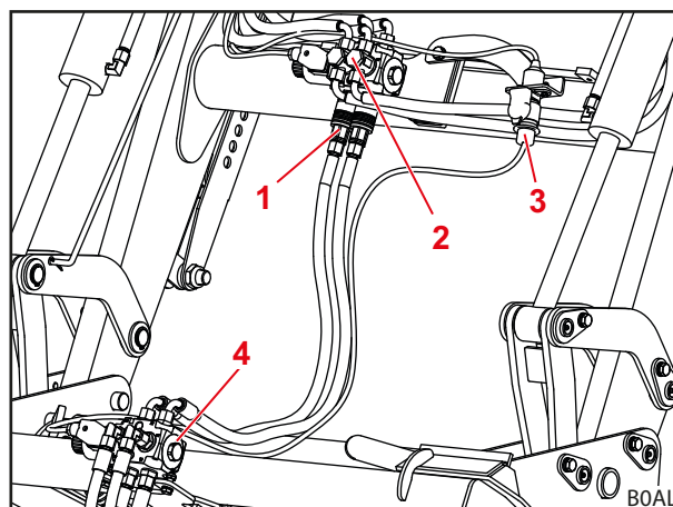
jn 46 Täiendav 4. juhtkontuur
