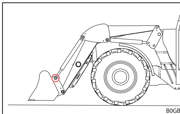
jn 104 Ülemise poldi väljatõmbamine
