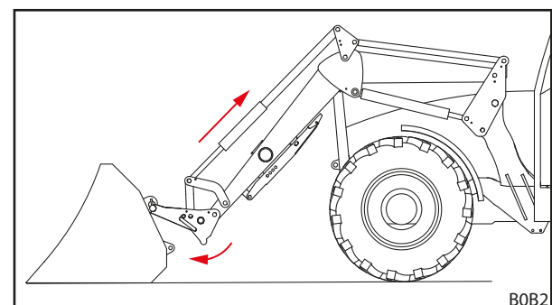
jn 91 Külgehaakimine
