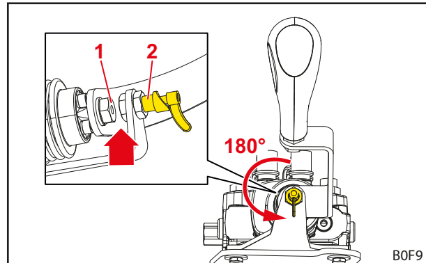
jn 65 Lukustusest vabastatud juhthoob
