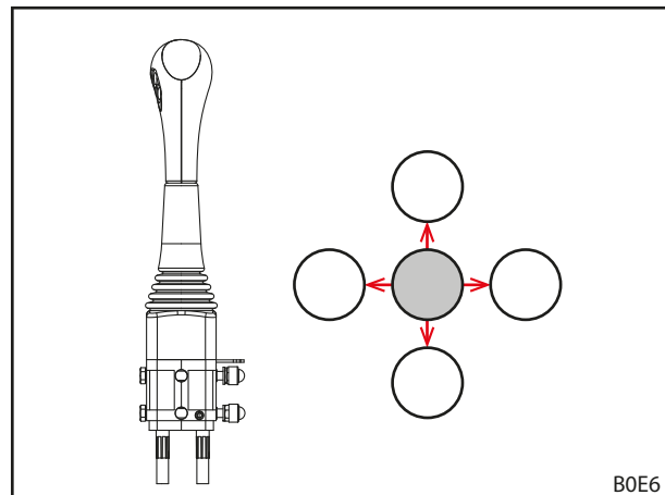
jn 62 Juhthoova liigutamine kõikidesse lõppasenditesse
