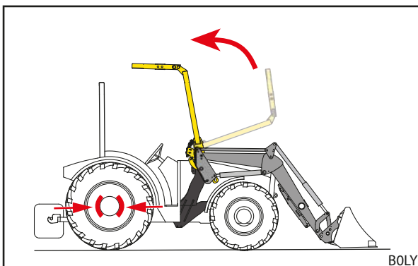
jn 55 OPG ülespööramine
