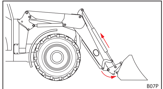
Abb. 111 Einhaken
