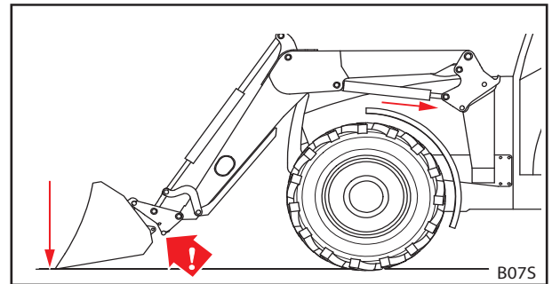
Abb. 85 Werkzeug auf den Boden drücken
