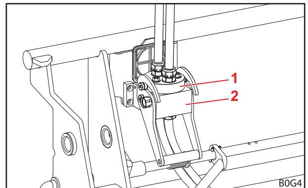
Abb. 82 Angekuppeltes Werkzeug-Fix
