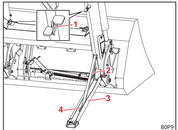
Abb. 77 Abstellstütze ausgeklappt
