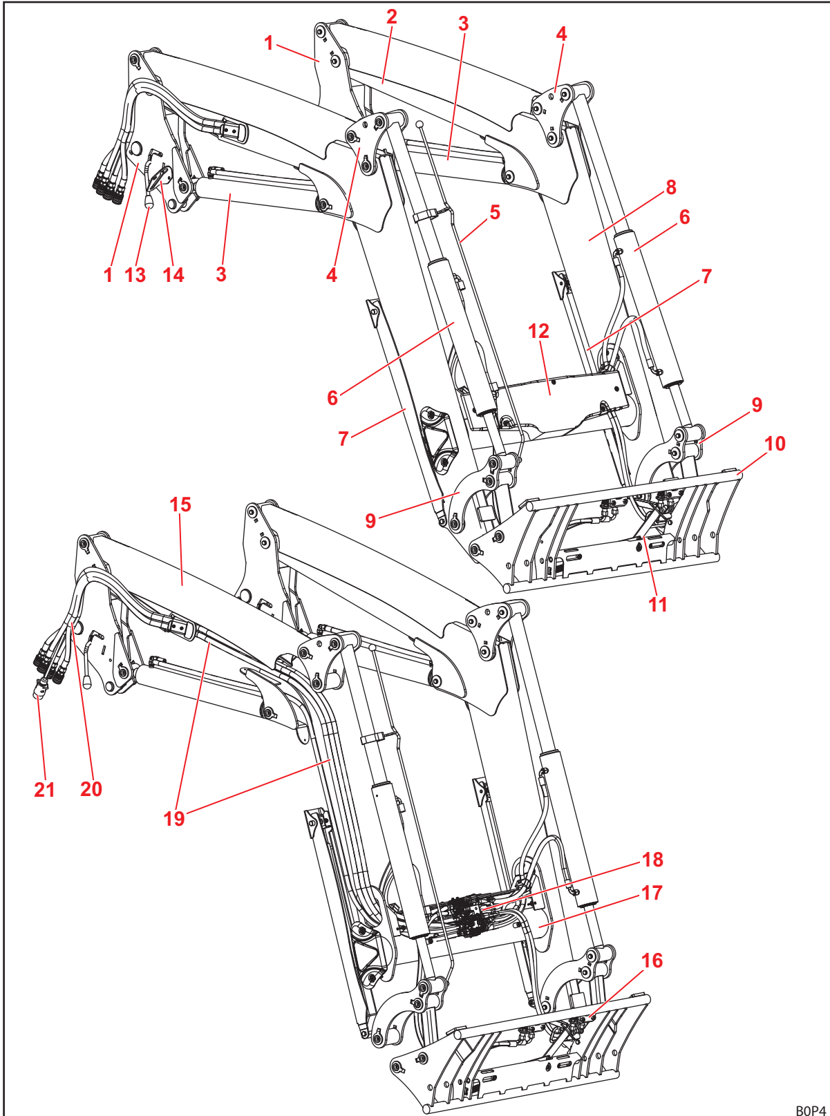
Abb. 10 Frontlader TL
