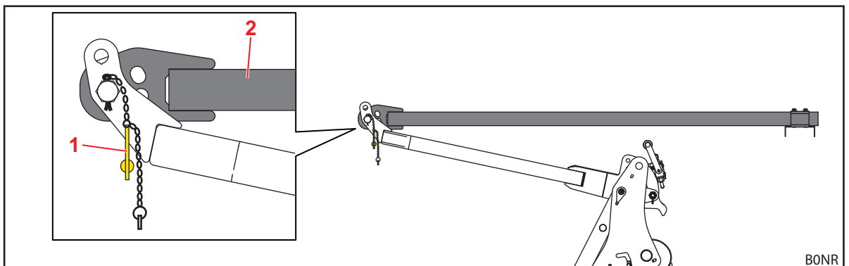
Abb. 40 Vollständig heruntergeklappte Traversen
