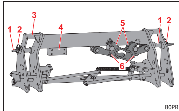
Abb. 17 Kombi-Wechselrahmen Euro-MX (vorbereitet für Euro-Werkzeug)
