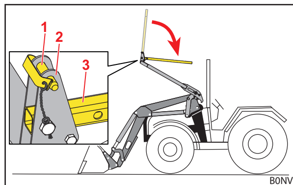
Abb. 42 Heruntergeklappter oberer Bügel
