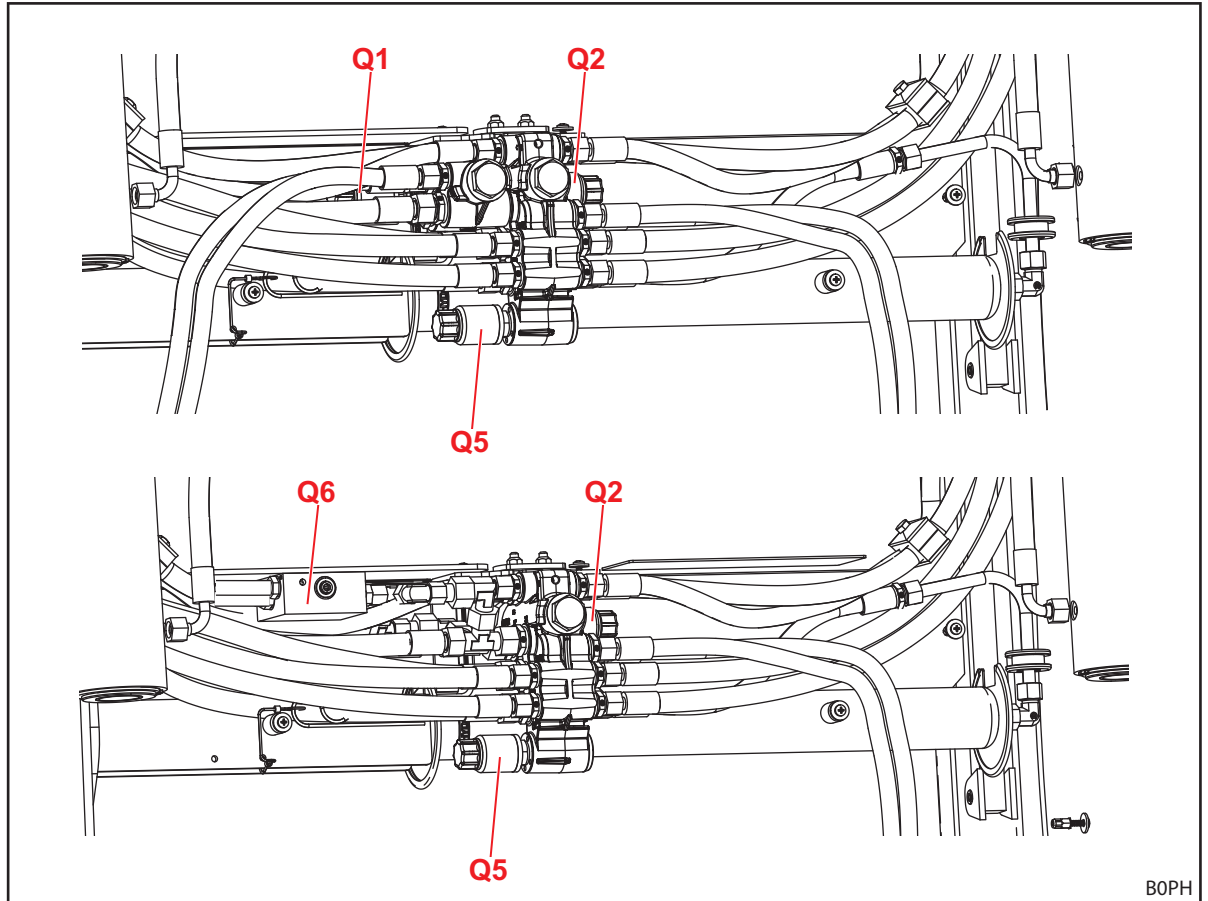
Abb. 135 Anordnung der Hydraulikventile für Zusatzfunktionen
