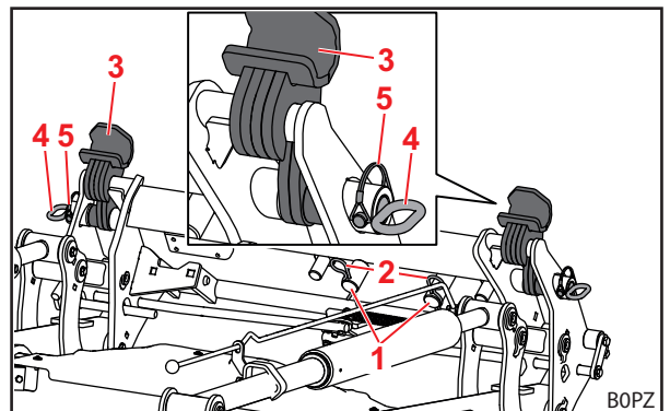
Abb. 102 Adapter in Arbeitsposition (Wechselrahmen vorbereitet für MX-Werkzeug)
