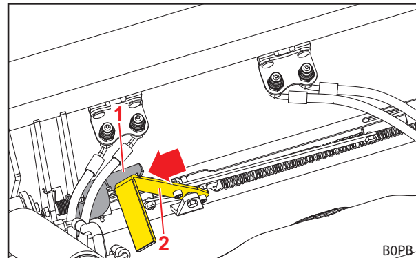
Abb. 83 Geöffnete Werkzeug-Verriegelung
