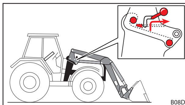
Abb. 127 Frontlader-Verriegelung lösen
