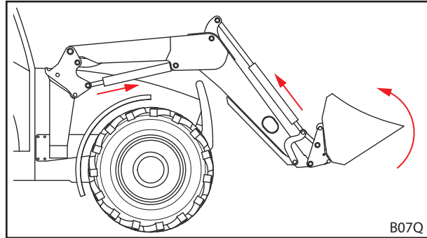
Abb. 108 Werkzeug-Verriegelung auslösen
