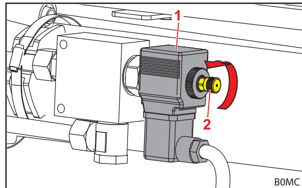
Abb. 34 Ventil öffnen
