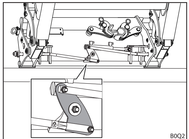
Abb. 94 Werkzeug-Verriegelung anhand des Aufklebers prüfen (Kombi-Wechselrahmen Euro-MX)
