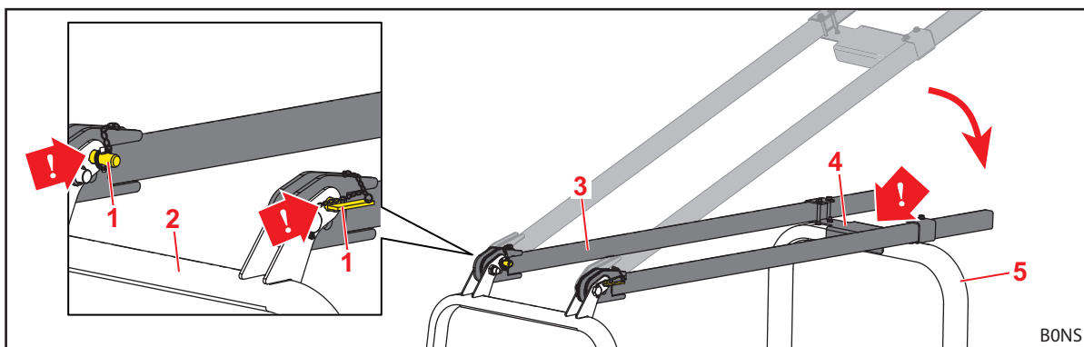
Abb. 41 Heruntergeklappte und in oberen Löchern gesicherte Traversen
