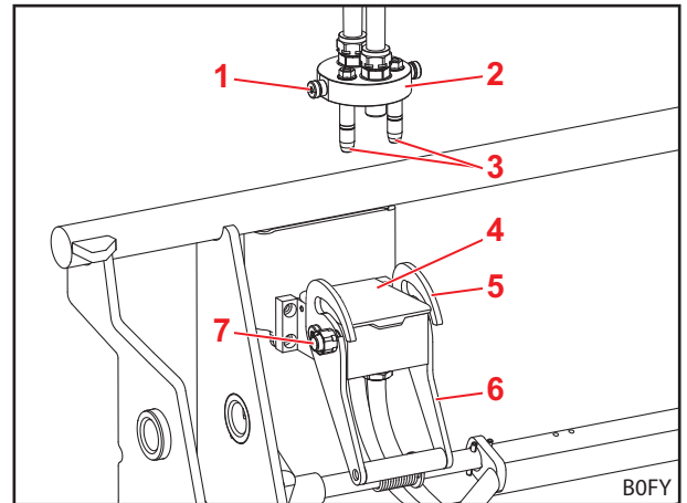
Abb. 81 Abgekuppeltes Werkzeug-Fix
