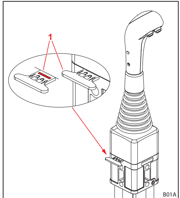
Abb. 65 Verriegelung des Bedienhebels (horizontale Verriegelung)
