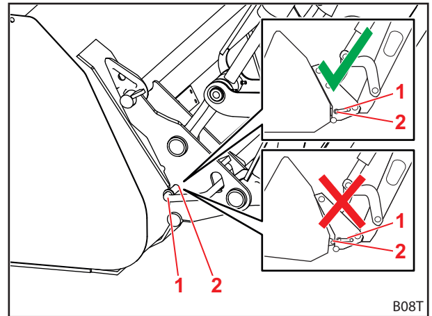
Abb. 89 Position der Verriegelungsbolzen prüfen
