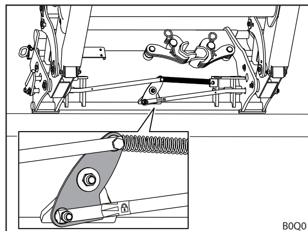
Abb. 88 Werkzeug-Verriegelung anhand des Aufklebers prüfen (Kombi-Wechselrahmen Euro-MX)
