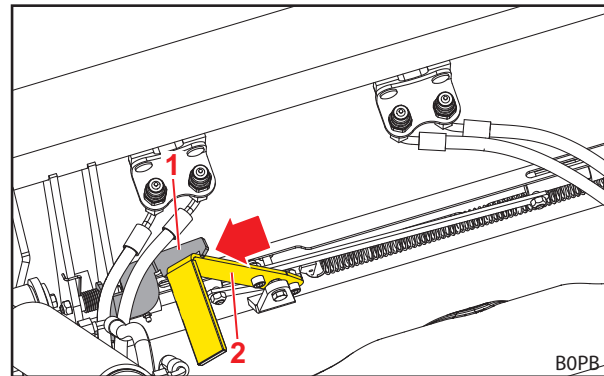
Abb. 103 Geöffnete Werkzeug-Verriegelung
