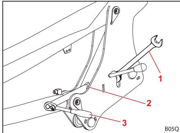
Abb. 59 Werkzeug anlegen
