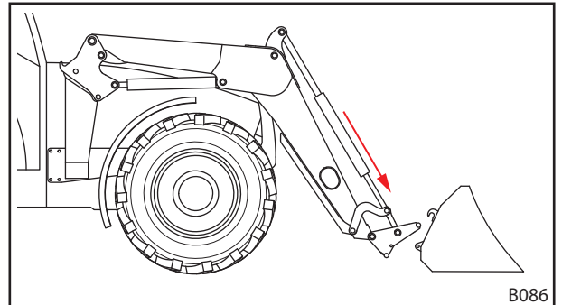
Abb. 105 Schwingen positionieren
