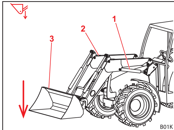
Abb. 28 Senken-Funktion
