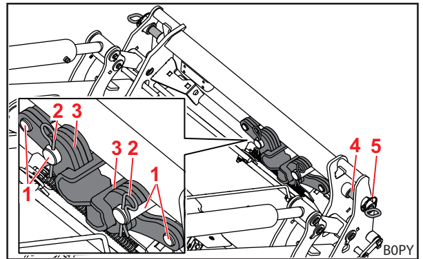
Abb. 101 Adapter in Parkposition (Wechselrahmen vorbereitet für Euro-Werkzeug)
