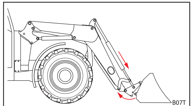
Abb. 114 Wechselrahmen aushaken
