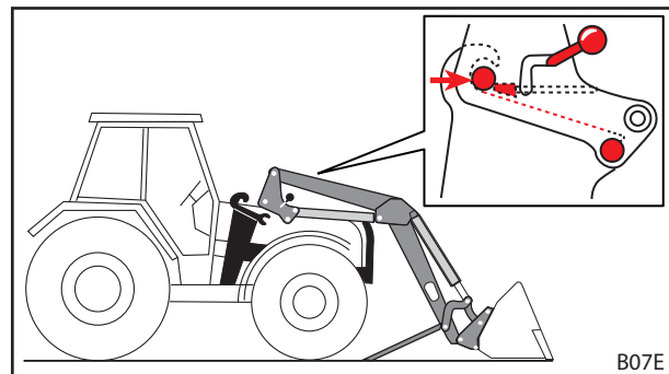
Abb. 52 Traktor in Schwinge einfahren
