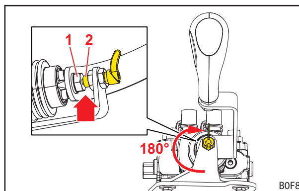
Abb. 69 Verriegelter Bedienhebel
