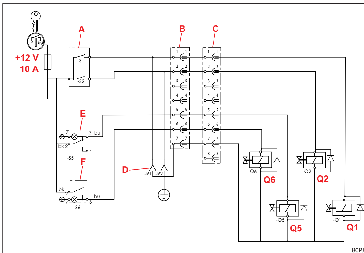
Abb. 134 Elektro-Schaltbild
