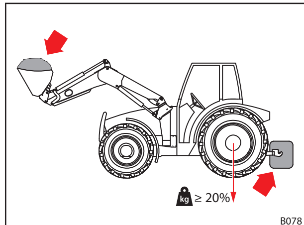
Abb. 48 Belastung bei Frontladerarbeiten
