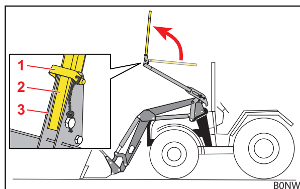
Abb. 43 Hochgeklappter oberer Bügel
