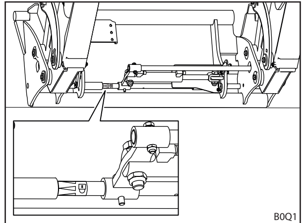
Abb. 93 Werkzeug-Verriegelung anhand des Aufklebers prüfen (Kombi-Wechselrahmen Euro-SMS)
