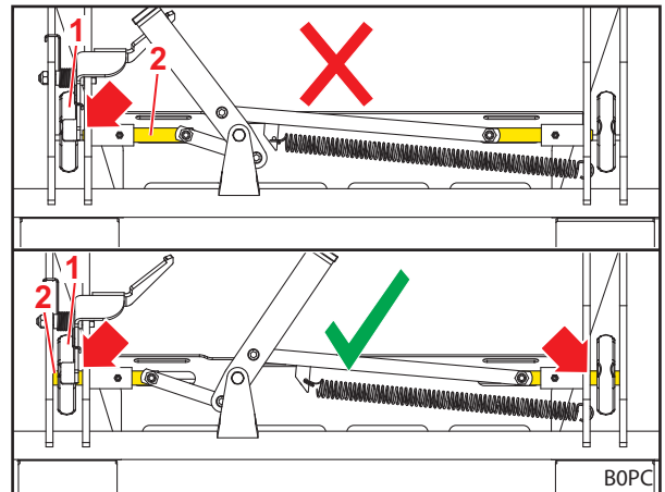
Abb. 84 Position der Verriegelungsbolzen prüfen
