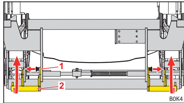
Abb. 99 Anlagen hochschwenken
