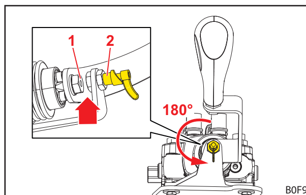
Abb. 70 Entriegelter Bedienhebel
