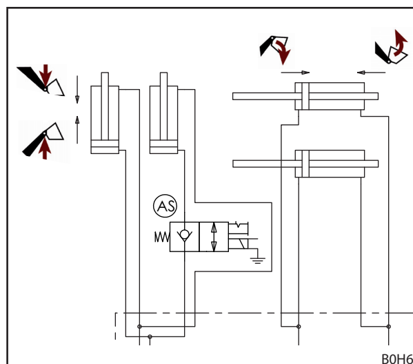
Abb. 133 Hydraulikplan Absenksicherung
