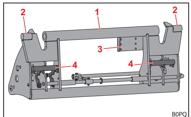
Abb. 16 Kombi-Wechselrahmen Euro-SMS (vorbereitet für SMS-Werkzeug)
