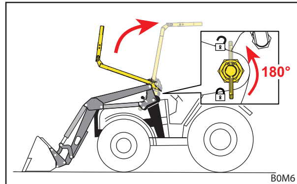
Abb. 37 OPG hochklappen
