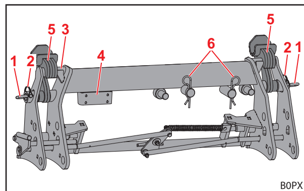
Abb. 18 Kombi-Wechselrahmen Euro-MX (vorbereitet für MX-Werkzeug)
