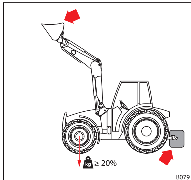
Abb. 49 Belastung bei Straßenfahrten
