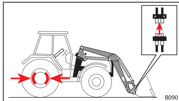
Abb. 113 Hydraulikleitungen lösen
