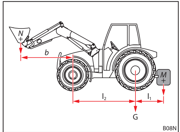
Abb. 50 Berechnung der statischen Standfestigkeit
