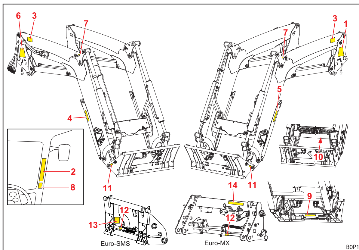
Abb. 4 Frontlader TL (beispielhafte Abbildung)
