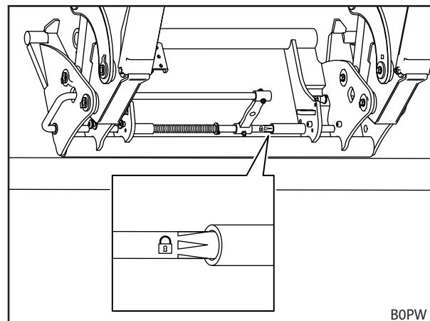
Abb. 87 Werkzeug-Verriegelung anhand des Aufklebers prüfen (Kombi-Wechselrahmen Euro-SMS)
