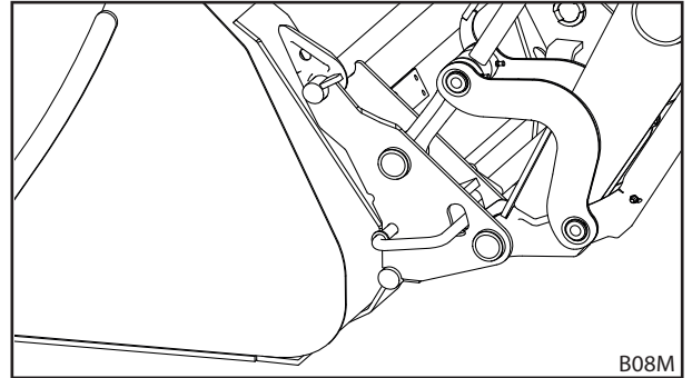
Abb. 104 Geöffnete Werkzeug-Verriegelung
