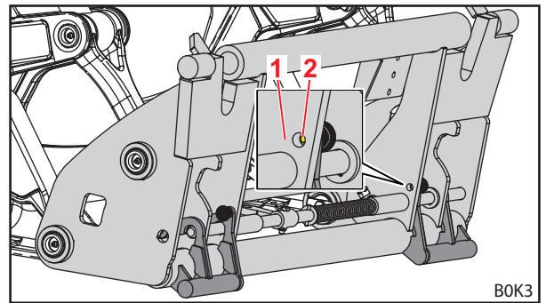
Abb. 98 Heruntergeschwenkte Anlagen
