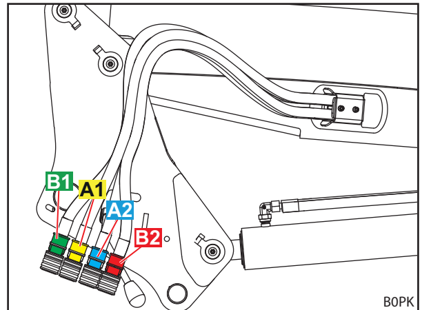
Abb. 19 Hydraulikleitungen
