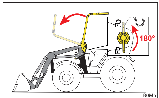
Abb. 35 OPG herunterklappen
