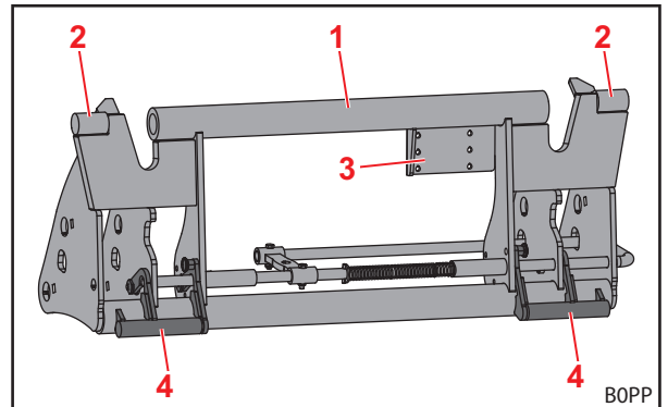
Abb. 15 Kombi-Wechselrahmen Euro-SMS (vorbereitet für Euro-Werkzeug)
