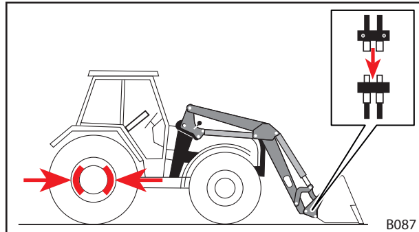
Abb. 109 Hydraulikleitungen des Werkzeuges mit Frontlader-Kupplungen verbinden
