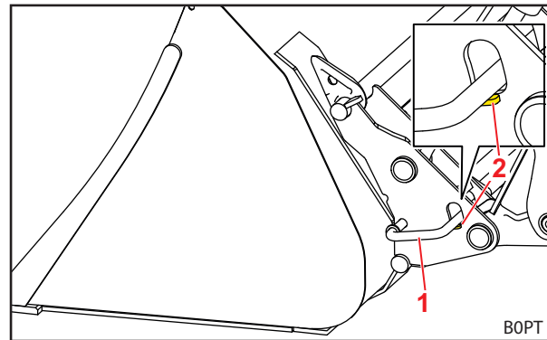
Abb. 86 Mechanische Werkzeug-Verriegelung
