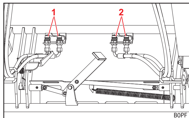
Abb. 45 Zusätzlicher 4. Steuerkreis
