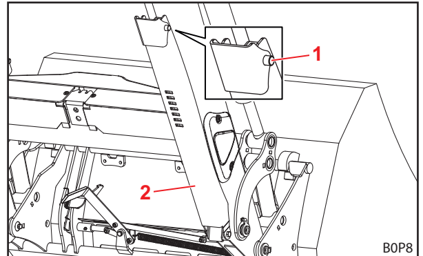
Abb. 76 Abstellstütze eingeklappt
