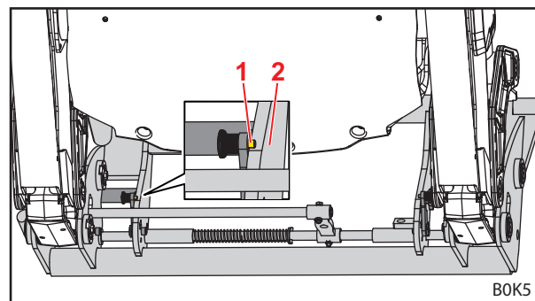
Abb. 100 Hochgeschwenkte Anlagen (Ansicht von hinten)
