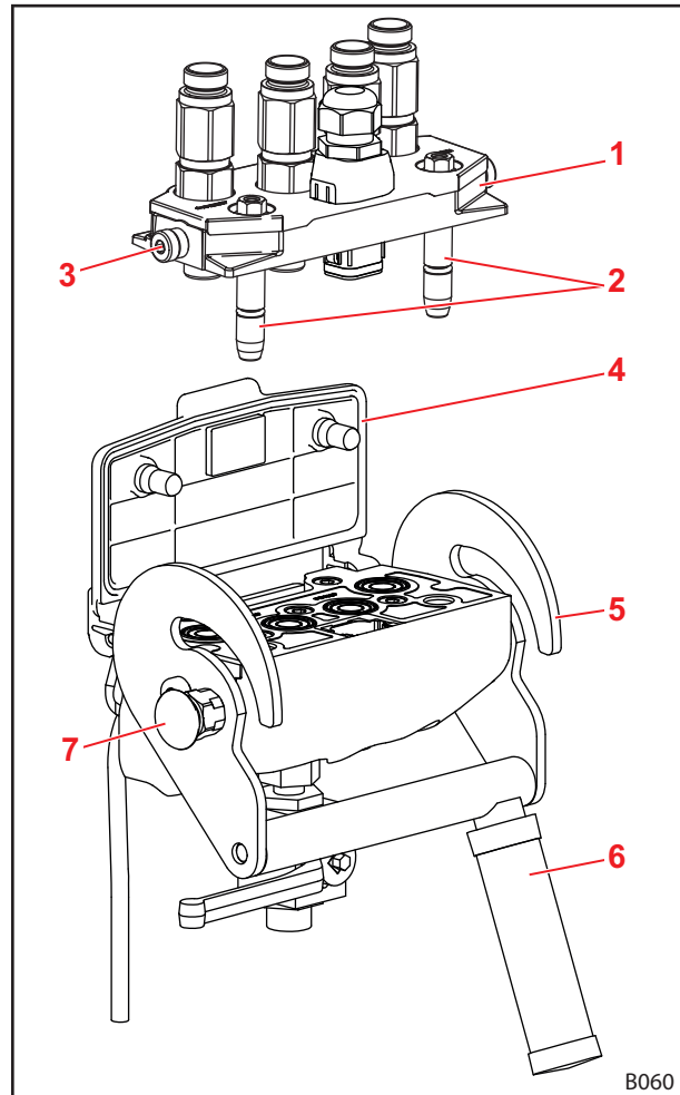
Abb. 80 Hydro-Fix (Beispiel: Hydro-Fix 4-fach)
