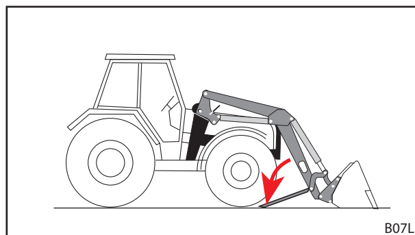
Abb. 128 Abstellstützen ausklappen
