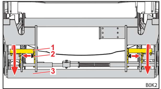
Abb. 97 Anlagen herunterschwenken
