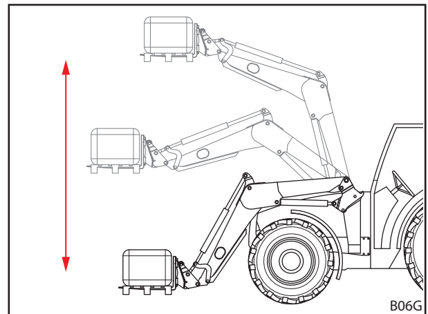
Abb. 33 Mechanische Parallelführung
