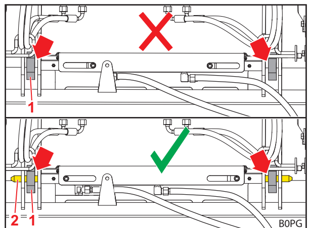
Abb. 95 Position der Verriegelungsbolzen prüfen (Beispiel: Euro-Wechselrahmen)
