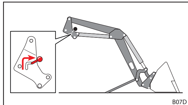
Abb. 51 Frontlader-Verriegelung öffnen
