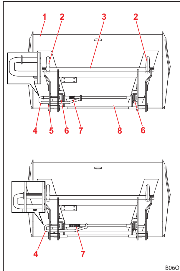
Abb. 26 Geöffnete (oben) und geschlossene (unten) Verriegelung (Beispieldarstellung)
