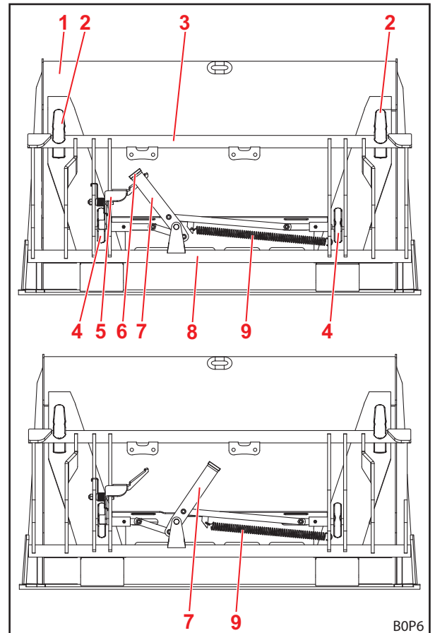
Abb. 25 Geöffnete (oben) und geschlossene (unten) Verriegelung
