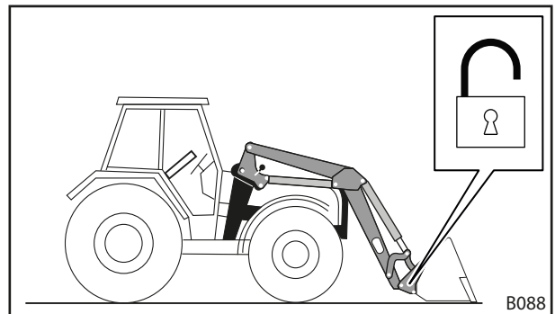
Abb. 98 Werkzeug-Verriegelung öffnen
