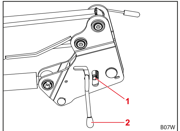
Abb. 118 Frontlader-Verriegelung prüfen
