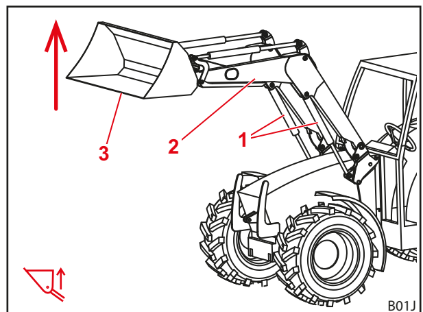
Abb. 27 Heben-Funktion
