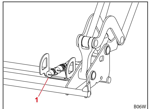
Abb. 37 Zusätzlicher 3. Steuerkreis
