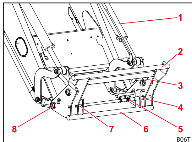
Abb. 10 Euro-Wechselrahmen
