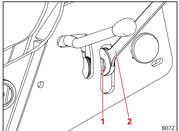
Abb. 58 Werkzeug anlegen
