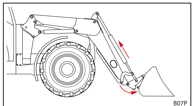
Abb. 100 Einhaken
