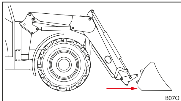
Abb. 102 Herantfahren
