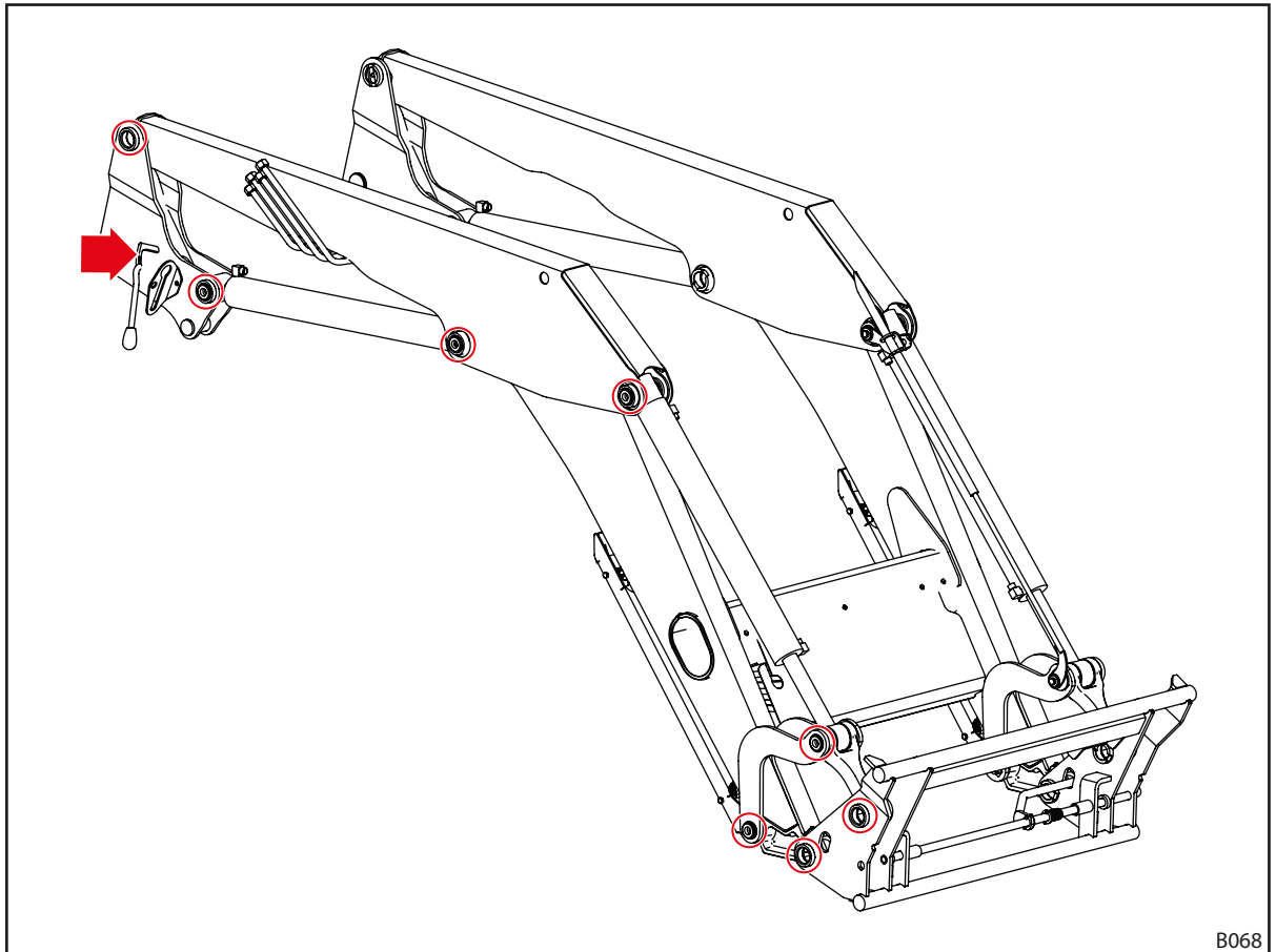
Abb. 114 Schmierstellen FS
