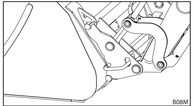
Abb. 92 Werkzeug-Verriegelung öffnen
