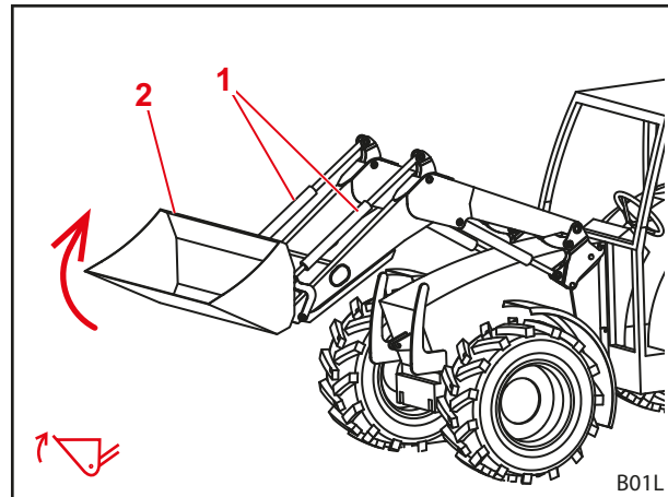
Abb. 29 Schöpfen-Funktion
