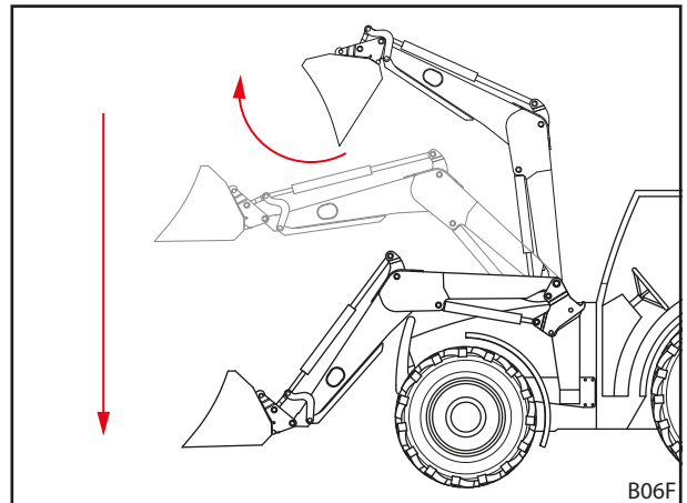
Abb. 35 Return-To-Level-Funktion
