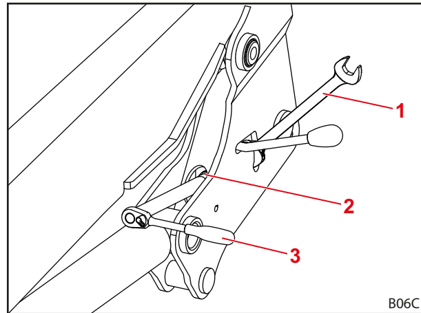
Abb. 54 Werkzeug anlegen
