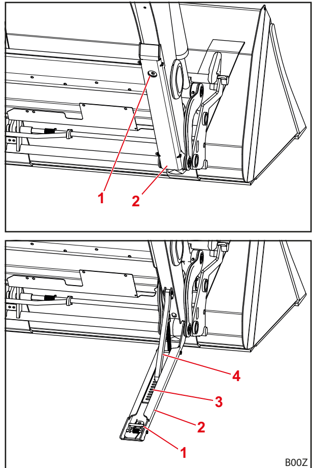
Abb. 74 Abstellstütze
