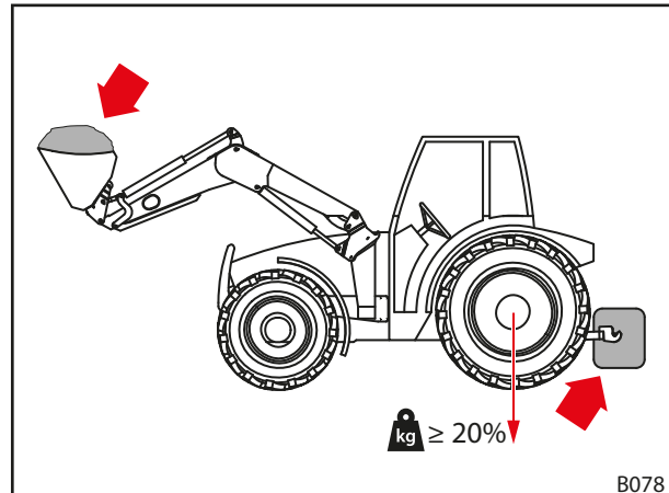
Abb. 44 Belastung bei Frontladerarbeiten
