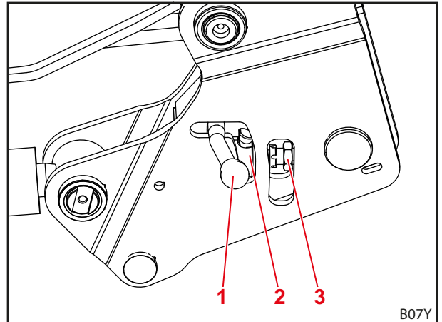
Abb. 63 Frontlader-Verriegelung öffnen
