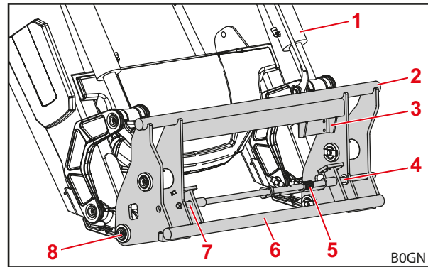
Abb. 10 Euro-Wechselrahmen
