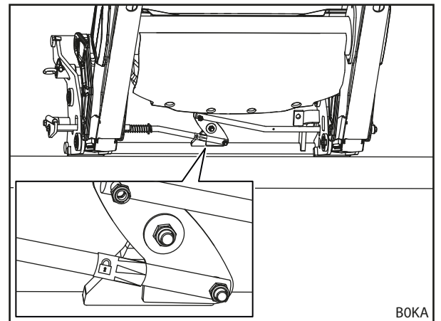
Abb. 79 Werkzeug-Verriegelung anhand des Aufklebers prüfen (Kombi-Wechselrahmen Euro-MX)
