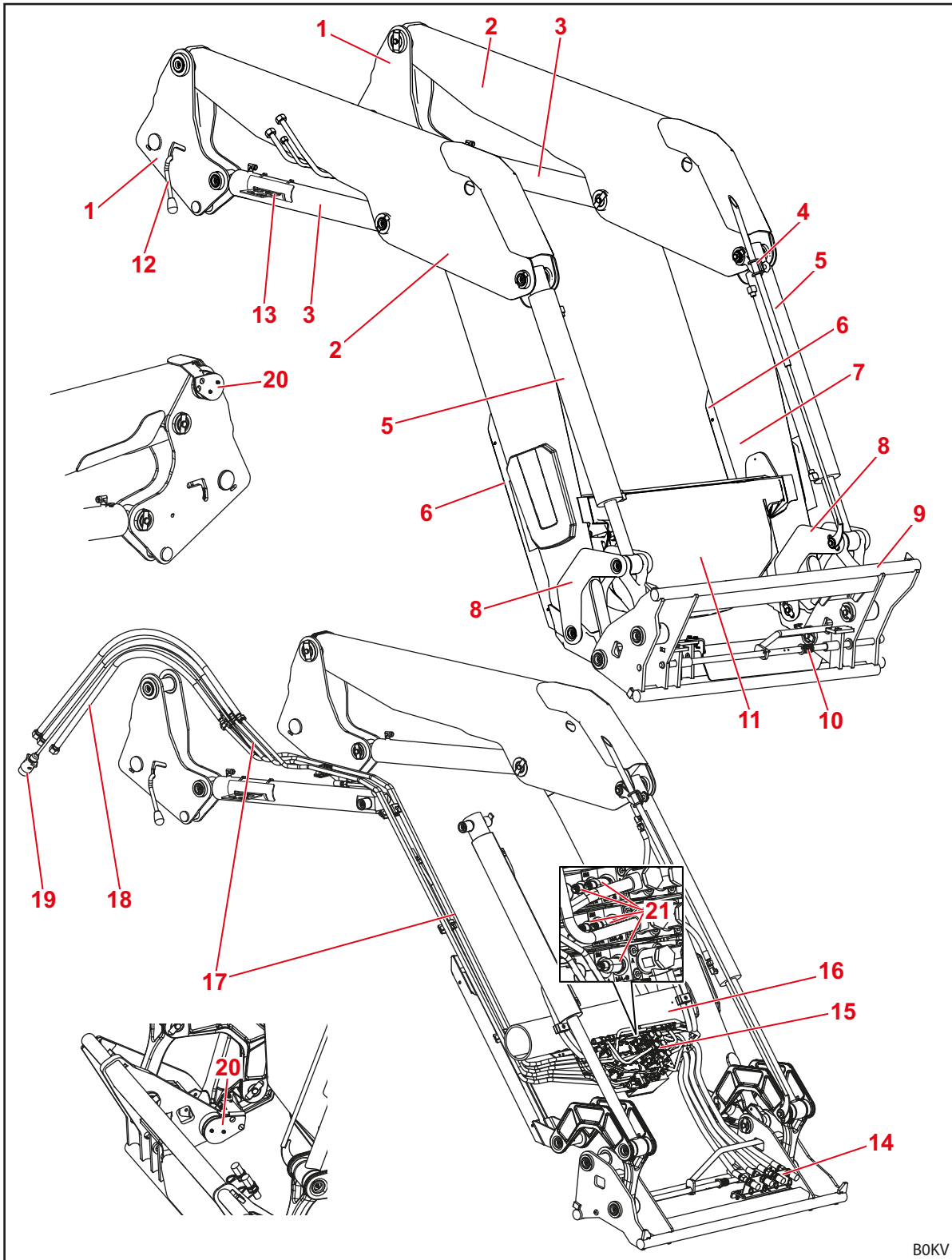
Abb. 7 Frontlader FS IB+
