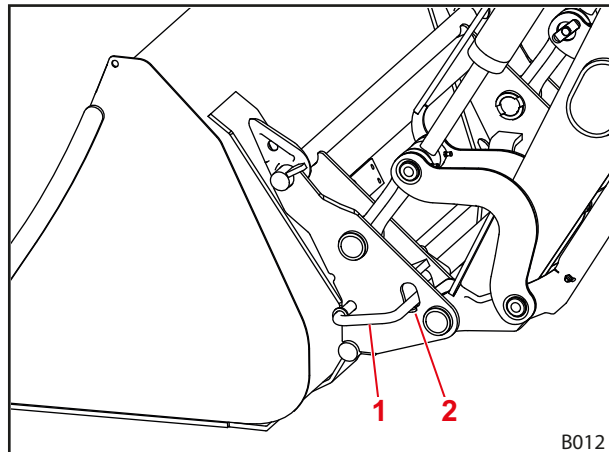
Abb. 77 Mechanische Werkzeug-Verriegelung
