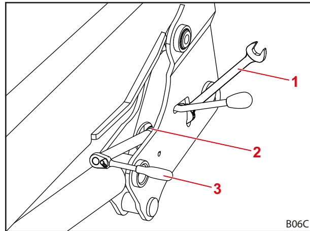
Abb. 60 Werkzeug anlegen
