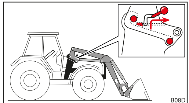
Abb. 121 Frontlader-Verriegelung lösen
