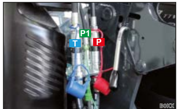
Abb. 18 Verbundene Steckkupplungen
