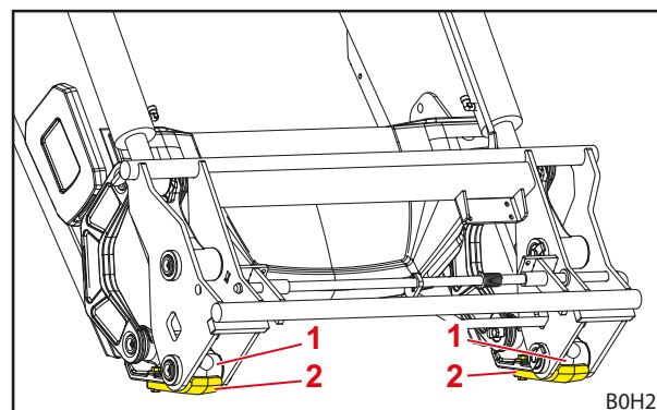
Abb. 16 Verschleißkufen
