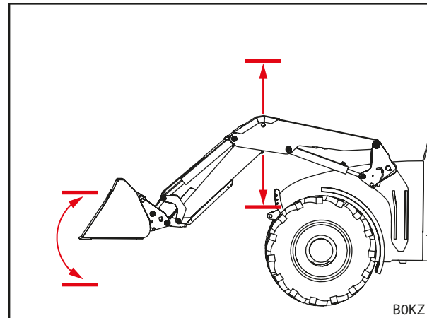
Abb. 36 Arbeitsbereiche
