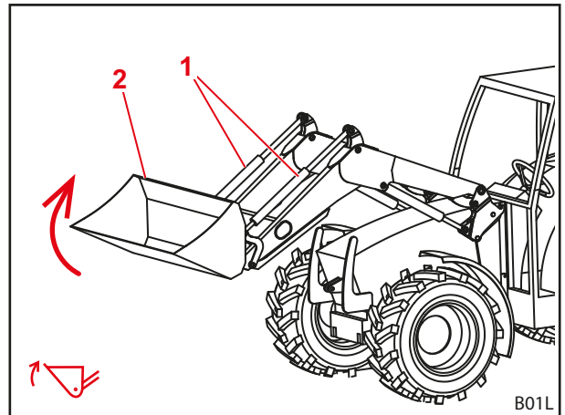
Abb. 26 Schöpfen-Funktion
