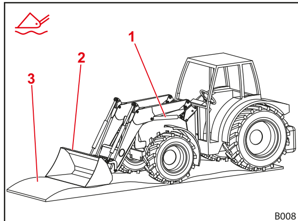
Abb. 40 Frontlader in Schwimmstellung
