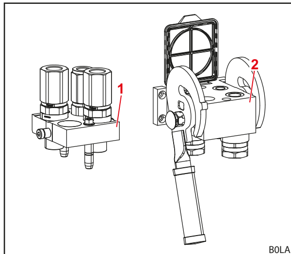
Abb. 20 Aufbau Hydro-Fix
