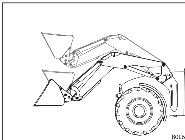
Abb. 39 Bewegungszyklus
