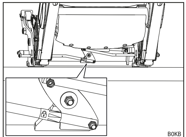
Abb. 84 Werkzeug-Verriegelung anhand des Aufklebers prüfen
