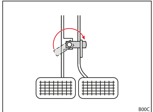
Abb. 49 Bremspedale koppeln
