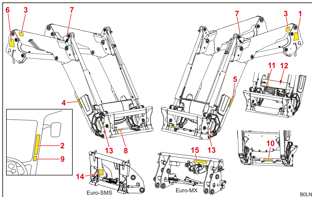
Abb. 4 Frontlader FZ IB+ (beispielhafte Abbildung)
