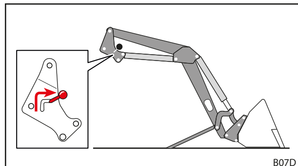
Abb. 53 Frontlader-Verriegelung öffnen
