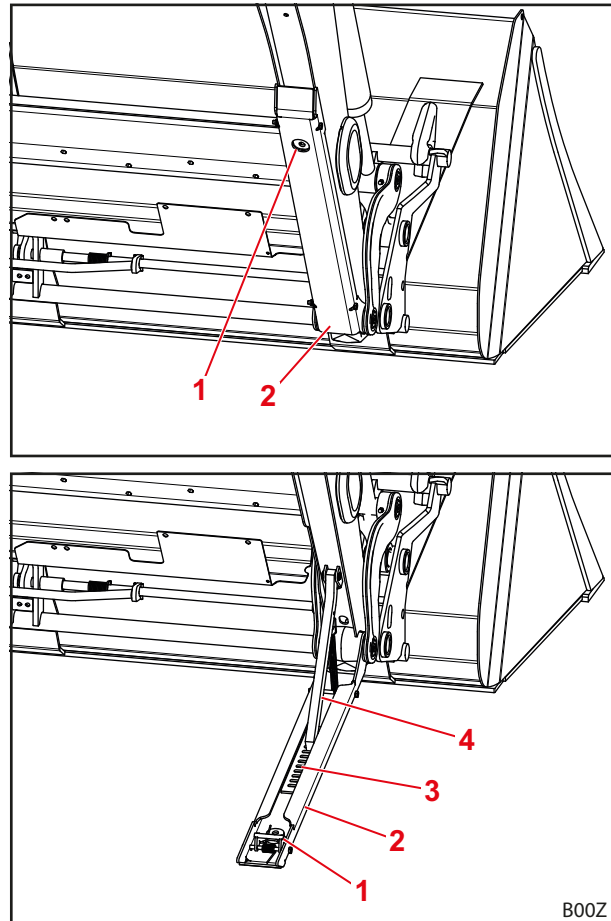
Abb. 71 Abstellstütze
