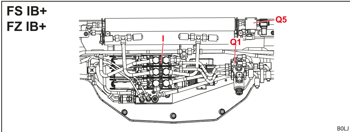
Abb. 128 Anordnung der Hydraulikventile für Zusatzfunktionen
