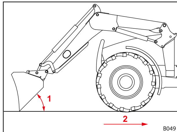
Abb. 105 Rückwärts planieren
