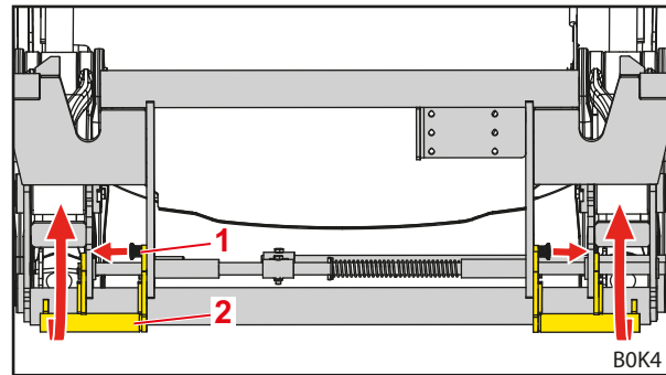
Abb. 89 Anlagen hochschwenken
