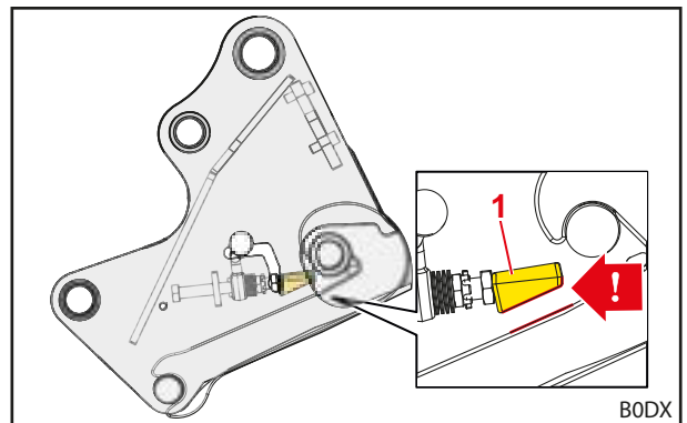
Abb. 58 Korrekte Einbauposition des Klemmkeils
