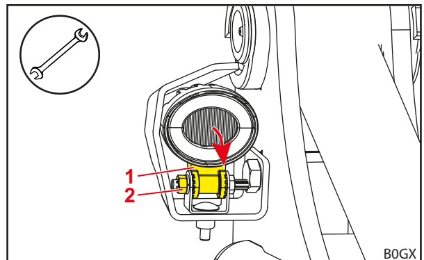
Abb. 48 Scheinwerfer vertikal einstellen
