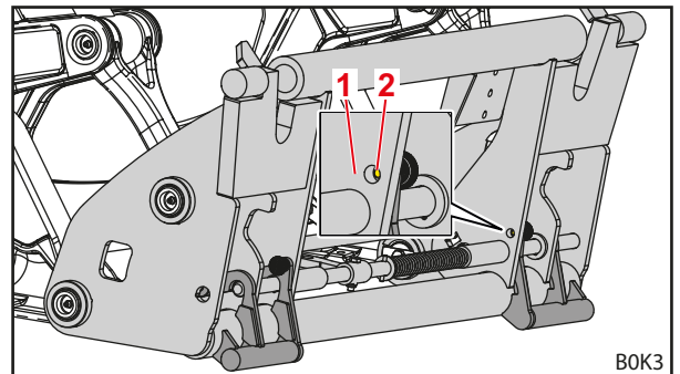
Abb. 88 Heruntergeschwenkte Anlagen
