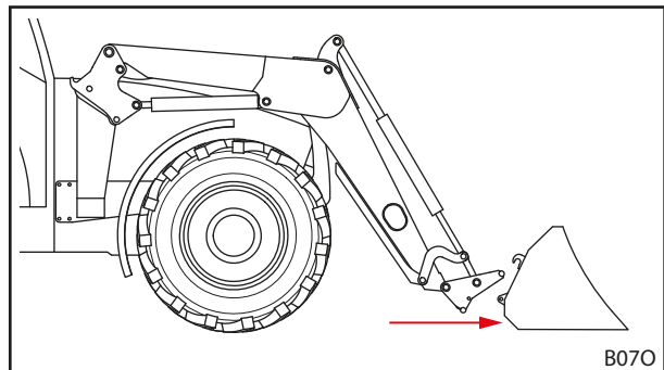
Abb. 95 Herantfahren
