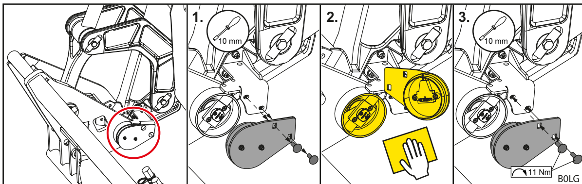
Abb. 111 Drehwinkelsensor reinigen
