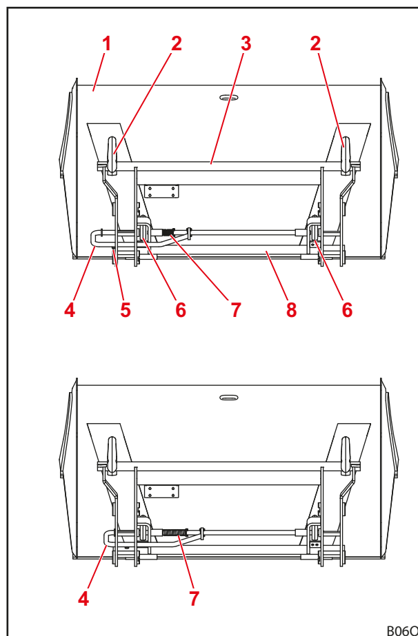
Abb. 23 Geöffnete (oben) und geschlossene (unten) Verriegelung
