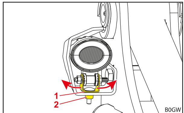
Abb. 47 Scheinwerfer horizontal einstellen
