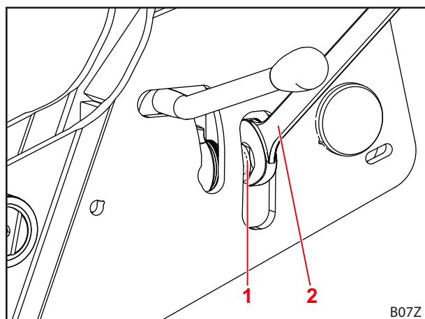
Abb. 67 Kontermutter anziehen
