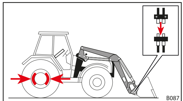
Abb. 98 Hydraulikleitungen des Werkzeuges mit Frontlader-Kupplungen verbinden
