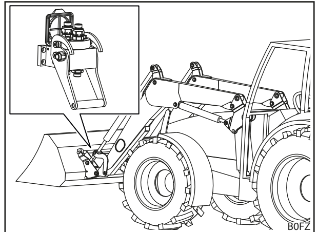
Abb. 21 Werkzeug-Fix: Position am Frontlader
