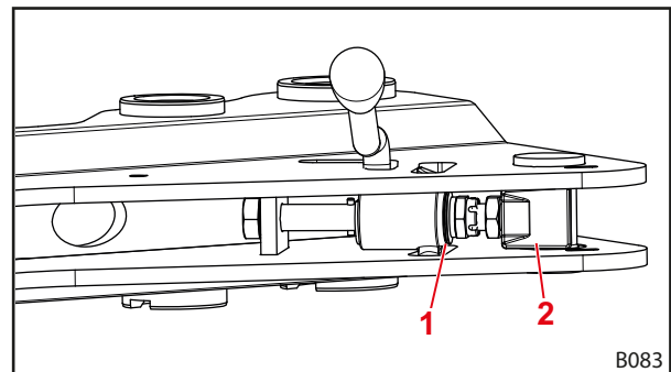
Abb. 66 Ansicht der Frontlader-Verriegelung von unten
