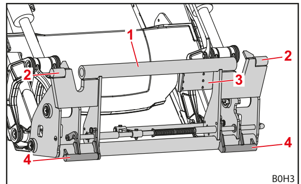
Abb. 11 Kombi-Wechselrahmen Euro-SMS (vorbereitet für Euro-Werkzeug)
