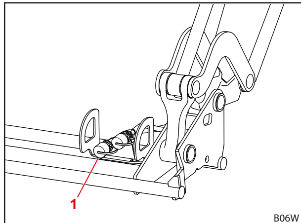
Abb. 43 Zusätzlicher 3. Steuerkreis
