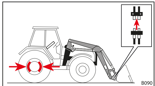
Abb. 102 Hydraulikleitungen lösen
