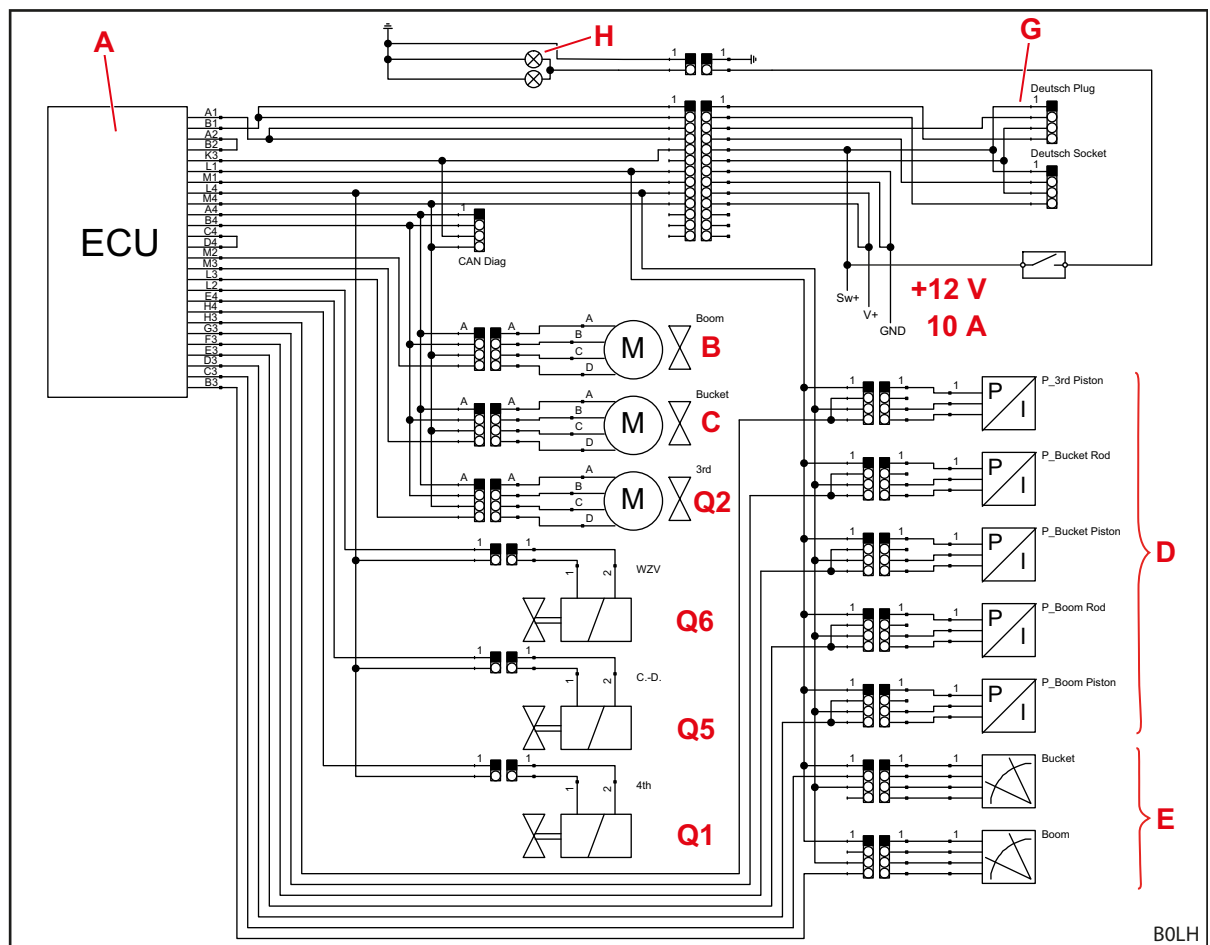
Abb. 127 Elektro-Schaltbild
