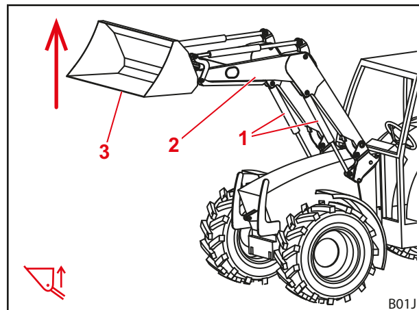
Abb. 24 Heben-Funktion
