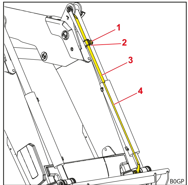
Abb. 41 Sichtanzeige für Werkzeugstellung
