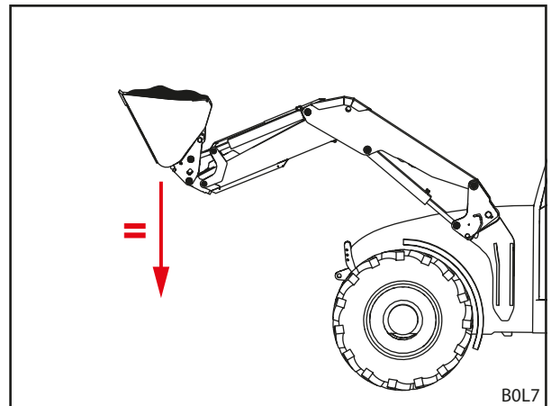
Abb. 30 Lastunabhängige Absenkgeschwindigkeit
