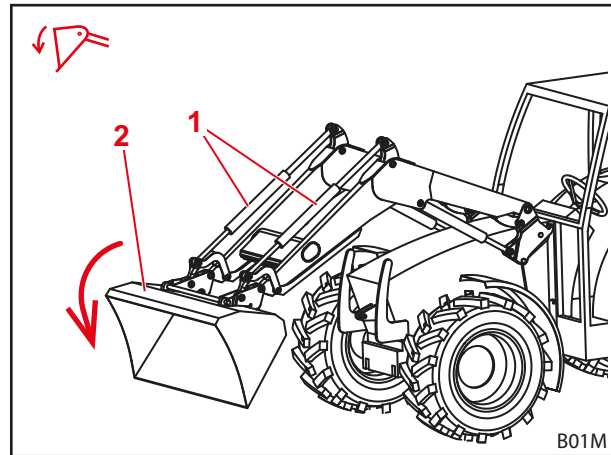
Abb. 27 Schütten-Funktion
