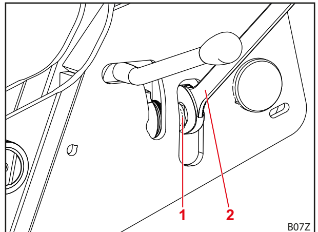
Abb. 64 Werkzeug anlegen
