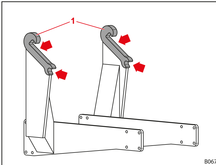
Abb. 112 Schmierstellen Frontlader-Aufnahmen
