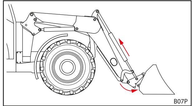
Abb. 96 Einhaken
