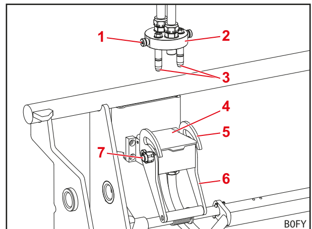
Abb. 75 Abgekuppeltes Werkzeug-Fix
