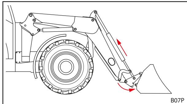
Abb. 100 Einhaken
