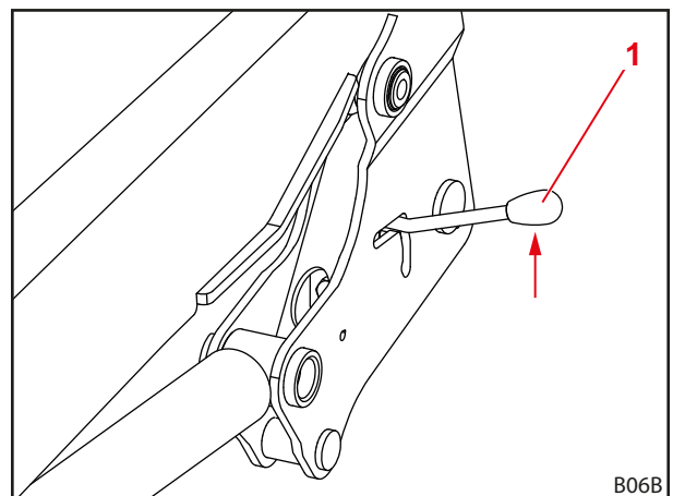
Abb. 116 Frontlader-Verriegelung prüfen
