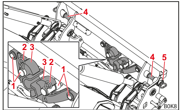
Abb. 91 Adapter in Parkposition (Wechselrahmen vorbereitet für Euro-Werkzeug)
