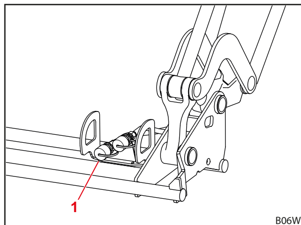
Abb. 45 REAL 3
