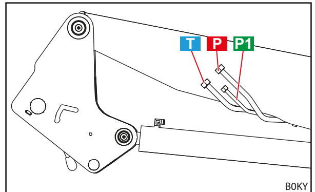
Abb. 17 Hydraulikleitungen
