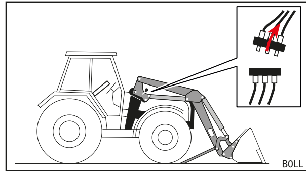
Abb. 123 Hydraulik abkoppeln
