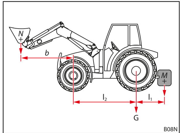
Abb. 52 Berechnung der statischen Standfestigkeit
