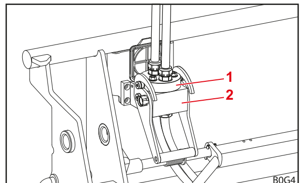
Abb. 76 Angekuppeltes Werkzeug-Fix
