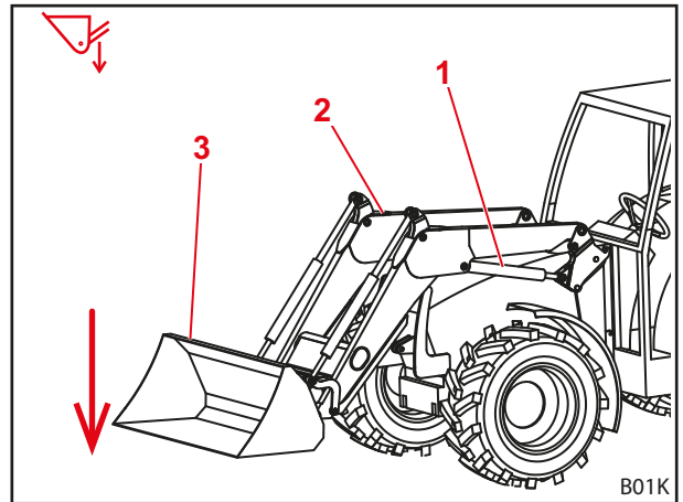
Abb. 25 Senken-Funktion
