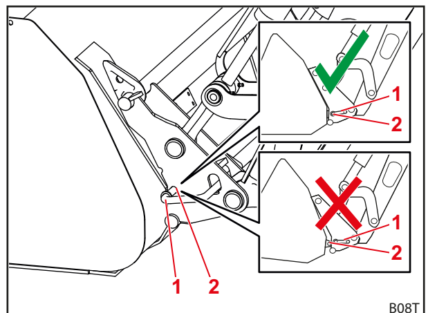
Abb. 80 Position der Verriegelungsbolzen prüfen
