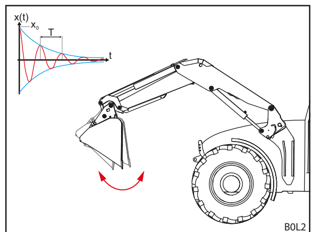
Abb. 35 Schaufel schütteln
