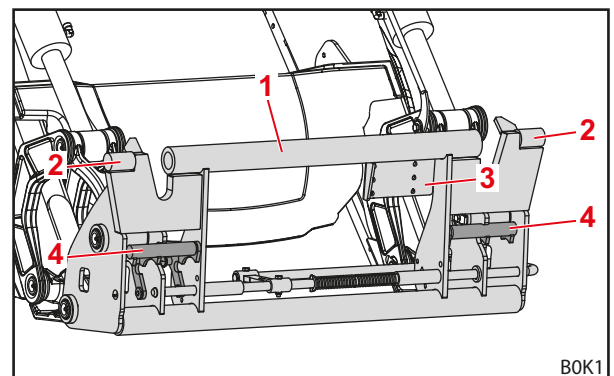
Abb. 12 Kombi-Wechselrahmen Euro-SMS (vorbereitet für SMS-Werkzeug)
