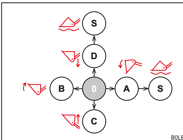
Abb. 68 Belegung des Bedienhebels
