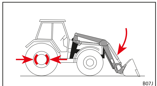
Abb. 120 Feststellbremse anziehen und Frontlader absenken
