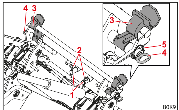
Abb. 92 Adapter in Arbeitsposition (Wechselrahmen vorbereitet für MX-Werkzeug)
