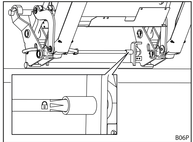
Abb. 78 Werkzeug-Verriegelung anhand des Aufklebers prüfen
