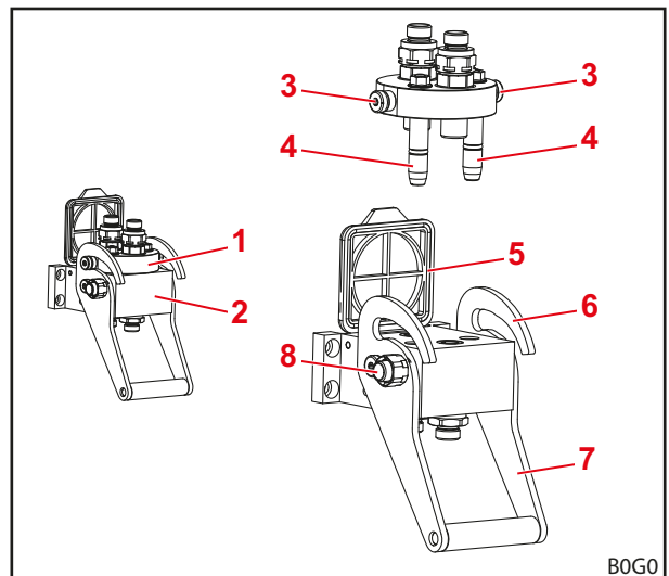
Abb. 22 Aufbau Werkzeug-Fix
