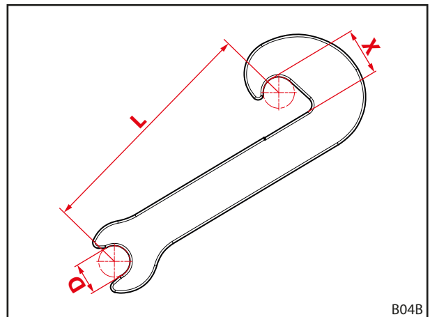
Abb. 115 Verschleißmaße des Fanghakens
