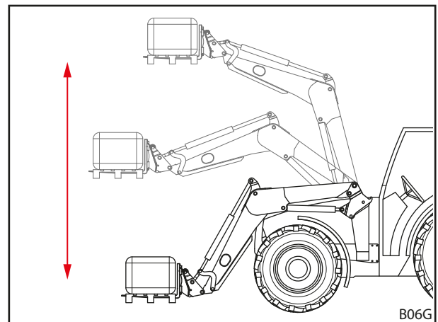
Abb. 42 Mechanische Parallelführung
