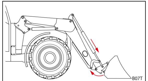
Abb. 103 Wechselrahmen aushaken
