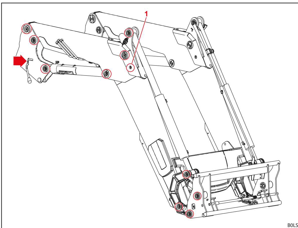
Abb. 114 Schmierstellen FZ IB+
