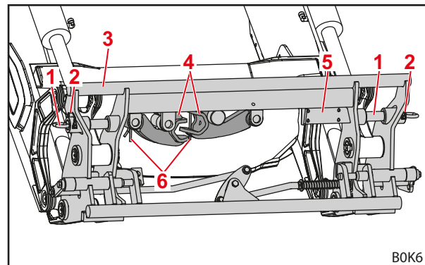
Abb. 14 Kombi-Wechselrahmen Euro-MX (vorbereitet für Euro-Werkzeug)
