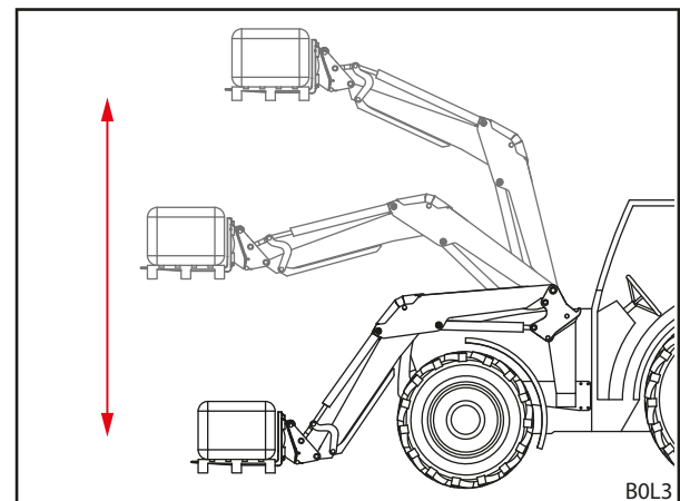
Abb. 28 Elektronische Parallelführung
