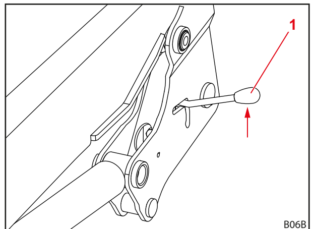
Abb. 59 Frontlader-Verriegelung öffnen
