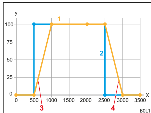
Abb. 32 Einstellbares Ansprechverhalten
