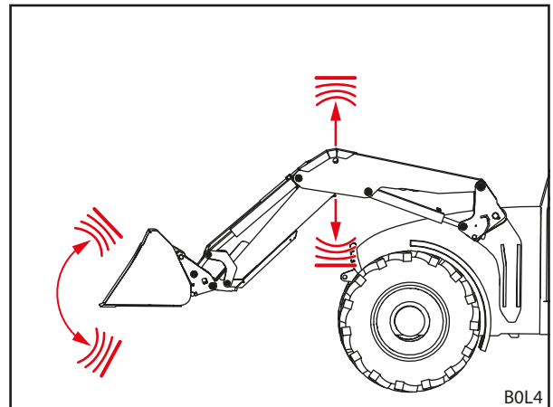
Abb. 34 Endlagendämpfung
