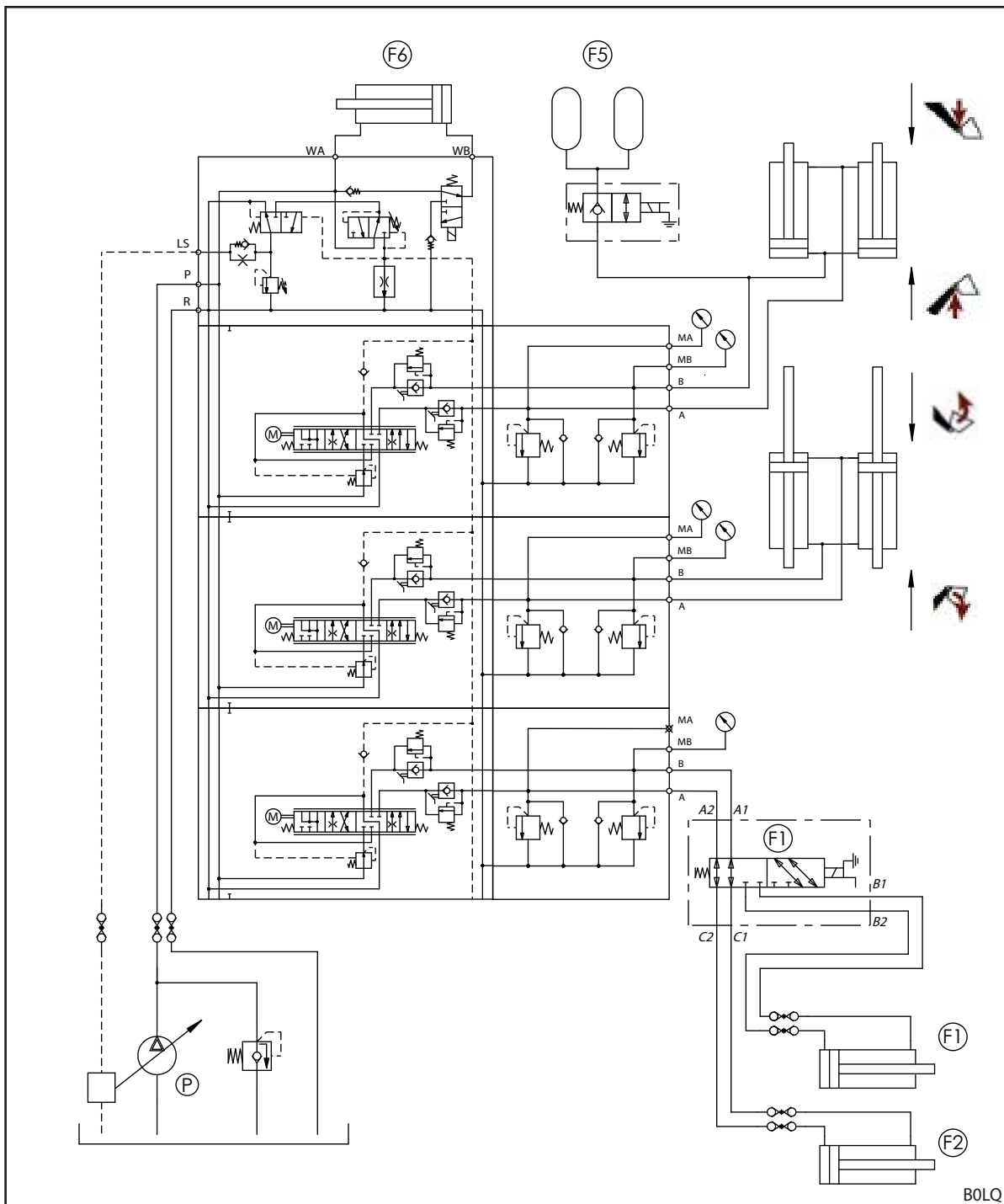
Abb. 126 Hydraulikplan FS IB+ und FZ IB+
