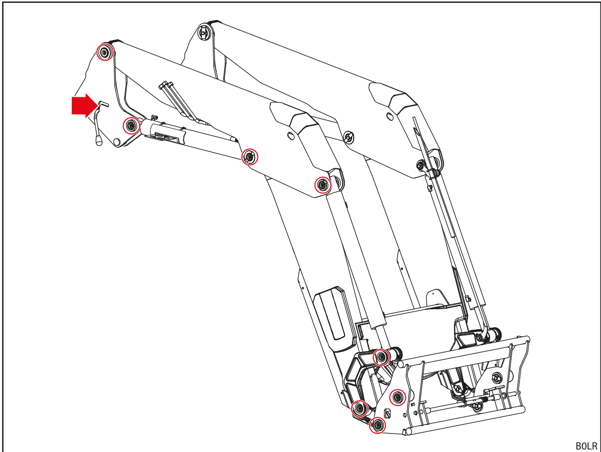
Abb. 113 Schmierstellen FS IB+
