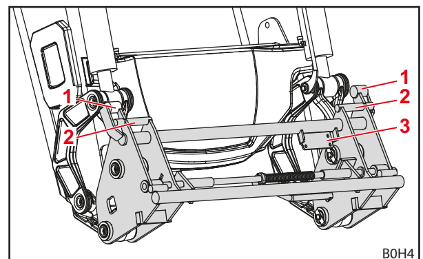
Abb. 13 Kombi-Wechselrahmen Euro-Alö3
