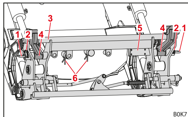
Abb. 15 Kombi-Wechselrahmen Euro-MX (vorbereitet für MX-Werkzeug)
