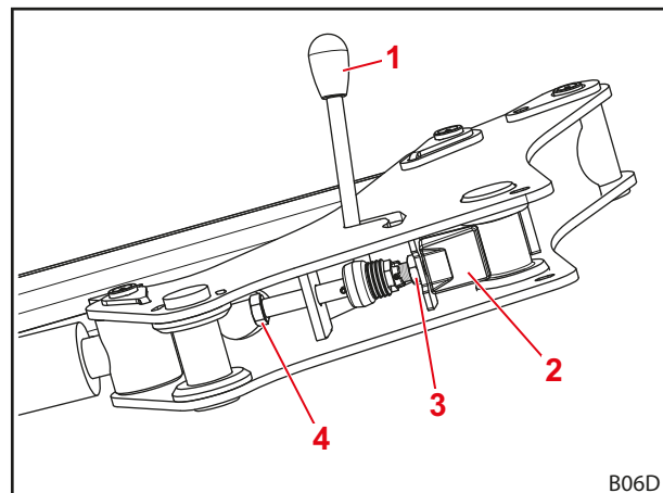
Abb. 62 Ansicht der Frontlader-Verriegelung von unten
