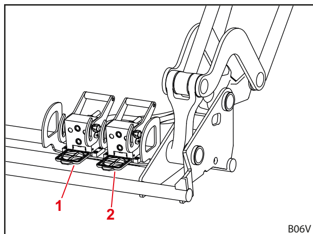
Abb. 44 Zusätzlicher 4. Steuerkreis
