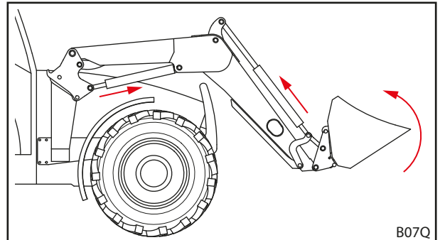
Abb. 97 Werkzeug-Verriegelung auslösen
