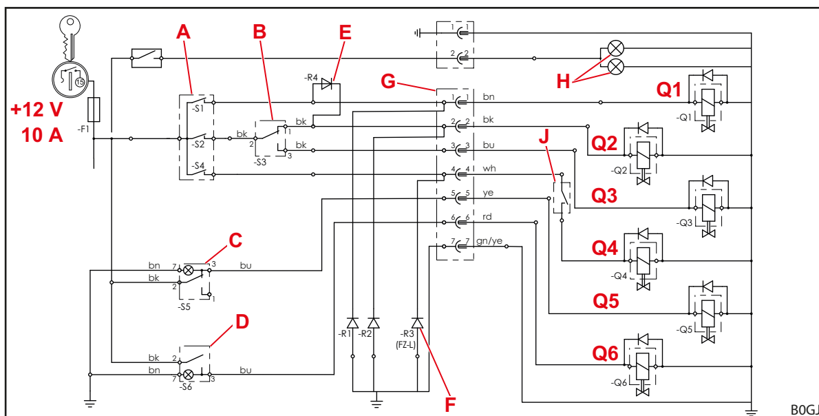
Abb. 149 Elektro-Schaltbild (bei Ausstattung mit 3. und 4. Steuerkreis)
