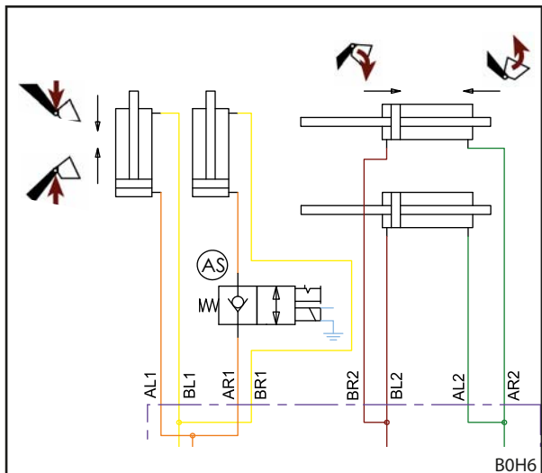
Abb. 147 Hydraulikplan Absenksicherung
