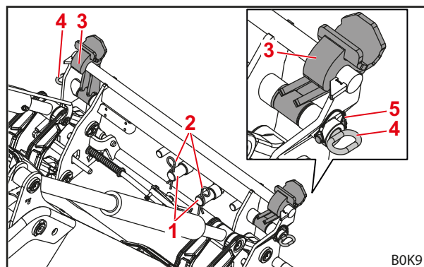
Abb. 106 Adapter in Arbeitsposition (Wechselrahmen vorbereitet für MX-Werkzeug)
