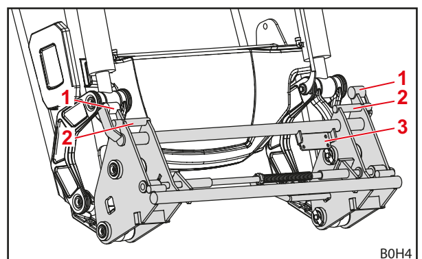
Abb. 13 Kombi-Wechselrahmen Euro-Alö3
