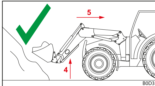
Abb. 128 Rückwärtsfahren unter Last – richtig
