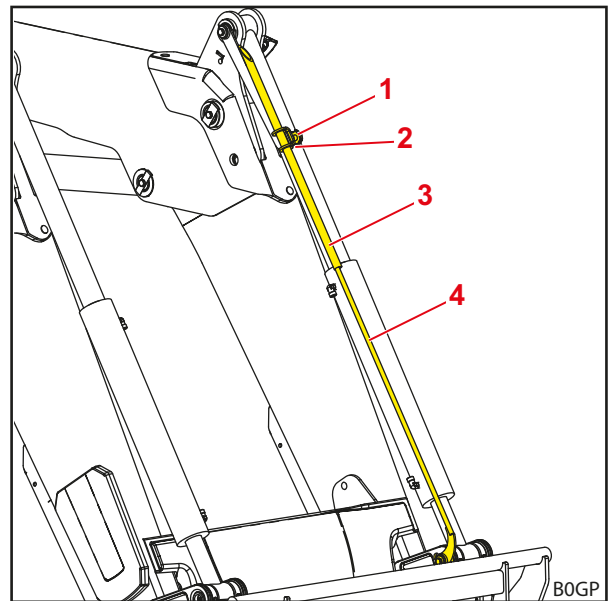
Abb. 33 Sichtanzeige für Werkzeugstellung
