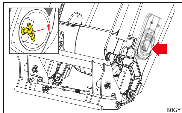
Abb. 41 Mechanisch betätigter Comfort-Drive
