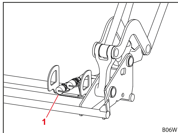
Abb. 38 Zusätzlicher 3. Steuerkreis
