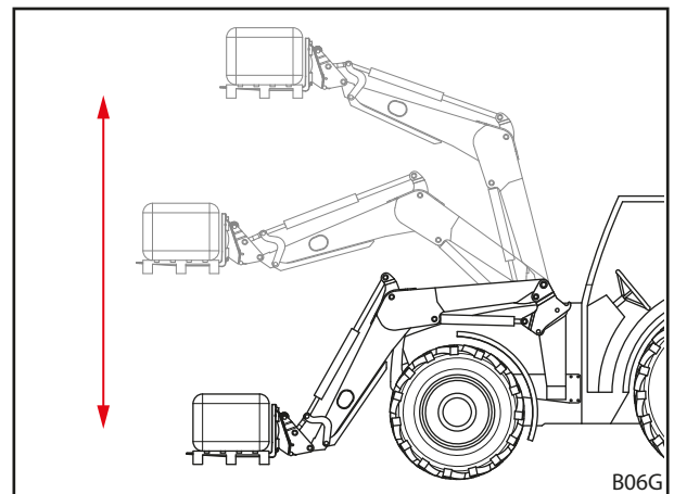
Abb. 34 Parallelführung
