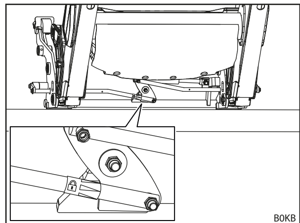
Abb. 98 Werkzeug-Verriegelung anhand des Aufklebers prüfen
