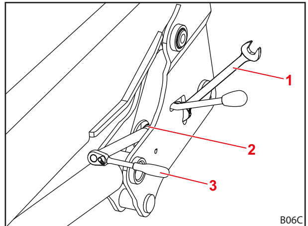
Abb. 60 Werkzeug anlegen
