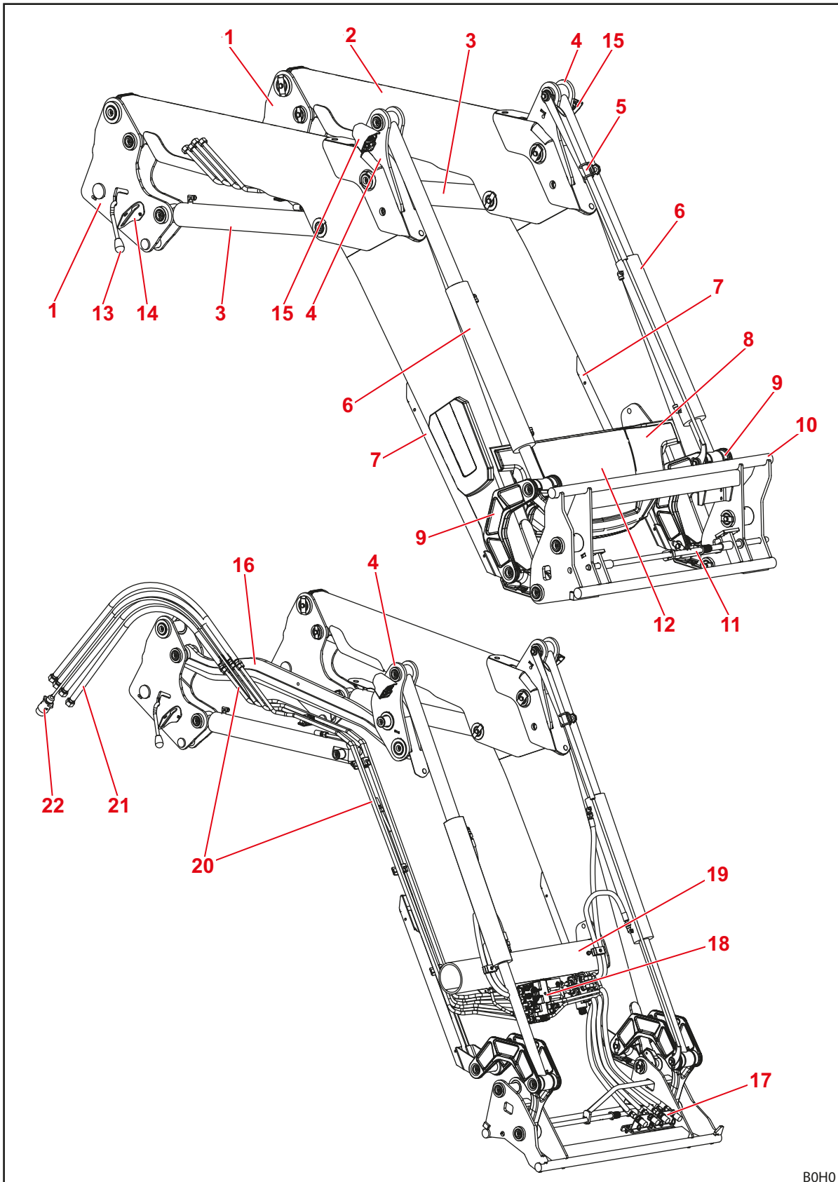
Abb. 8 Frontlader FZ
