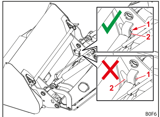
Abb. 99 Position der Verriegelungsbolzen prüfen
