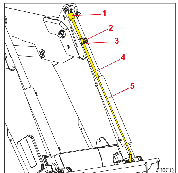
Abb. 37 Return-To-Level-Sensor an der Sichtanzeige
