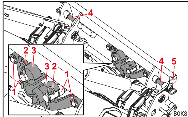
Abb. 105 Adapter in Parkposition (Wechselrahmen vorbereitet für Euro-Werkzeug)
