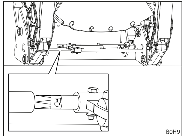
Abb. 97 Werkzeug-Verriegelung anhand des Aufklebers prüfen
