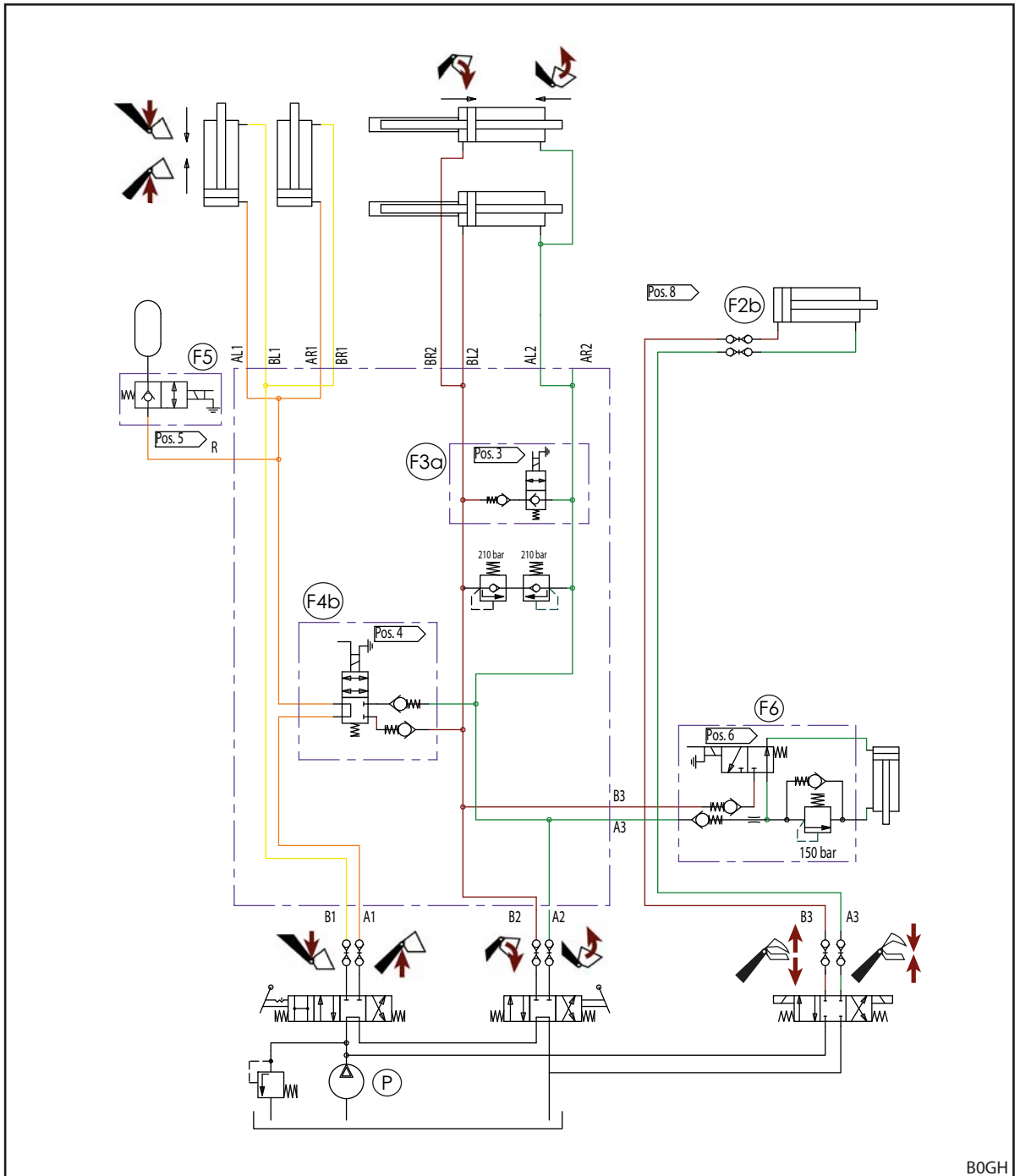
Abb. 146 Hydraulikplan FZ und FZ-L (bei Ausstattung mit REAL 3 )
