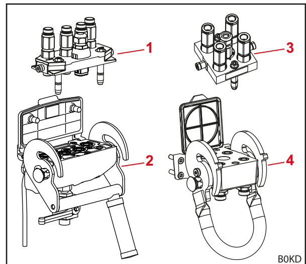
Abb. 23 Aufbau Hydro-Fix und Multikuppler
