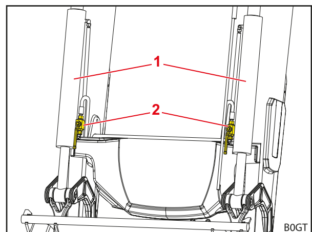
Abb. 45 Absperrhähne an den Werkzeug-Zylindern
