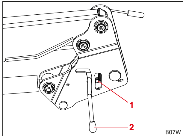
Abb. 134 Frontlader-Verriegelung prüfen
