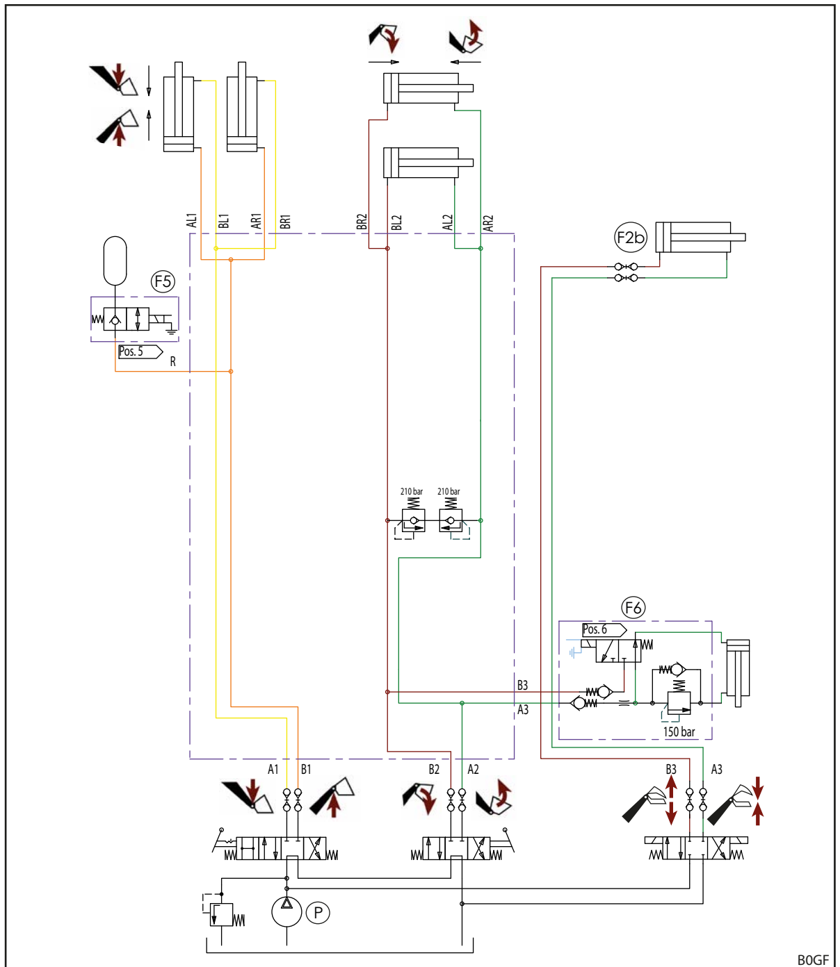
Abb. 144 Hydraulikplan FS (bei Ausstattung mit REAL 3 )
