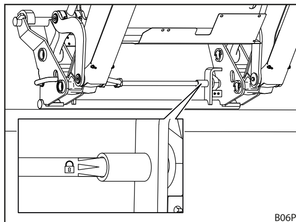
Abb. 89 Werkzeug-Verriegelung anhand des Aufklebers prüfen
