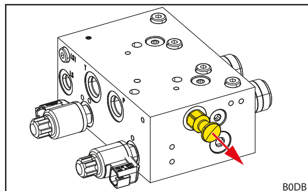
Abb. 80 Druckentlastungsventil am REAL 3 -Ventil herausziehen
