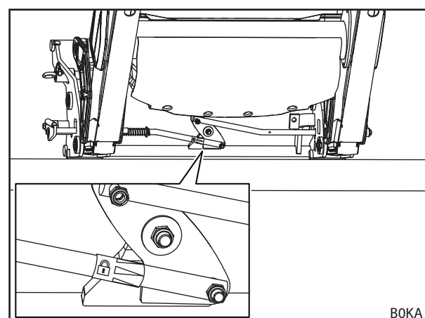
Abb. 90 Werkzeug-Verriegelung anhand des Aufklebers prüfen (Kombi-Wechselrahmen Euro-MX)
