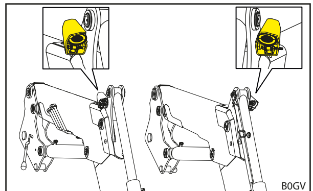
Abb. 46 Scheinwerfer
