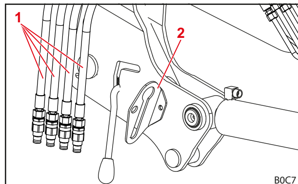
Abb. 142 Hydraulikleitungen in Kupplungshalter einhängen (Darstellung mit Steckkupplungen)
