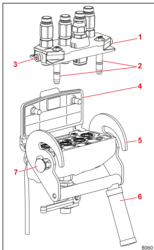
Abb. 85 Hydro-Fix (Beispiel: Hydro-Fix 4-fach)
