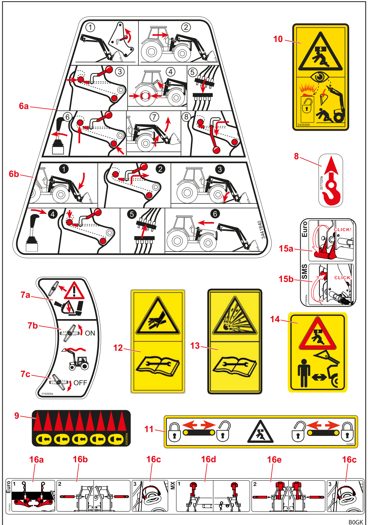
Abb. 6 Sicherheitsaufkleber Position 6-16
