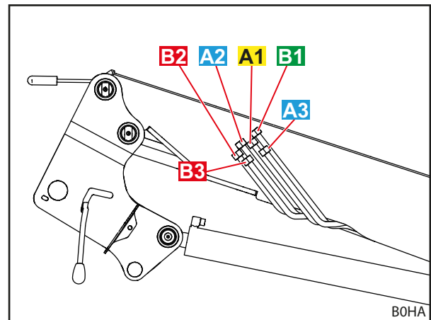
Abb. 19 Hydraulikleitungen (Option REAL 3 )
