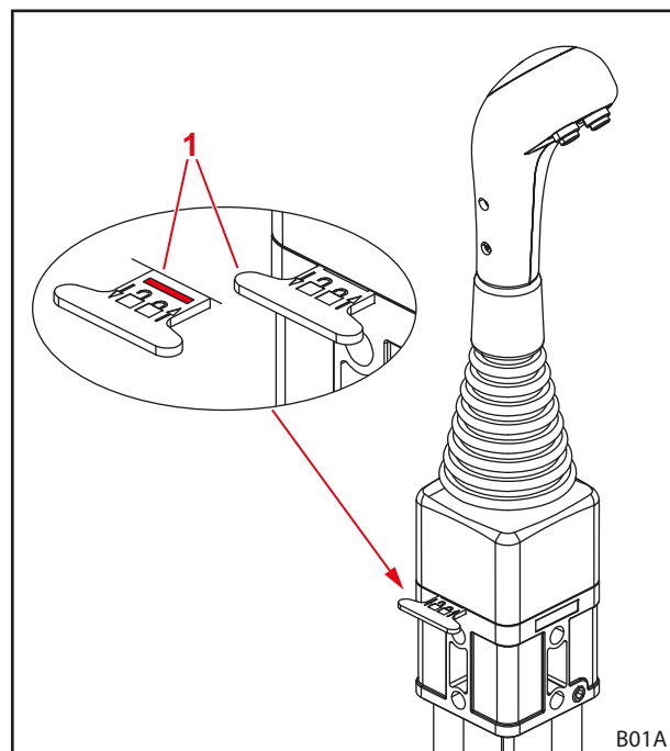
Abb. 71 Verriegelung des Bedienhebels (horizontale Verriegelung)
