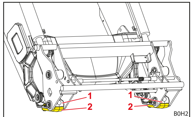
Abb. 17 Verschleißkufen
