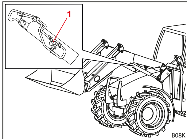
Abb. 44 Absenkdrossel
