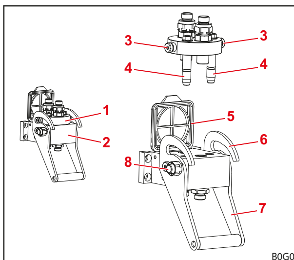
Abb. 25 Aufbau Werkzeug-Fix
