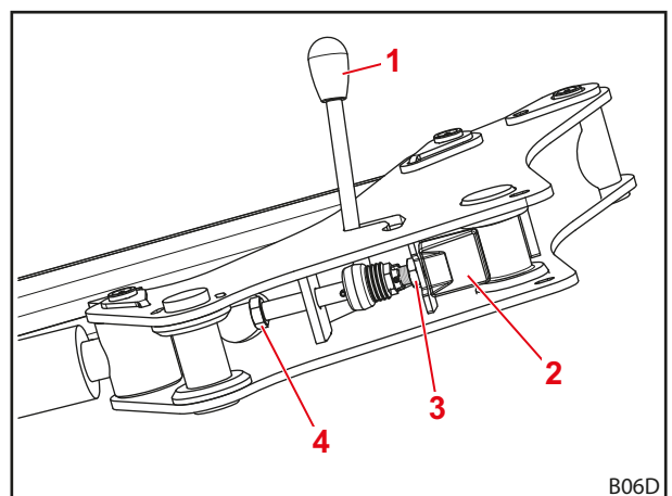
Abb. 62 Ansicht der Frontlader-Verriegelung von unten
