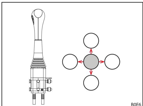
Abb. 73 Bedienhebel in alle Endlagen bewegen
