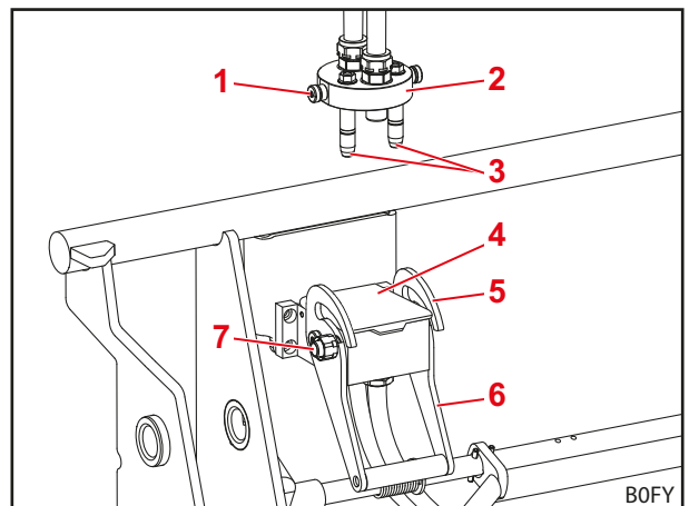
Abb. 86 Abgekuppeltes Werkzeug-Fix
