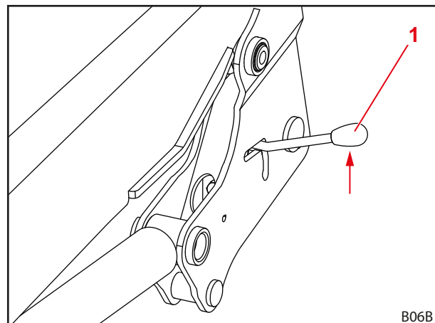
Abb. 59 Frontlader-Verriegelung öffnen
