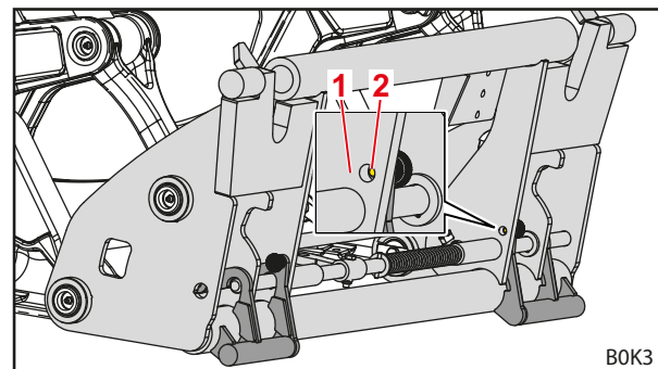
Abb. 102 Heruntergeschwenkte Anlagen
