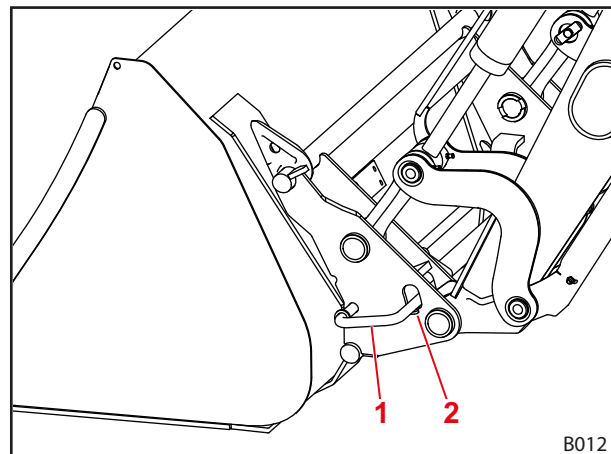
Abb. 88 Mechanische Werkzeug-Verriegelung
