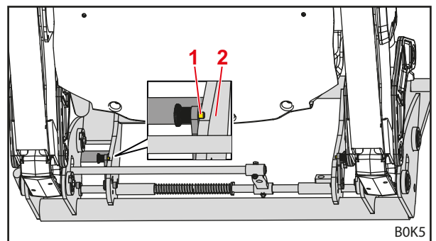
Abb. 104 Hochgeschwenkte Anlagen (Ansicht von hinten)
