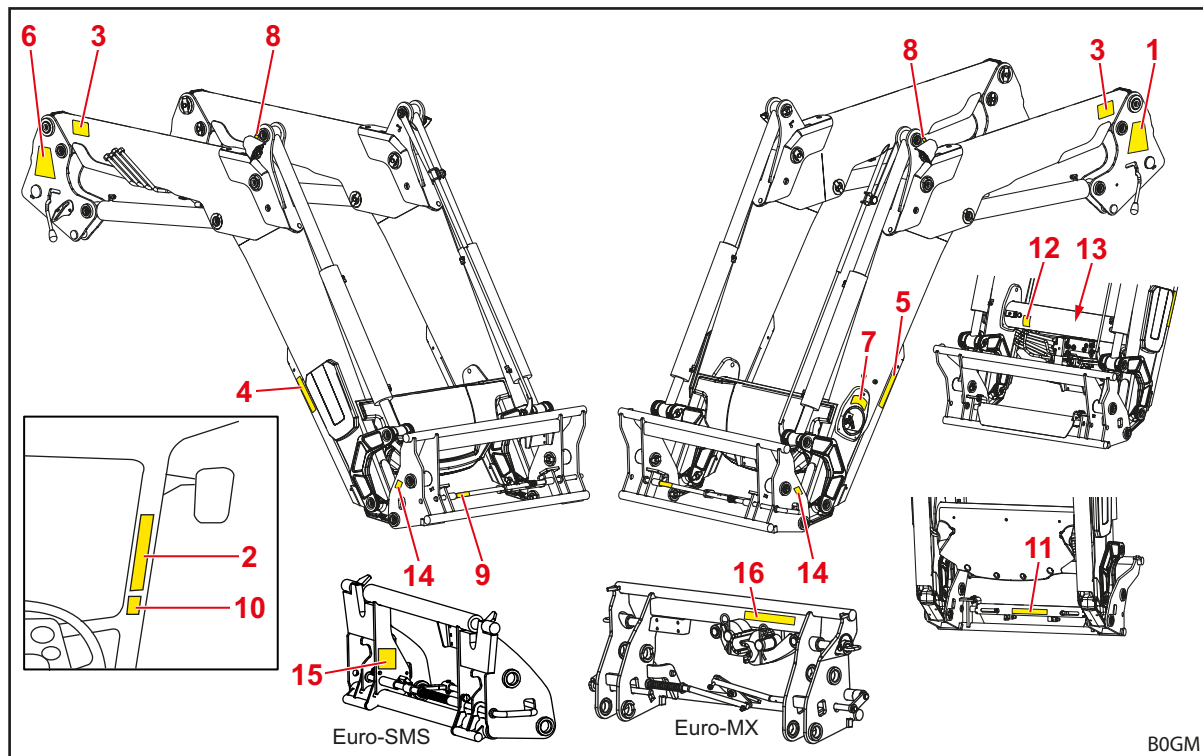
Abb. 4 Frontlader FZ (beispielhafte Abbildung)
