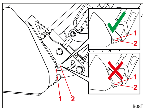
Abb. 91 Position der Verriegelungsbolzen prüfen
