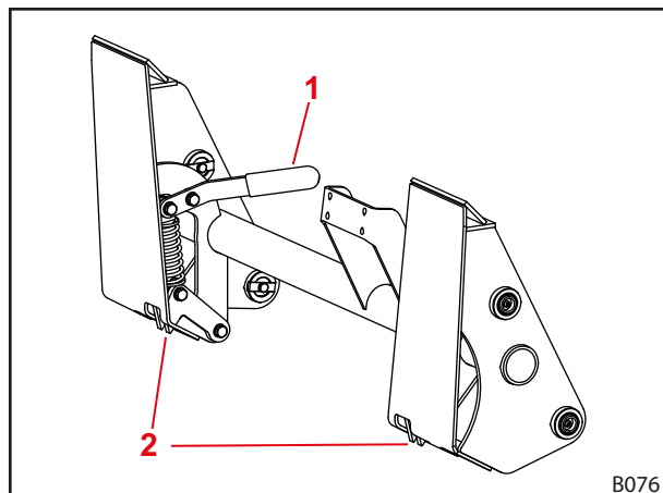
Abb. 93 Werkzeug-Verriegelung am Skid-Steer-Wechselrahmen
