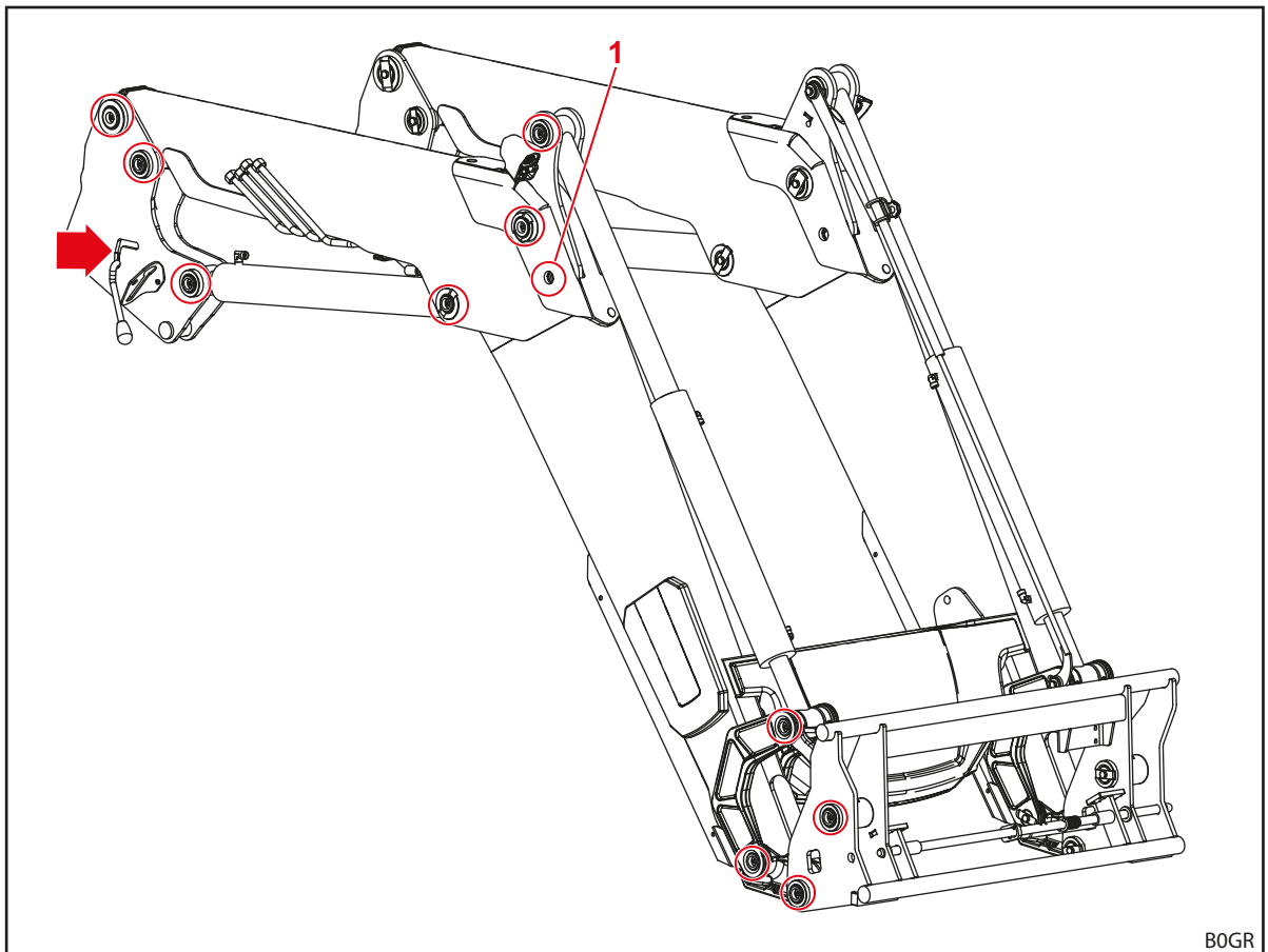
Abb. 131 Schmierstellen FZ
