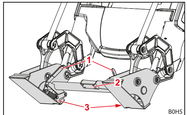
Abb. 16 Skid-Steer-Wechselrahmen
