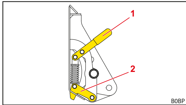
Abb. 59 Mechanische Werkzeug-Verriegelung Skid-Steer (halb geschlossener Zustand)
