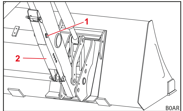
Abb. 51 Abstellstütze eingeklappt
