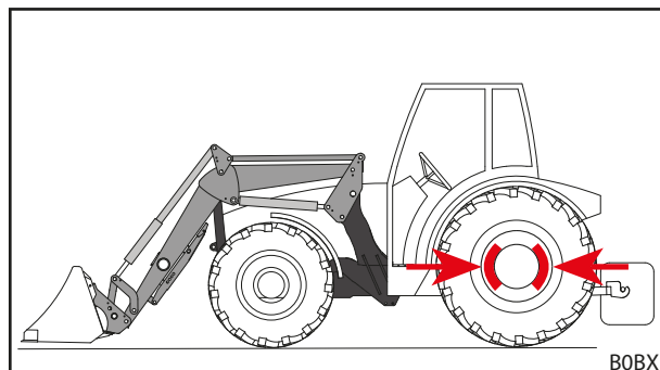
Abb. 87 Werkzeug zum Ablegen positionieren und Feststellbremse anziehen
