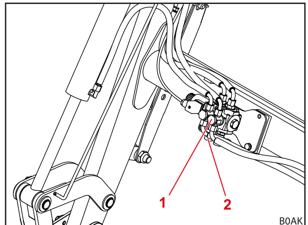
Abb. 30 Zusätzlicher 3. Steuerkreis
