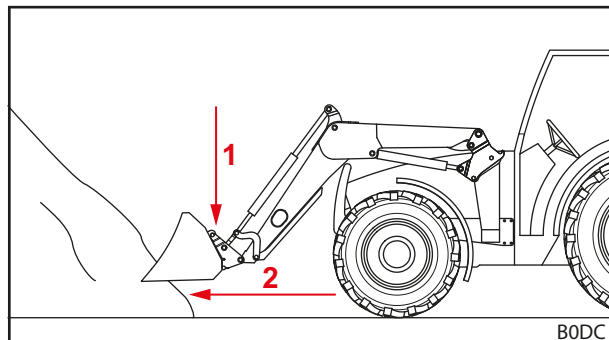
Abb. 93 Frontlader absenken und gerade in Ladegut einfahren
