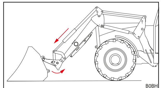
Abb. 85 Wechselrahmen aushaken
