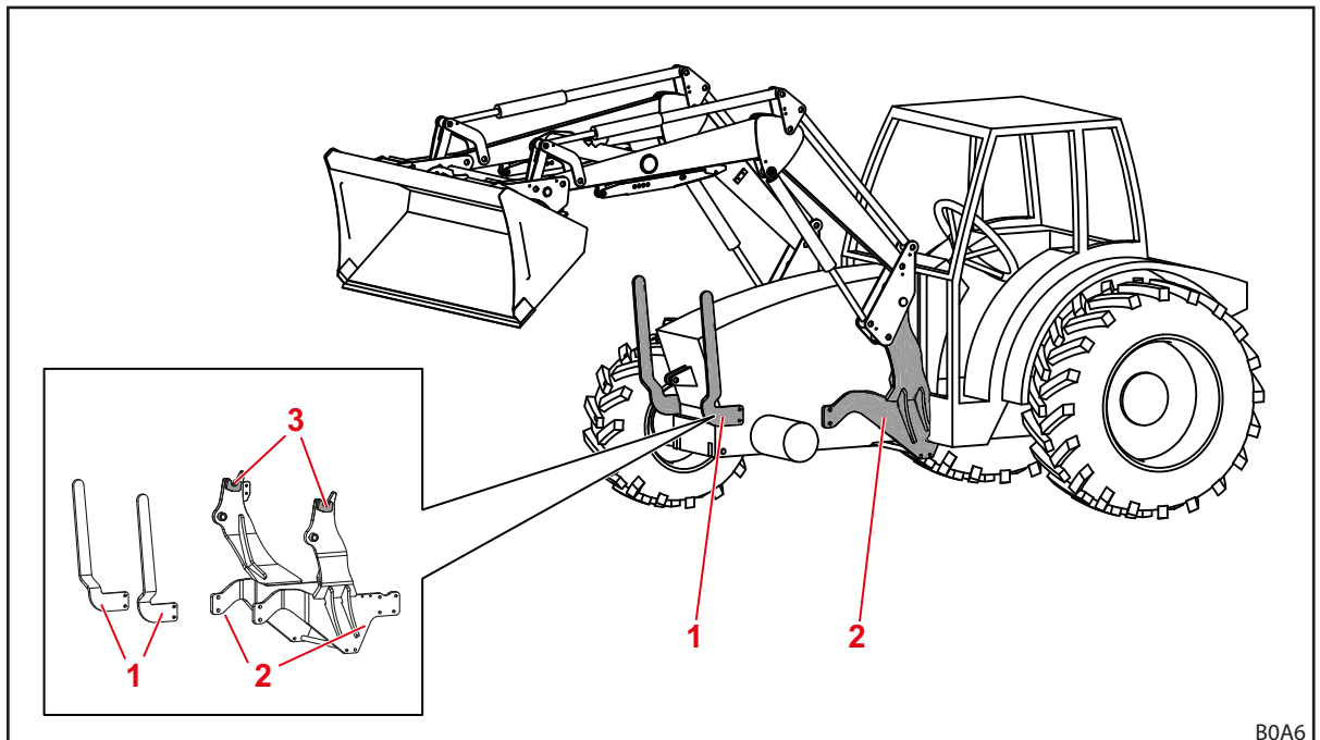
Abb. 10 Anbausatz für Traktor
