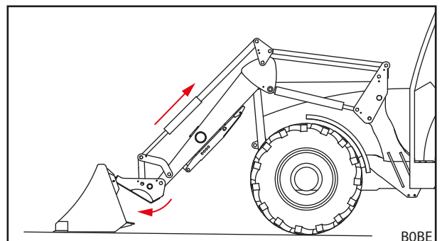
Abb. 70 Einhängen
