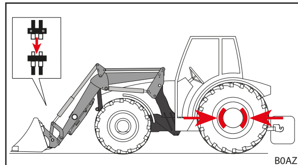
Abb. 72 Steuerkreis ankuppeln
