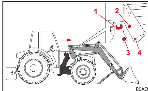
Abb. 38 Traktor in Schwinge einfahren
