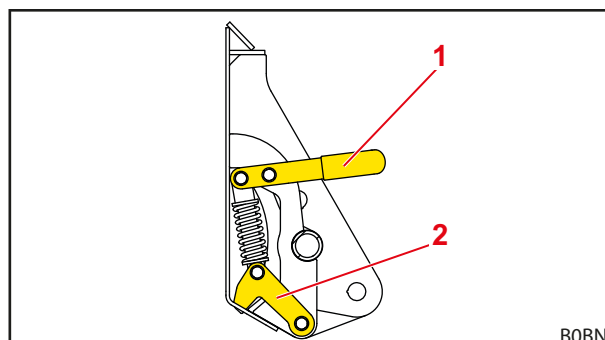
Abb. 58 Mechanische Werkzeug-Verriegelung Skid-Steer (geöffneter Zustand)
