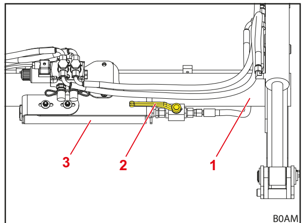
Abb. 32 Mechanisch betätigter Comfort-Drive (Hebelstellung Comfort-Drive an)
