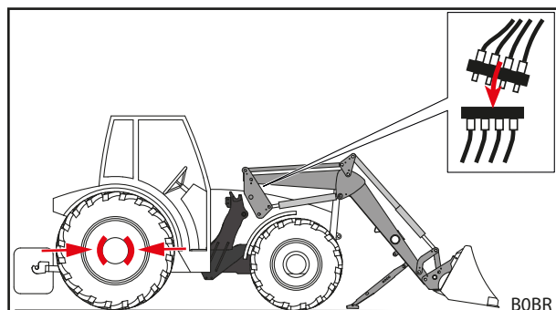
Abb. 104 Hydraulik abkoppeln
