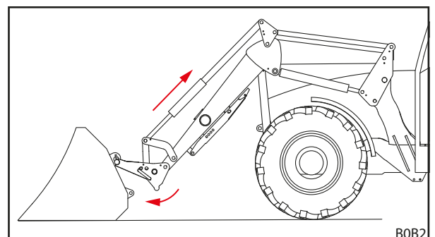
Abb. 75 Einhängen
