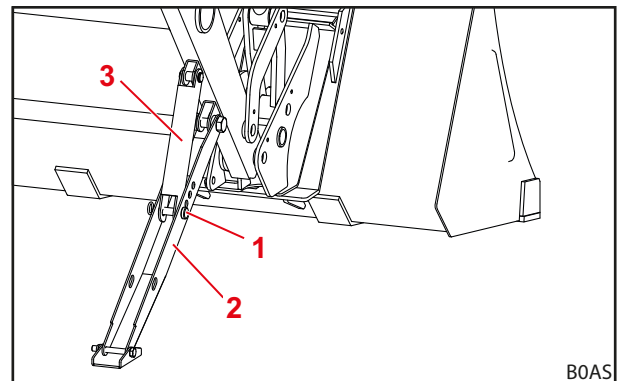
Abb. 52 Abstellstütze ausgeklappt
