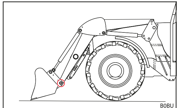
Abb. 89 Untere Bolzen herausziehen
