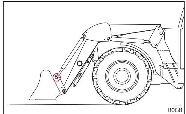
Abb. 88 Obere Bolzen herausziehen
