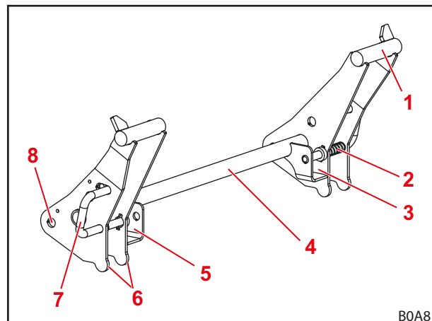
Abb. 64 Werkzeug-Verriegelung am Euro-Wechselrahmen
