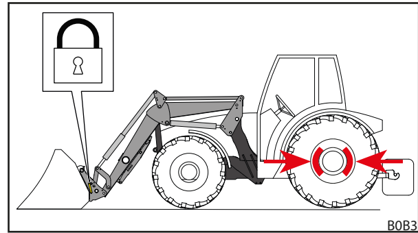
Abb. 76 Werkzeug-Verriegelung schließen
