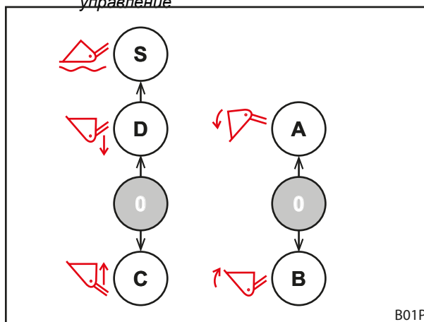
Фиг. 63 Разпределение при 2 лоста за управление
