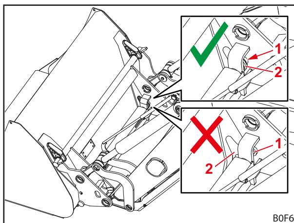
Фиг. 90 Проверка на положението на заключващия палец
