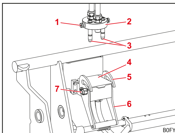
Фиг. 78 Разединено устройство за фиксиране на инструмента
