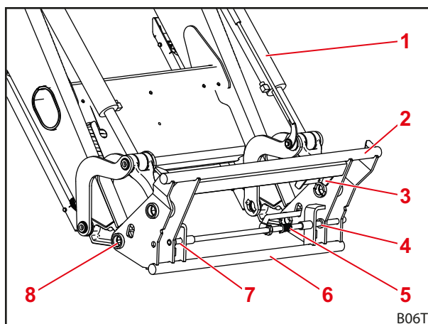
Фиг. 10 Сменна рама Euro
