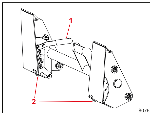
Фиг. 15 Сменна рама Skid-Steer
