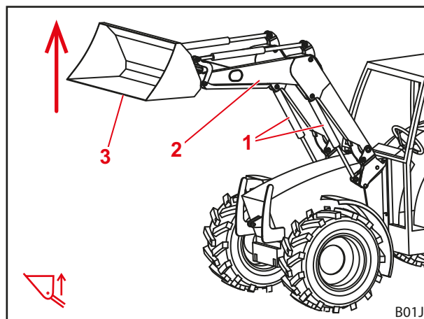
Фиг. 27 Функция повдигане
