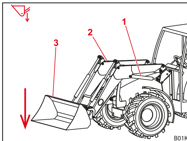
Фиг. 28 Функция спускане
