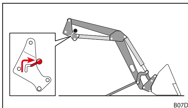
Фиг. 47 Отваряне на заключването на предния товарач
