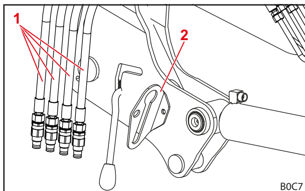
Фиг. 126 Окачване на хидравличните тръбопроводи в носача на теглича (изображение със съединителни муфи)
