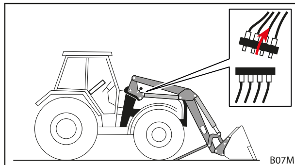
Фиг. 124 Разкачване на хидравликата
