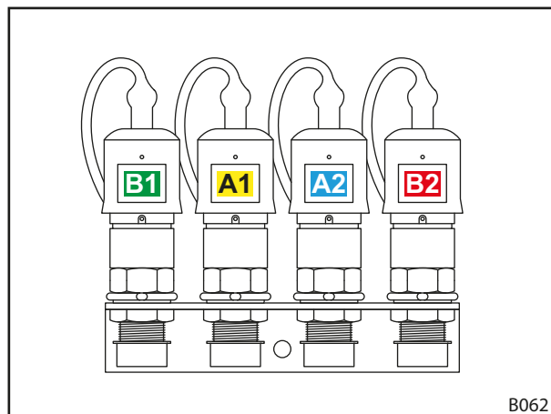
Фиг. 19 Свързване на щекерни съединители
