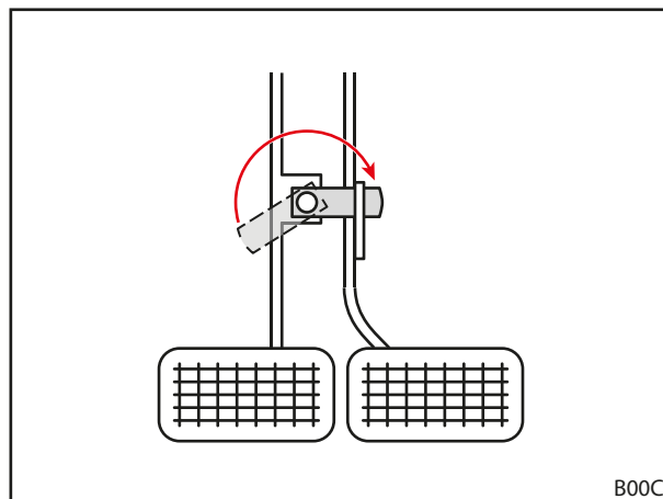
Фиг. 43 Свързване на спирачните педали
