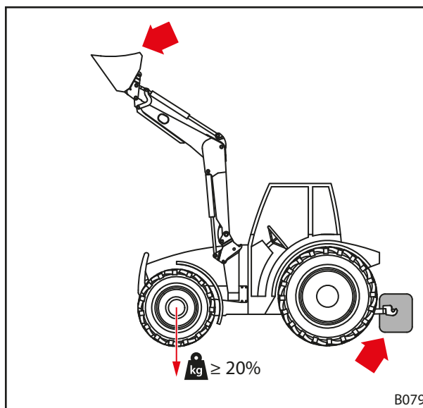
Фиг. 45 Натоварване при движение по пътища
