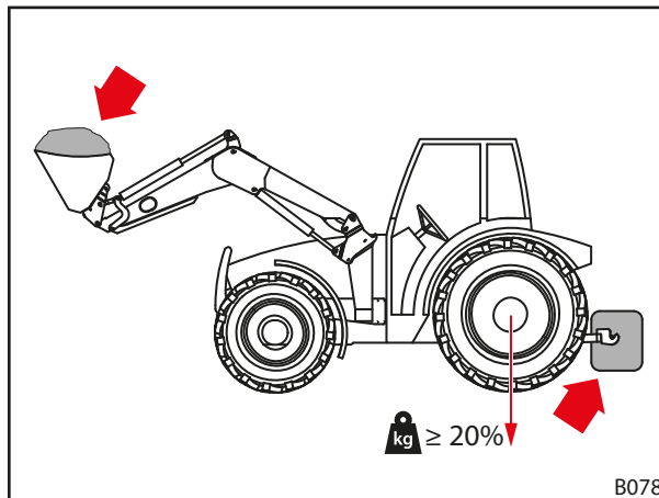
Фиг. 44 Натоварване при работи с предния товарач
