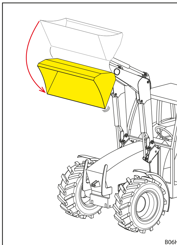
Фиг. 34 Изпразване на бърз ход, респ. бързо изпразване
