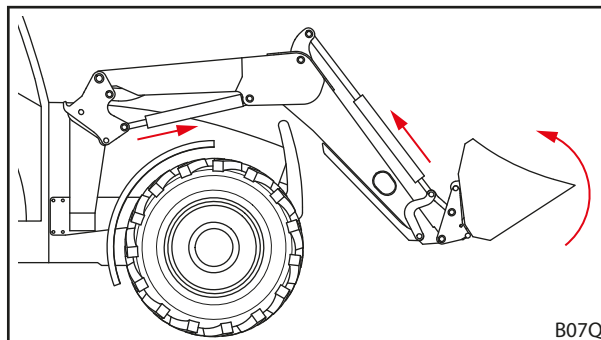
Фиг. 96 Отключване на заключването на инструмента
