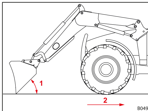
Фиг. 108 Подравняване назад
