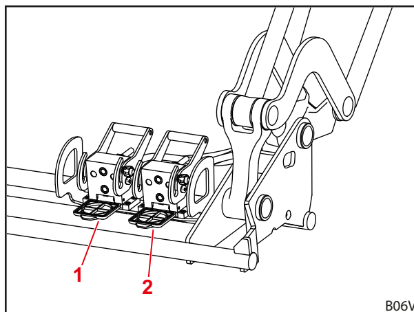
Фиг. 38 Допълнителна 4-та верига за управление
