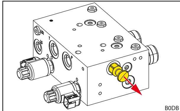
Фиг. 72 Издърпайте вентила за освобождаване на налягането REAL 3
