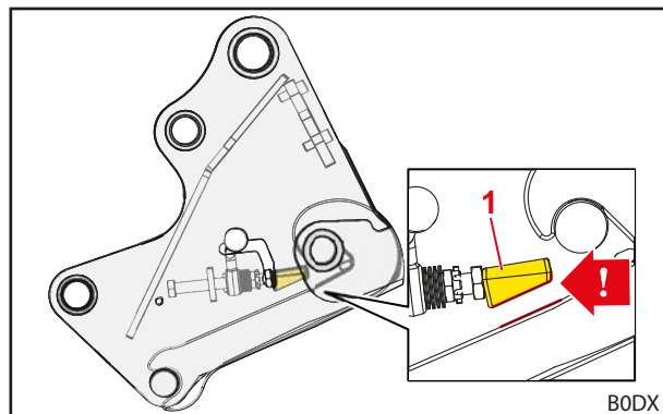
Фиг. 52 Правилно монтажно положение на затягащия клин
