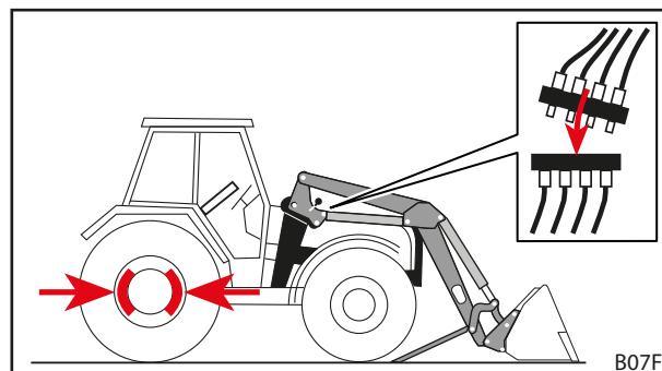
Фиг. 49 Изключване на трактора и свързване на хидравличните тръбопроводи
