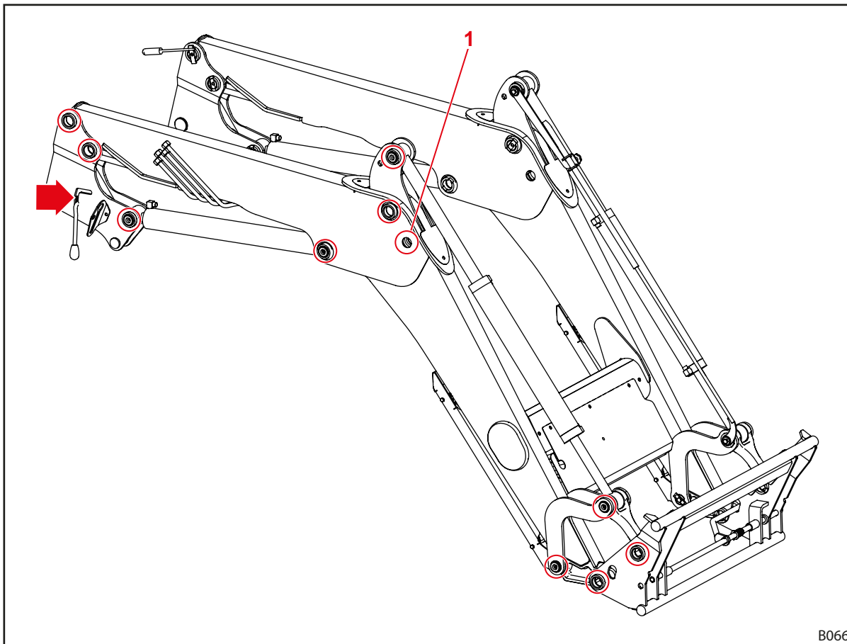
Фиг. 115 Места на смазване на FZ
