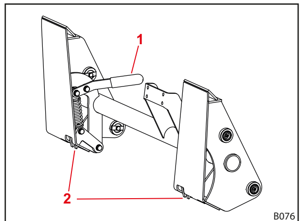
Фиг. 85 Заклучване на инструмента към сменна рама Skid-Steer
