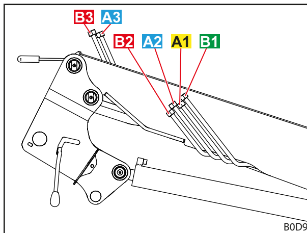
Фиг. 18 Хидравлични тръбопроводи (опция REAL 3 )
