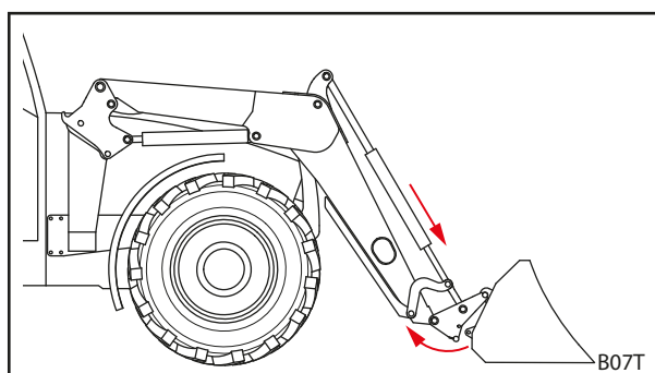
Фиг. 106 Откачване на сменната рама
