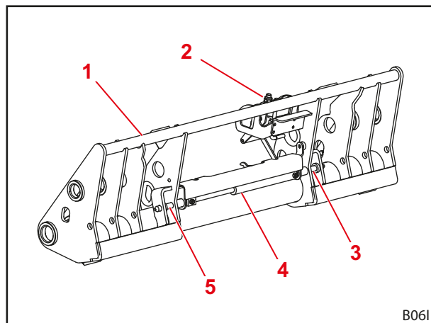
Фиг. 16 Усилена сменна рама Euro (FZ 100)
