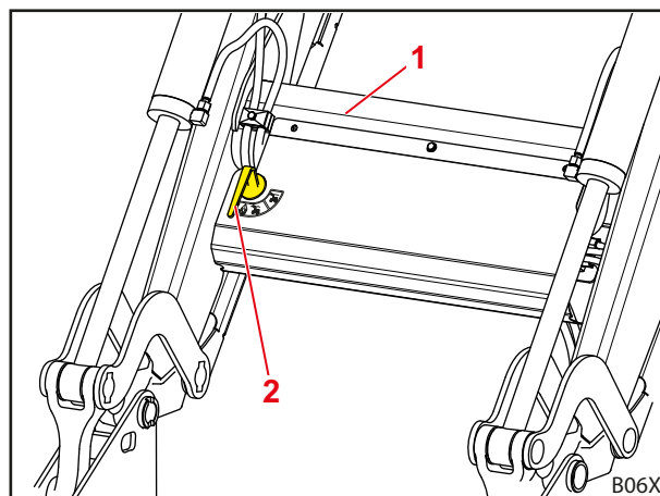
Фиг. 40 Comfort-Drive с ръчно управление
