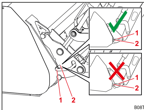
Фиг. 83 Проверка на положението на заключващия палец
