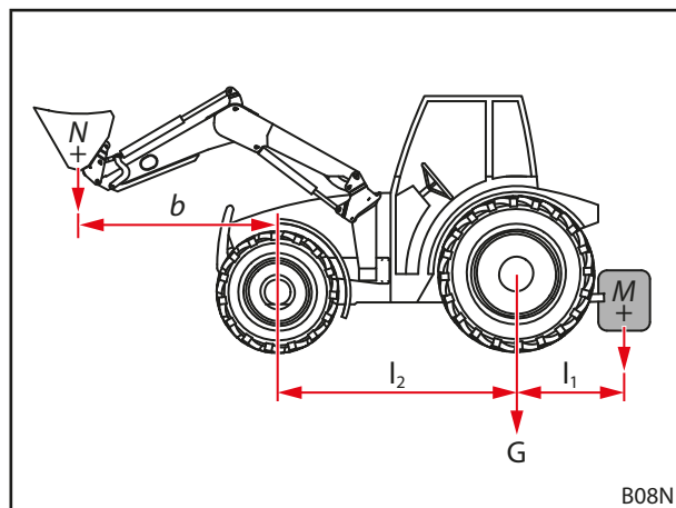
Фиг. 46 Изчисляване на статичната стабилност
