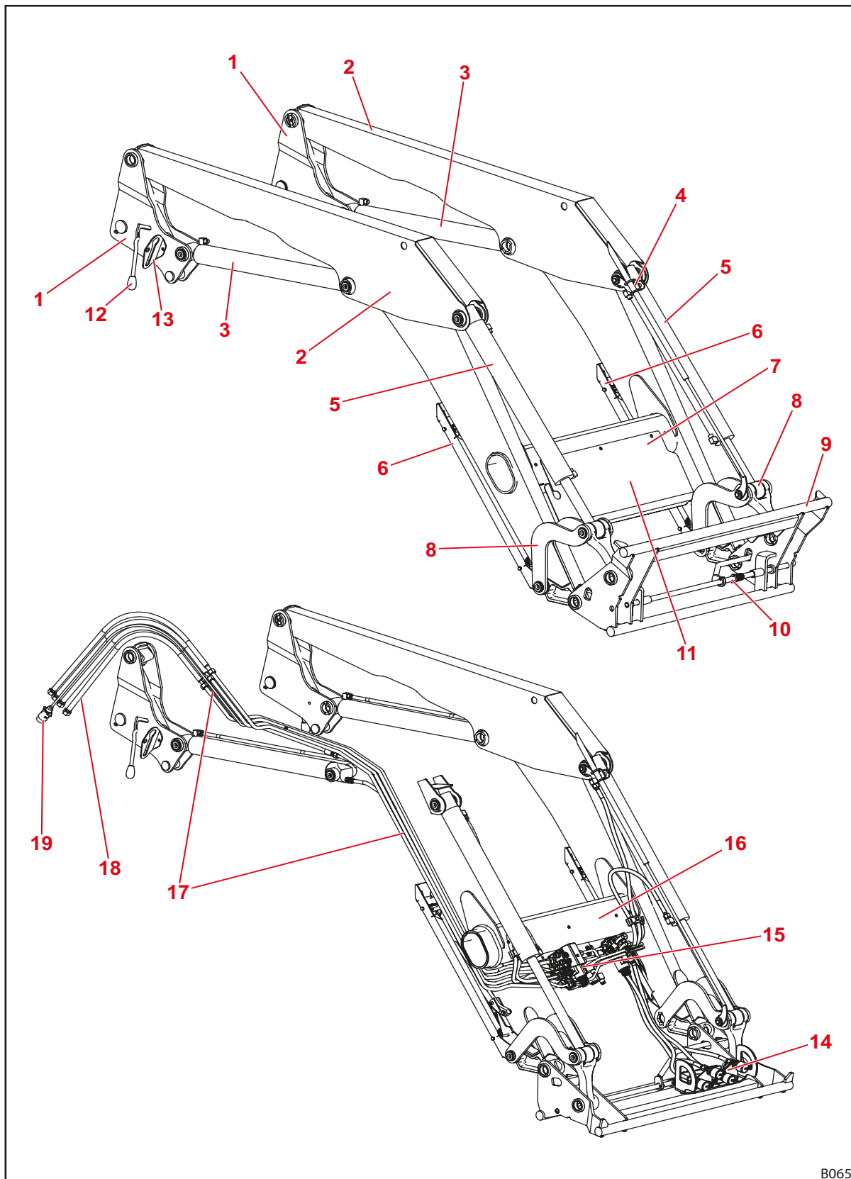
Фиг. 7 Преден товарач FS
