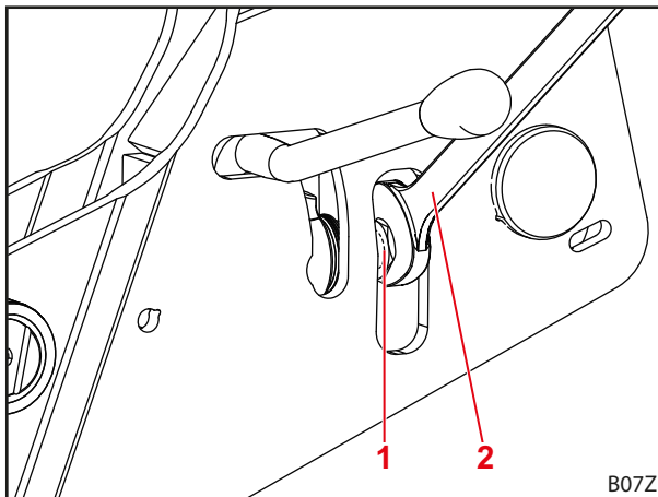
Фиг. 61 Затягане на контрагайката
