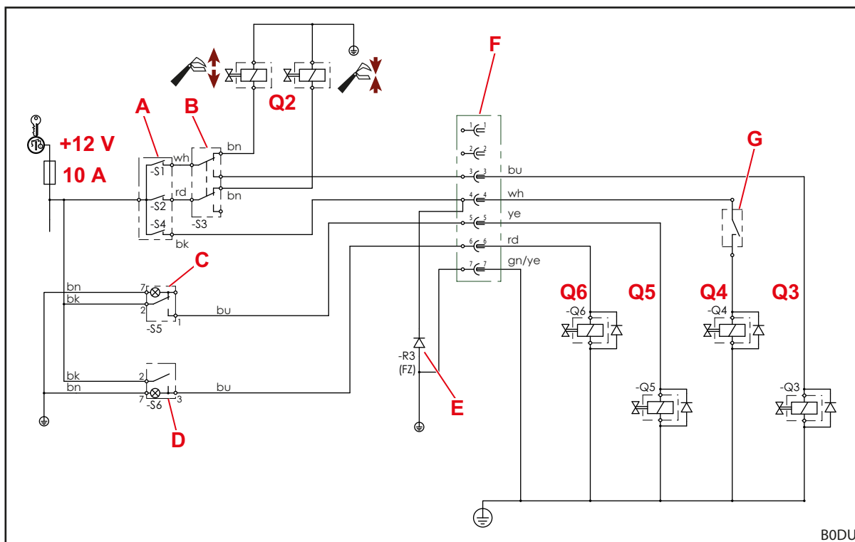
Фиг. 132 Електрическа схема (при оборудване с REAL 3 )
