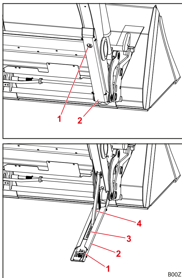
Фиг. 74 Опора за паркиране
