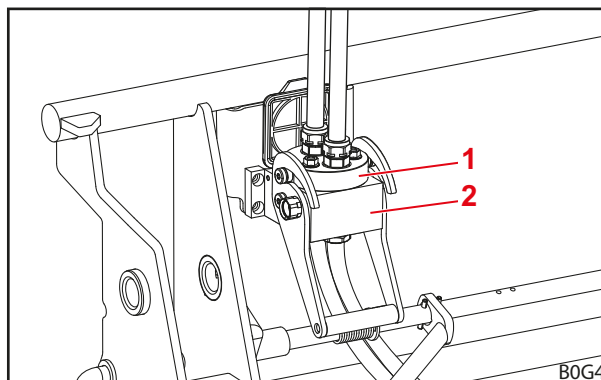
Фиг. 79 Свързано устройство за фиксиране на инструмента
