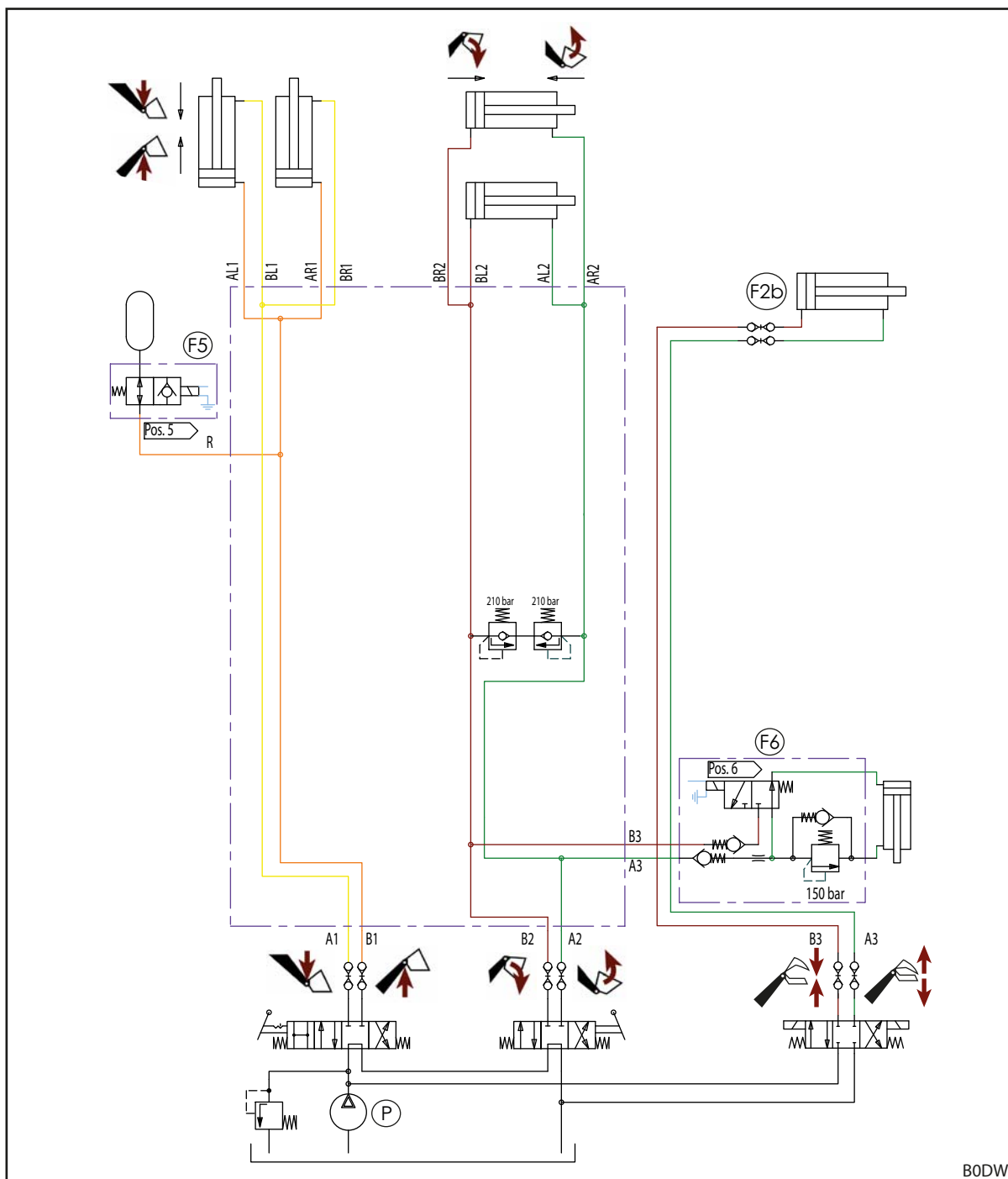
Фиг. 128 Хидравлична схема FS (при оборудване с REAL 3 )
