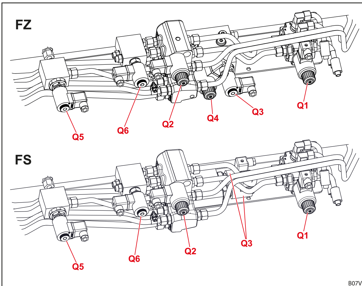
Фиг. 133 Разположение на хидравличните вентили за допълнителни функции
