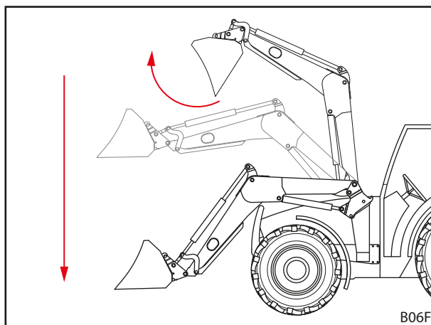
Фиг. 35 Функция връщане към нивото
