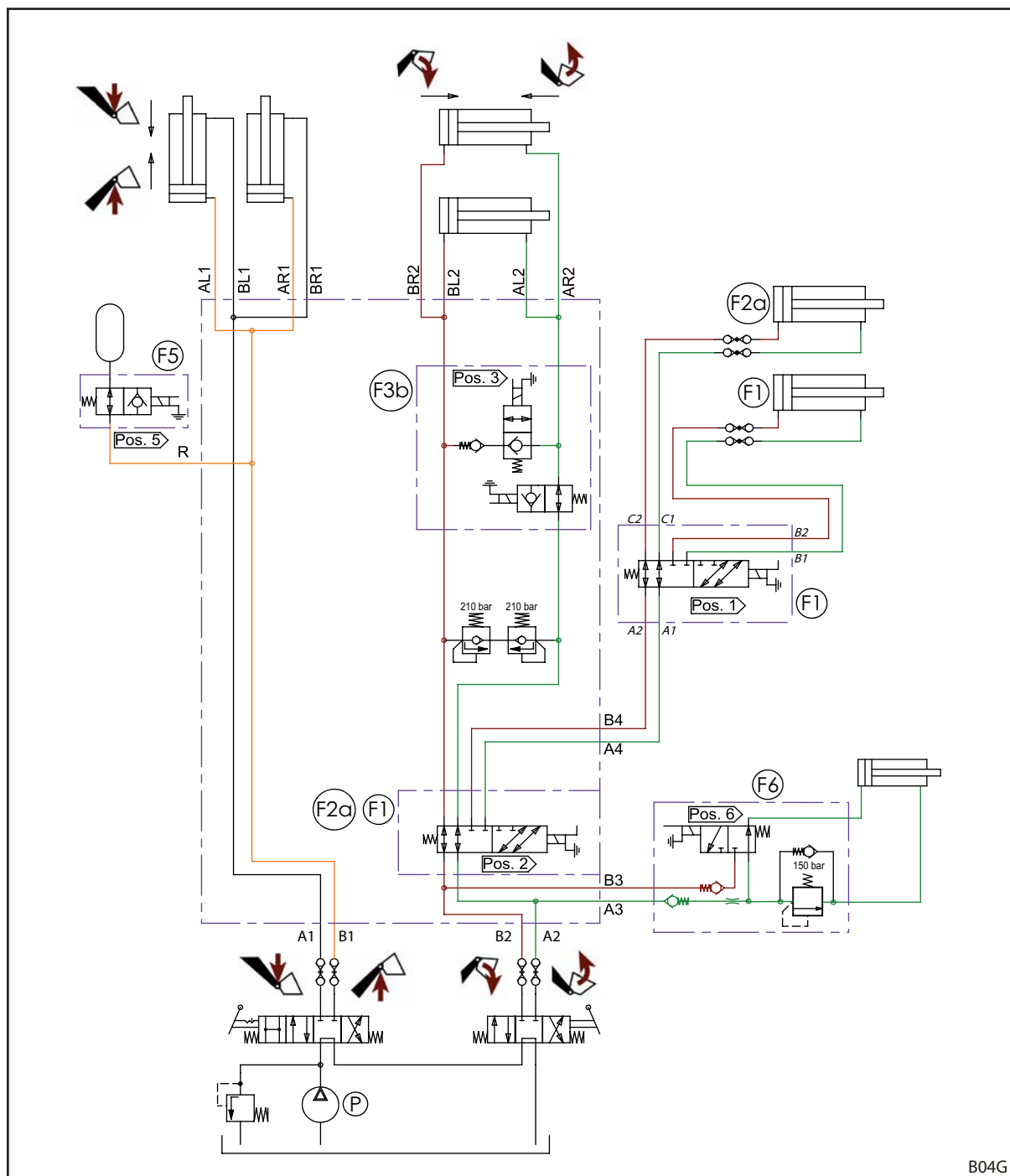
Фиг. 127 Хидравлична схема FS и FS-бърз ход (при оборудване с 3-та и 4-та верига за управление)
