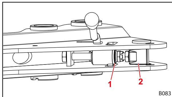
Фиг. 60 Изглед на заключването на предния товарач отдолу
