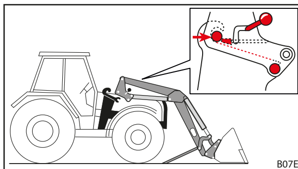
Фиг. 48 Прибиране на трактора в стрелата
