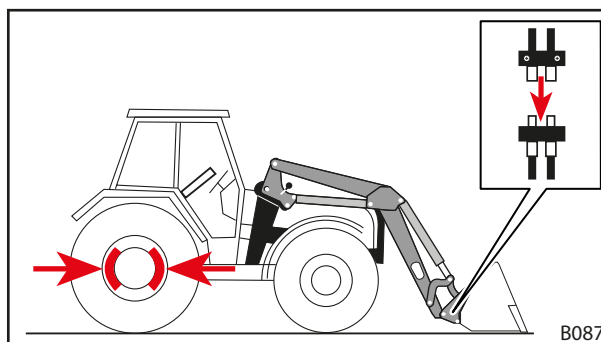
Фиг. 97 Свързване на хидравличните тръбопроводи на инструмента със съединителите на предния товарач
