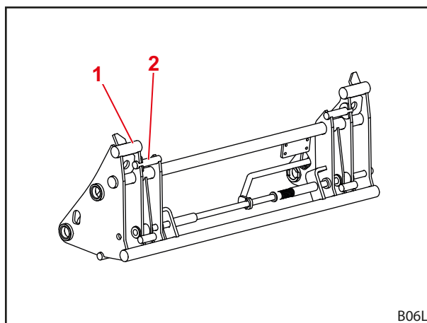
Фиг. 13 Комбинирана сменна рама Euro-Alö3
