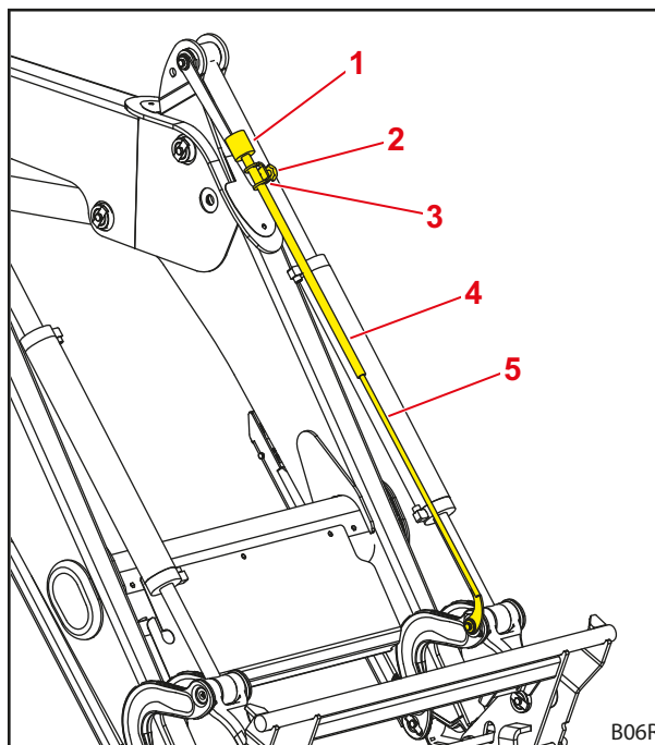
Фиг. 36 Сензор за връщане към нивото на визуалната индикация
