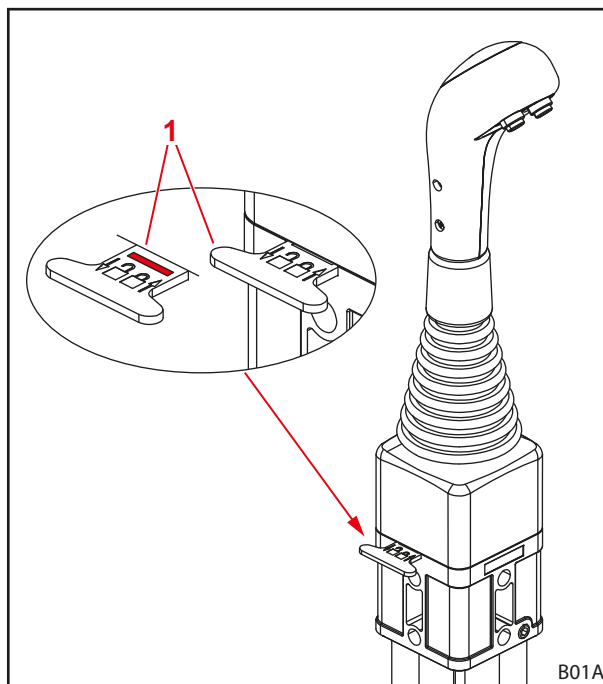
Фиг. 65 Блокировка на лоста за управление
