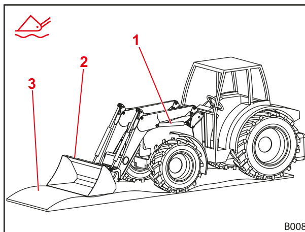
Фиг. 31 Преден товарач в плаващо положение
