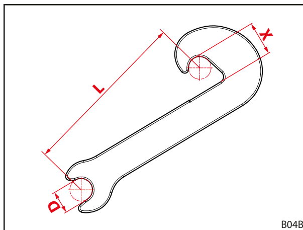
Фиг. 116 Размери на износването на захващащите куки
