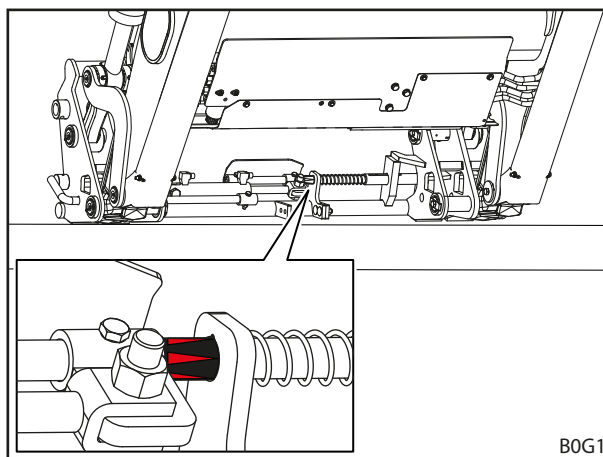
Фиг. 88 Проверка на заключването на инструмента с помощта на стикера
