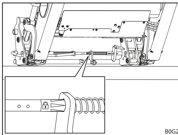
Фиг. 82 Проверка на заключването на инструмента с помощта на стикера (комбинирана сменна рама Euro-FR)
