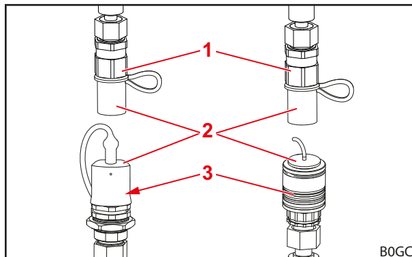
Фиг. 75 Щекерни съединители (примерни изображения)
