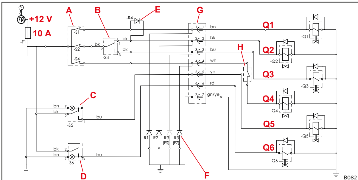
Фиг. 131 Електрическа схема (при оборудване с 3-та и 4-та верига за управление)
