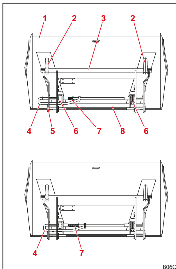
Фиг. 25 Отворено (горе) и затворено (долу) заключване
