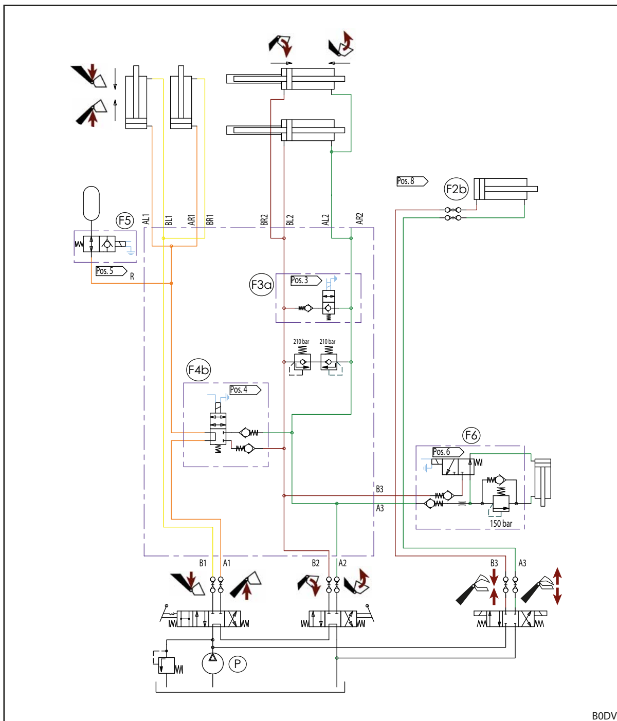
Фиг. 130 Хидравлична схема FZ и FZ-L (при оборудване с REAL 3 )
