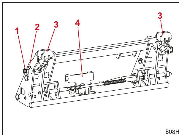
Фиг. 14 Комбинирана сменна рама Euro-FR
