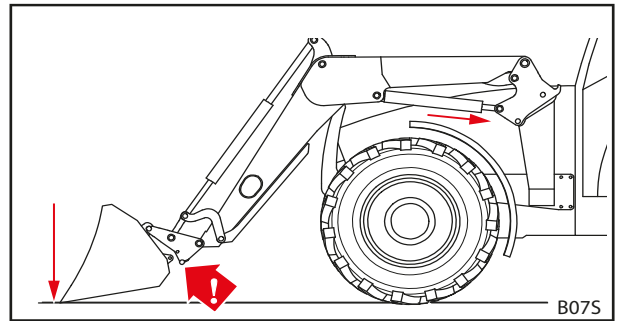
Фиг. 84 Притискане на инструмента към земята
