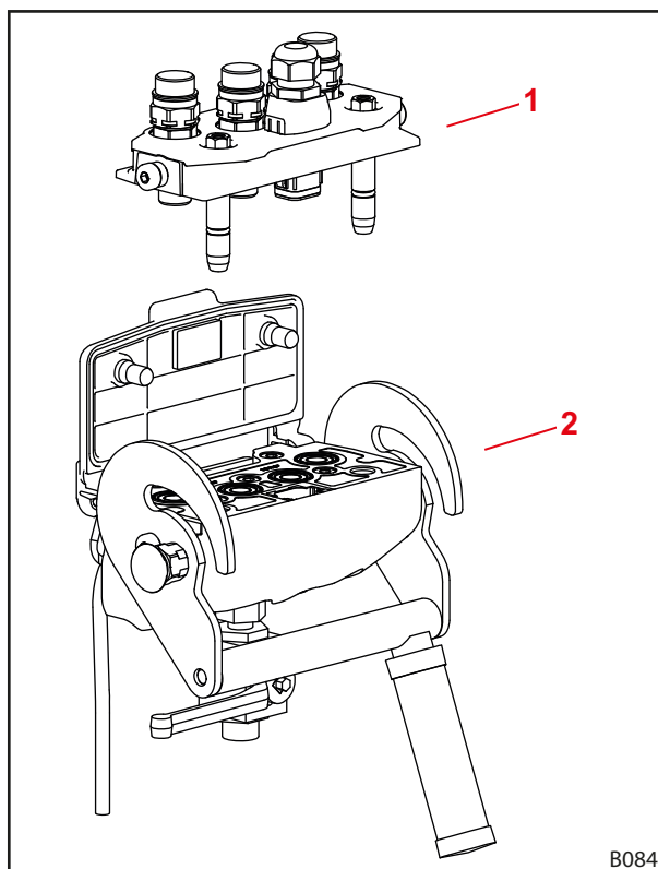
Фиг. 22 Конструкция Hydro-Fix
